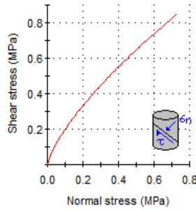
Şekil 7.19 : Kuvarsit birimi için yerinde jeomekanik büyüklükler.
