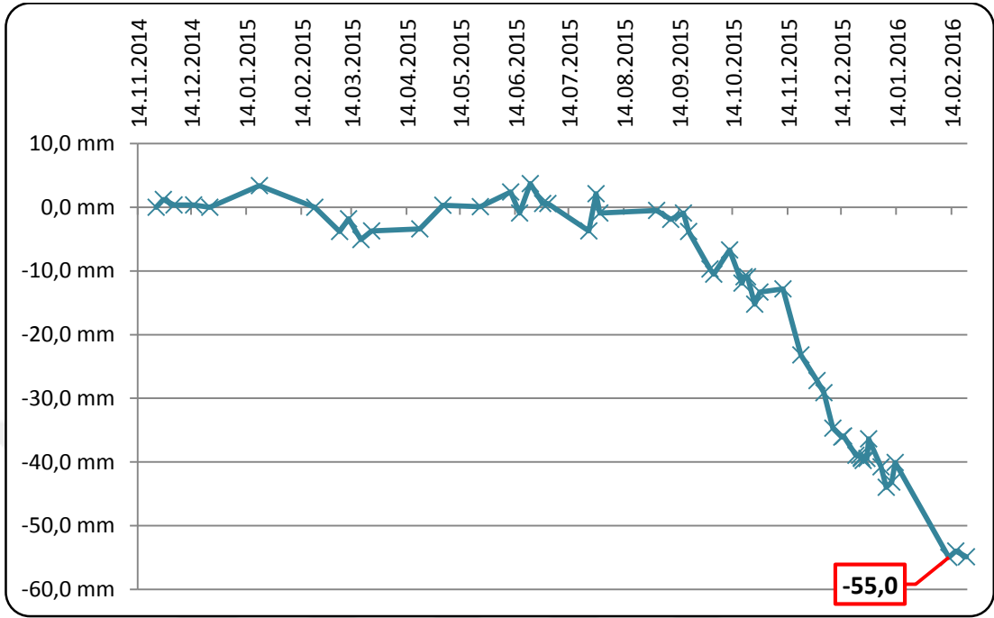
Şekil C.5 : RS2 noktasına ait zamana bağlı nivelman ölçüm sonuçları
