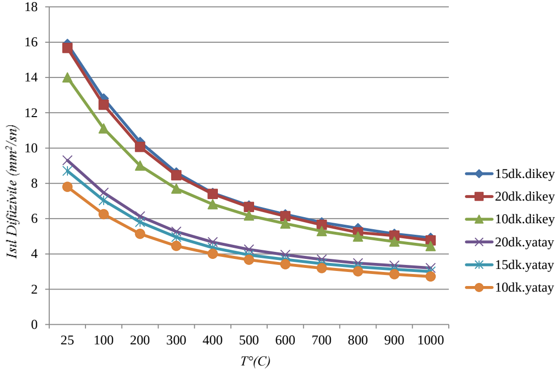
Şekil 4.27. % 4 GNP ilaveli Sonikasyon işleminden geçirilmiş numunelerin 1875°C’de 10-15-20 dk. süreyle sinterlenmesi sonrasında elde edilen yatay ve dikey ısıl difüzivite sonuçları
