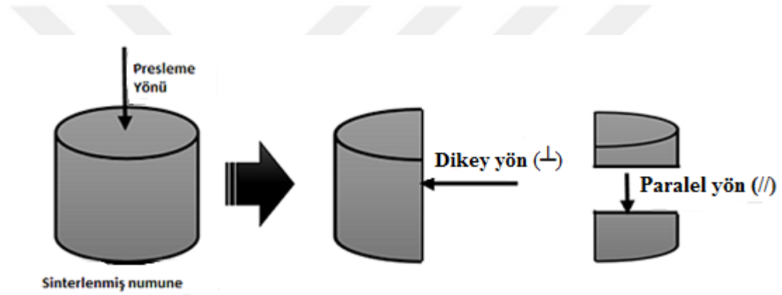
Şekil 3.4 Numunelerin kesilme ve inceleme yönü
