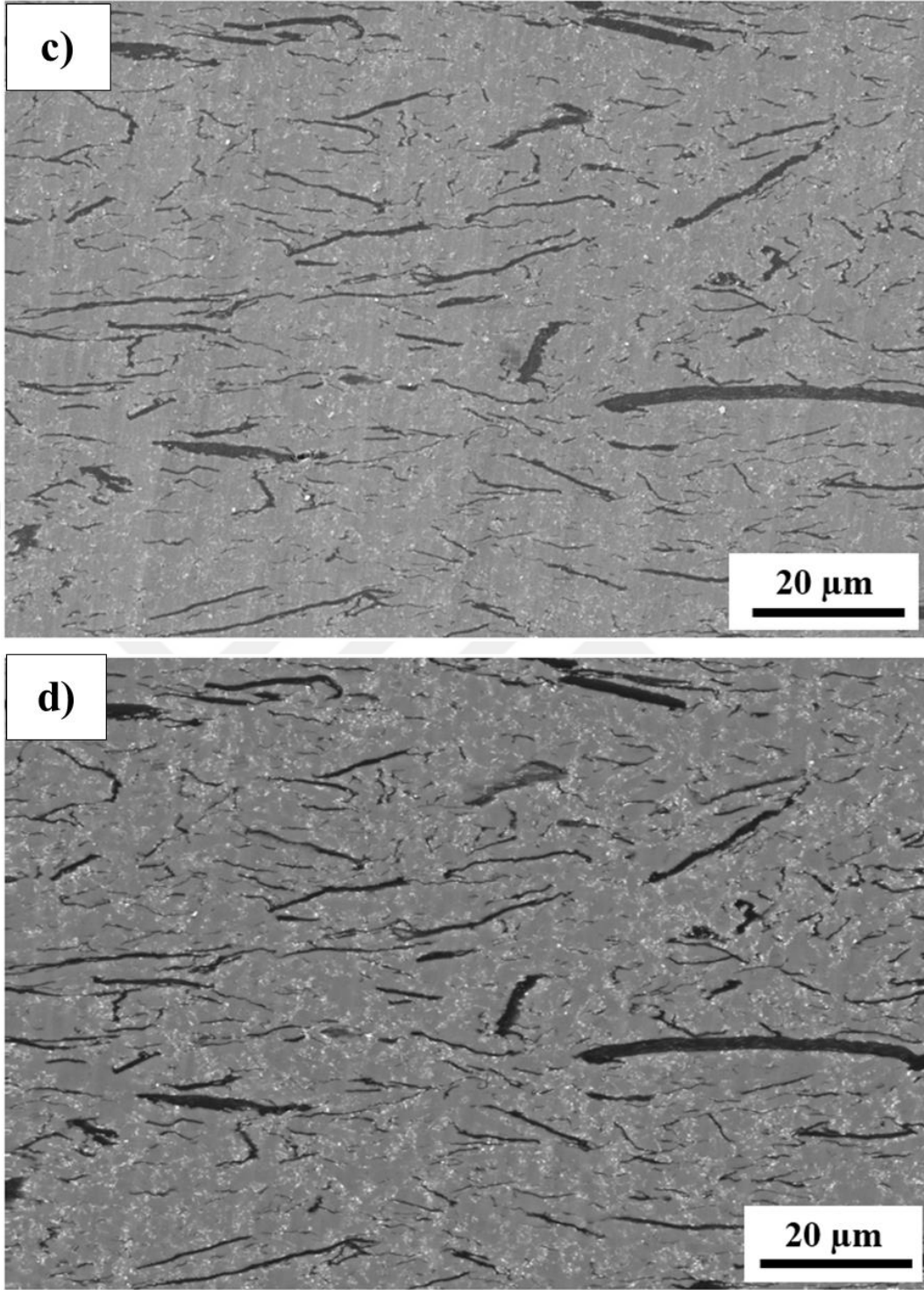
Şekil 4.5. % 8 GNP katkılı SiAlON matris kompozitin dikey yüzeyinden CP ile elde edilmiş (c) SE ve (d) BSE görüntüleri.
