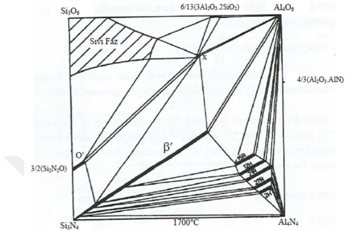
Şekil 2.6. \text{Si}_3\text{N}_4\text{-AlN-SiO}_2\text{-Al}_2\text{O}_3 sisteminin 1700^\circ\text{C} 'deki faz diagramı
