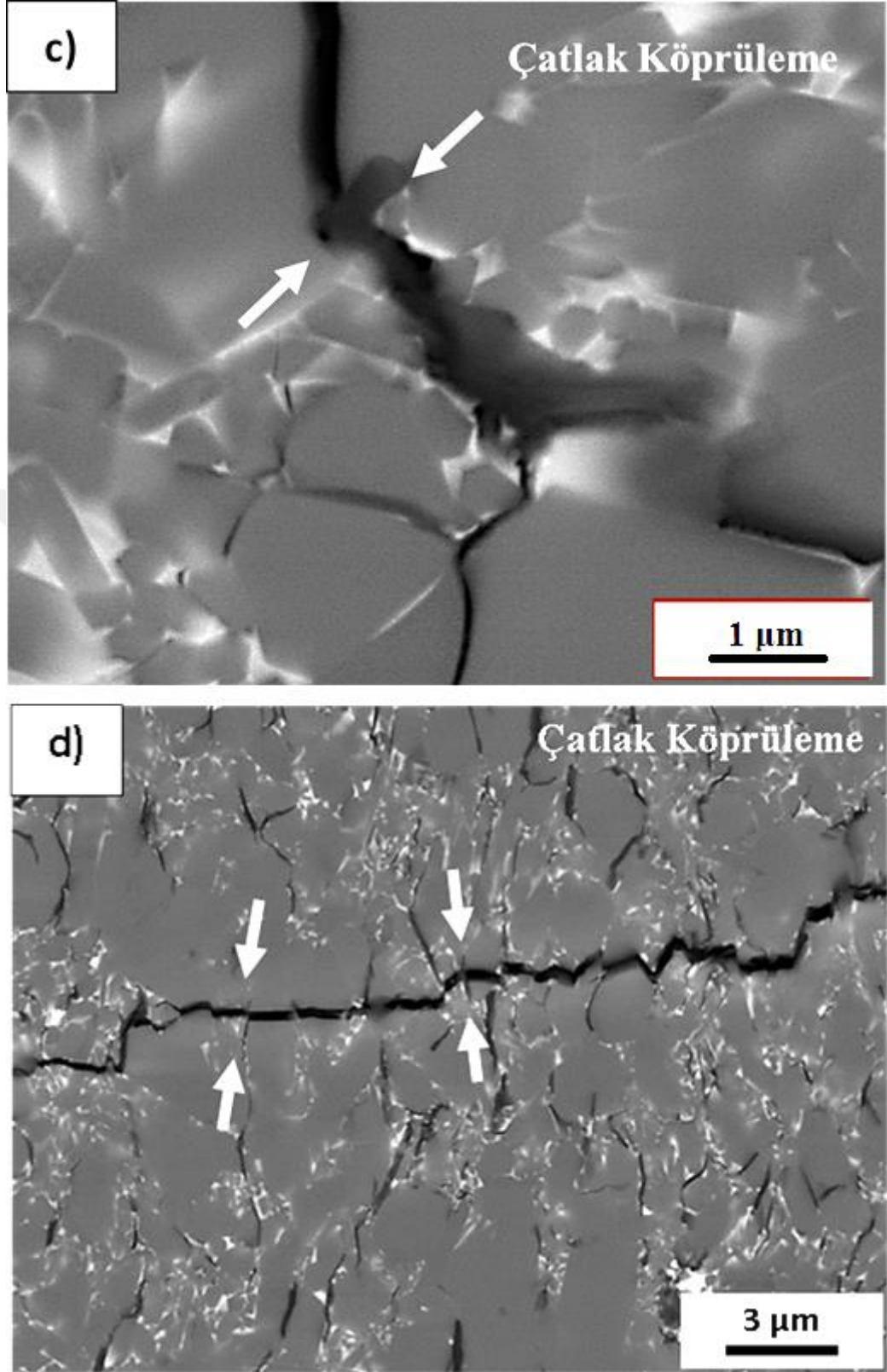
Şekil 4.19. (devam)(a-c) Sonikasyon, (b-d) Mikroakışkanlaştırıcı ile hazırlanmış %4 GNP katkılı SiAlON matris kompozitlerinin toklaştırma mekanizmaları
