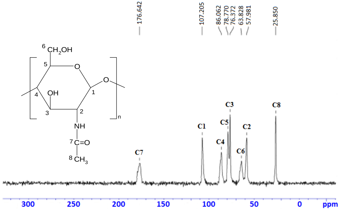
Şekil 4.2. Kitine ilişkin ^{13}\text{C} CP/MAS NMR spektrumu
