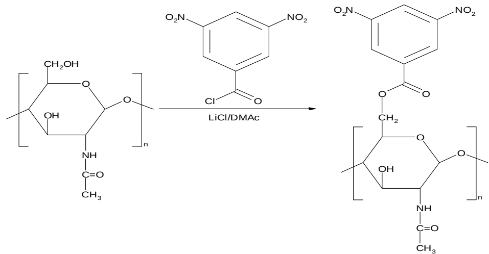
Şekil 3.1. K35DK maddesinin oluşum tepkimesi
