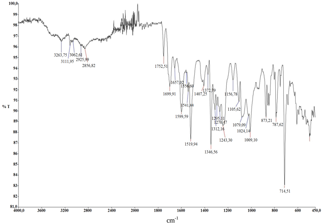
Şekil 4.19. K4NK maddesine ilişkin FT-IR spektrumu
