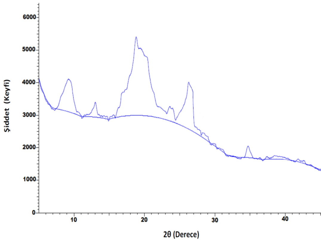
Şekil 4.21. K4NK maddesine ilişkin XRD spektrumu
