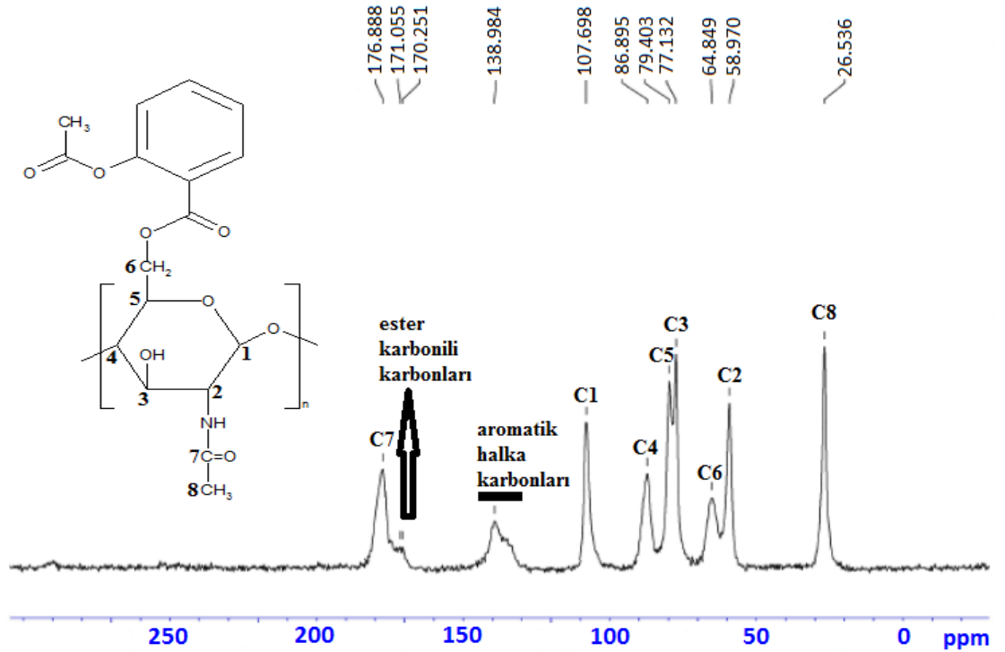
Şekil 4.26. KOAK maddesine ilişkin 13 C CP/MAS NMR spektrumu
