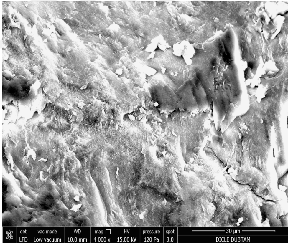
Şekil 4.10. K35DK maddesine ilişkin SEM görüntüsü
