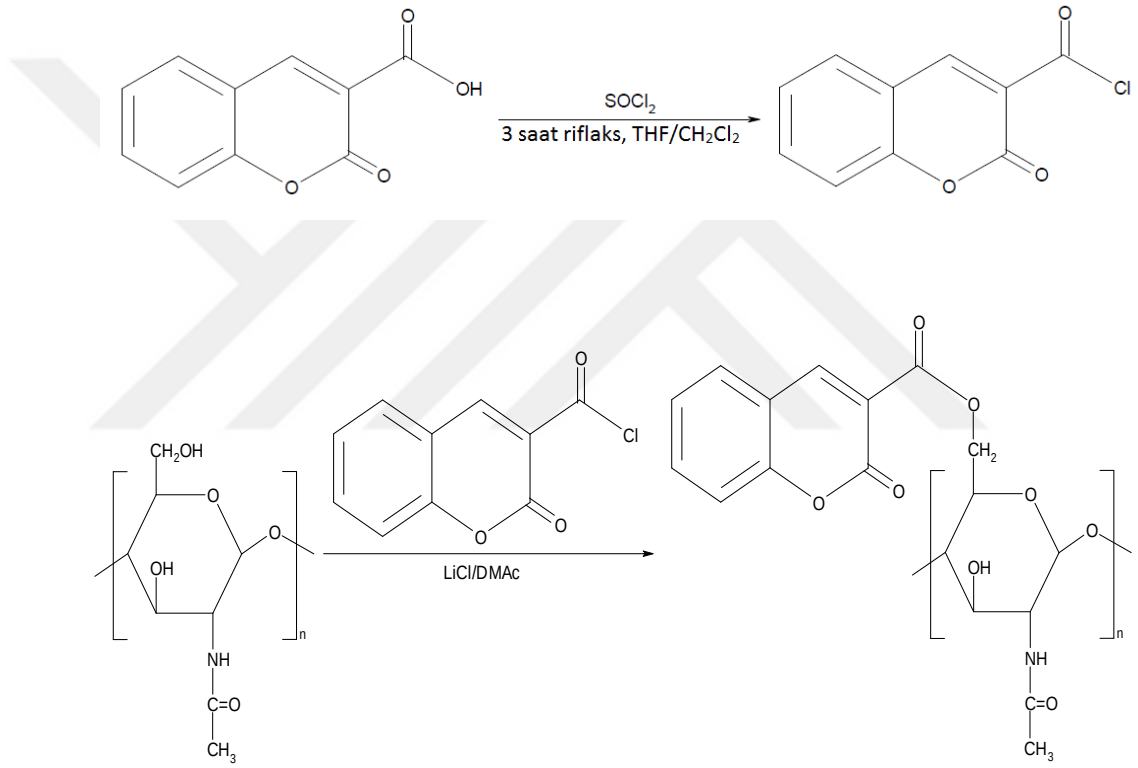
Şekil 3.8. KK3KA maddesinin oluşum tepkimesi
