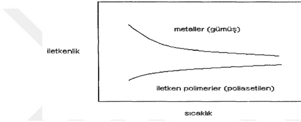
Şekil 1.4. İletken polimerlerin ve metallerin iletkenliklerinin sıcaklıkla değişimi
