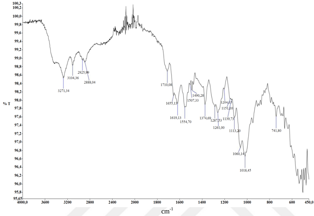
Şekil 4.31. KFD maddesine ilişkin FT-IR spektrumu
