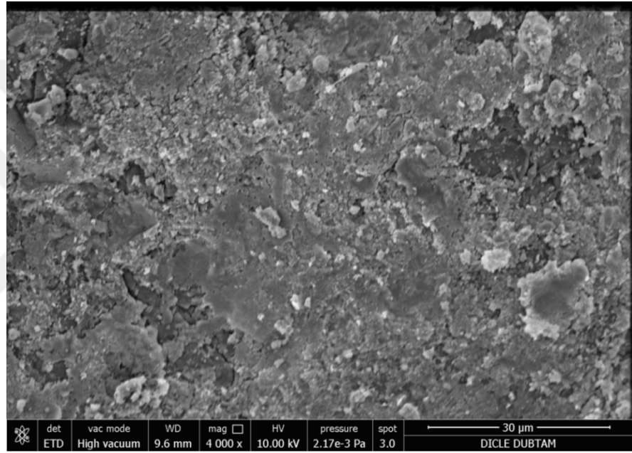
Şekil 4.4. Kitine ilişkin SEM görüntüsü
