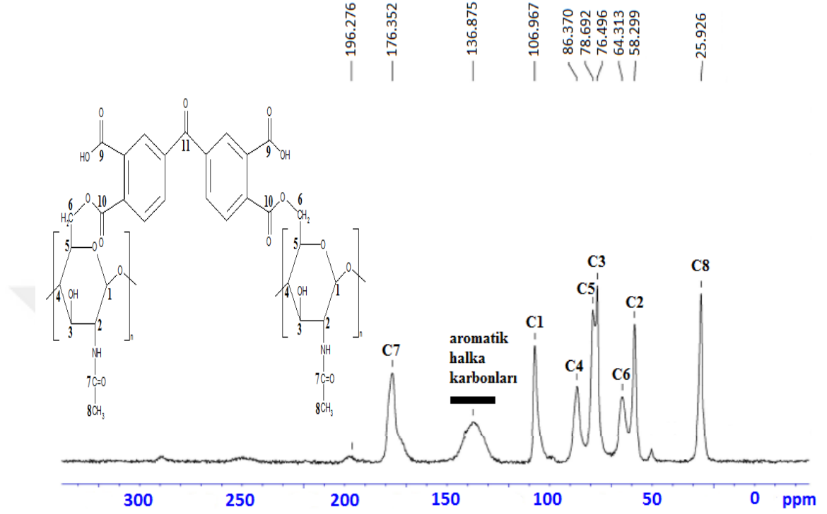
Şekil 4.44. KB33'44'TD maddesine ilişkin ^{13}\text{C} CP/MAS NMR spektrumu
