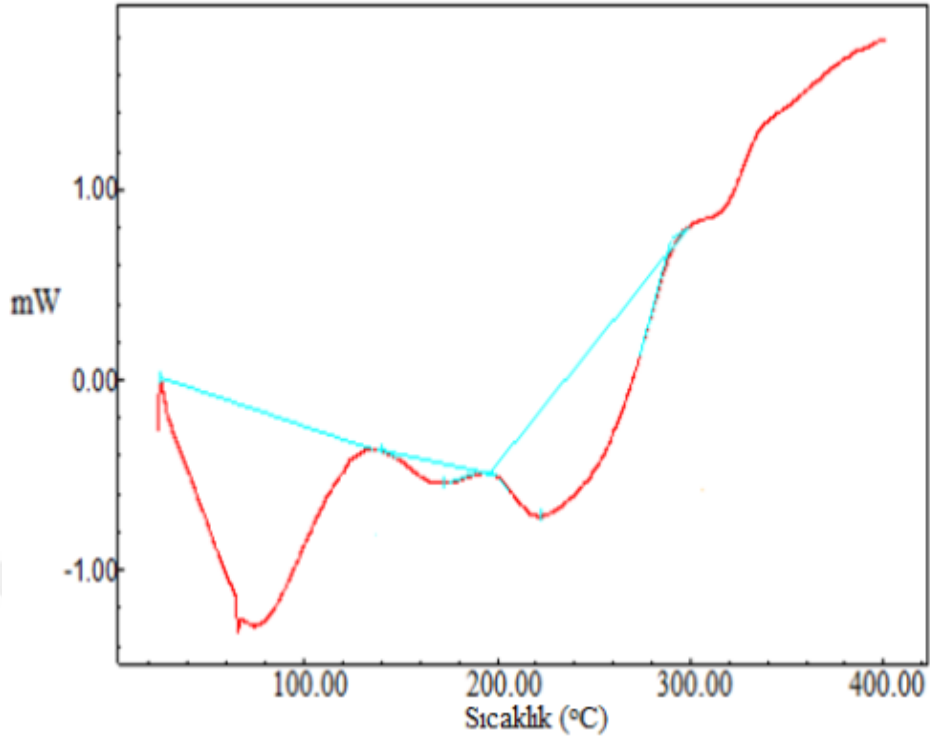
Şekil 4.18. K45DA maddesine ilişkin DSC eğrisi
