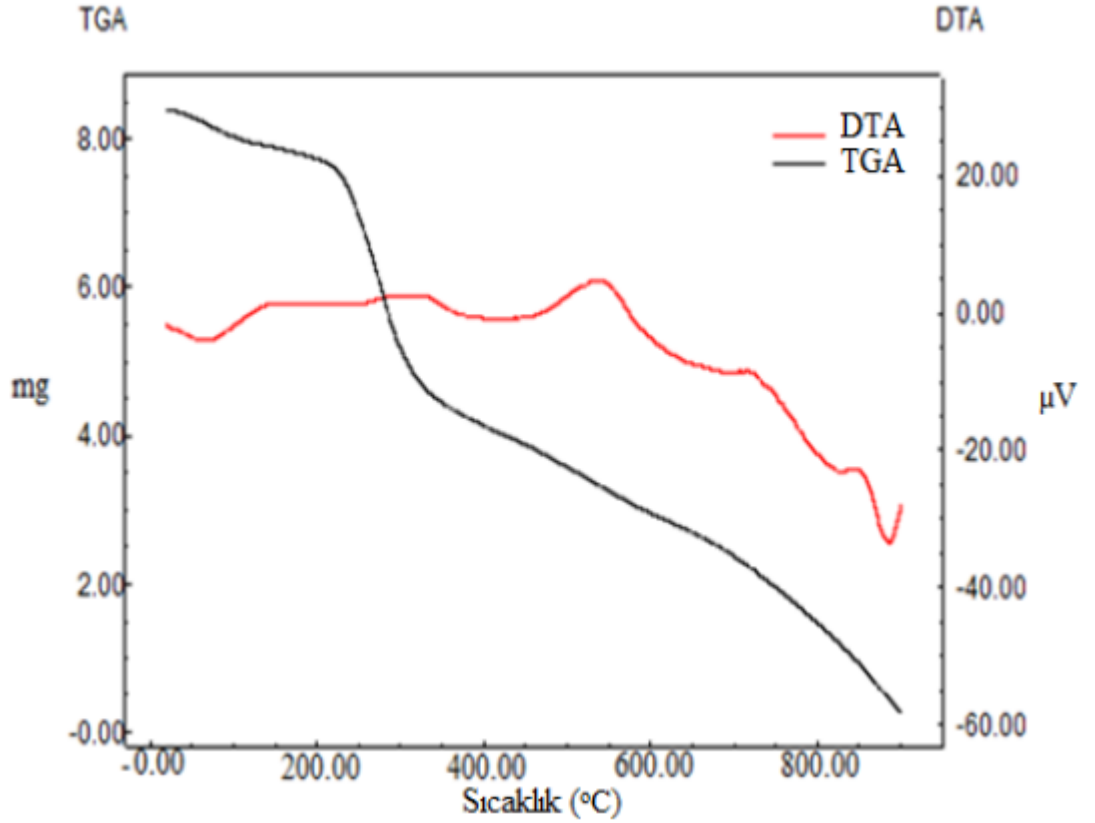
Şekil 4.47. KB33'44'TD maddesine ilişkin TGA ve DTA eğrileri
