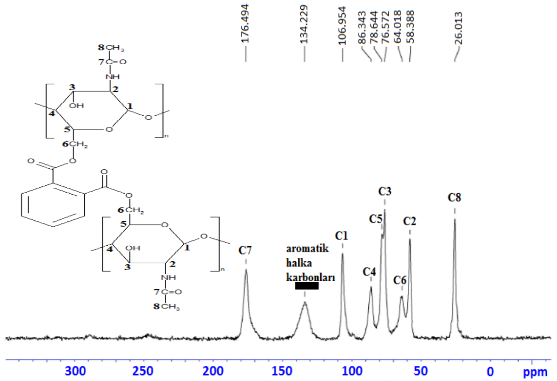
Şekil 4.32. KFD maddesine ilişkin ^{13}\text{C} CP/MAS NMR spektrumu
