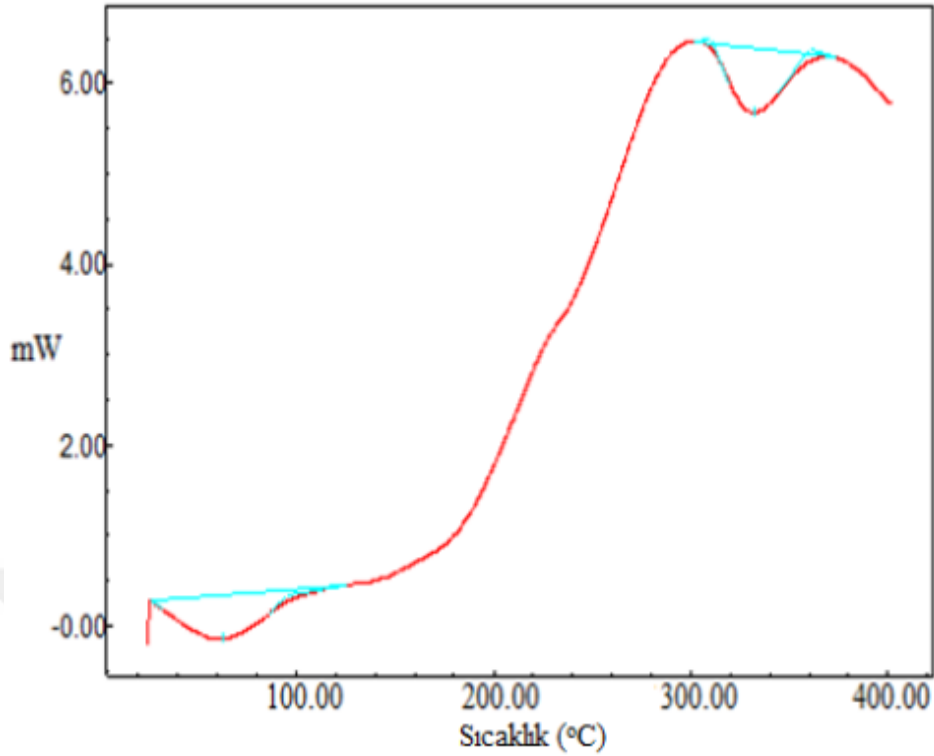
Şekil 4.12. K35DK maddesine ilişkin DSC eğrisi
