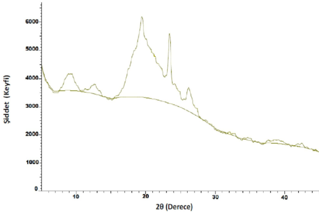
Şekil 4.9. K35DK maddesine ilişkin XRD spektrumu
