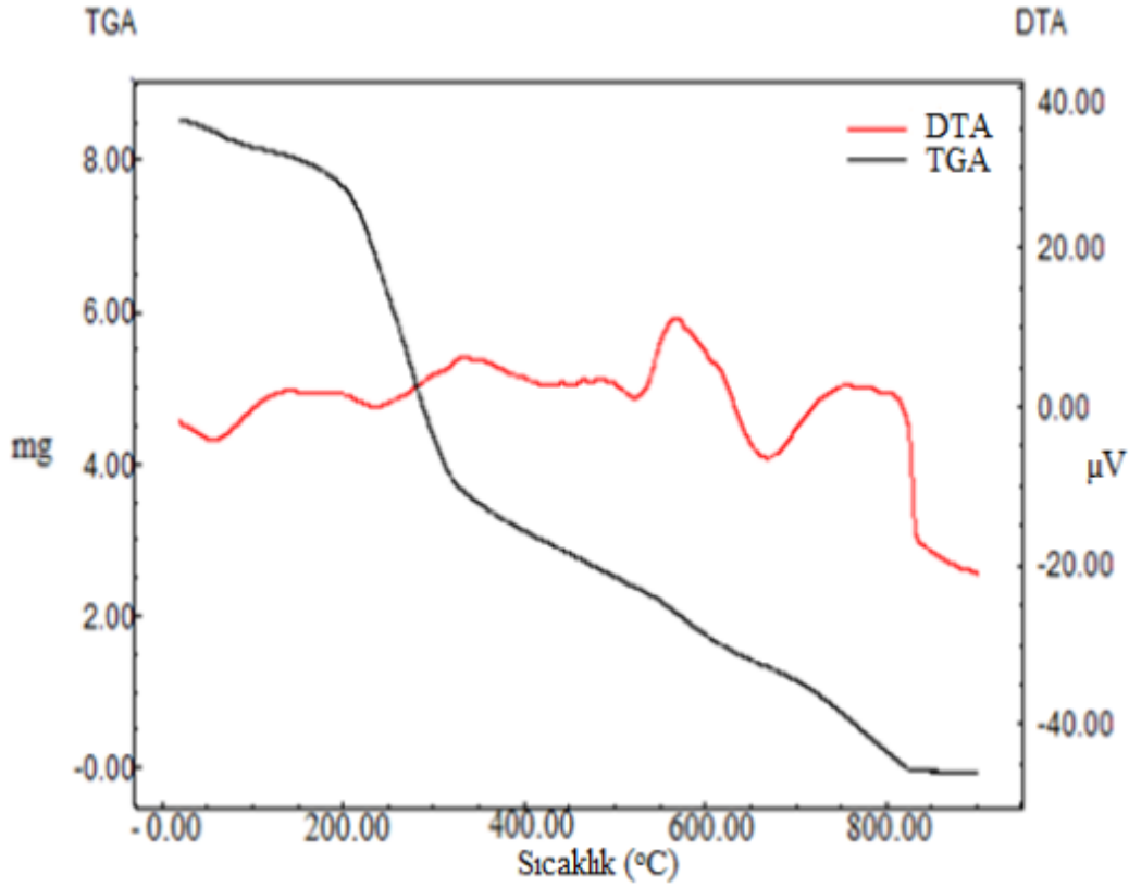
Şekil 4.17. K45DA maddesine ilişkin TGA ve DTA eğrileri
