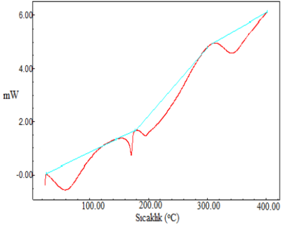
Şekil 4.24. K4NK maddesine ilişkin DSC eğrisi
