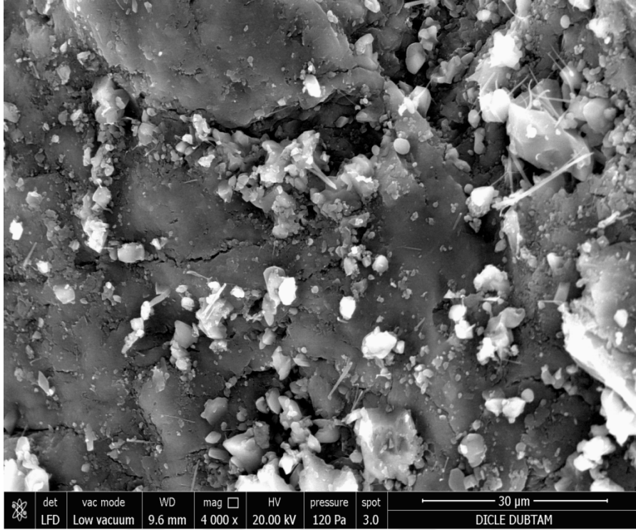
Şekil 4.52. KK3KA maddesine ilişkin SEM görüntüsü
