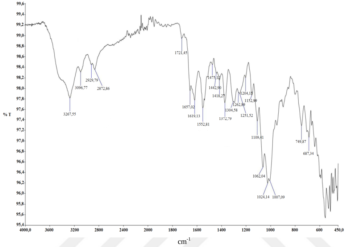
Şekil 4.37. KDA maddesine ilişkin FT-IR spektrumu
