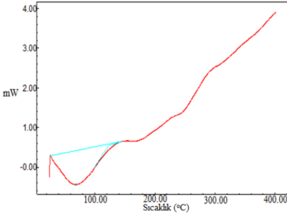
Şekil 4.48. KB33'44'TD maddesine ilişkin DSC eğrisi
