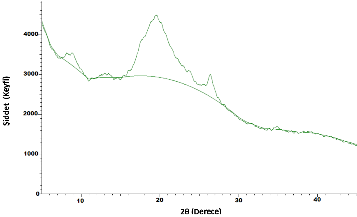
Şekil 4.33. KFD maddesine ilişkin XRD spektrumu
