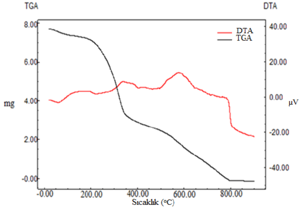
Şekil 4.41. KDA maddesine ilişkin TGA ve DTA eğrileri
