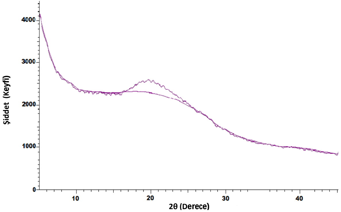
Şekil 4.51. KK3KA maddesine ilişkin XRD spektrumu
