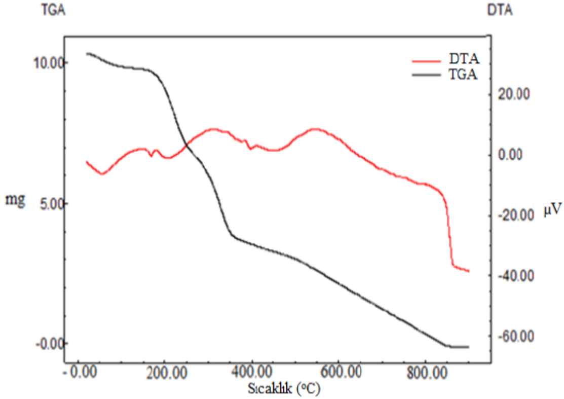
Şekil 4.23. K4NK maddesine ilişkin TGA ve DTA eğrileri
