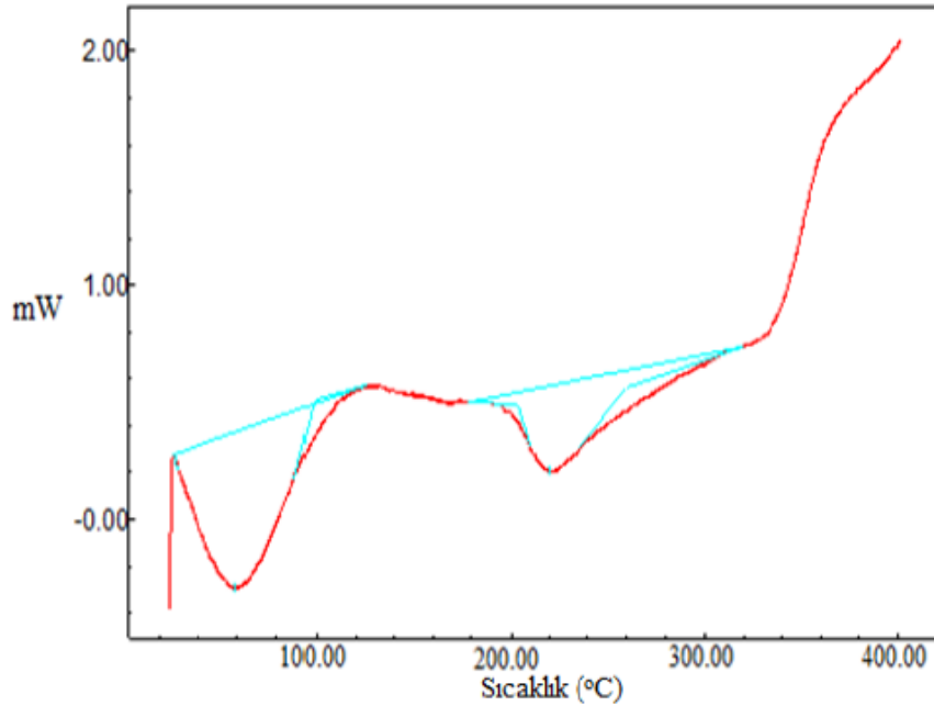
Şekil 4.42. KDA maddesine ilişkin DSC eğrisi
