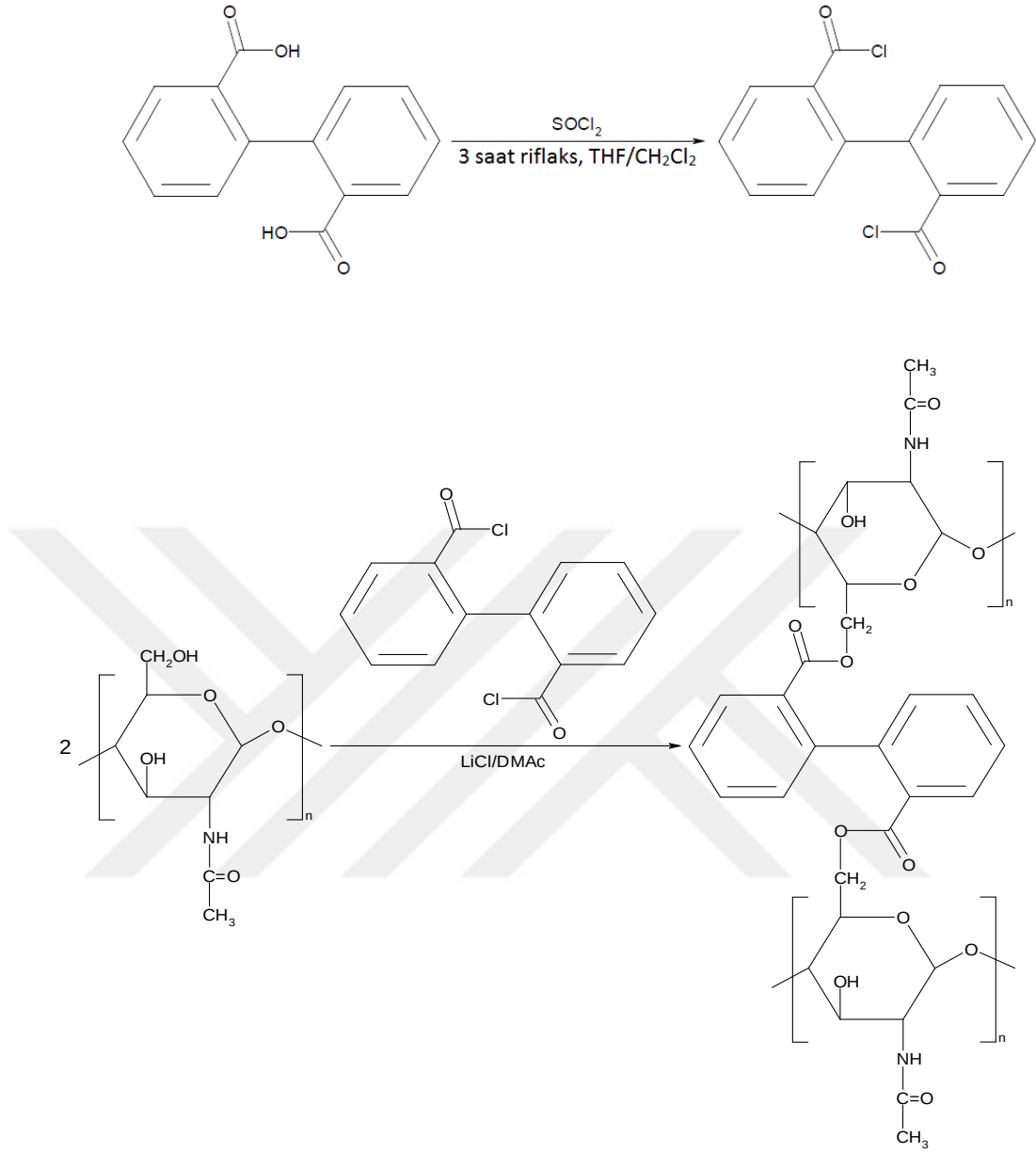
Şekil 3.6. KDA maddesinin oluşum tepkimesi
