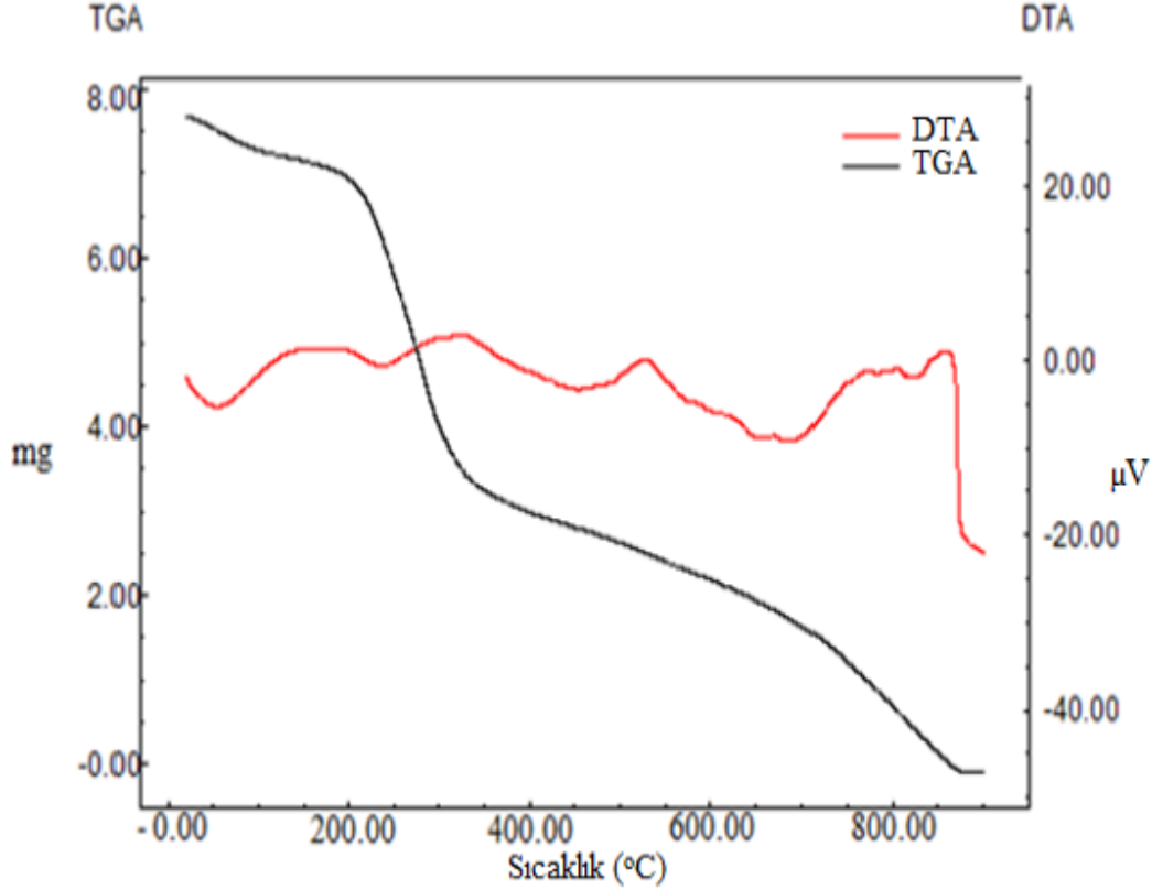
Şekil 4.35. KFD maddesine ilişkin TGA ve DTA eğrileri
