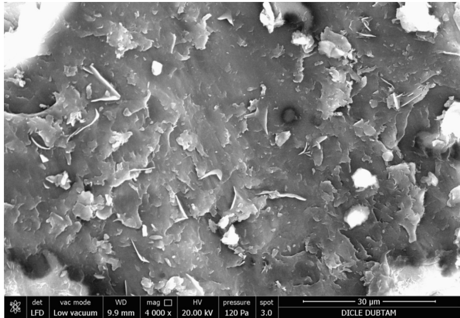
Şekil 4.16. K45DA maddesine ilişkin SEM görüntüsü
