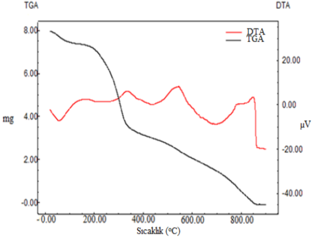
Şekil 4.29. KOAK maddesine ilişkin TGA ve DTA eğrileri
