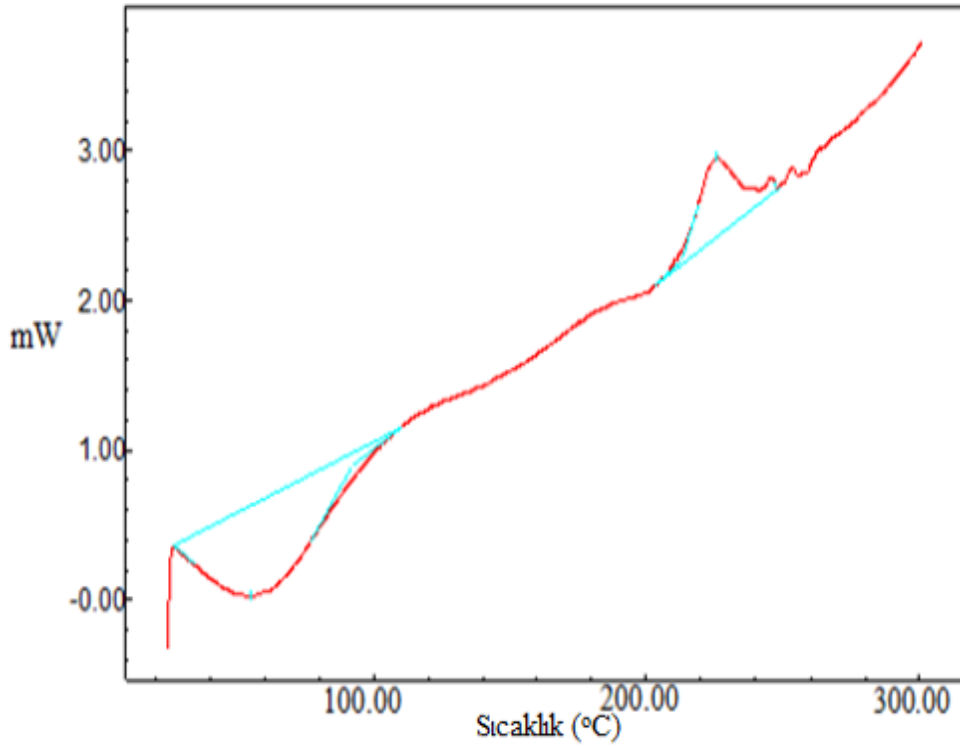
Şekil 4.54. KK3KA maddesine ilişkin DSC eğrisi
