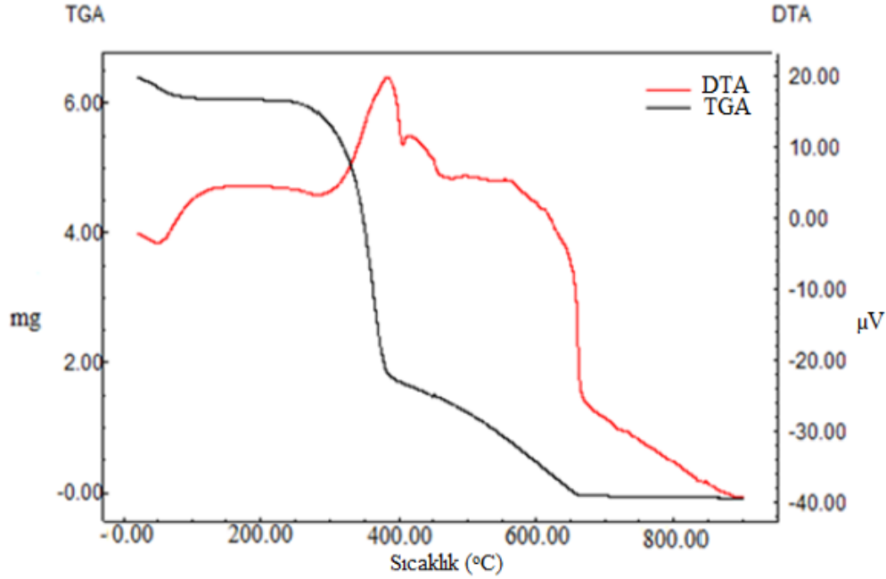
Şekil 4.5. Kitine ilişkin TGA ve DTA eğrileri
