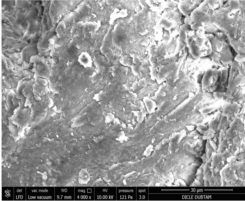
Şekil 4.40. KDA maddesine ilişkin SEM görüntüsü
