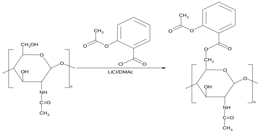
Şekil 3.4. KOAK maddesinin oluşum tepkimesi
