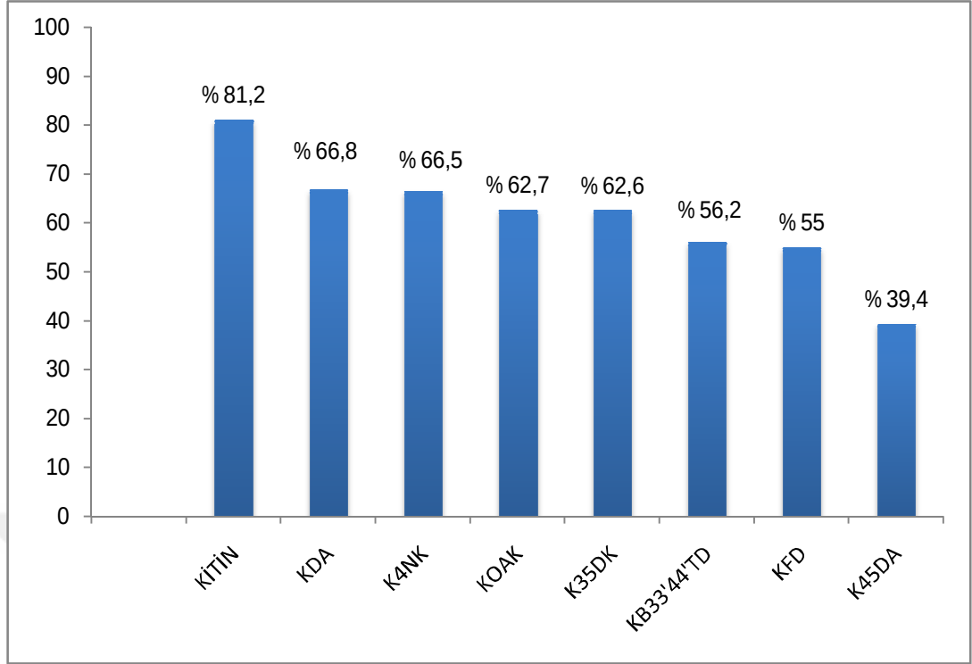
Şekil 4.55. Sentezlenen maddelerin kristallik indekslerinin kitinin kristallik indeksi ile karşılaştırılması
