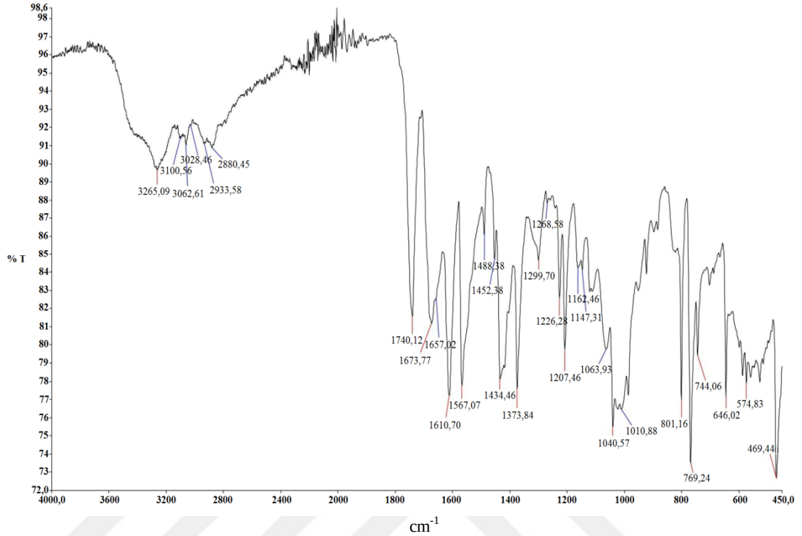
Şekil 4.49. KK3KA maddesine ilişkin FT-IR spektrumu
