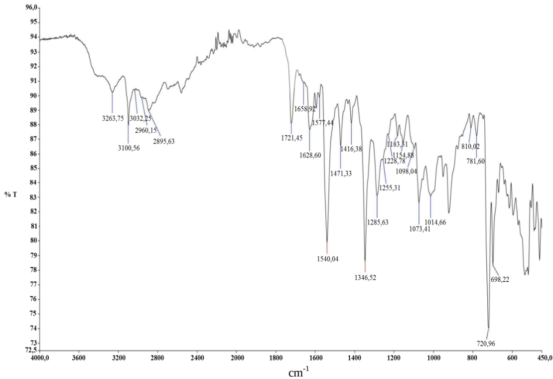
Şekil 4.7. K35DK maddesine ilişkin FT-IR spektrumu
