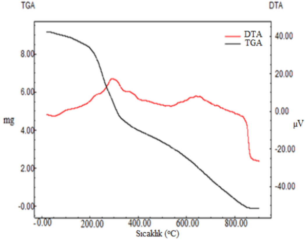
Şekil 4.11. K35DK maddesine ilişkin TGA ve DTA eğrileri
