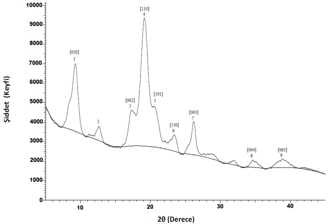
Şekil 4.3. Kitine ilişkin XRD spektrumu
