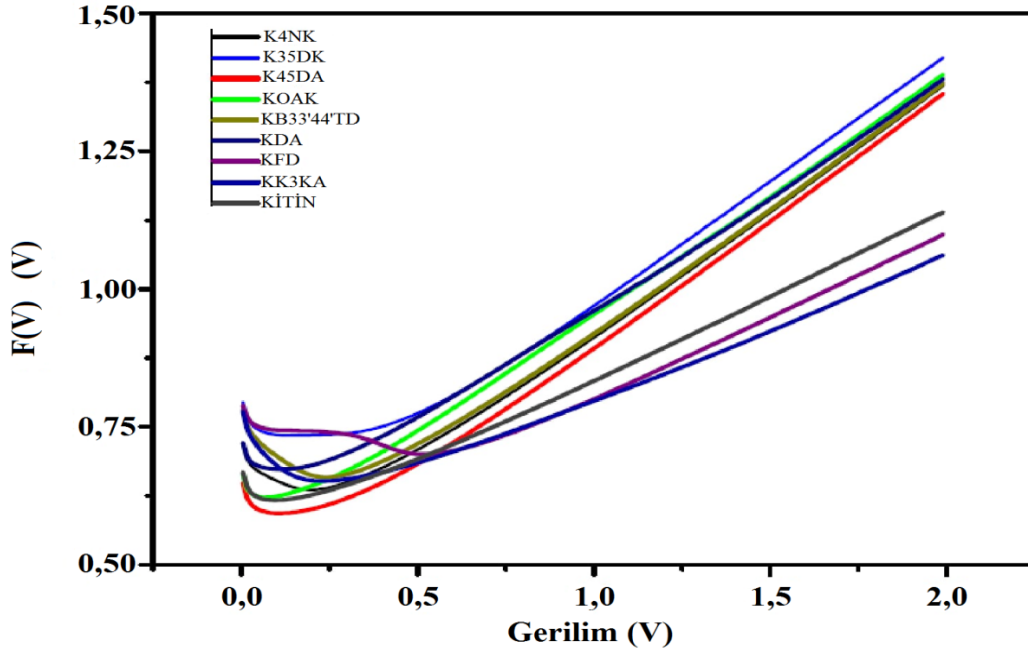
Şekil 4.57. Diyotlara ait Norde fonksiyon grafikleri
