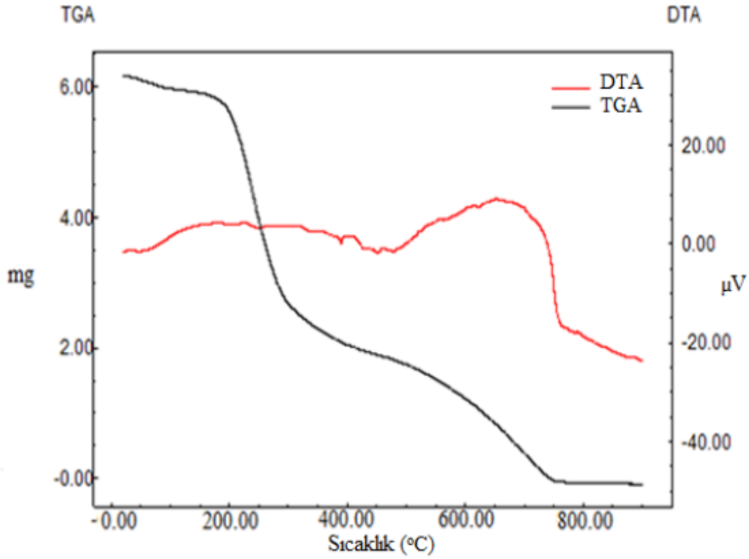
Şekil 4.53. KK3KA maddesine ilişkin TGA ve DTA eğrileri
