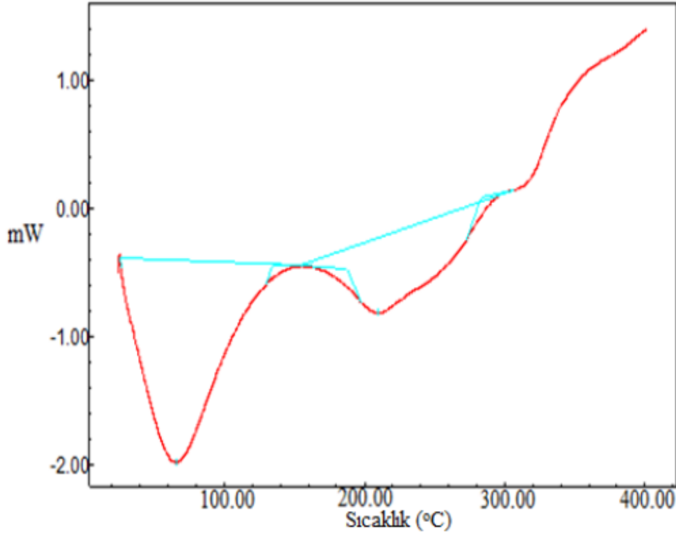
Şekil 4.30. KOAK maddesine ilişkin DSC eğrisi
