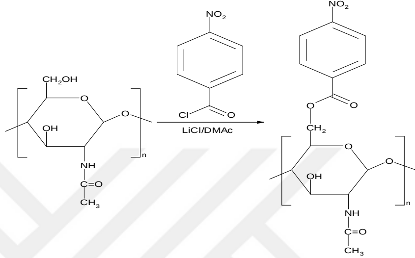
Şekil 3.3. K4NK maddesinin oluşum tepkimesi
