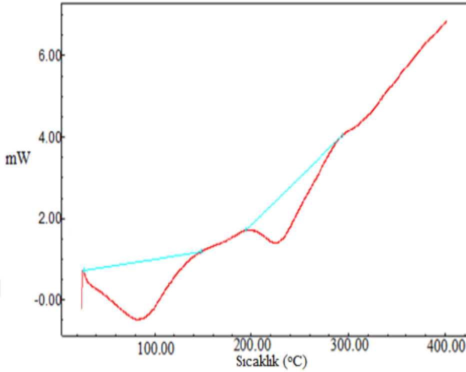
Şekil 4.36. KFD maddesine ilişkin DSC eğrisi
