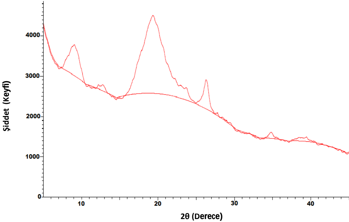
Şekil 4.27. KOAK maddesine ilişkin XRD spektrumu
