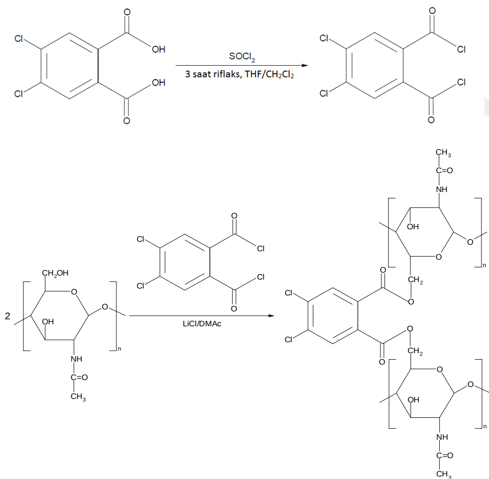
Şekil 3.2. K45DA maddesinin oluşum tepkimesi
