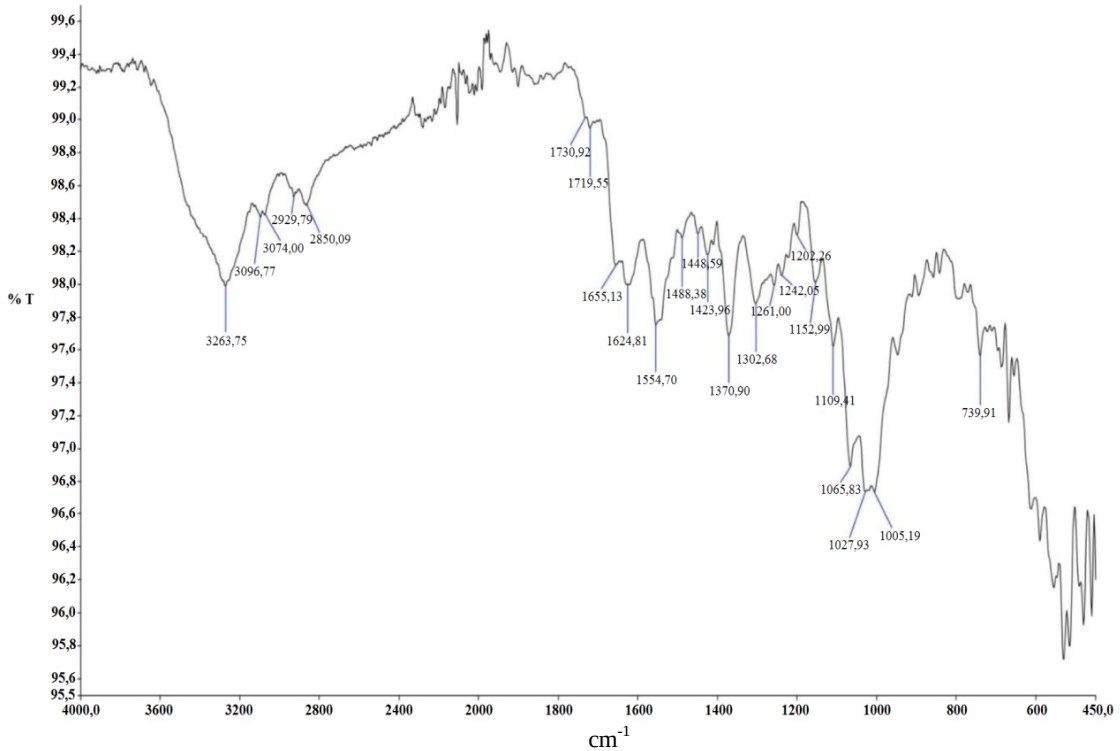
Şekil 4.43. KB33'44'TD maddesine ilişkin FT-IR spektrumu
