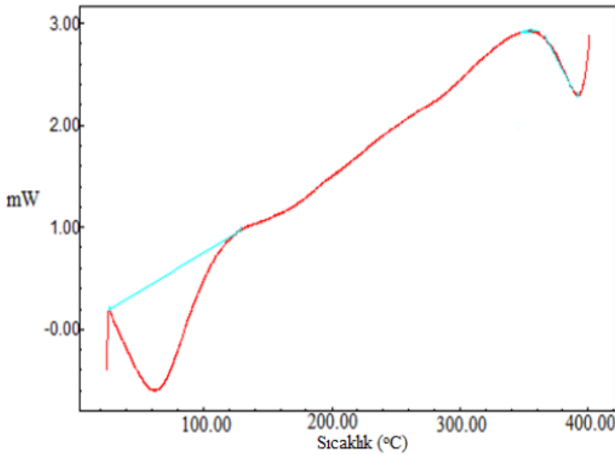
Şekil 4.6. Kitine ilişkin DSC eğrisi
