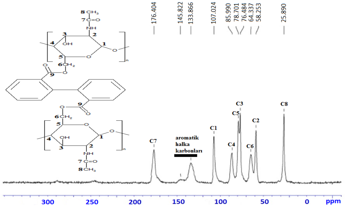
Şekil 4.38. KDA maddesine ilişkin ^{13}\text{C} CP/MAS NMR spektrumu
