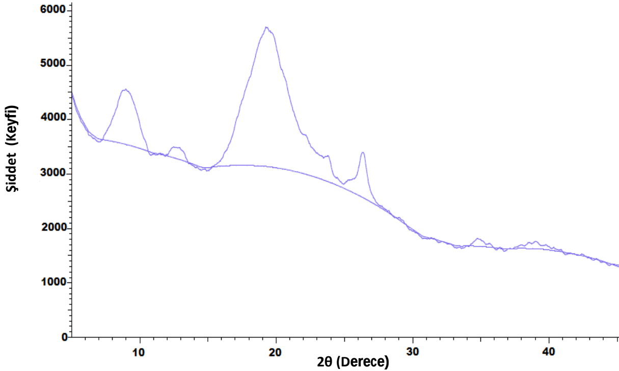
Şekil 4.39. KDA maddesine ilişkin XRD spektrumu
