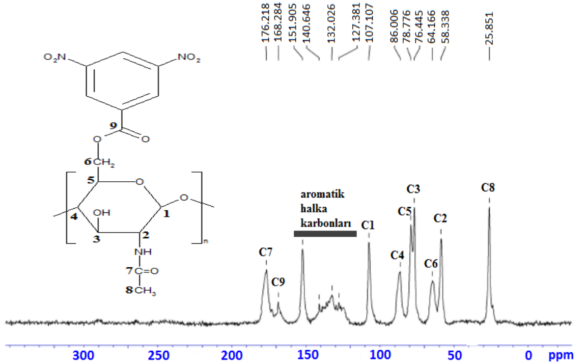
Şekil 4.8. K35DK maddesine ilişkin ^{13}\text{C} CP/MAS NMR spektrumu
