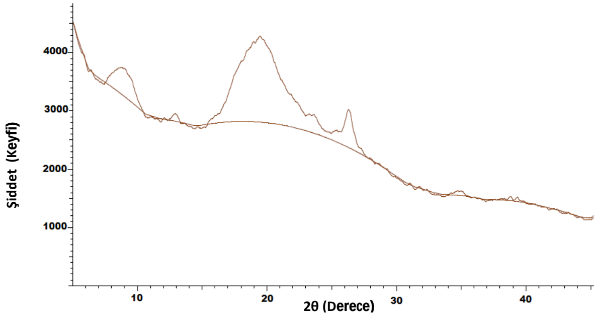
Şekil 4.45. KB33'44'TD maddesine ilişkin XRD spektrumu
