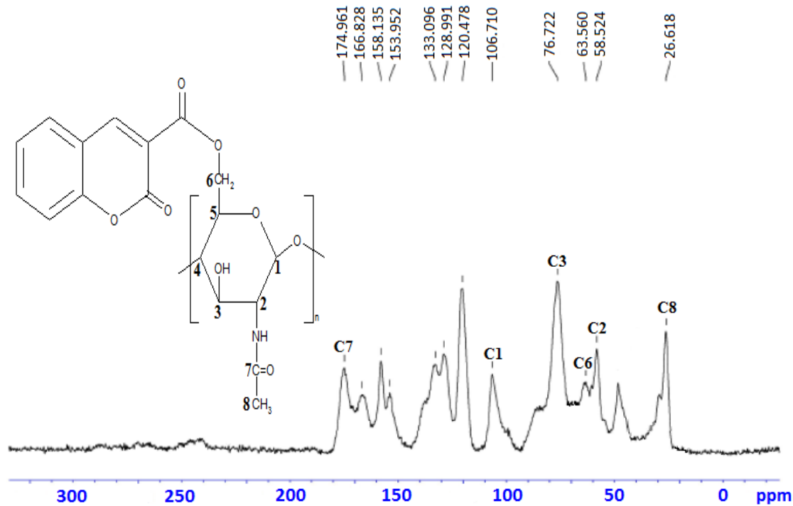
Şekil 4.50. KK3KA maddesine ilişkin ^{13}\text{C} CP/MAS NMR spektrumu
