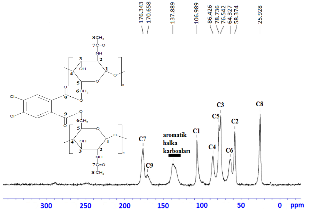
Şekil 4.14. K45DA maddesine ilişkin 13 C CP/MAS NMR spektrumu
