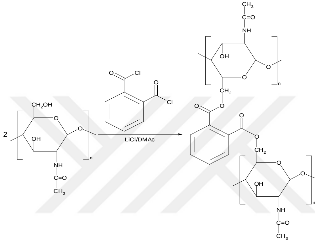
Şekil 3.5. KFD maddesinin oluşum tepkimesi
