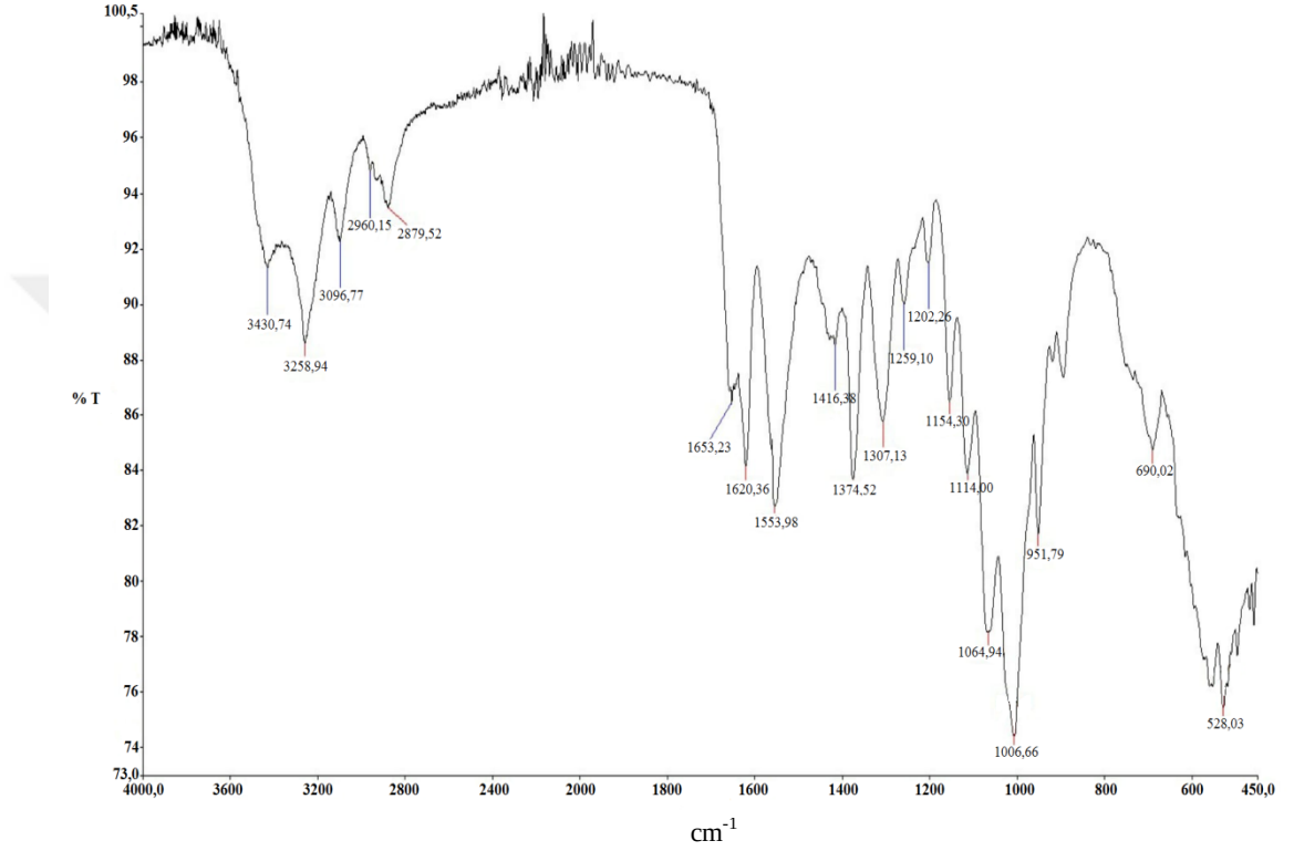
Şekil 4.1. Kitine ilişkin FT-IR spektrumu
