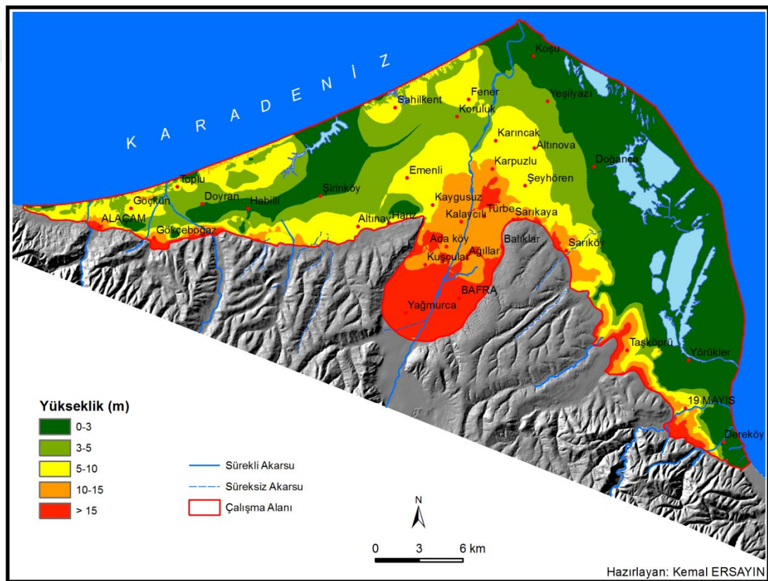
Şekil 10.Kızılırmak Deltası'nda yükselti sınıfları.
