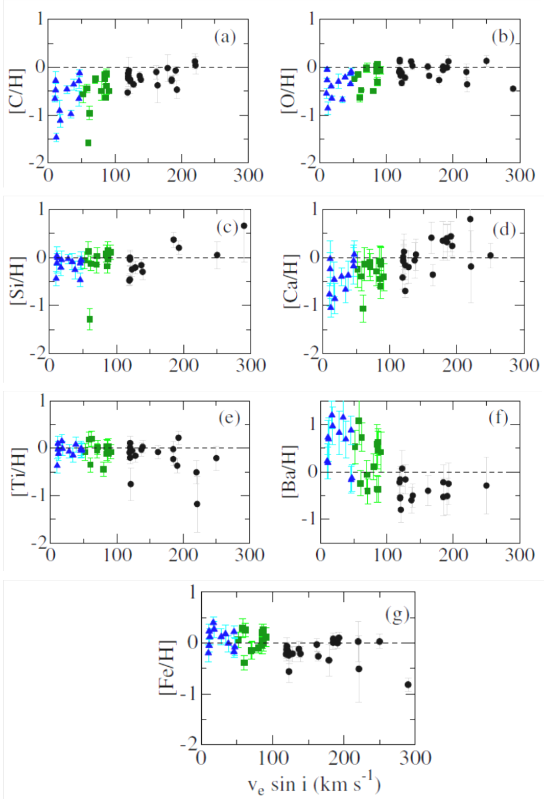
Şekil 2.2 Takeda vd. (2008) çalışmasına ait [element] - v \sin i grafikleri
