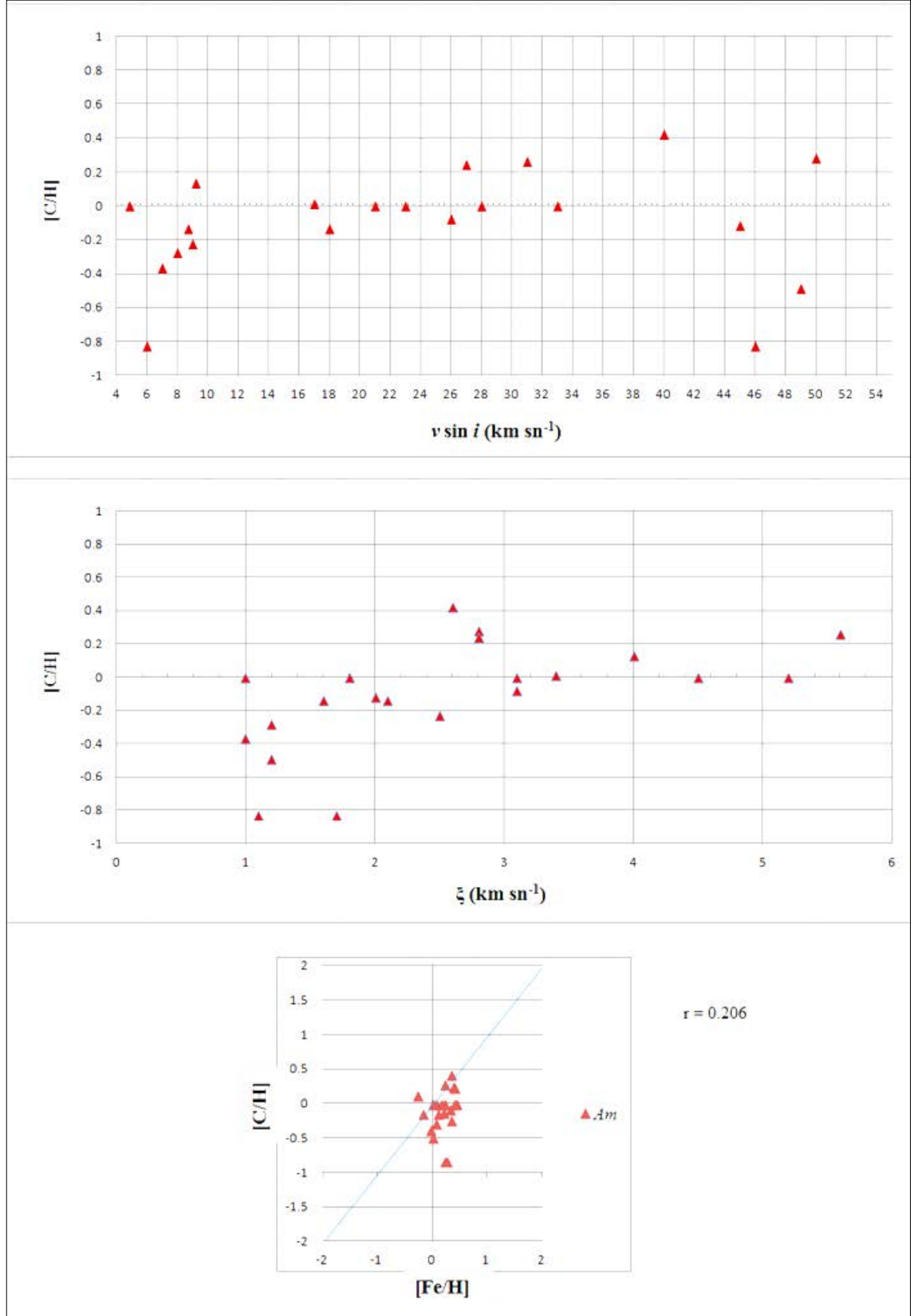
EK 5 Am tipi yıldızların [C/H] bolluk değerlerine göre; dönme hızı (üst panel), mikrotürbülans hızı (orta panel), ve [Fe/H] (alt panel) karşılaştırılması
