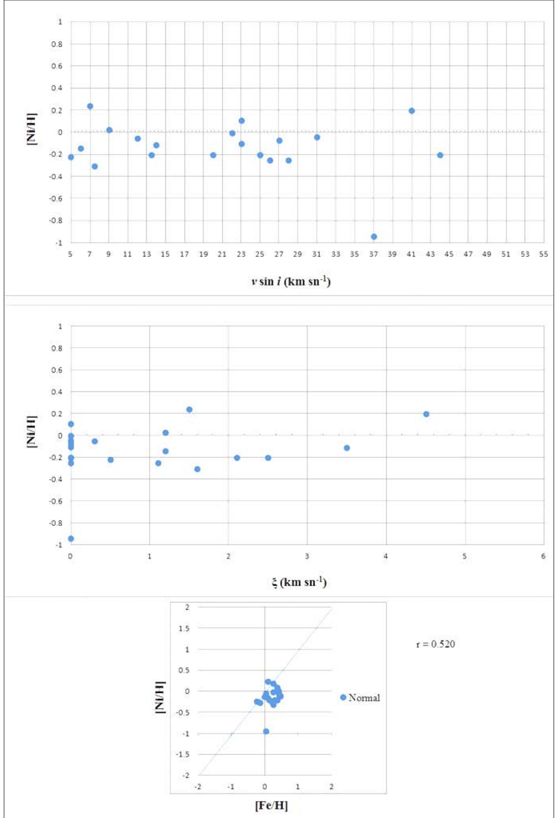
EK 4 Normal A tipi yıldızların [\text{Ni}/\text{H}] bolluk değerlerine göre; dönme hızı (üst panel), mikrotürbülans hızı (orta panel), ve [\text{Fe}/\text{H}] (alt panel) karşılaştırılması
