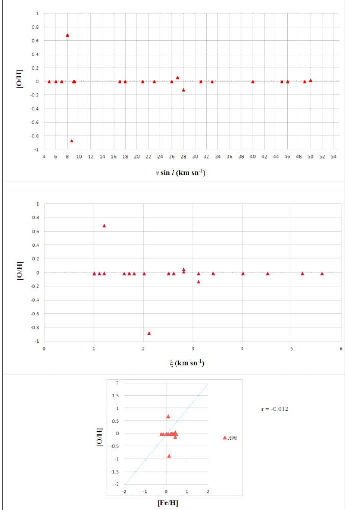
EK 5 Am tipi yıldızların [O/H] bolluk değerlerine göre; dönme hızı (üst panel), mikrotürbülans hızı (orta panel), ve [Fe/H] (alt panel) karşılaştırılması
