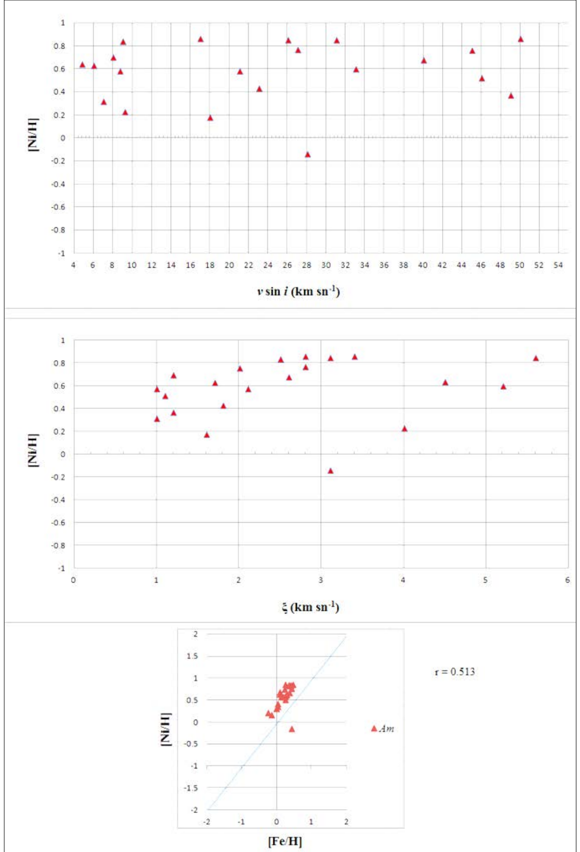
EK 5 Am tipi yıldızların [Ni/H] bolluk değerlerine göre; dönme hızı (üst panel), mikrotürbülans hızı (orta panel), ve [Fe/H] (alt panel) karşılaştırılması
