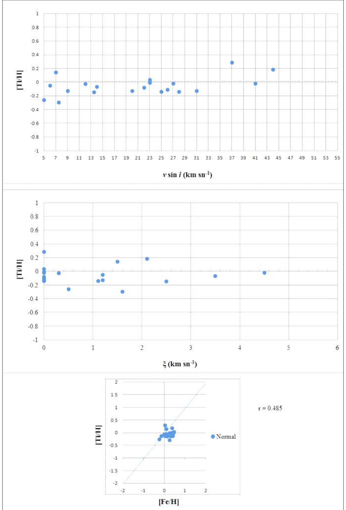
EK 4 Normal A tipi yıldızların [Ti/H] bolluk değerlerine göre; dönme hızı (üst panel), mikrotürbülans hızı (orta panel), ve [Fe/H] (alt panel) karşılaştırılması
