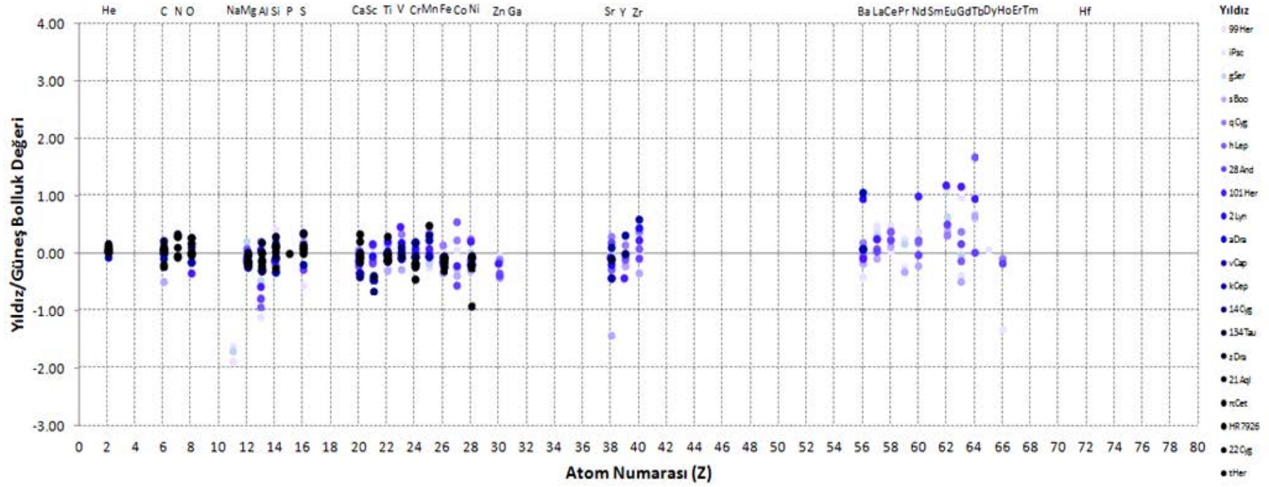
Şekil 4.7 Normal A tipi yıldızların element bolluk dağılımı
