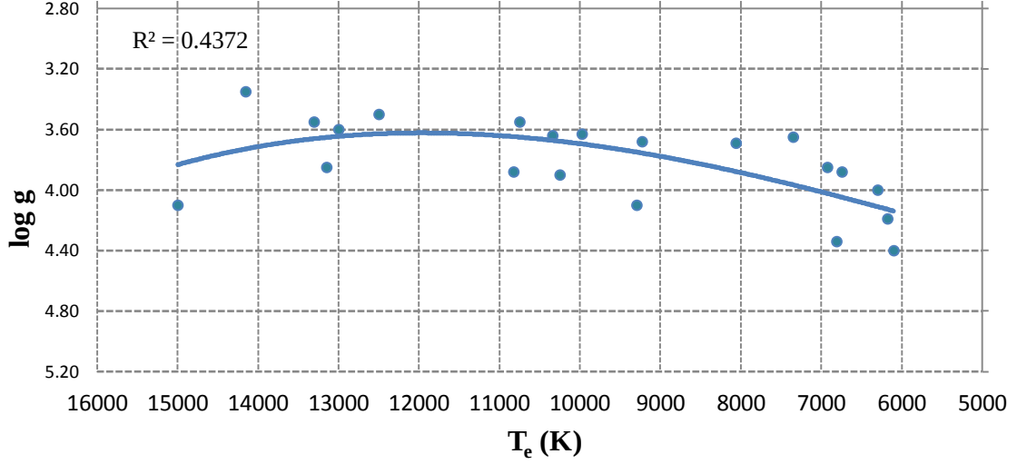
Şekil 4.1 Normal A tipi yıldızlar için T_e - \log g grafiği
