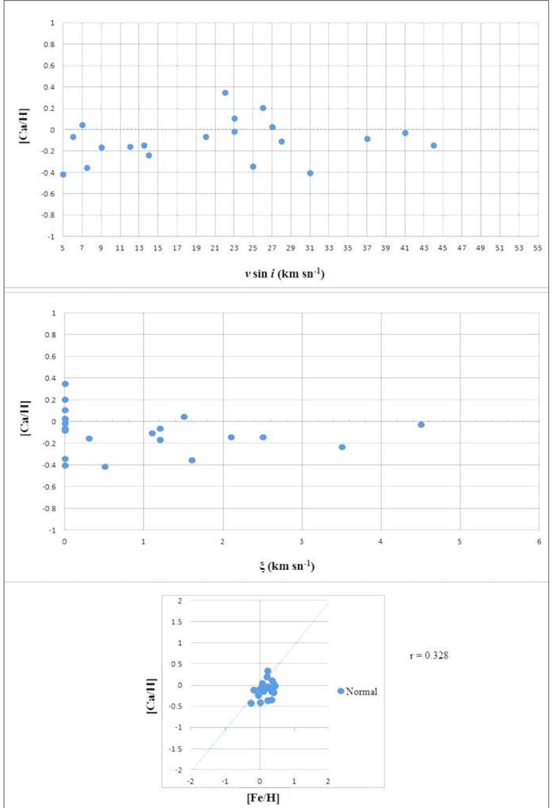
EK 4 Normal A tipi yıldızların [Ca/H] bolluk değerlerine göre; dönme hızı (üst panel), mikrotürbülans hızı (orta panel), ve [Fe/H] (alt panel) karşılaştırılması
