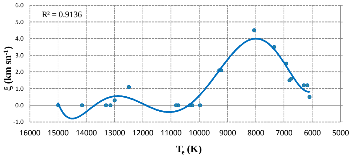
Şekil 4.3 Normal A tipi yıldızlar için T_e - \xi grafiği
