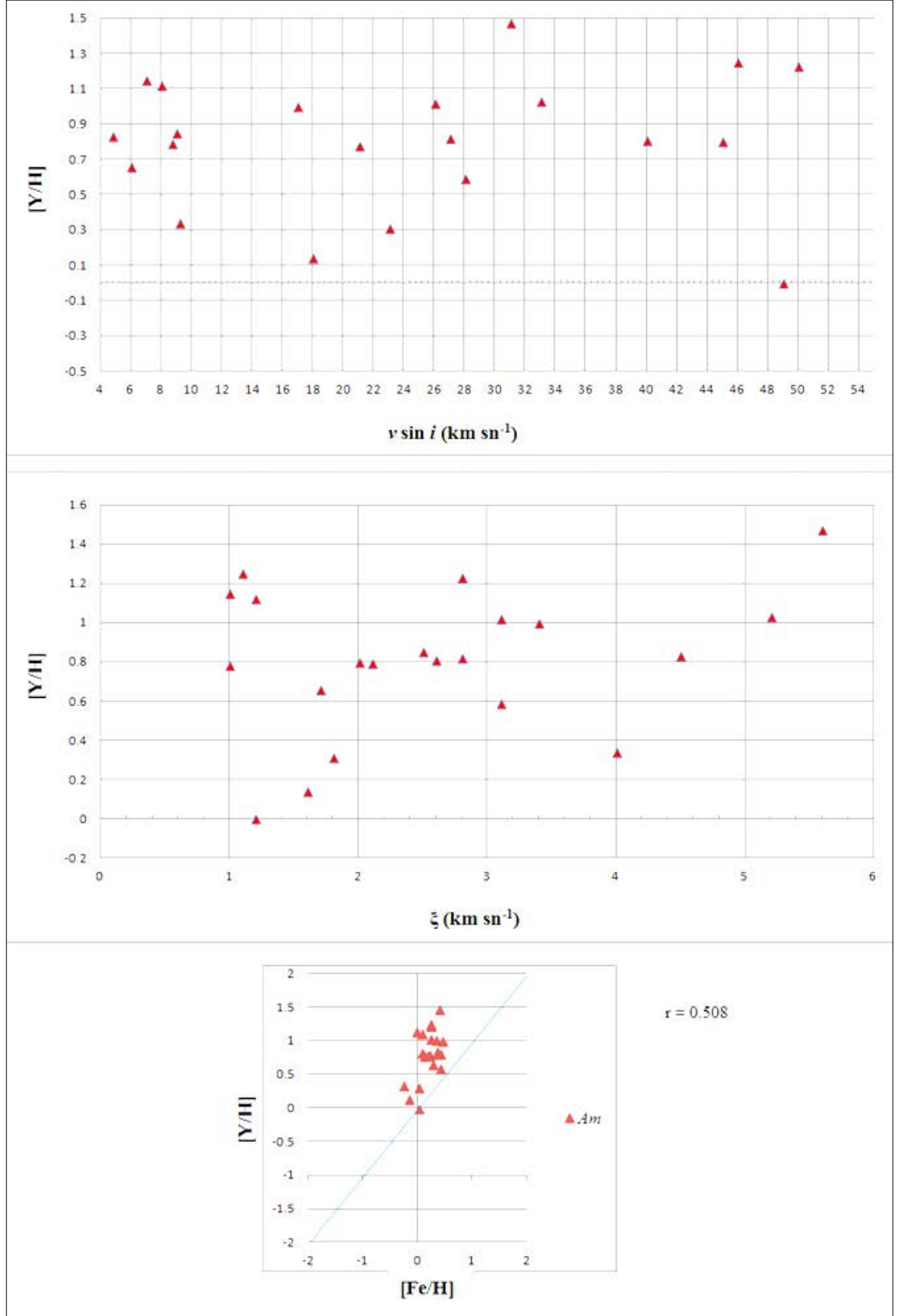
EK 5 Am tipi yıldızların [Y/H] bolluk değerlerine göre; dönme hızı (üst panel), mikrotürbülans hızı (orta panel), ve [Fe/H] (alt panel) karşılaştırılması
