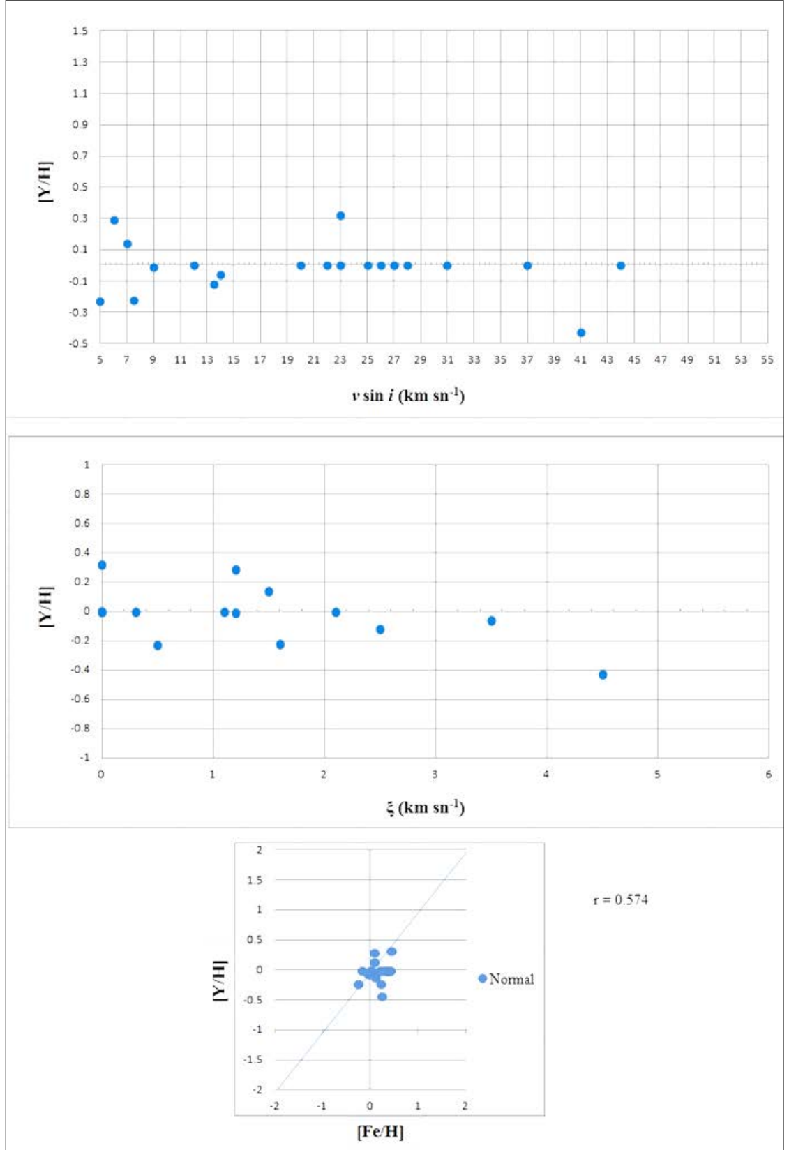
EK 4 Normal A tipi yıldızların [Y/H] bolluk değerlerine göre; dönme hızı (üst panel), mikrotürbülans hızı (orta panel), ve [Fe/H] (alt panel) karşılaştırılması
