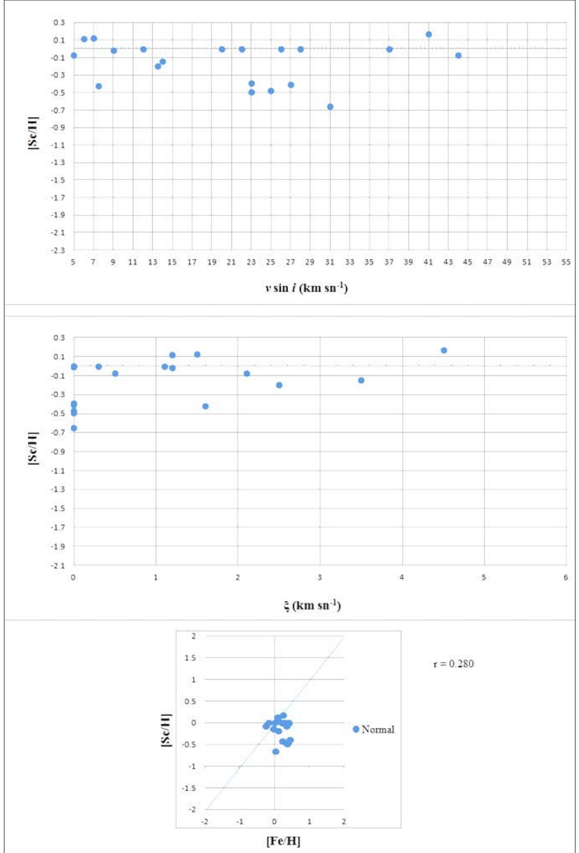
EK 4 Normal A tipi yıldızların [Sc/H] bolluk değerlerine göre; dönme hızı (üst panel), mikrotürbülans hızı (orta panel), ve [Fe/H] (alt panel) karşılaştırılması
