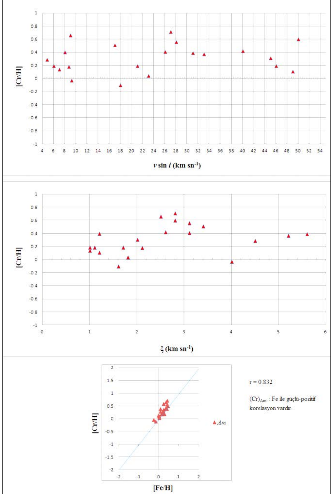
EK 5 Am tipi yıldızların [Cr/H] bolluk değerlerine göre; dönme hızı (üst panel), mikrotürbülans hızı (orta panel), ve [Fe/H] (alt panel) karşılaştırılması
