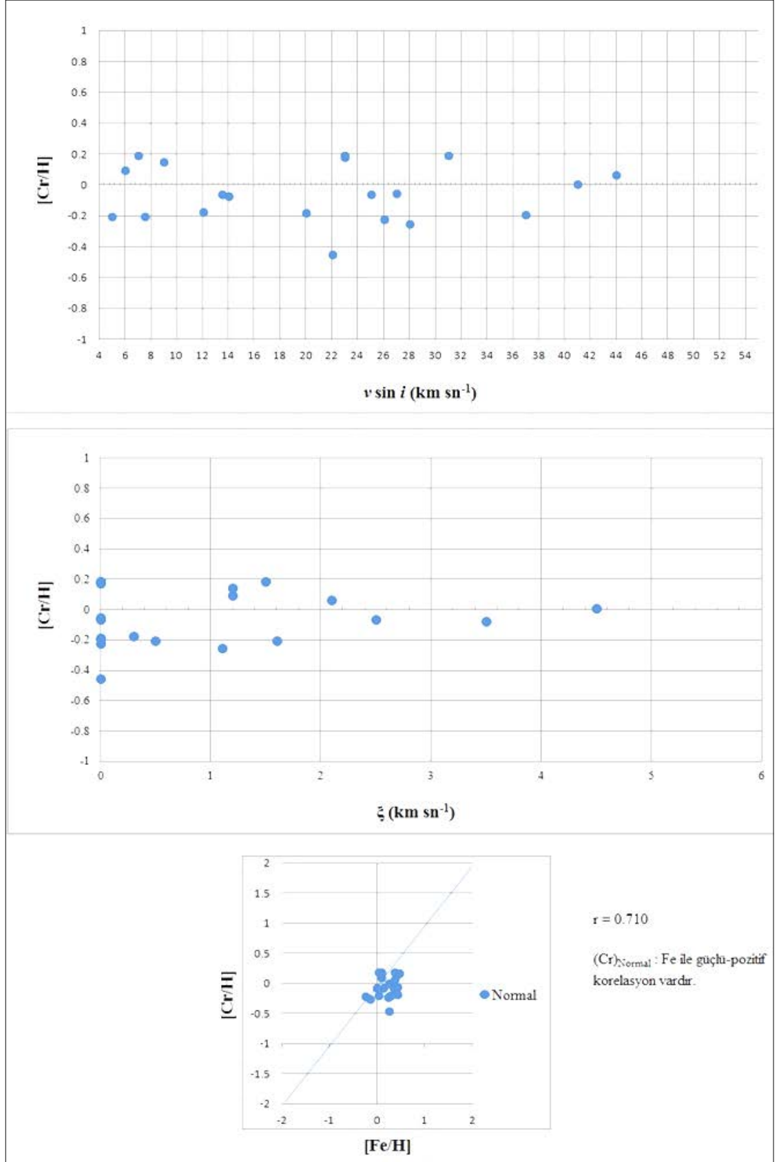
EK 4 Normal A tipi yıldızların [\text{Cr}/\text{H}] bolluk değerlerine göre; dönme hızı (üst panel), mikrotürbülans hızı (orta panel), ve [\text{Fe}/\text{H}] (alt panel) karşılaştırılması
