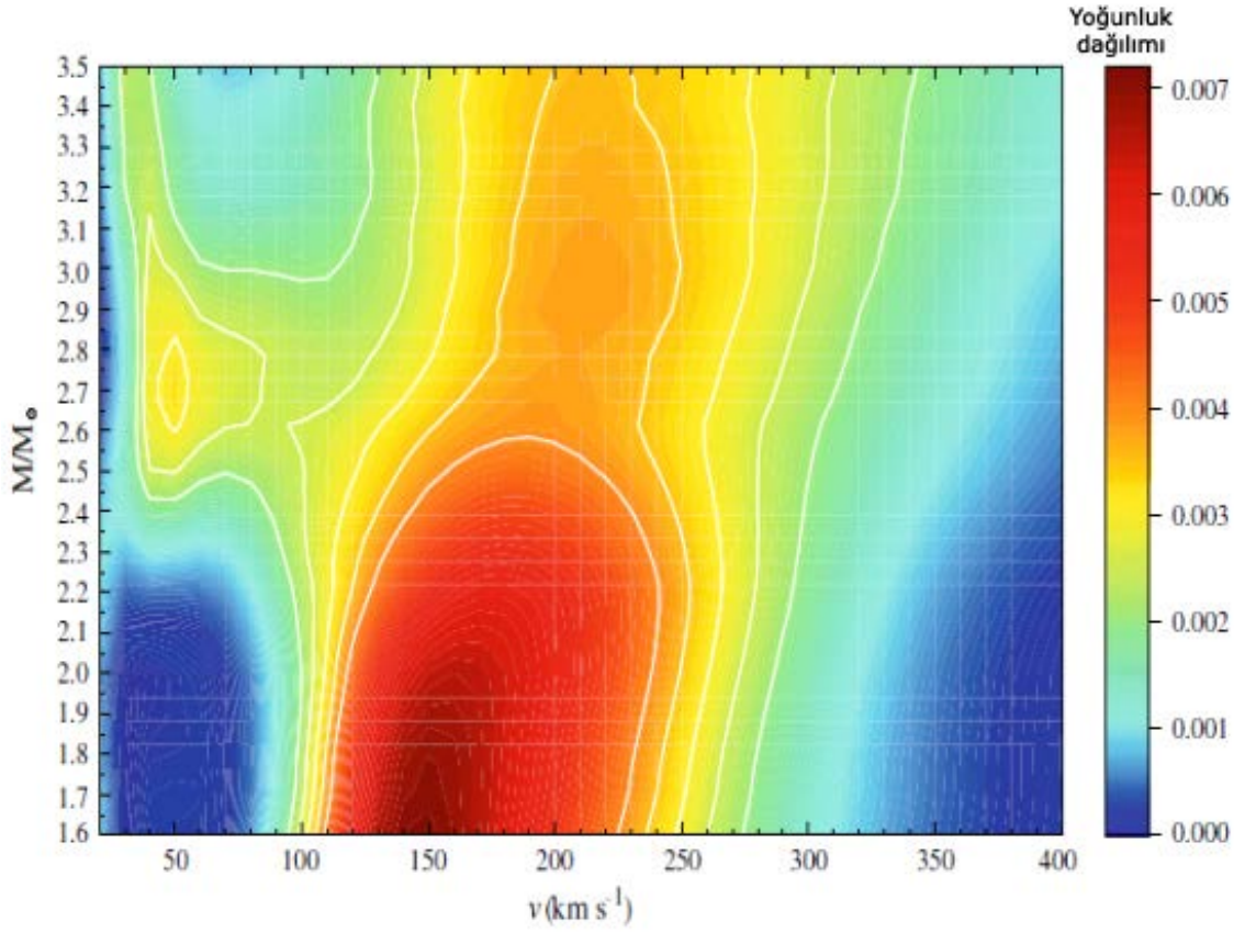
Şekil 2.3 Normal yıldızlarda, kütlenin bir fonksiyonu olarak ( M/M_{\odot} ) gerçek dönme hızlarının ( v ) dağılımları (Zorec ve Royer 2012)
