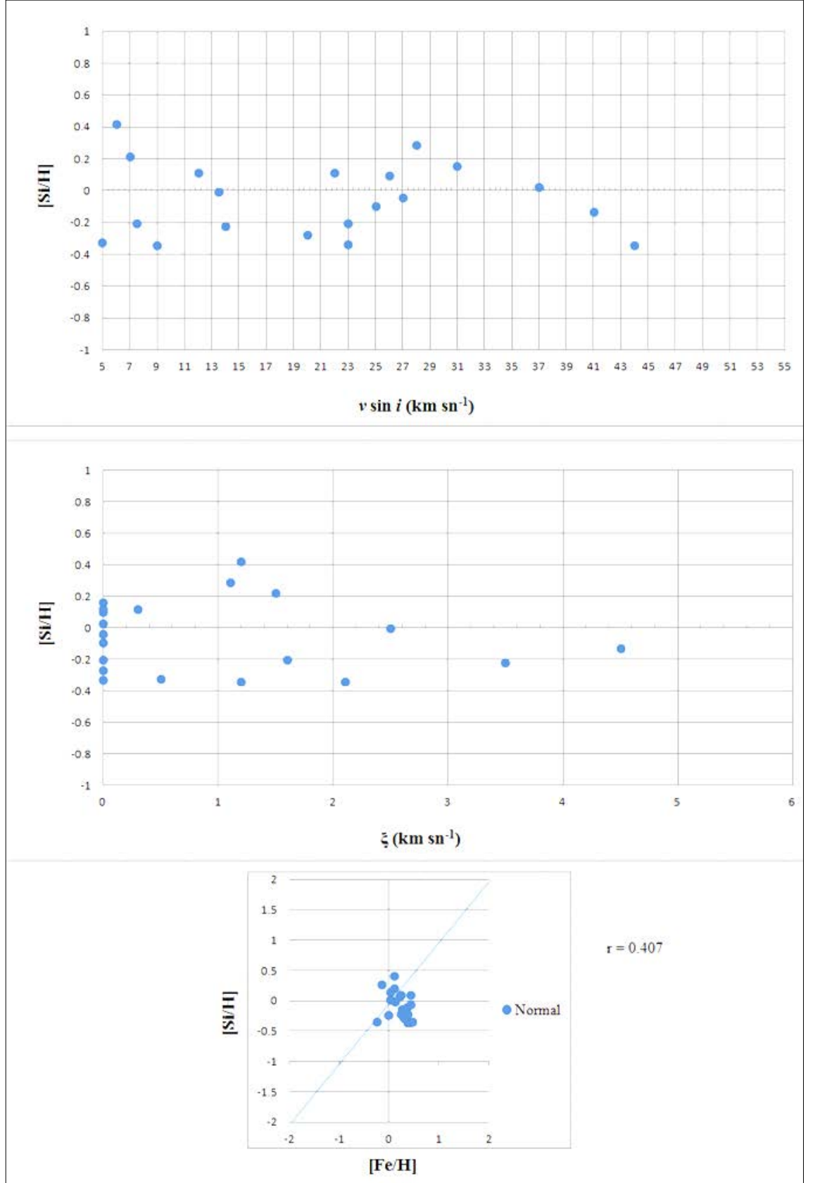
EK 4 Normal A tipi yıldızların [Si/H] bolluk değerlerine göre; dönme hızı (üst panel), mikrotürbülans hızı (orta panel), ve [Fe/H] (alt panel) karşılaştırılması
