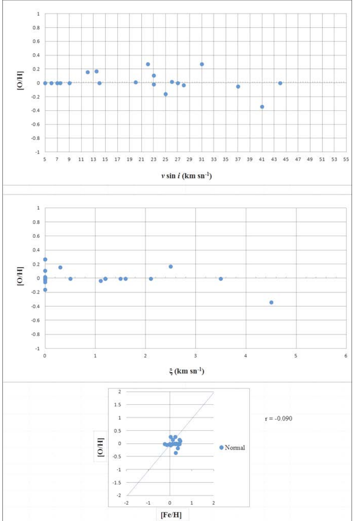
EK 4 Normal A tipi yıldızların [O/H] bolluk değerlerine göre; dönme hızı (üst panel), mikrotürbülans hızı (orta panel), ve [Fe/H] (alt panel) karşılaştırılması
