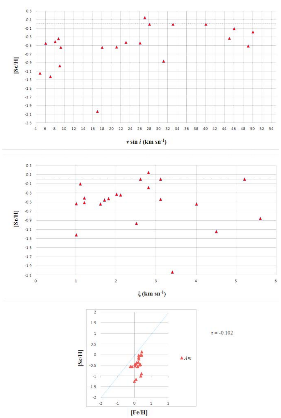
EK 5 Am tipi yıldızların [Sc/H] bolluk değerlerine göre; dönme hızı (üst panel), mikrotürbülans hızı (orta panel), ve [Fe/H] (alt panel) karşılaştırılması
