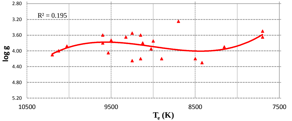
Şekil 4.2 Am tipi yıldızlar için T_e - \log g grafiği
