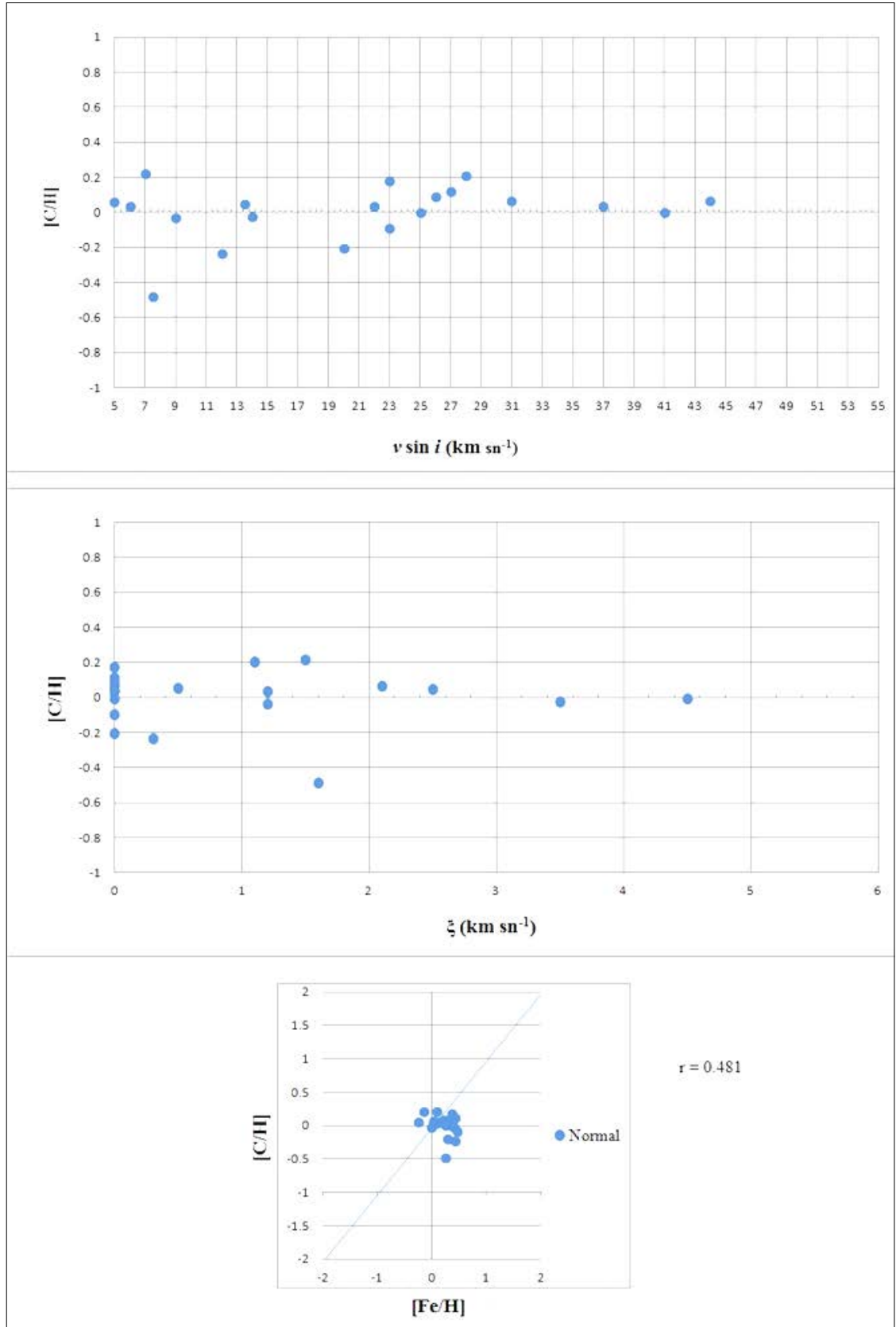
EK 4 Normal A tipi yıldızların [C/H] bolluk değerlerine göre; dönme hızı (üst panel), mikrotürbülans hızı (orta panel), ve [Fe/H] (alt panel) karşılaştırılması
