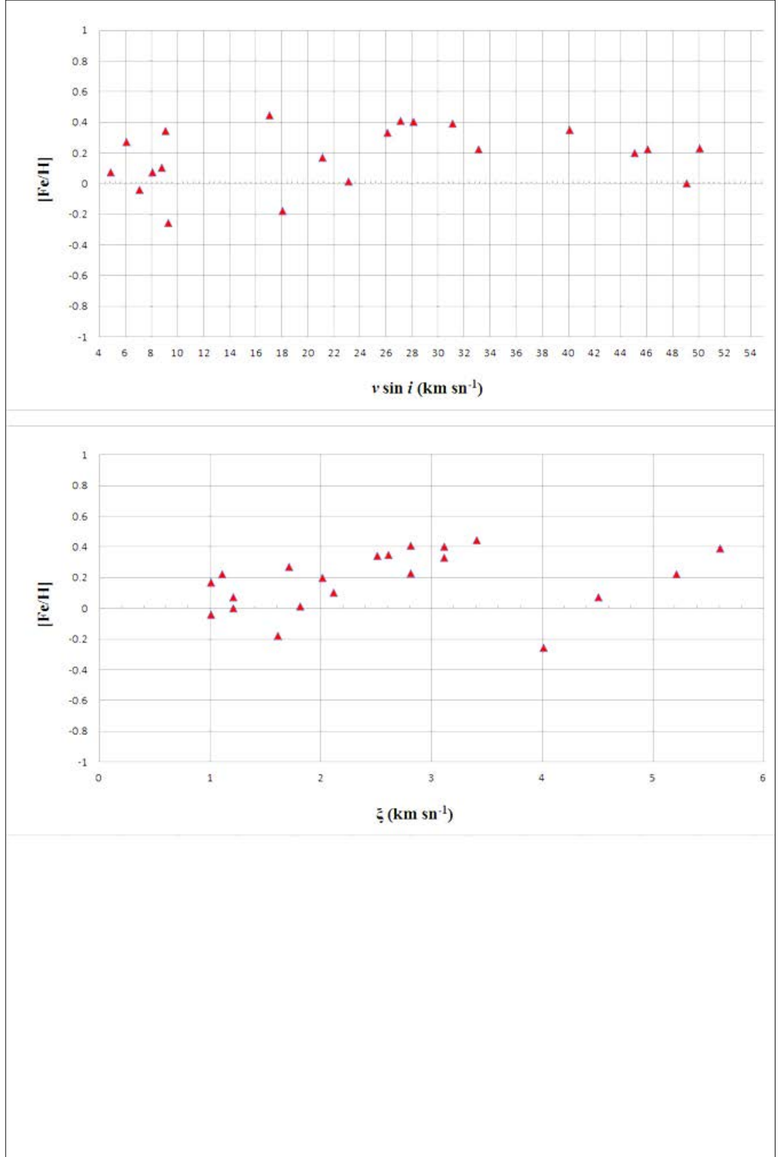
EK 5 Am tipi yıldızların [Fe/H] bolluk değerlerine göre; dönme hızı (üst panel) ve mikrotürbülans hızı (orta panel)
