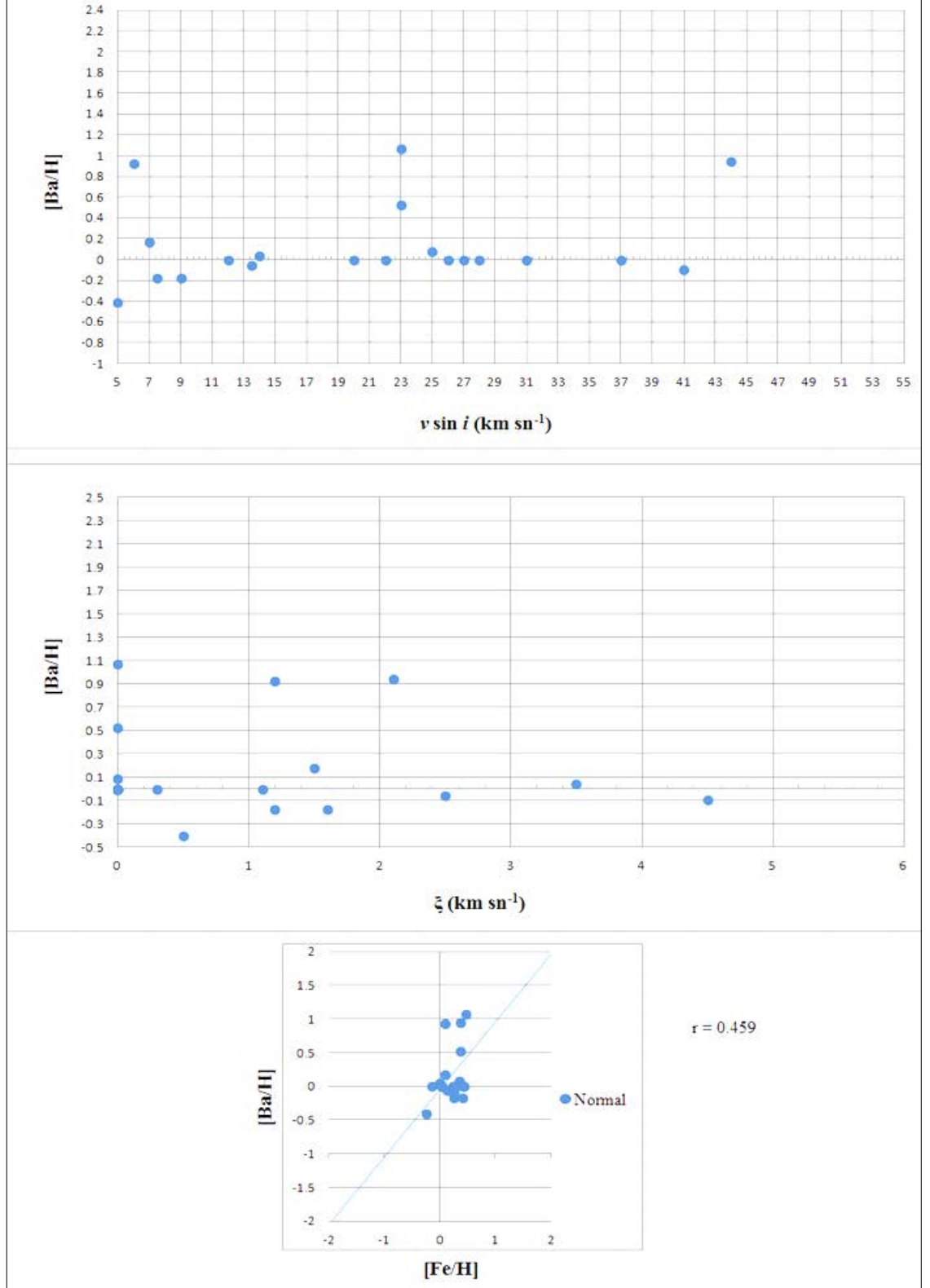
EK 4 Normal A tipi yıldızların [\text{Ba}/\text{H}] bolluk değerlerine göre; dönme hızı (üst panel), mikrotürbülans hızı (orta panel), ve [\text{Fe}/\text{H}] (alt panel) karşılaştırılması
