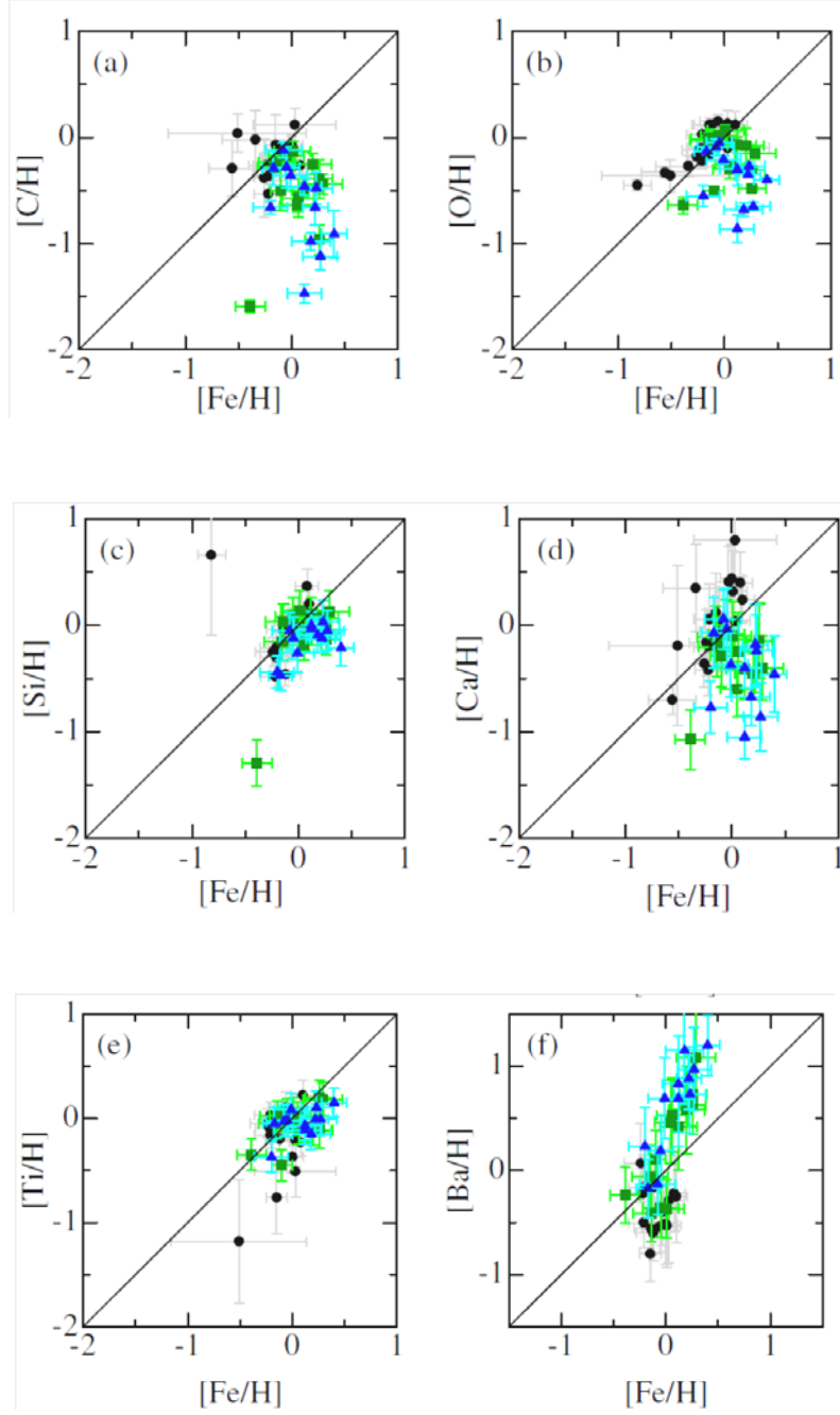
Şekil 2.4 Takeda vd. (2008) çalışmasına ait [element] - [Fe/H] grafikleri
