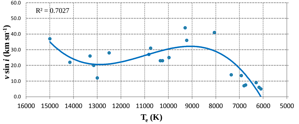
Şekil 4.5 Normal A tipi yıldızlar için T_e - v \sin i grafiği
