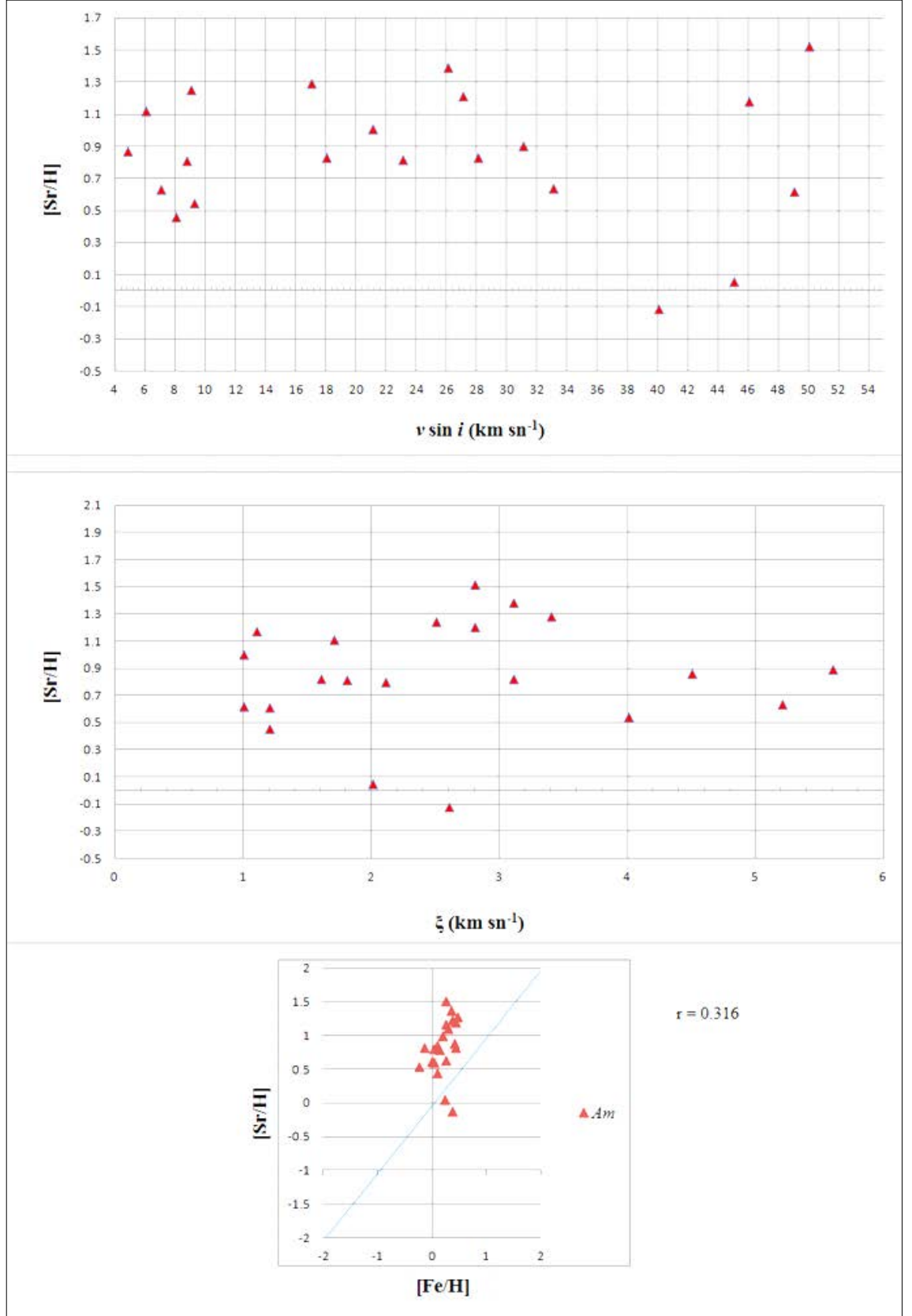
EK 5 Am tipi yıldızların [Sr/H] bolluk değerlerine göre; dönme hızı (üst panel), mikrotürbülans hızı (orta panel), ve [Fe/H] (alt panel) karşılaştırılması
