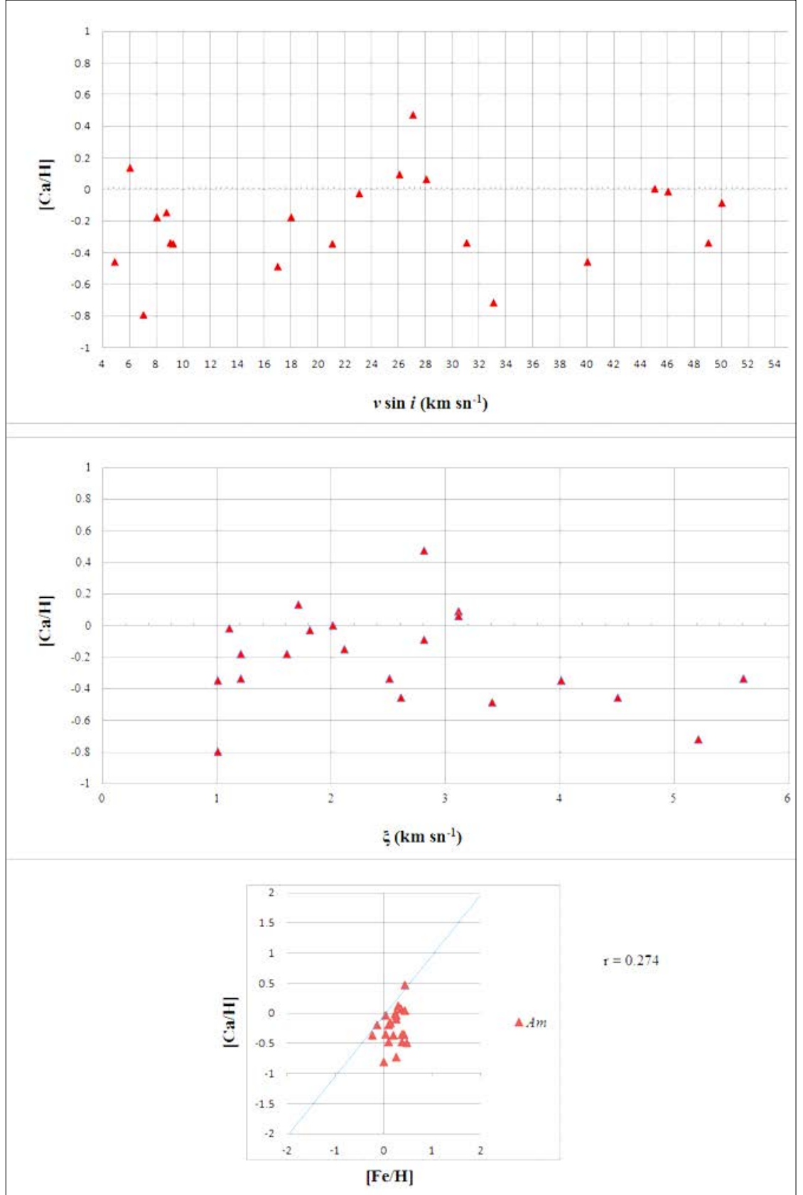
EK 5 Am tipi yıldızların [Ca/H] bolluk değerlerine göre; dönme hızı (üst panel), mikrotürbülans hızı (orta panel), ve [Fe/H] (alt panel) karşılaştırılması
