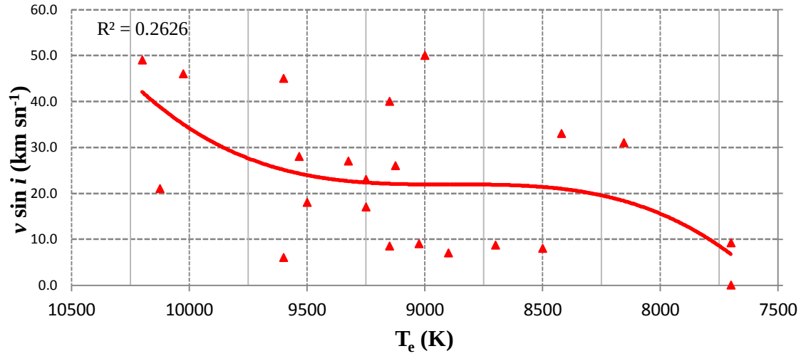
Şekil 4.6 Am tipi yıldızlar için T_e - v \sin i grafiği
