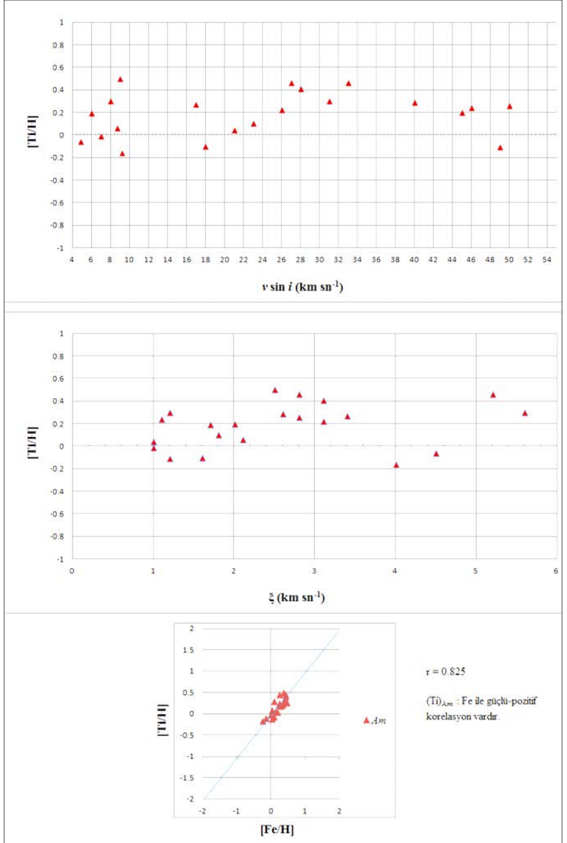
EK 5 Am tipi yıldızların [Ti/H] bolluk değerlerine göre; dönme hızı (üst panel), mikrotürbülans hızı (orta panel), ve [Fe/H] (alt panel) karşılaştırılması
