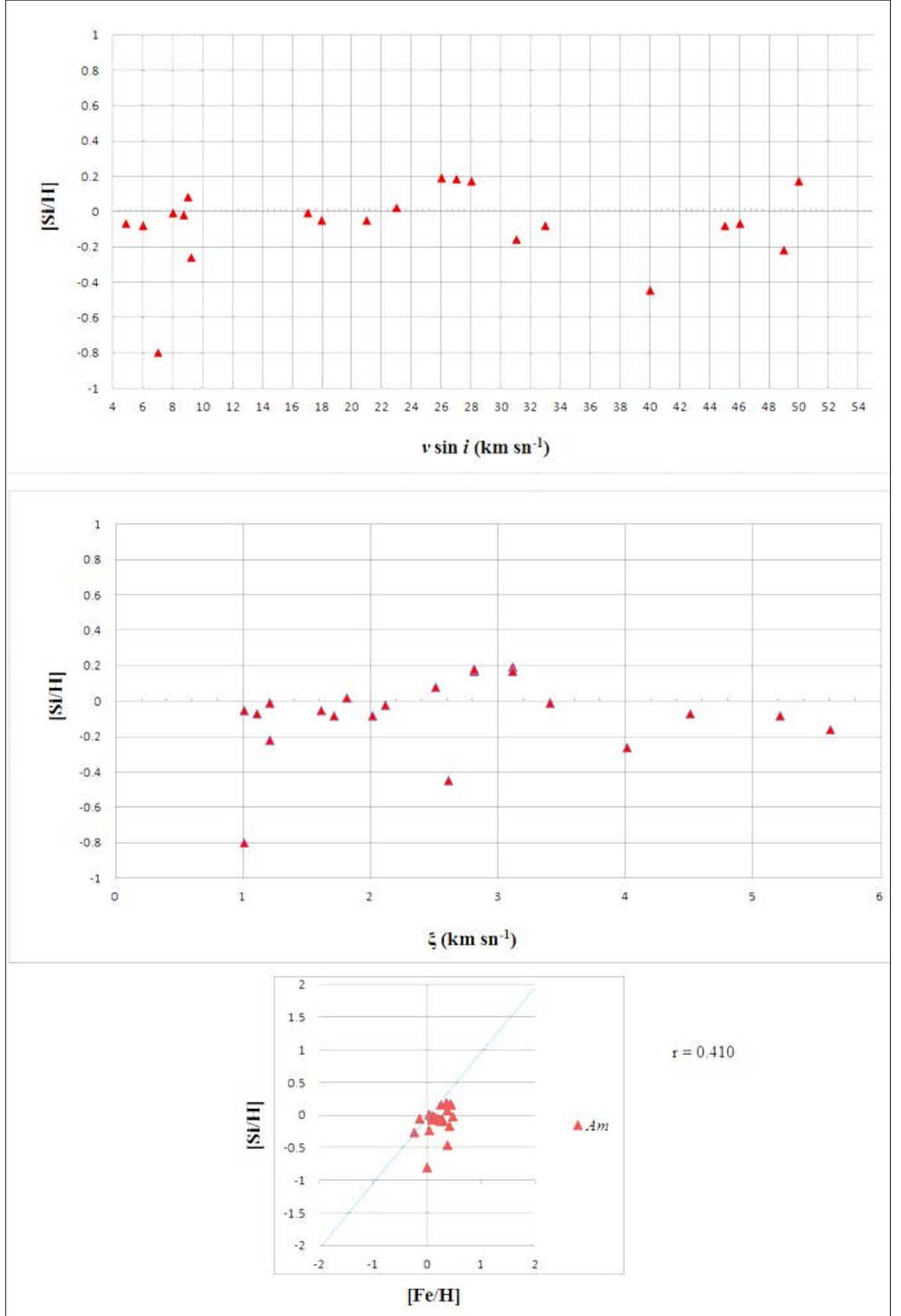
EK 5 Am tipi yıldızların [Si/H] bolluk değerlerine göre; dönme hızı (üst panel), mikrotürbülans hızı (orta panel), ve [Fe/H] (alt panel) karşılaştırılması
