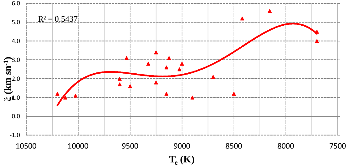
Şekil 4.4 Am tipi yıldızlar için T_e - \xi grafiği
