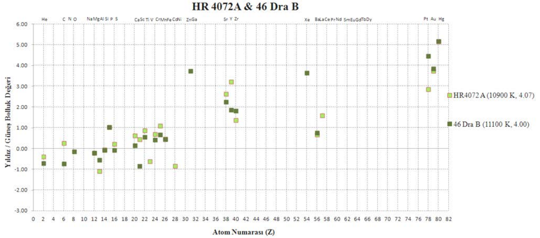
Şekil 4.9 HR 4072 A ve 46 Dra B yıldızlarına ait element bolluklarının karşılaştırılması
