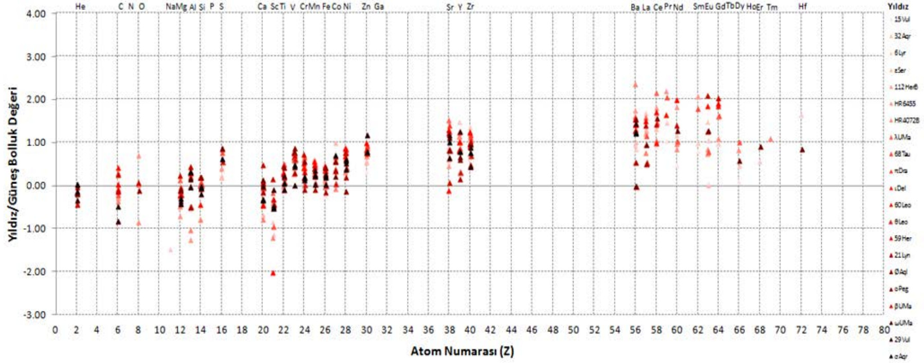
Şekil 4.8 Am tipi yıldızların element bolluk dağılımı
