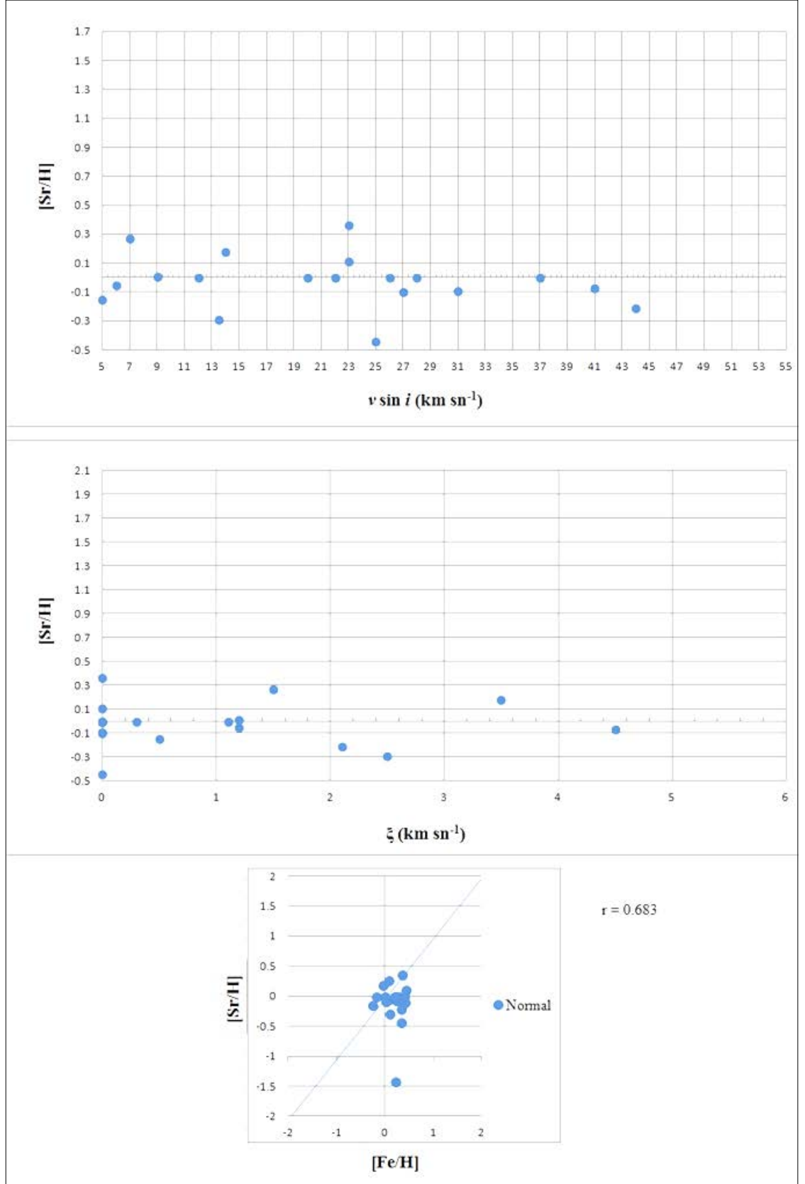
EK 4 Normal A tipi yıldızların [Sr/H] bolluk değerlerine göre; dönme hızı (üst panel), mikrotürbülans hızı (orta panel), ve [Fe/H] (alt panel) karşılaştırılması
