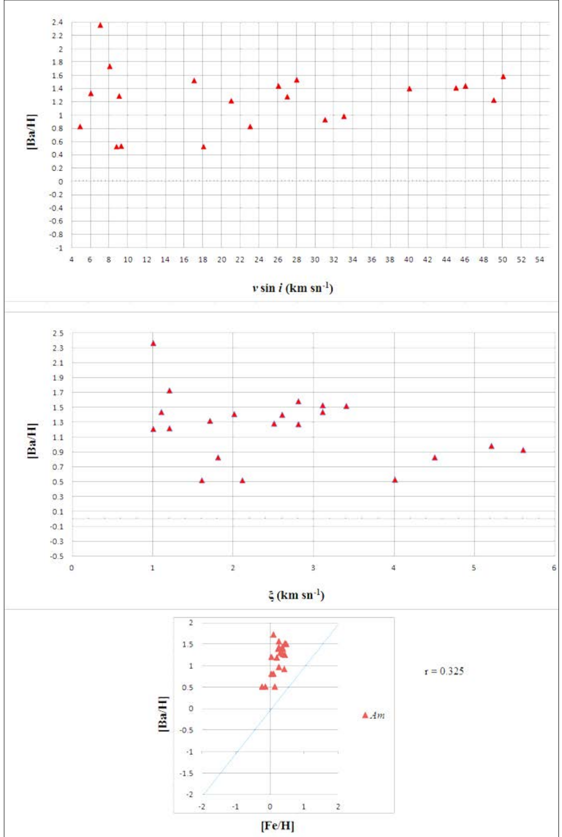
EK 5 Am tipi yıldızların [Ba/H] bolluk değerlerine göre; dönme hızı (üst panel), mikrotürbülans hızı (orta panel), ve [Fe/H] (alt panel) karşılaştırılması
