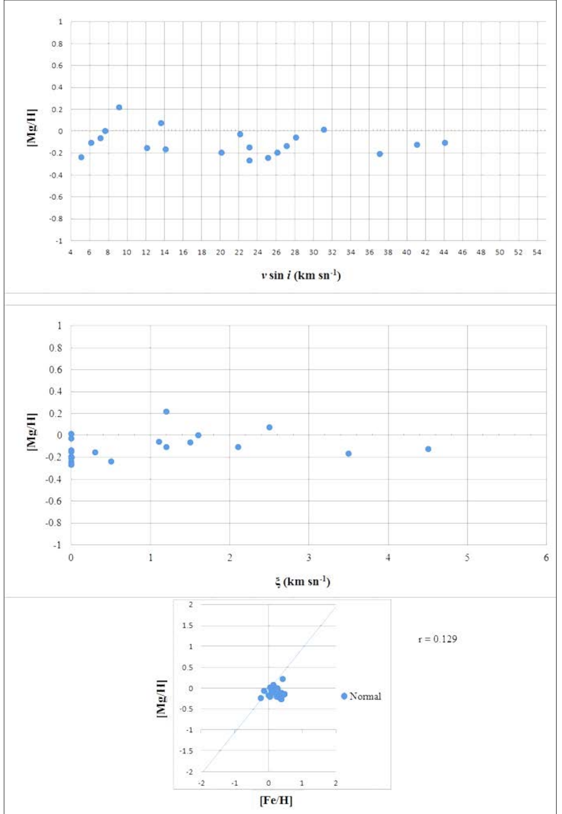
EK 4 Normal A tipi yıldızların [Mg/H] bolluk değerlerine göre; dönme hızı (üst panel), mikrotürbülans hızı (orta panel), ve [Fe/H] (alt panel) karşılaştırılması
