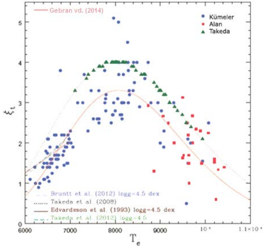
Şekil 2.1 Gebran vd. (2014) çalışmasına ait T_e - \xi grafiği
