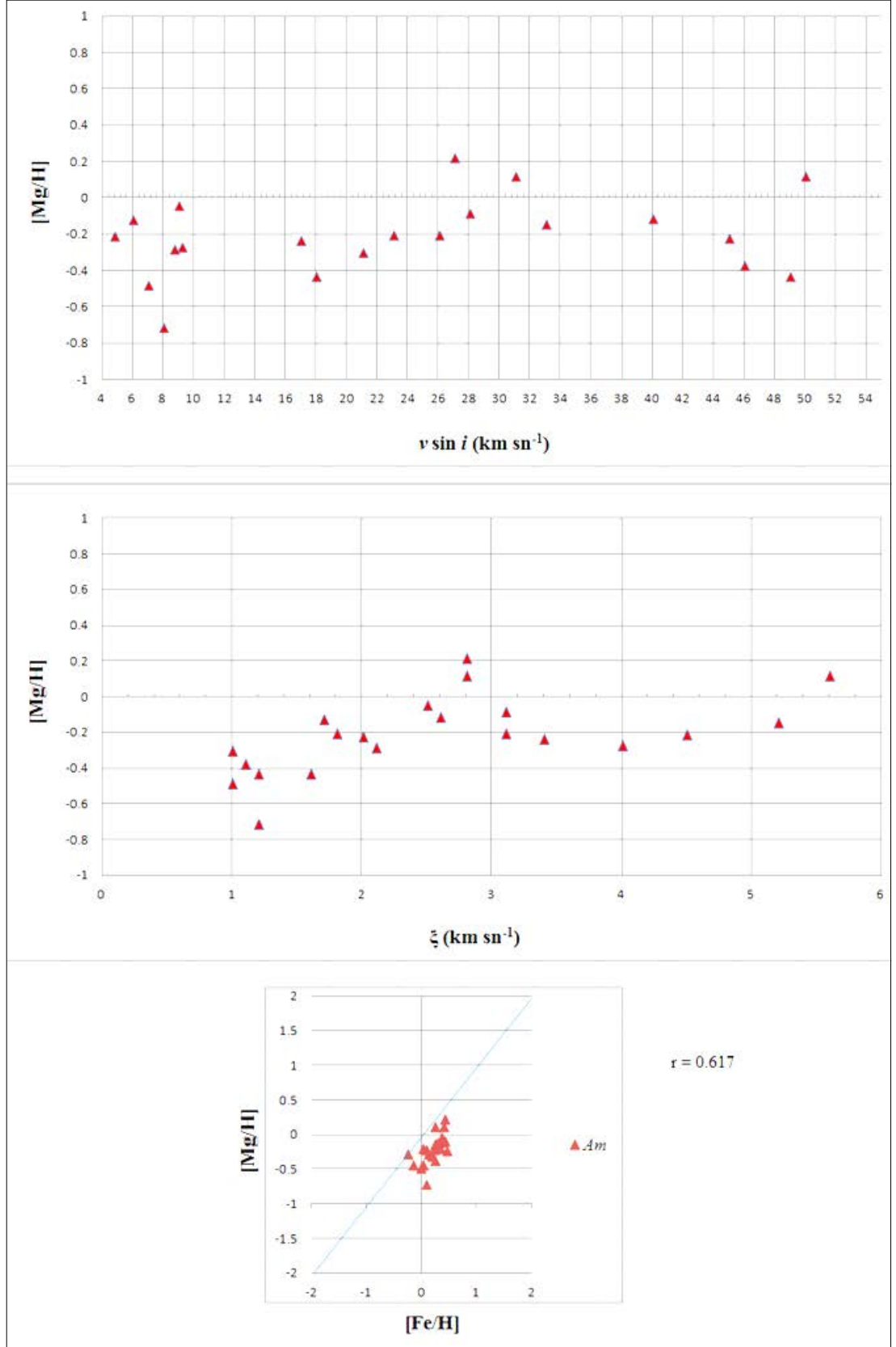
EK 5 Am tipi yıldızların [Mg/H] bolluk değerlerine göre; dönme hızı (üst panel), mikrotürbülans hızı (orta panel), ve [Fe/H] (alt panel) karşılaştırılması
