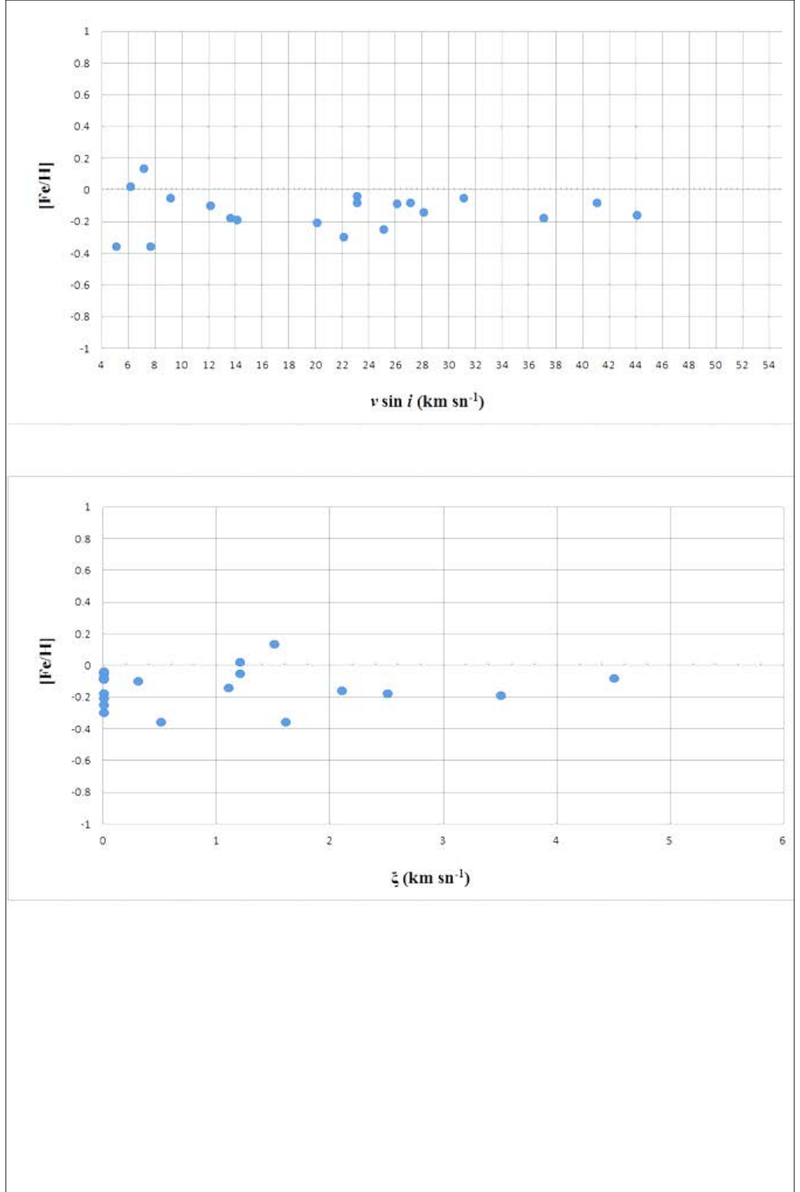
EK 4 Normal A tipi yıldızların [Fe/H] bolluk değerlerine göre; dönme hızı (üst panel) ve mikrotürbülans hızı (orta panel)
