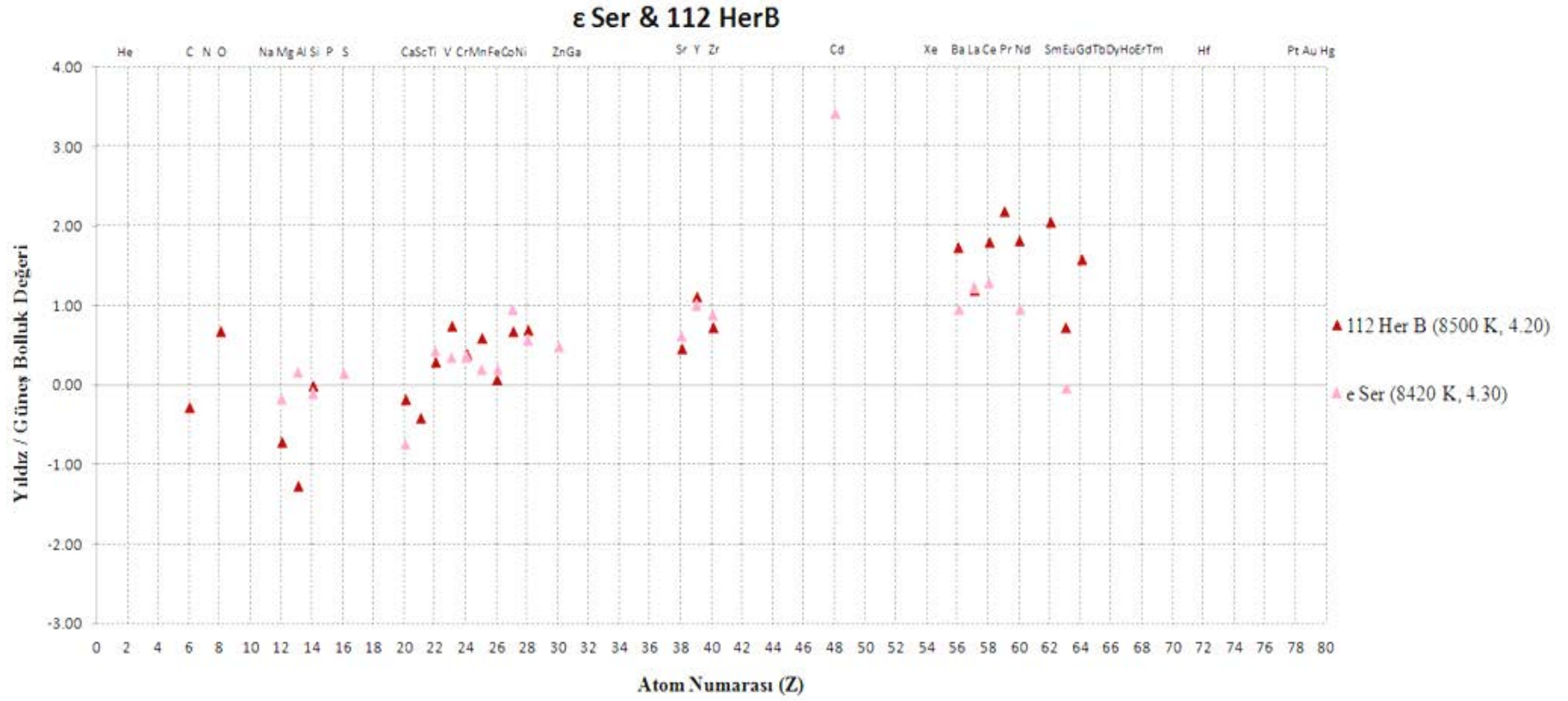
Şekil 4.11 \epsilon Ser ve 112 Her B yıldızlarına ait element bolluklarının karşılaştırılması
