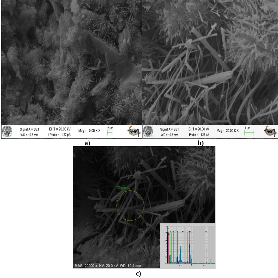
Şekil 4.13. SDC-NMS (1) jet-grout kolonlarına ait numunelerden elde edilen SEM görüntüleri
