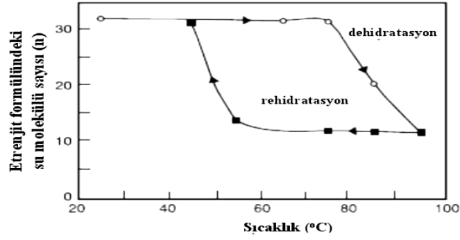
Şekil 4.8. Etrenjit kristalinin su molekülü sayısının sıcaklıkla değişimi (Zhou ve Glasser, 2001)
