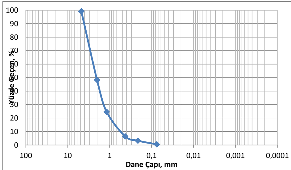
Şekil 3.30. Doğal kum zemine ait granülometri eğrisi
