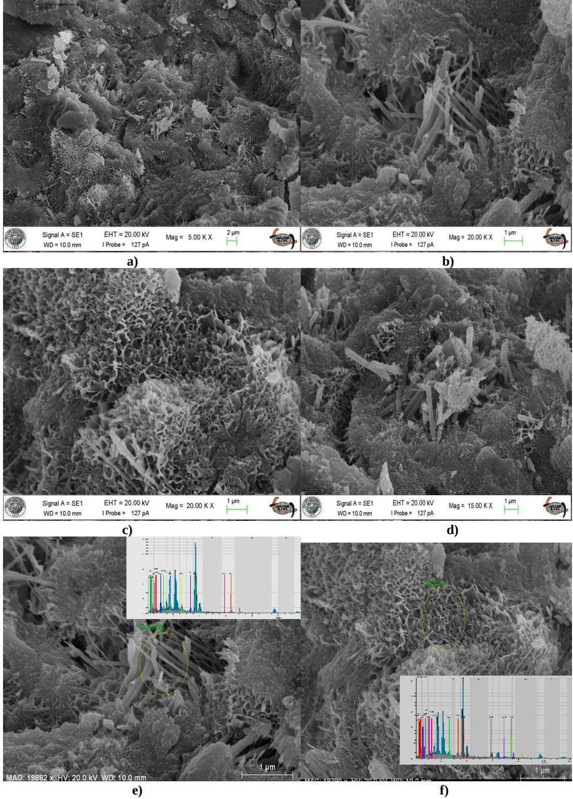
Şekil 4.16. SDÇ-SYS (3) jet-grout kolonlarına ait numunelerden elde edilen SEM görüntüleri
