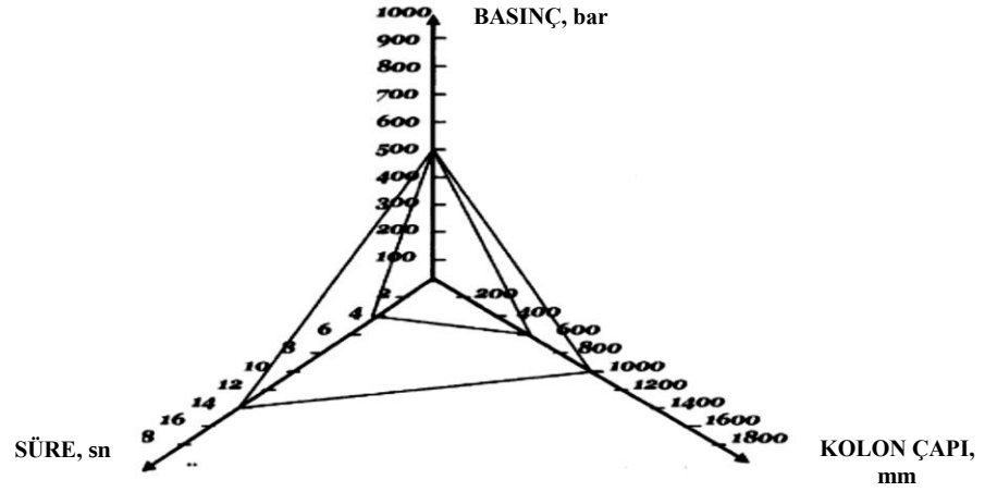
Şekil 3.10. Basınç - bekleme süresi - kolon çapı ilişkisi (Melegari ve Garassino, 1997)
