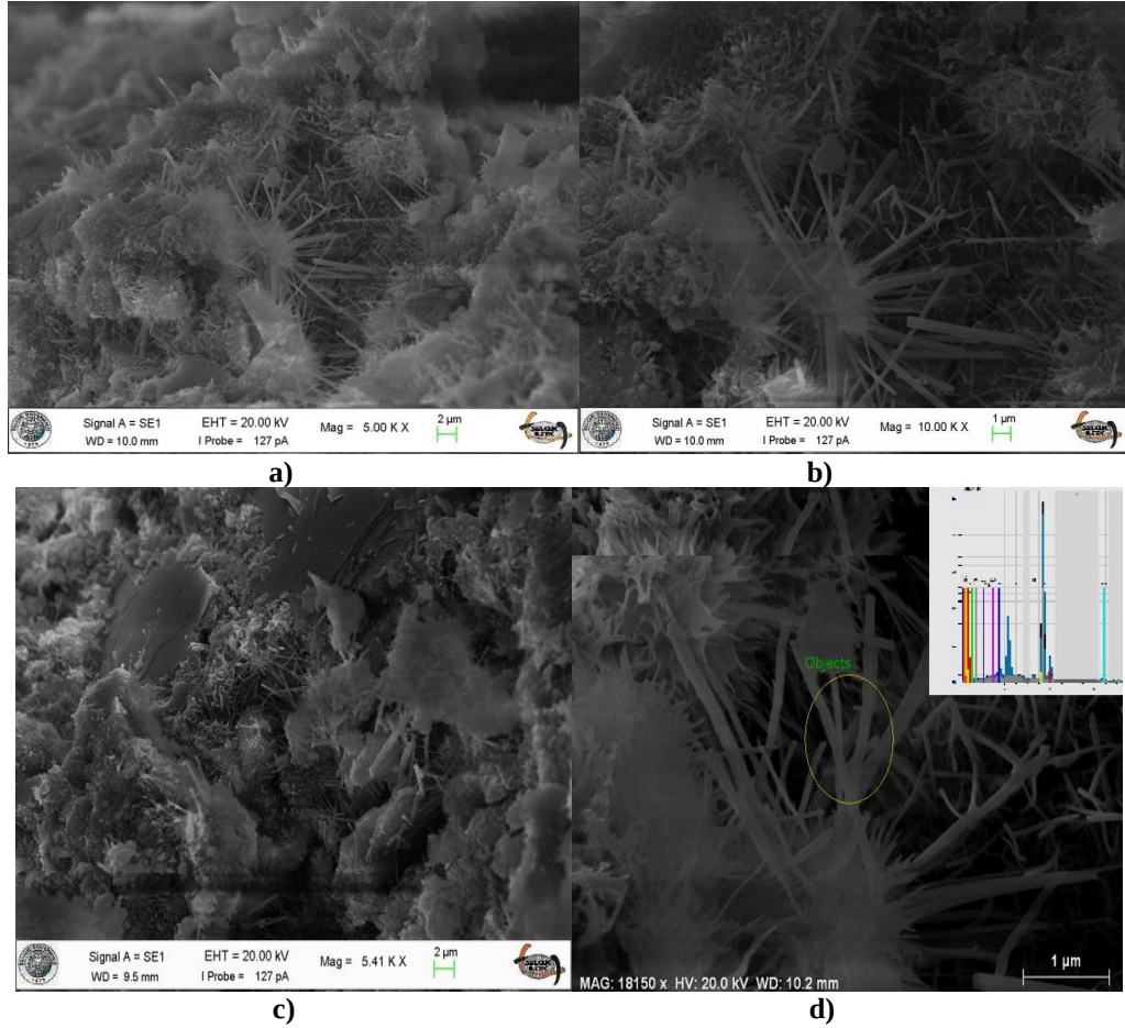
Şekil 4.9. a), b), c) NP-NMS (1) jet-grout kolonlarına ait numunelerden elde edilen SEM görüntüleri ve d) SEM analizi esnasında yapılan EDS analizi
