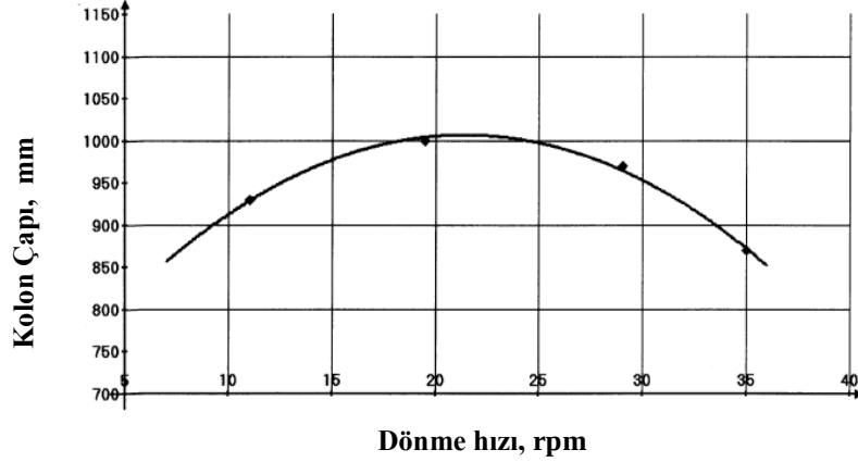
Şekil 2.8. Dönme hızının jet-grout kolon çapı üzerindeki etkisi (Malinin ve ark., 2010)
