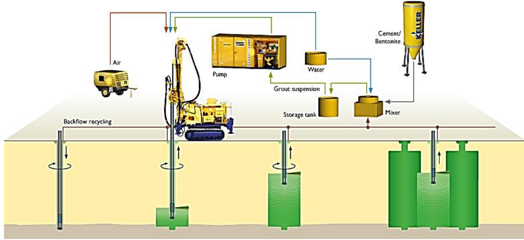
Şekil 3.3. Jet-grout ekipmanlarının şematik gösterimi (Keller-Ground-Engineering)
