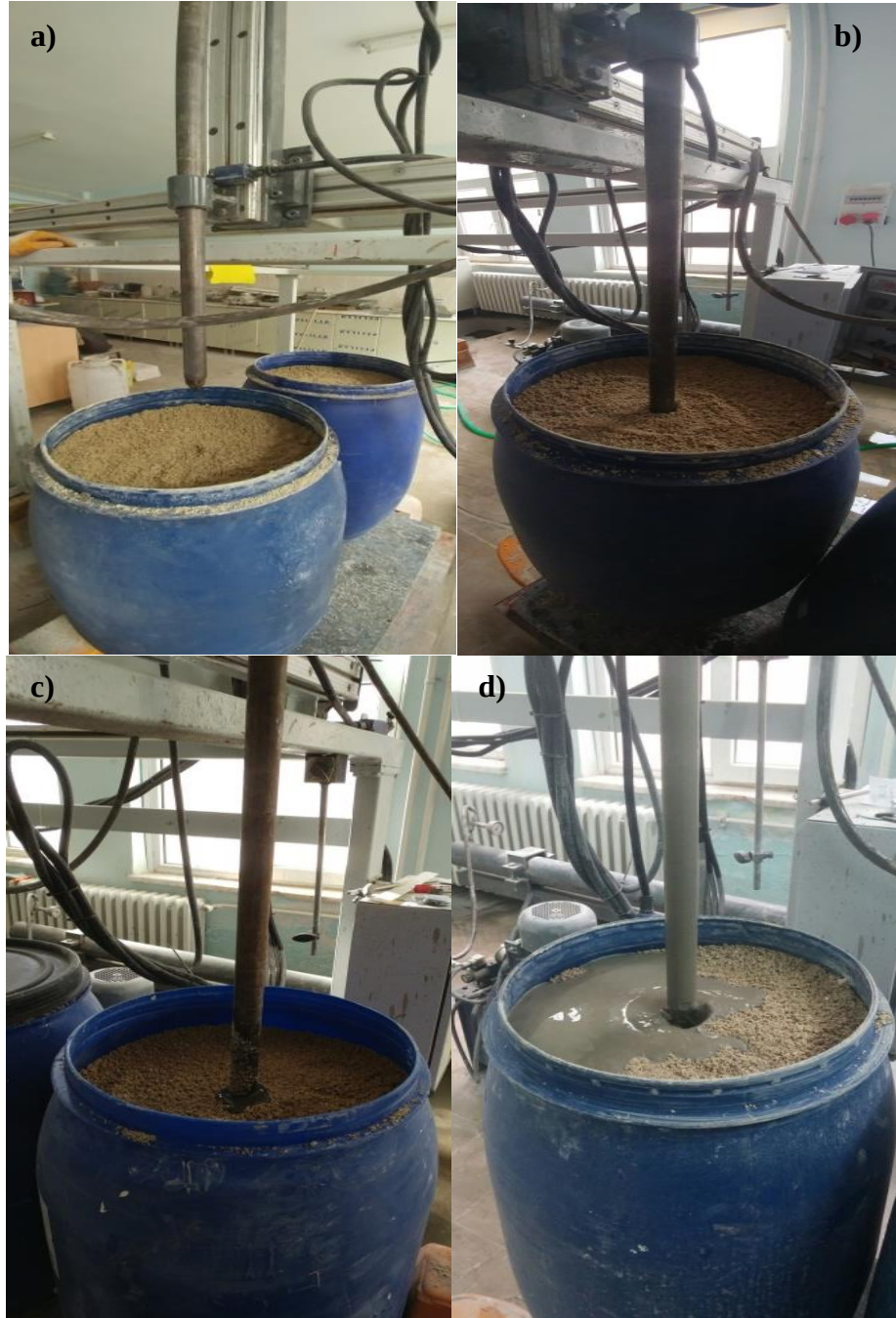
Şekil 3.35 a), b), c), d). Jet-grout kolon imalat aşamaları
