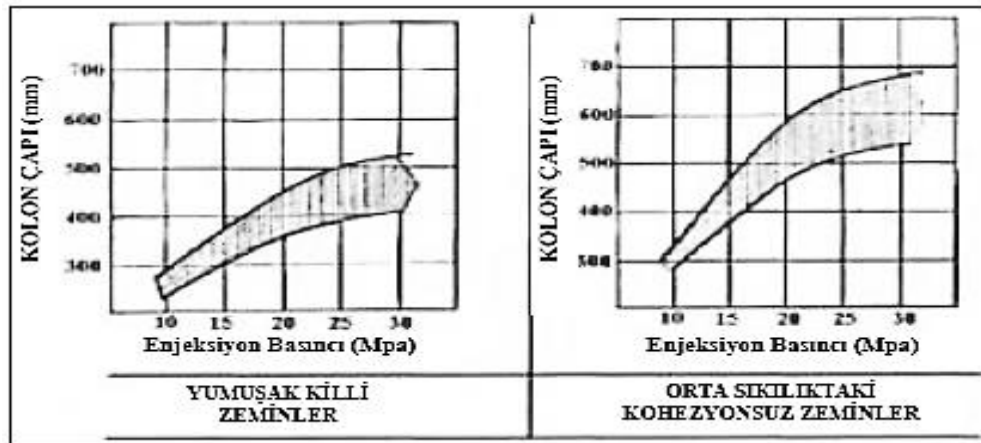
Şekil 3.9. Zemin tipine bağlı olarak oluşturulan kolon çapı ve enjeksiyon basıncı arasındaki ilişki (Xanthakos ve ark., 1994)
