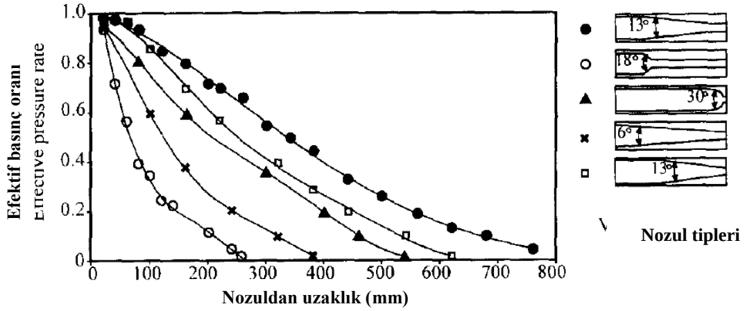
Şekil 3.11. Jet ekseninde nozul daralma açısının dinamik basınç üzerindeki etkisi (Shibazaki, 2003)
