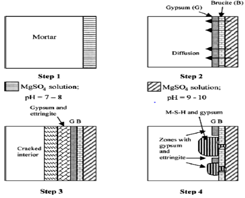
Şekil 3.24. Magnezyum sülfat saldırısı için (Santhanam ve ark., 2003) tarafından önerilen mekanizma şeması
