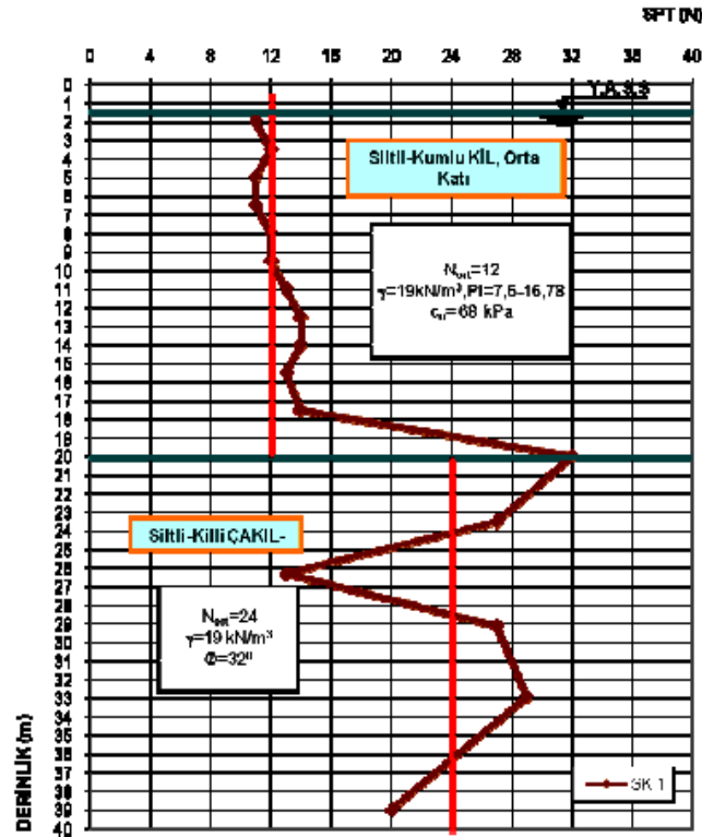
Şekil 2.3. Phase 6.018 programı için kullanılan idealize zemin profili ve mühendislik parametreleri (Küçükali, 2008)
