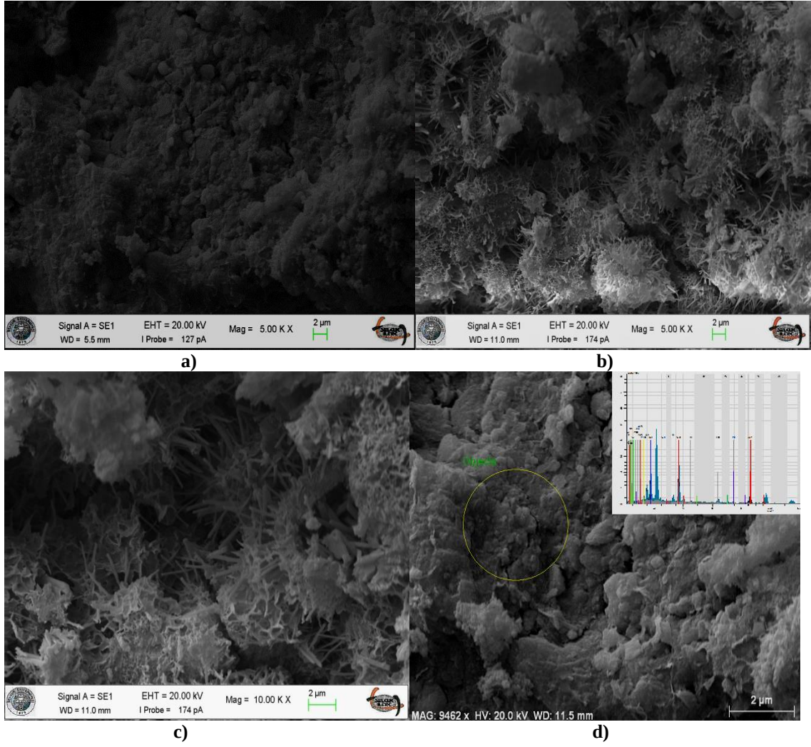
Şekil 4.10. NP-SYS (1) jet-grout kolonlarına ait numunelerden elde edilen SEM görüntüleri
