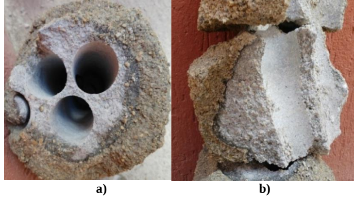
Şekil 4.4 a), b). Enine ve boyuna kesit alınan jet-grout kolonda iyi çimentolaşmış ve az çimentolaşmış bölgeler
