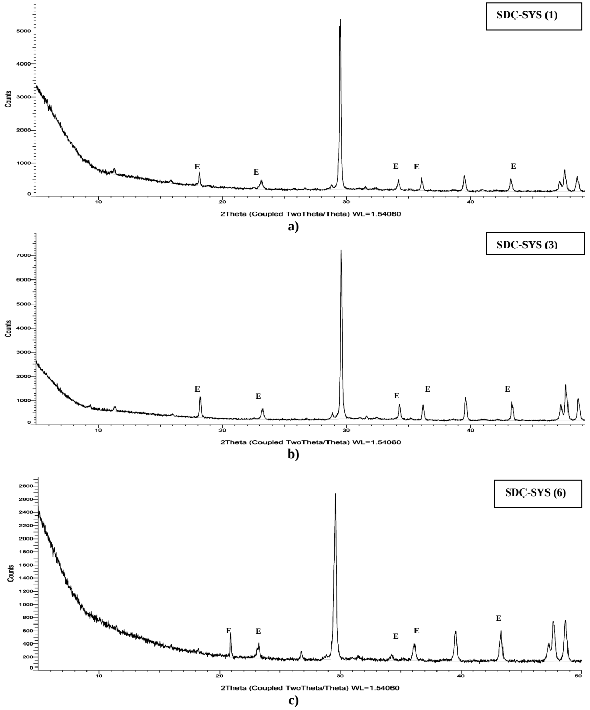
Şekil 4.21. a), b) ve c) Sülfata dayanıklı çimento ve sülfat içerikli yeraltı suyu kullanılarak oluşturulan jet-grout kolonların XRD analiz sonuçları
