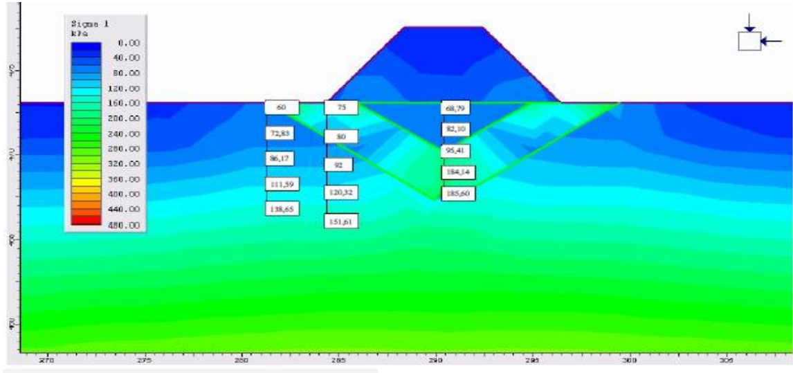
Şekil 2.5. İyileştirme sonrasında zeminde oluşan düşey gerilmeler (Küçükali, 2008)
