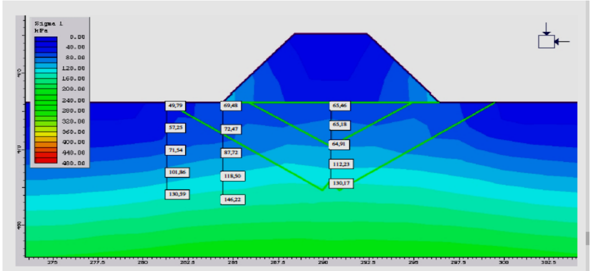
Şekil 2.4. İyileştirme öncesi zeminde oluşan düşey gerilmeler (Küçükali, 2008)
