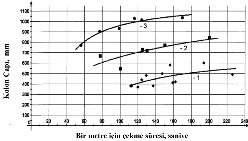
Şekil 2.6. Zemin iyileştirme süresinin jet-grout kolon çapı üzerindeki etkisi (Malinin ve ark., 2010) 1- kohezyonlu zemin ( c= 47 kPa), 2- düşük kohezyonlu zemin ( c= 7 kPa), 3- kohezyonsuz zemin ( c= 1 kPa)
