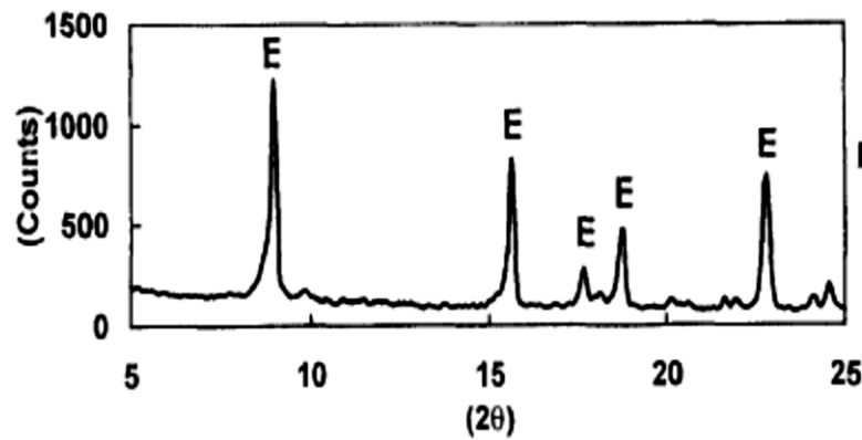
Şekil 4.17. Etrenjit mineralinin XRD pikleri (Felekoğlu, 2008)
