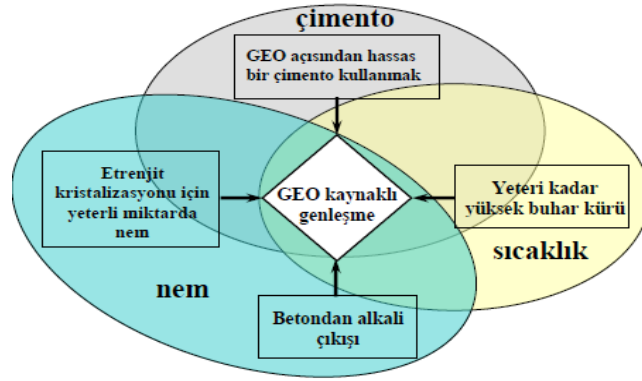
Şekil 3.22. Dış sülfat etkisi ile ilgili GEO (Gecikmiş Etrenjit Oluşumu) mekanizması (Tosun, 2007)
