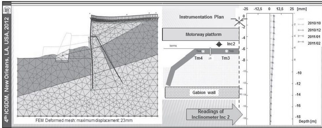
Şekil 2.10. Uygulanmış FEM analizi görünüşü ve yanal deplasmanlar (Pinto ve ark., 2012)
