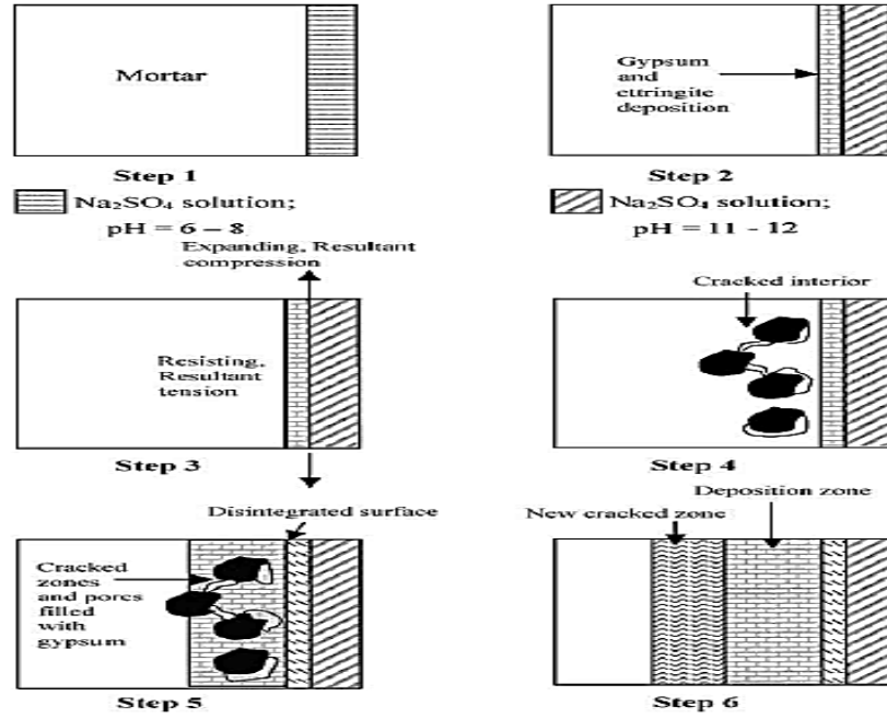
Şekil 3.23. Sodyum sülfat saldırısı için önerilen mekanizma şeması (Santhanam ve ark., 2003)
