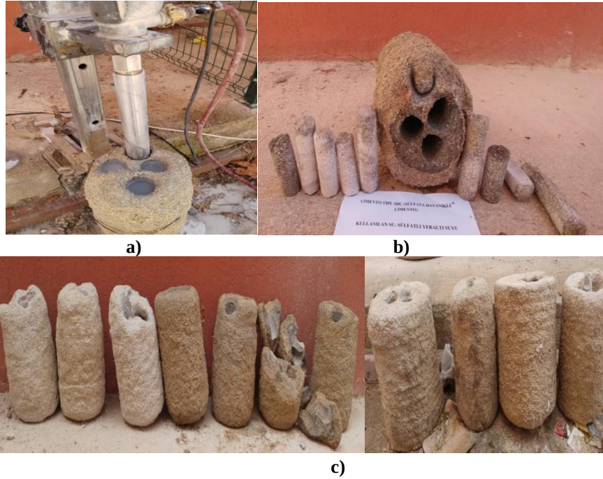
Şekil 4.3. a) Jet-grout kolonlardan karot alınması b) Jet-grout kolondan alınan karot numuneler c) Karot alınmış jet-grout kolonlar
