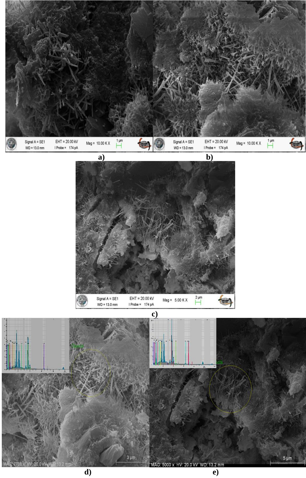
Şekil 4.11. NP-NMS (3) jet-grout kolonlarına ait numunelerden elde edilen SEM görüntüleri
