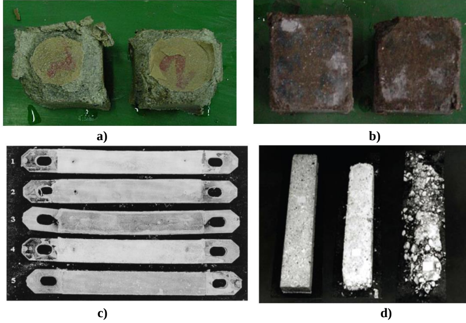
Şekil 3.26. Beton bozulma mekanizmasının fiziksel incelemesine ait literatürde yer alan fotoğraflar: a) ve b) (Lee ve ark., 2005), c) (Tian ve M.D., 2000) ve d) (Hartell, 2008)
