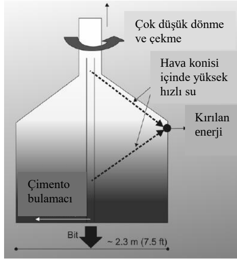
Şekil 3.8. X-Jet sisteminin şematik gösterimi (Burke, 2004)
