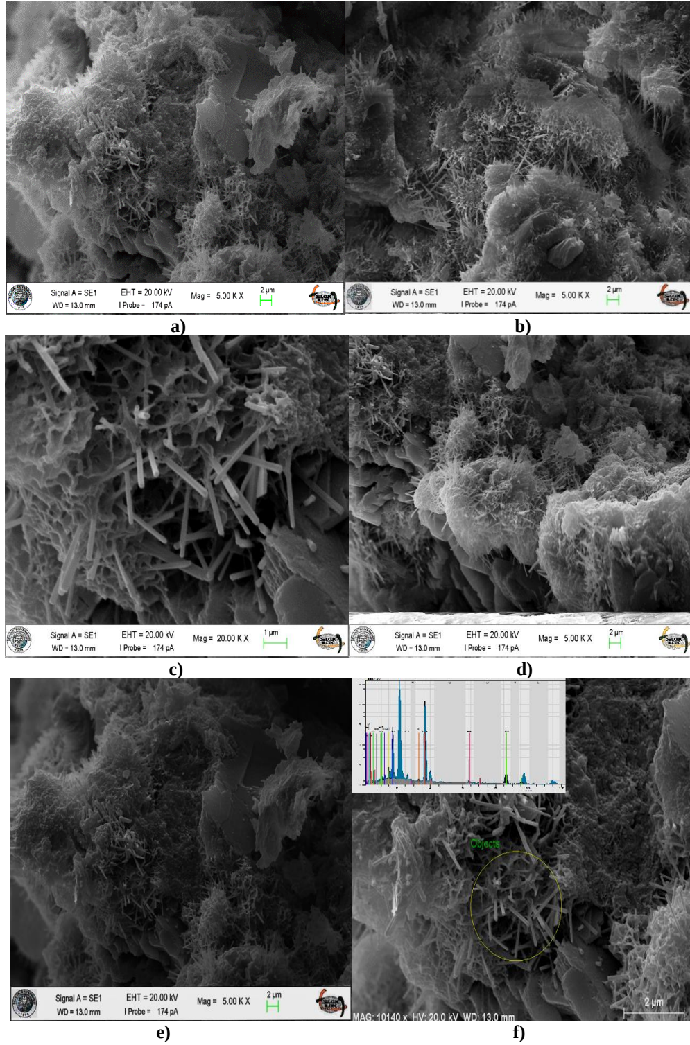
Şekil 4.12. NP-SYS (3) jet-grout kolonlarına ait numunelerden elde edilen SEM görüntüleri
