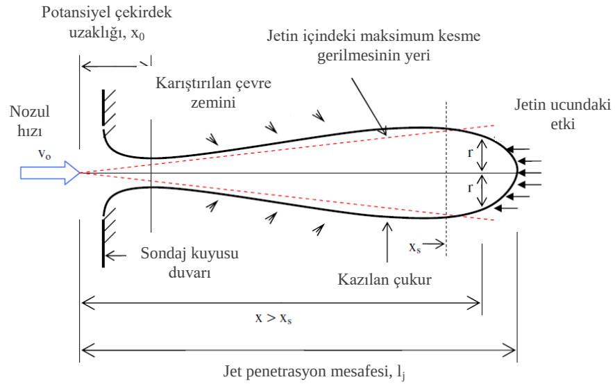
Şekil 2.2. Zemindeki jet penetrasyon modeli (Ho, 2007)
