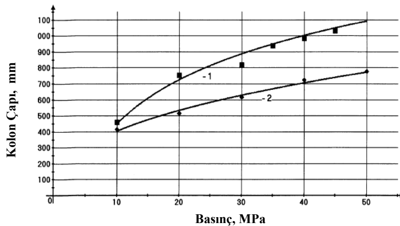
Şekil 2.7. Enjeksiyon basıncının jet-grout kolon çapı üzerindeki etkisi (Malinin ve ark., 2010) 1- kohezyonsuz zemin ( c=1 kPa), 2- düşük kohezyonlu zemin ( c= 7 kPa)
