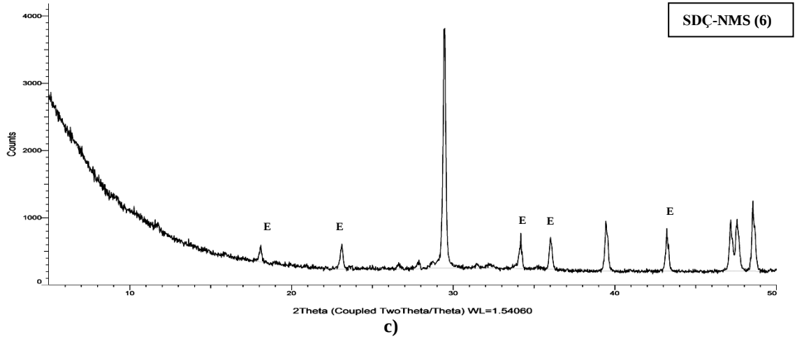
Şekil 4.20. a), b) ve c) Sülfata dayanıklı çimento ve normal musluk suyu kullanılarak oluşturulan jet-grout kolonların XRD analiz sonuçları
