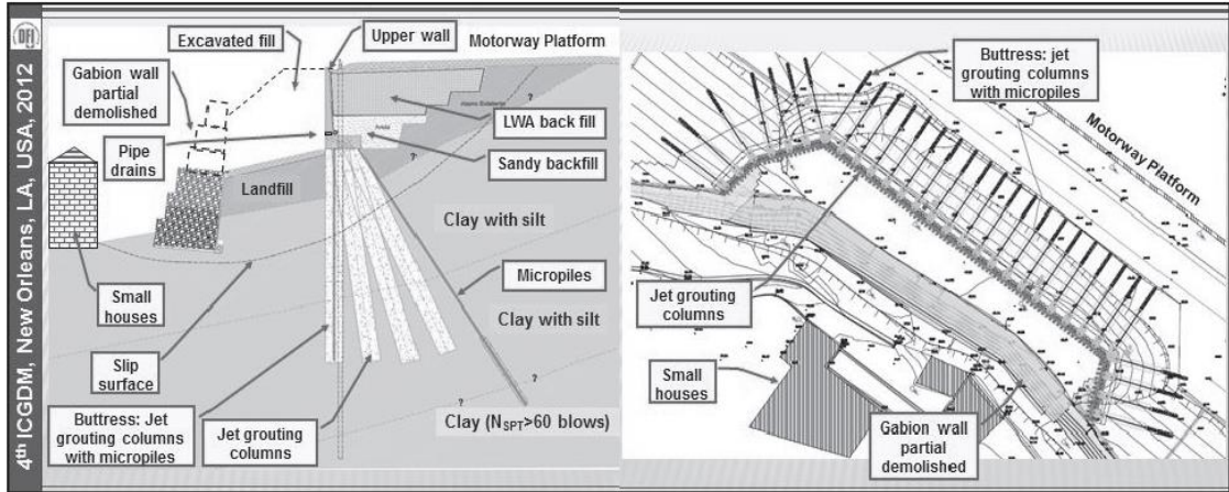
Şekil 2.9. Uygulanan iyileştirmenin plan ve en kesiti (Pinto ve ark., 2012)
