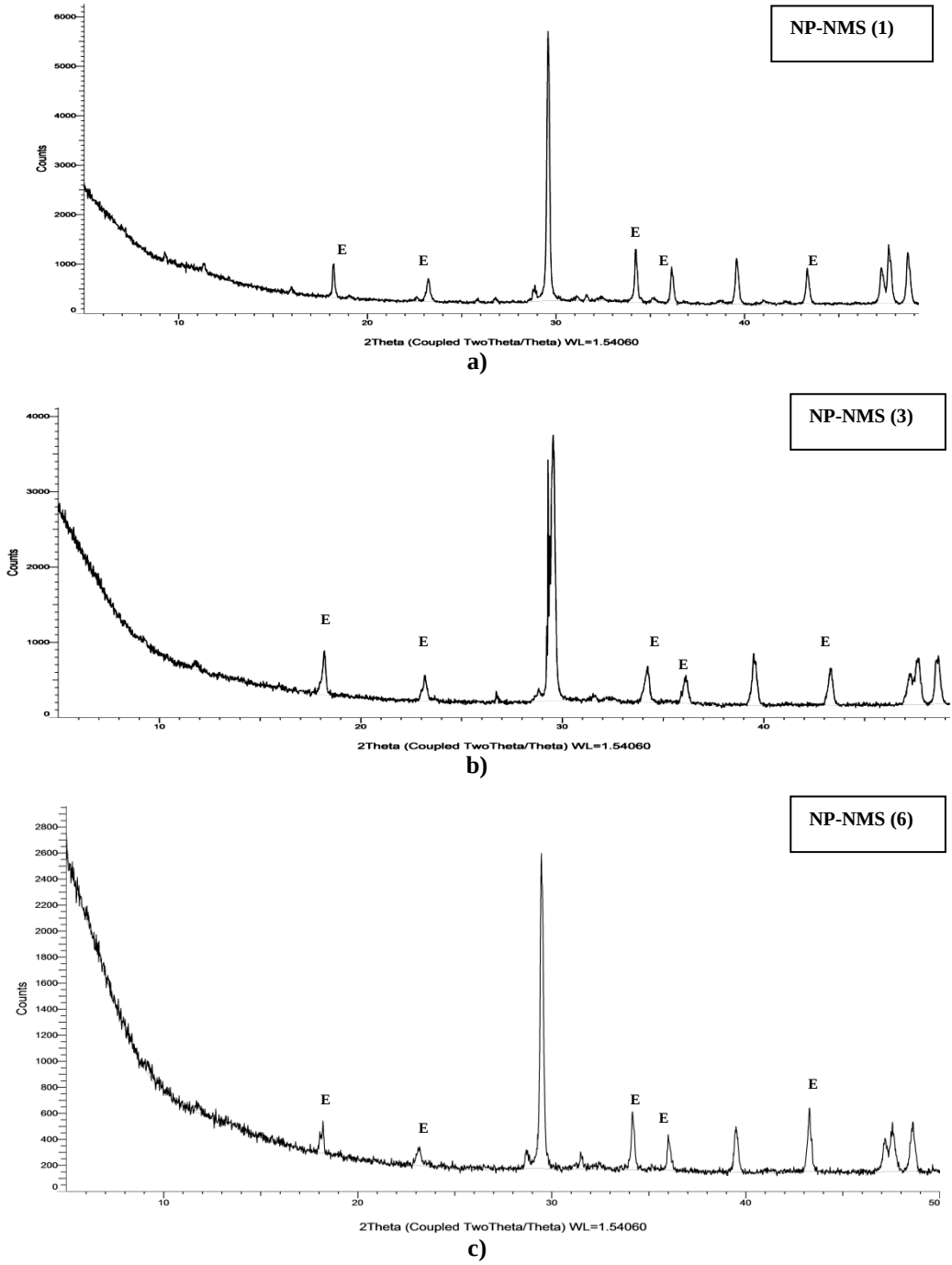
Şekil 4.18. a), b) ve c) Normal portland çimentosu ve normal musluk suyu kullanılarak oluşturulan jet-grout kolonların XRD analiz sonuçları
