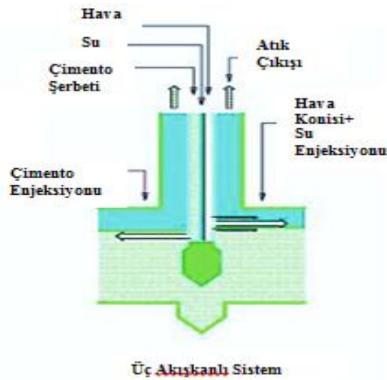
Şekil 3.7. Üç akışkanlı jet-grout sisteminin şematik gösterimi (Keller-Ground-Engineering)
