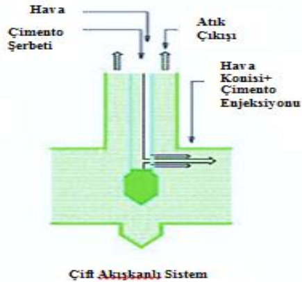
Şekil 3.6. Çift akışkanlı jet-grout sisteminin şematik gösterimi (Keller-Ground-Engineering)
