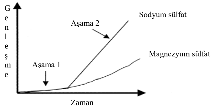
Şekil 2.12. Na_2SO_4 ve MgSO_4 çözeltilisine maruz Portland çimentolu numunelerin idealize genleşme davranışı (Aşama 1 ve Aşama 2 Na_2SO_4 çözeltisi için) (Santhanam ve ark., 2002)
