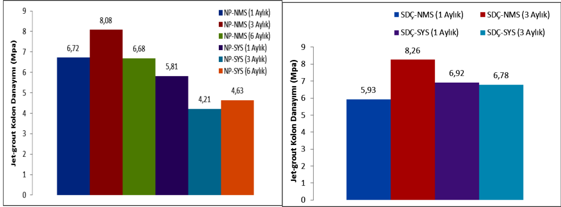
Şekil 4.7. Normal portland çimentosu ve sülfata dayanıklı çimento kullanılarak oluşturulan jet-grout kolon dayanımlarının kullanılan kür suyu ve kür süresine bağlı değişiminin grafik gösterimi
