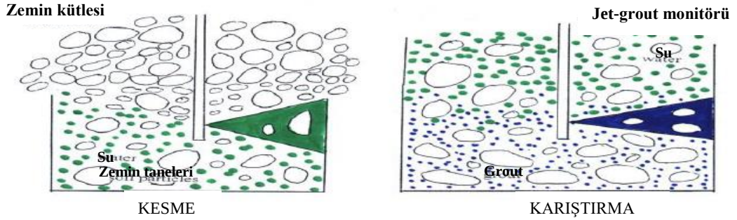
Şekil 3.1. Jet-grout enjeksiyonu ile zemin kütlesinin parçalanıp, karıştırılmasının şematik gösterimi (Chan, 2005)
