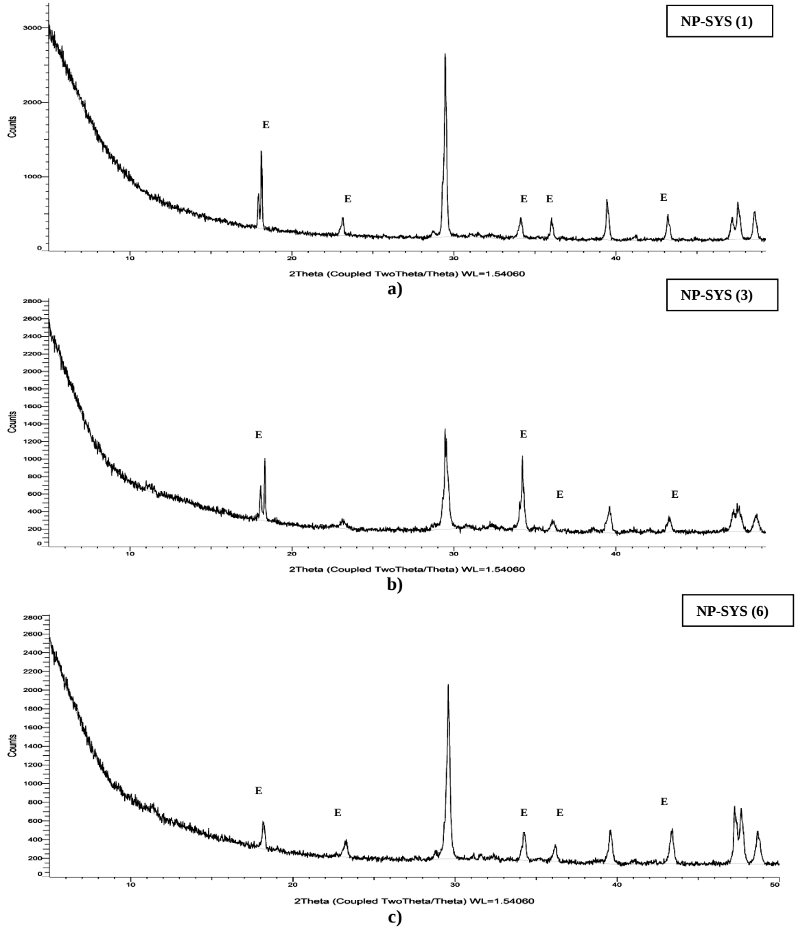
Şekil 4.19. a), b) ve c) Normal portland çimentosu ve sülfat içerikli yeraltı suyu kullanılarak oluşturulan jet-grout kolonların XRD analiz sonuçları
