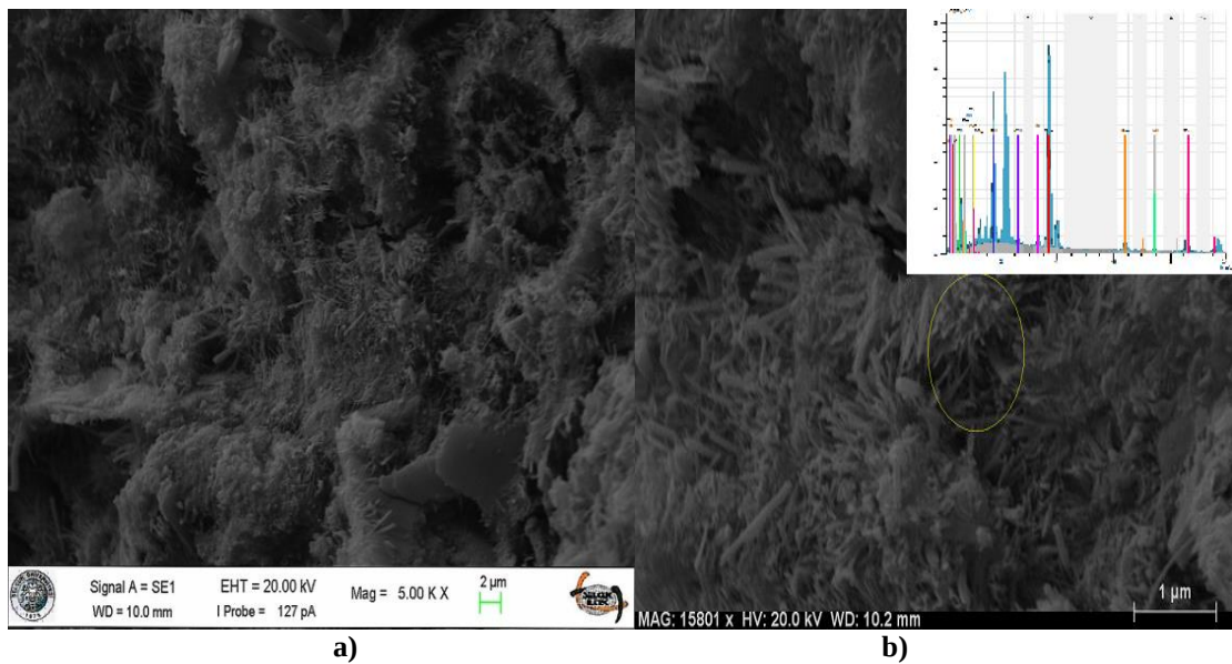
Şekil 4.15. SDÇ-NMS (3) jet-grout kolonlarına ait numunelerden elde edilen SEM görüntüleri
