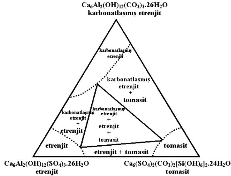
Şekil 3.19. 20°C’de Etrenjit Yapılı Fazların Stabilité Diyagramı (Tosun, 2007)
