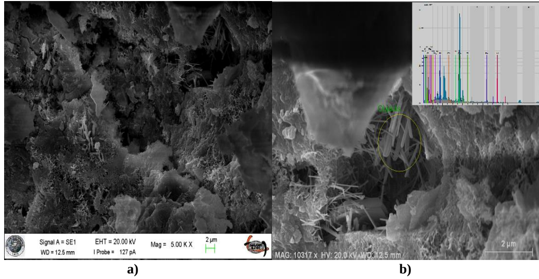
Şekil 4.14. SDÇ-SYS (1) jet-grout kolonlarına ait numunelerden elde edilen SEM görüntüleri
