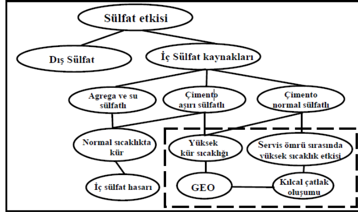
Şekil 3.21. Klasik iç sülfat etkisi ve GEO gruplandırılması (Tosun, 2007)
