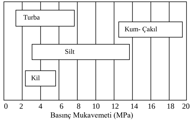
Şekil 2.1. Jet-grout yöntemi ile iyileştirilmiş zeminlerin basınç dayanımları (Lunardi, 1997)
