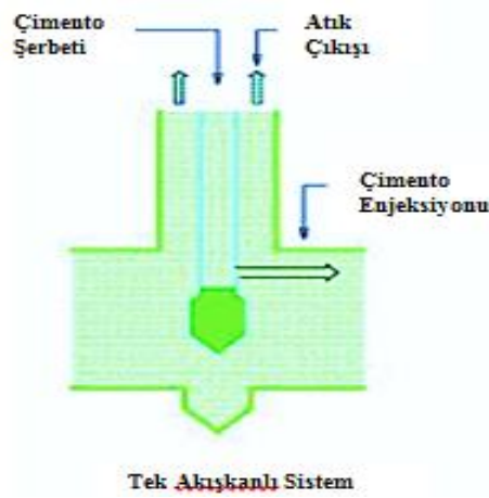
Şekil 3.5. Tek akışkanlı jet-grout sisteminin şematik gösterimi (Keller-Ground-Engineering)
