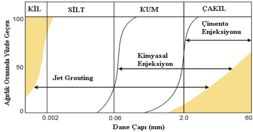
Şekil 3.14. Zemin cinslerine göre enjeksiyon uygulama aralığı (Keller)
