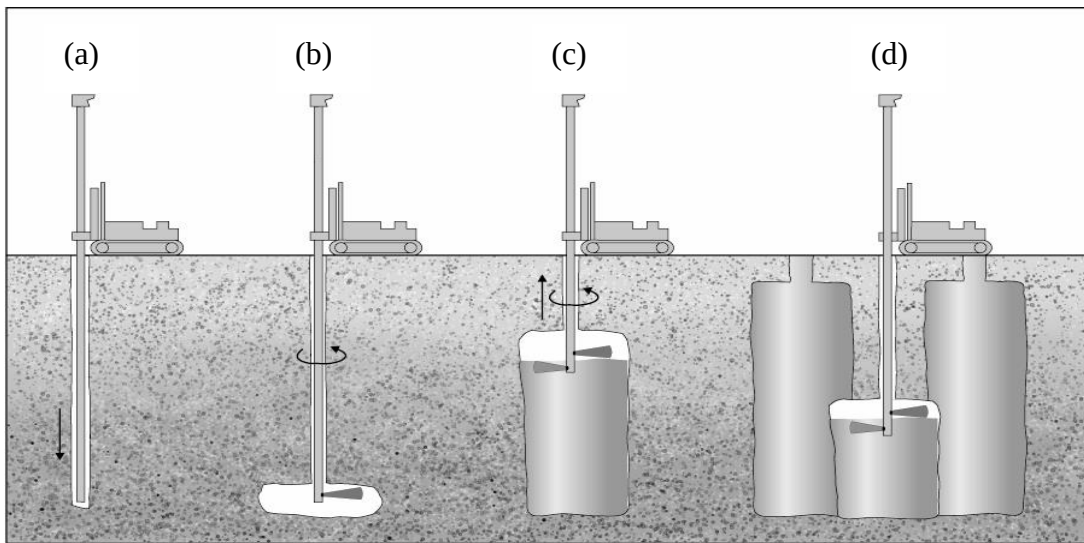
Şekil 3.2. Jet-grout yönteminin aşamalarının şematik gösterimi: (a) Tijin sondaj ile belli derinliğe indirilmesi (delgi aşaması), (b), (c) ve (d) Enjeksiyon ile kolon imalatı (Burke, 2004)
