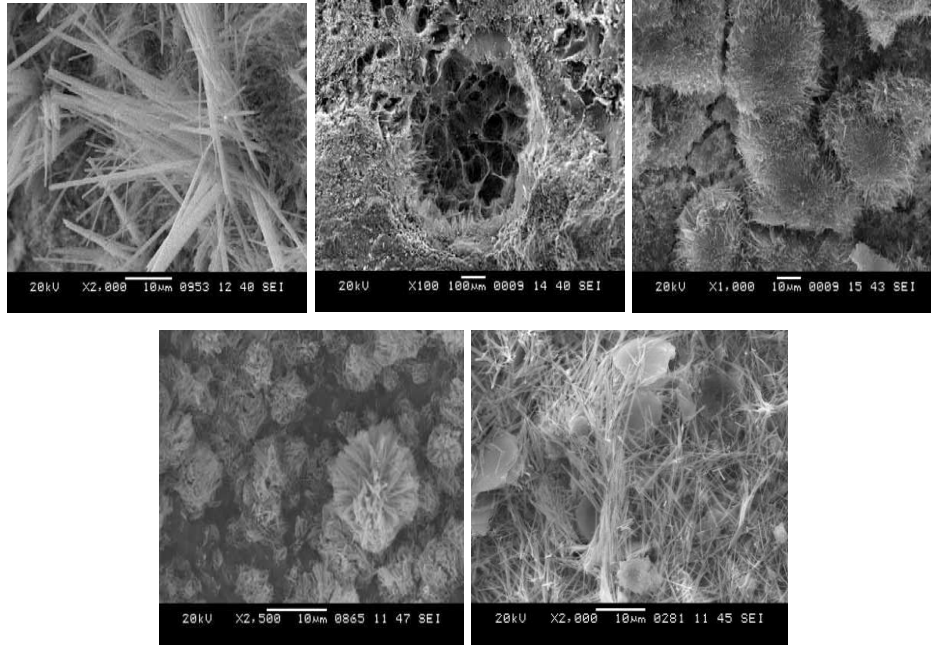
Şekil 3.18. Farklı morfolojik formlara sahip etrenjit kristallerinin SEM görüntüsü (Tosun, 2007)
