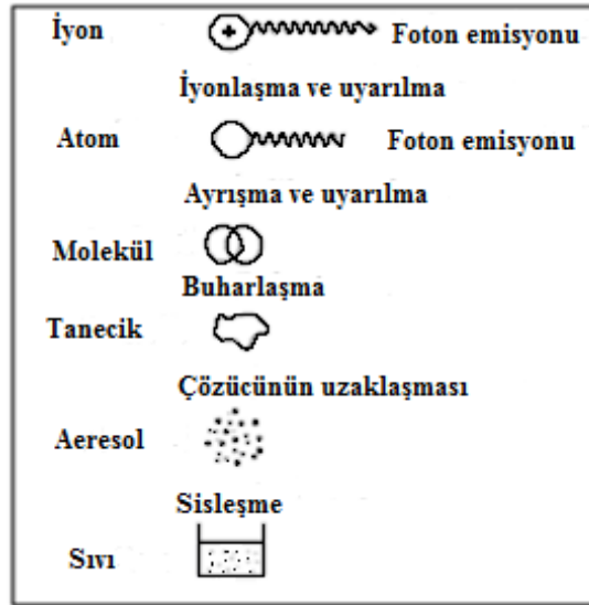
Şekil 3.3. Atomlaşma ve uyarılmanın şematik gösterimi [34]
