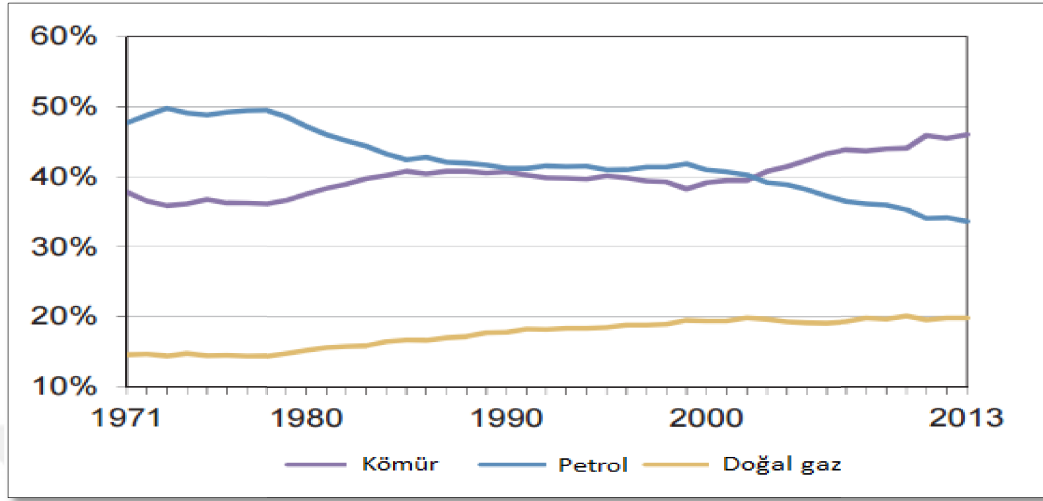
Şekil 8. Küresel Karbondioksit Salınımında Yakıtların Payları, 1971-2013
