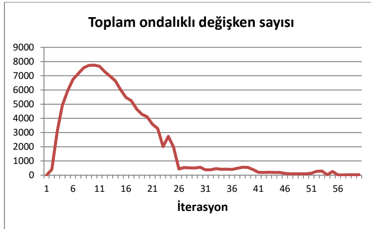
Şekil 4.10 : Optimizasyon süresince ondalıklı değişken sayısının değişimi.
