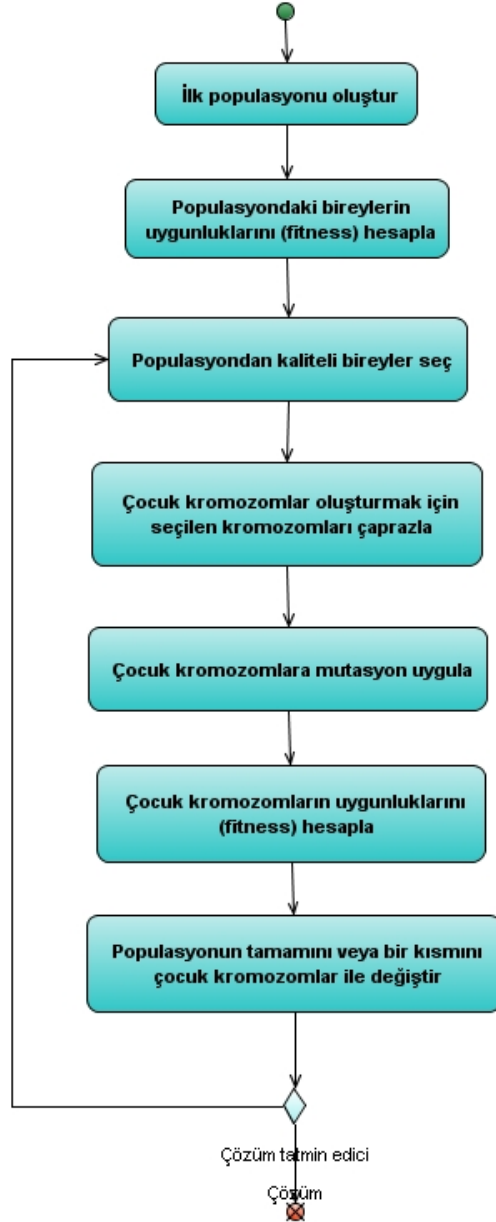
Şekil 2.1 : Temel genetik algoritma döngüsü.
