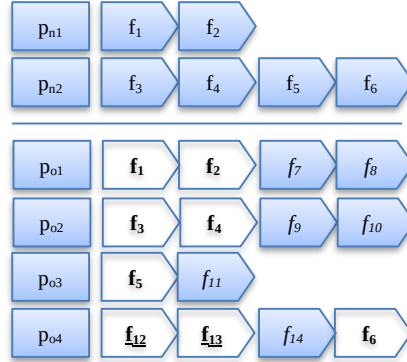
Şekil 4.5 : İterasyonlar arası ekip eşleme karşılaştırması.
