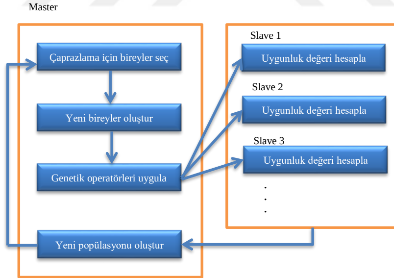
Şekil 2.7 : Global populasyon modeli (Master-Slave).
