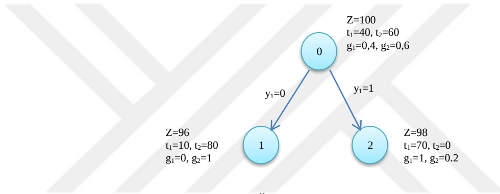
Şekil 3.1 : Örnek dal-sınır düğümü.
