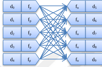
Şekil 4.3 : Tam-bağlı görev ağı örneği.
