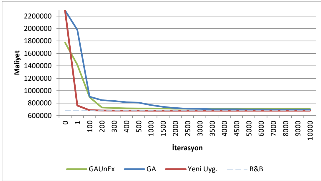
Şekil 2.6 : İterasyon ve maliyet değişimi karşılaştırması.
