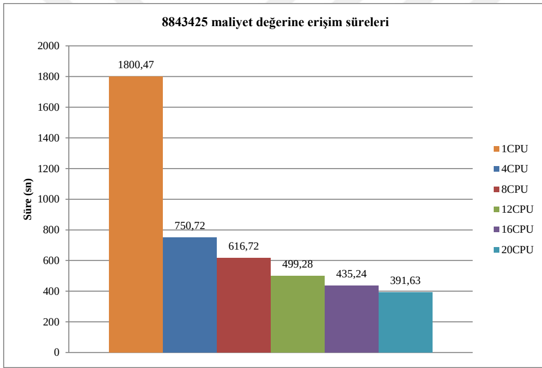
Şekil 2.11 : Farklı CPU sayıları ile 737 çözümü performans karşılaştırması.
