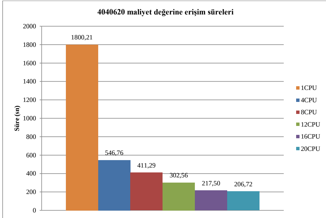
Şekil 2.10 : Farklı CPU sayıları ile 320 çözümü performans karşılaştırması.
