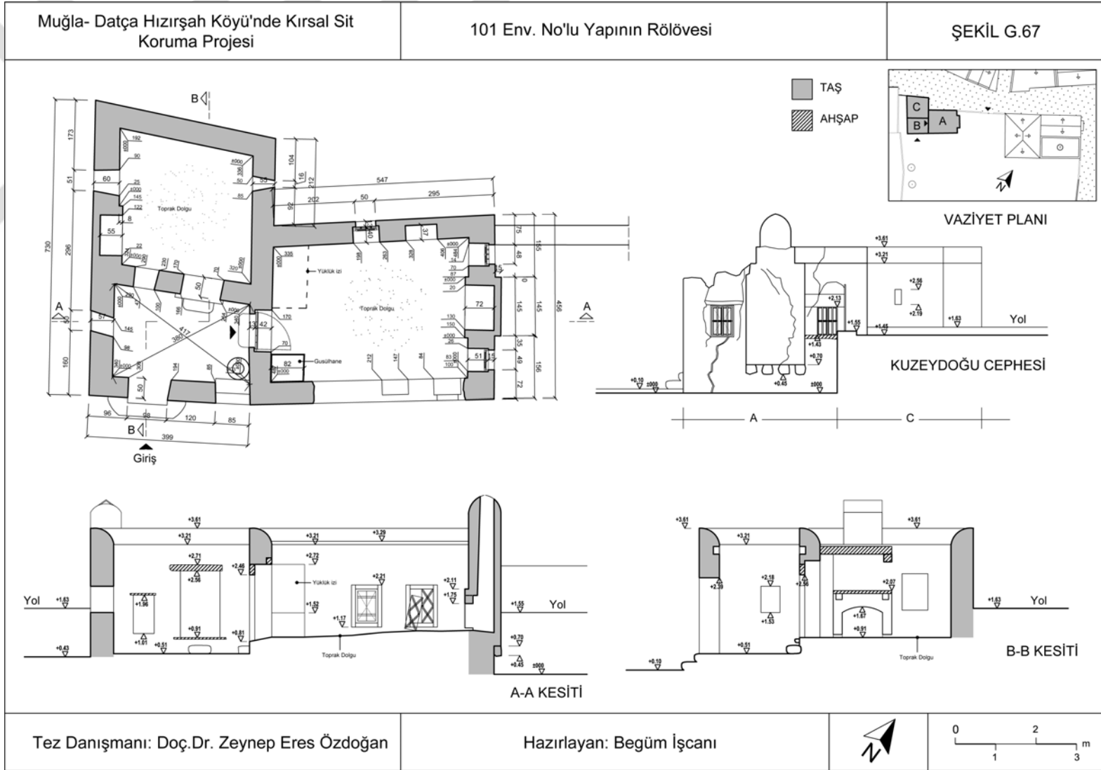
Şekil G.67 : 101 Env. No'lu Konutun Rölövesi.
