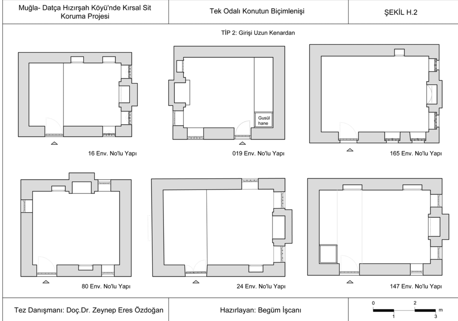
Şekil H.2 : Girişi uzun kenardan tek odalı konutun plan biçimlenişi.
