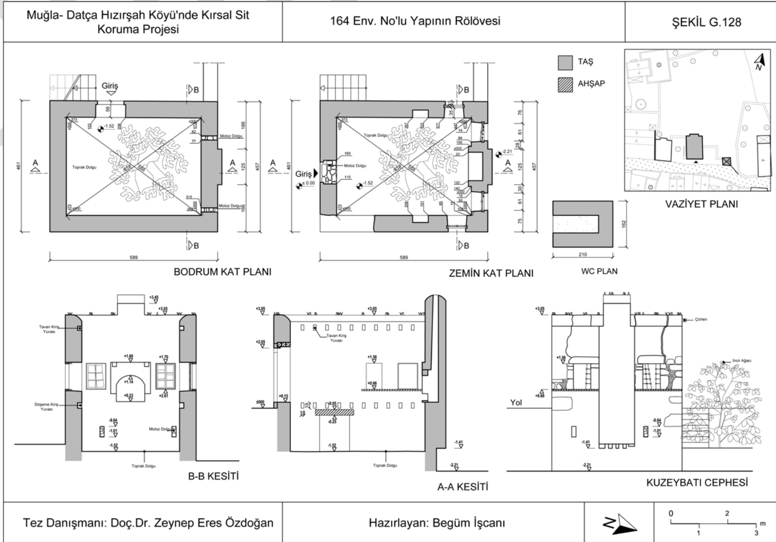
Şekil G.128 : 164 Env. No'lu Konutun Rölövesi.
