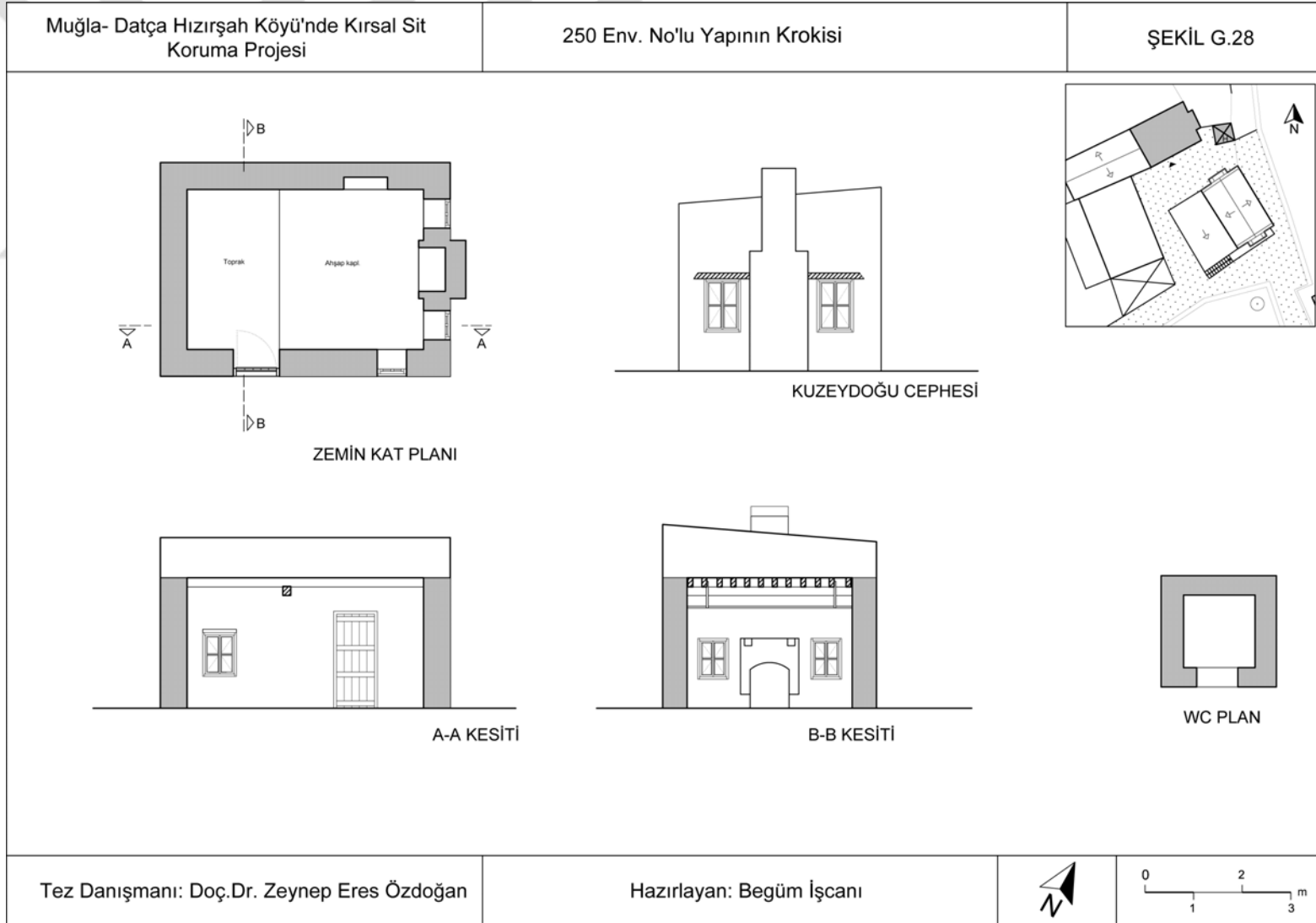
Şekil G.28 : 250 Env. No'lu yapının krokisi.
