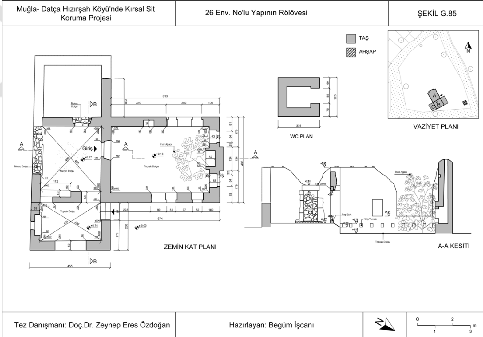
Şekil G.85 : 26 Env. No'lu Konutun Rölövesi.
