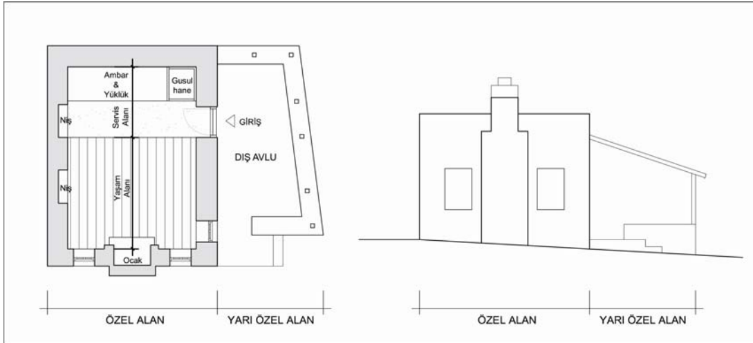
Şekil 2.4 : Datça Yarımadası'nda yaygın görülen tek odalı konutun plan ve cephesi, Hızırşah Köyü.
