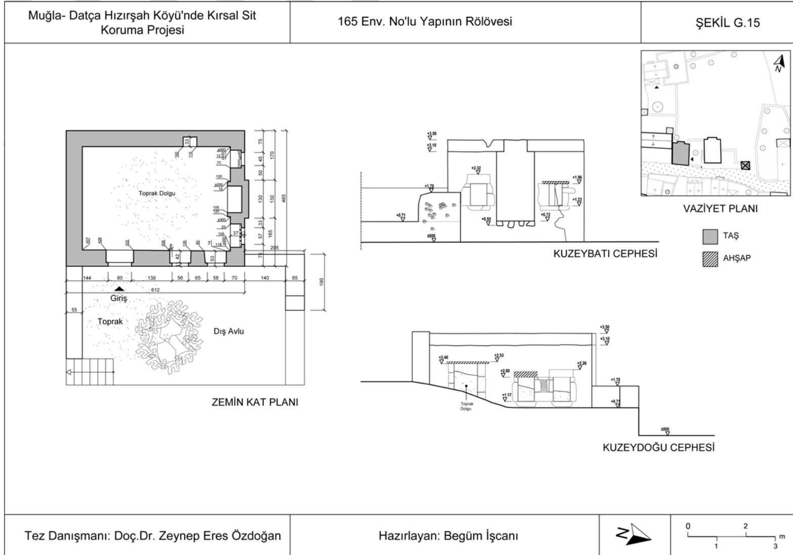
Şekil G.15 : 165 Env. No'lu yapının rölövesi.
