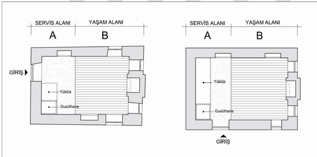
Şekil 5.2 : Kısa ve uzun kenardan girilen tek mekanlı konut planları (163 ve 147 Env. no'lu yapılar).
