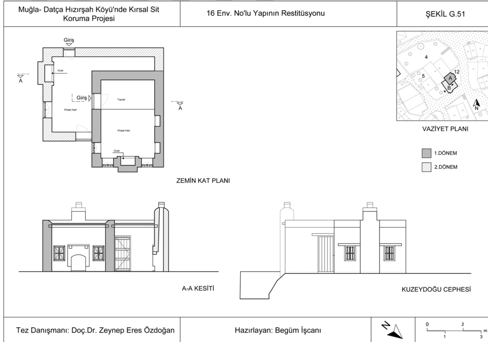
Şekil G.51 : 16 Env. No'lu Konutun Restitüsyonu.
