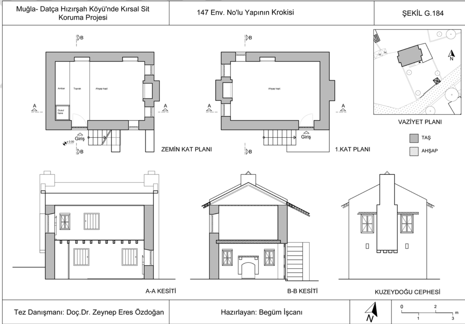
Şekil G.184 : 147 Env. No'lu Konutun Krokisi.
