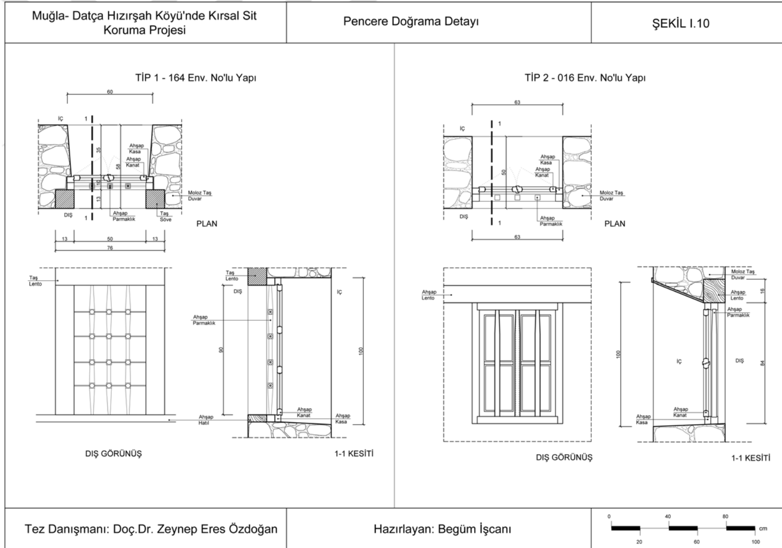
Şekil I.10 : Pencere doğrama detayı.
