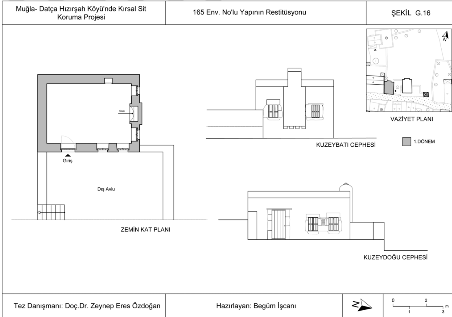
Şekil G.16 : 165 Env. No'lu yapının restitüsyonu.
