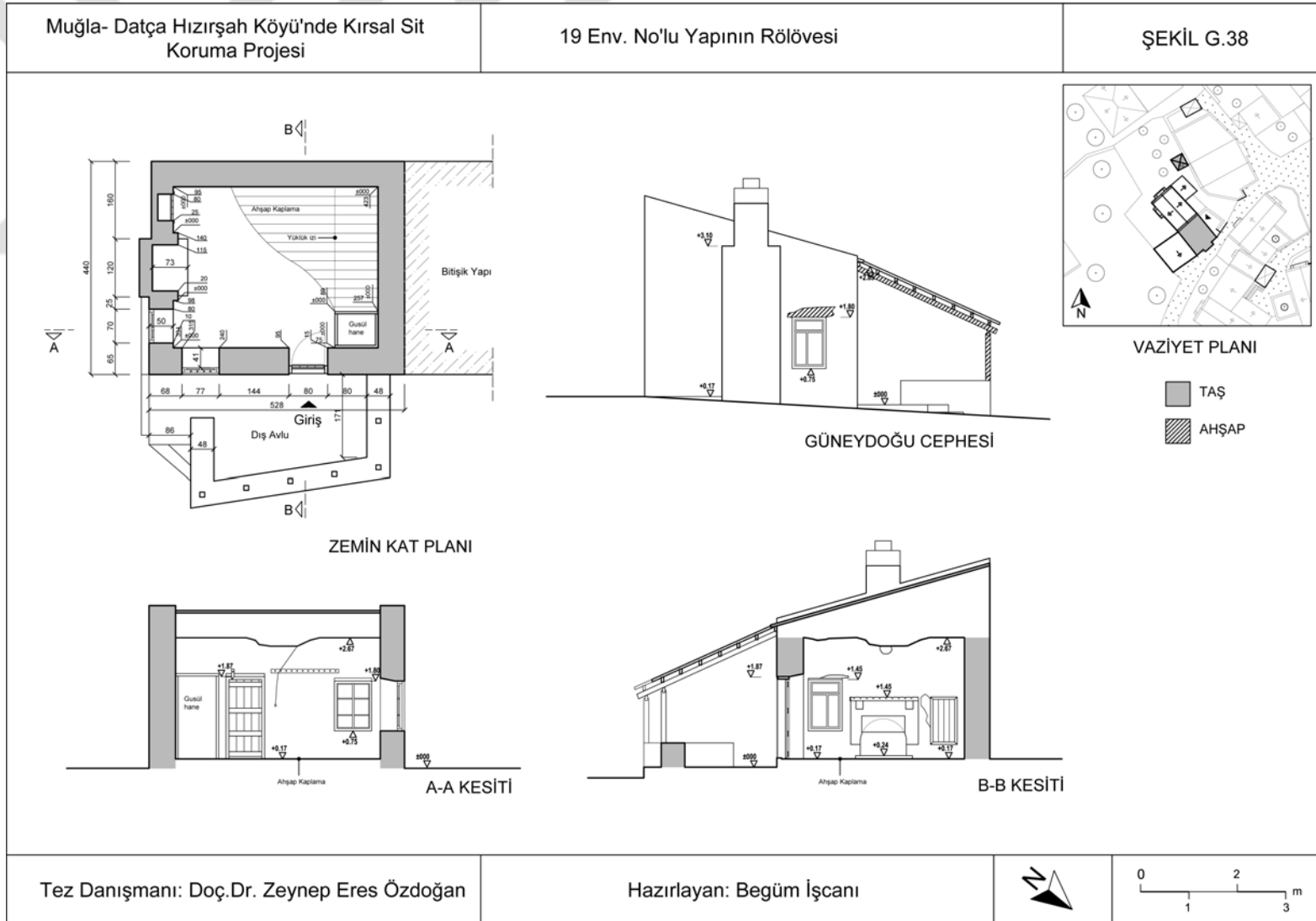
Şekil G.38 : 19 Env. No'lu Konutun Rölövesi.
