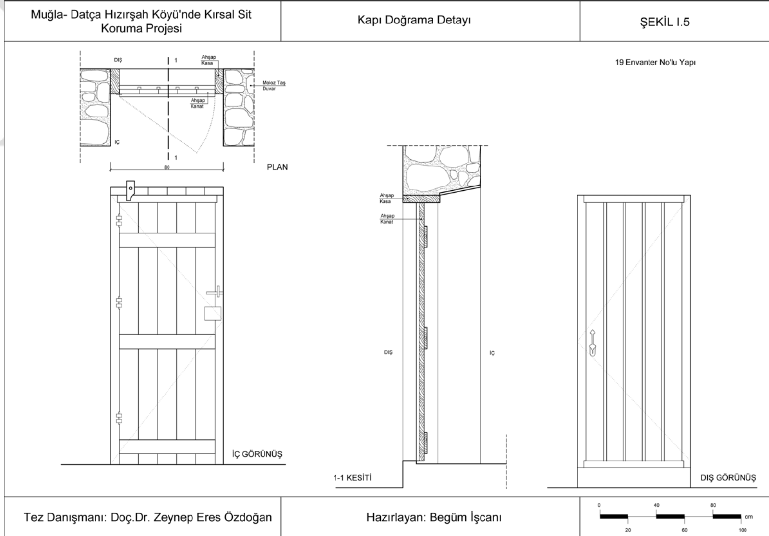
Şekil I.5 : Yaygın kullanılan kapının plan, kesit ve görünüşü.
