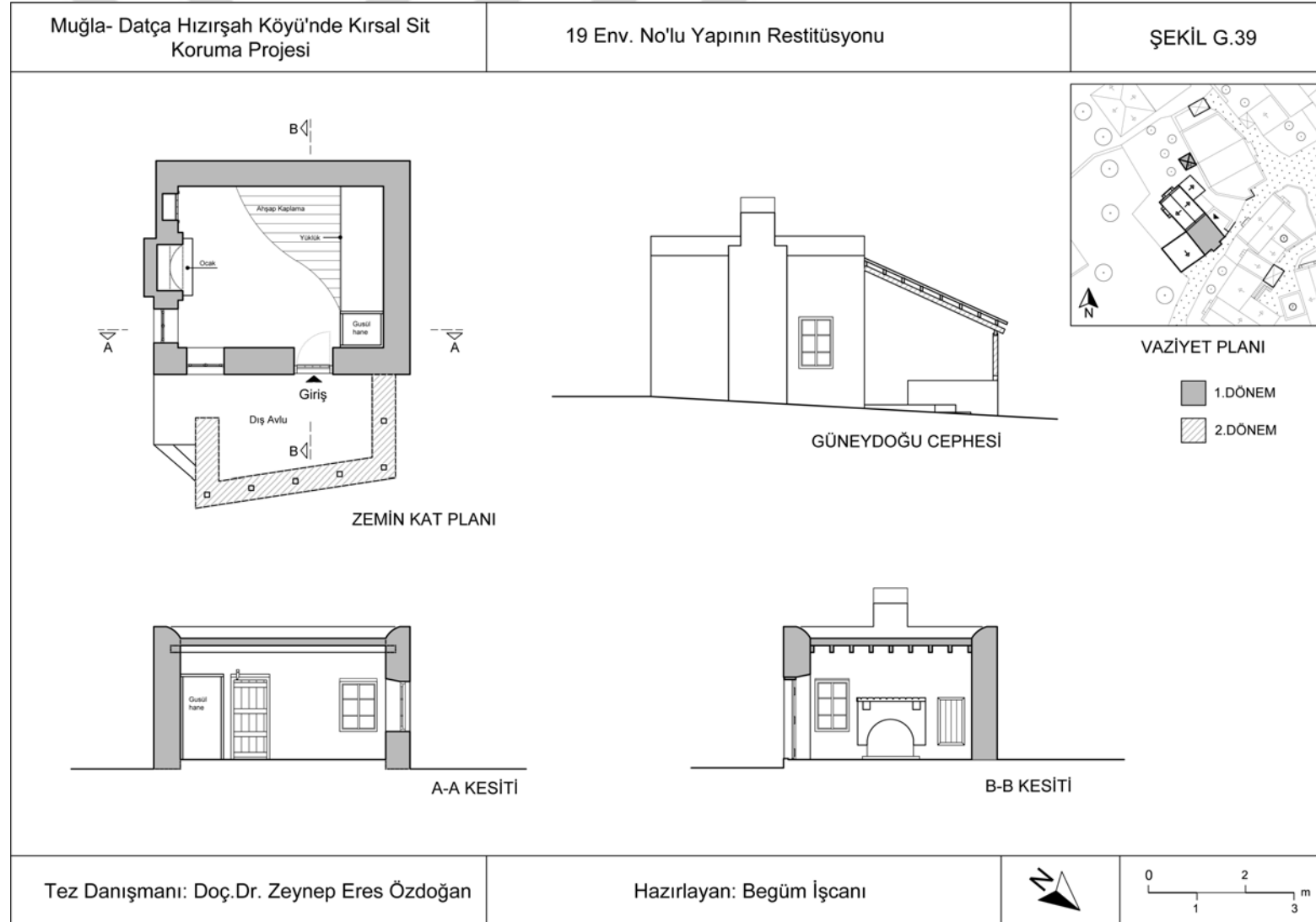
Şekil G.39 : 19 Env. No'lu Konutun Restitüsyonu.
