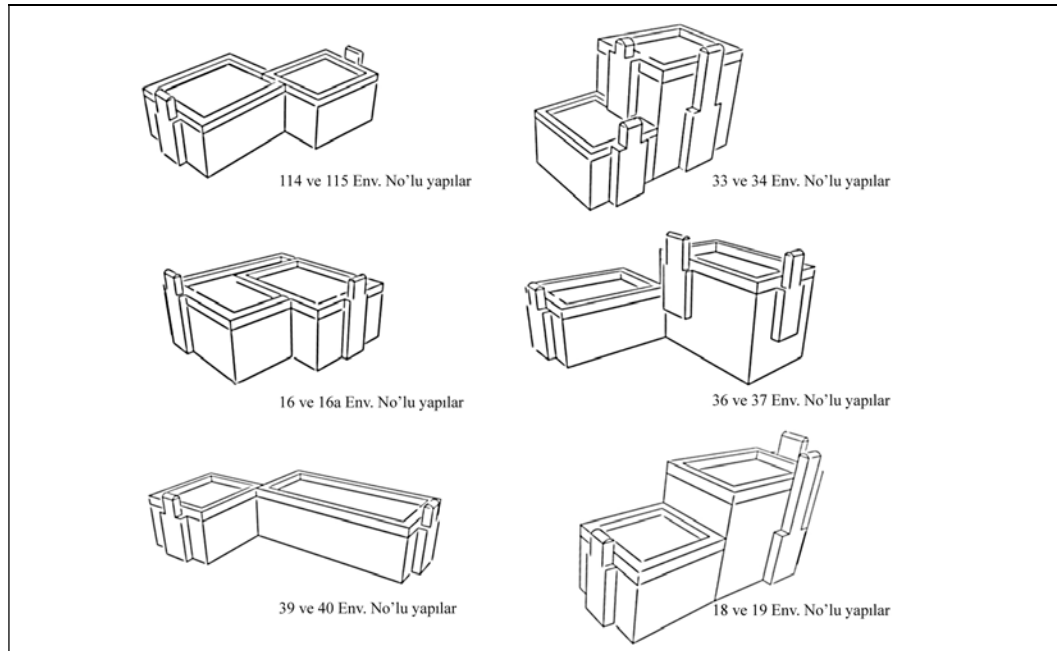
Şekil 5.17 : Tek odalı konuta ikinci odanın eklenmesi, Hızırşah Köyü.
