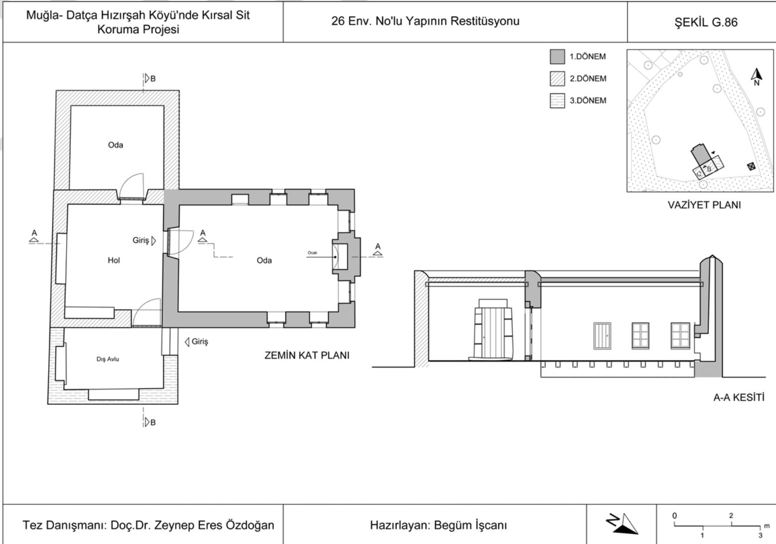
Şekil G.86 : 26 Env. No'lu Konutun Restitüsyonu.
