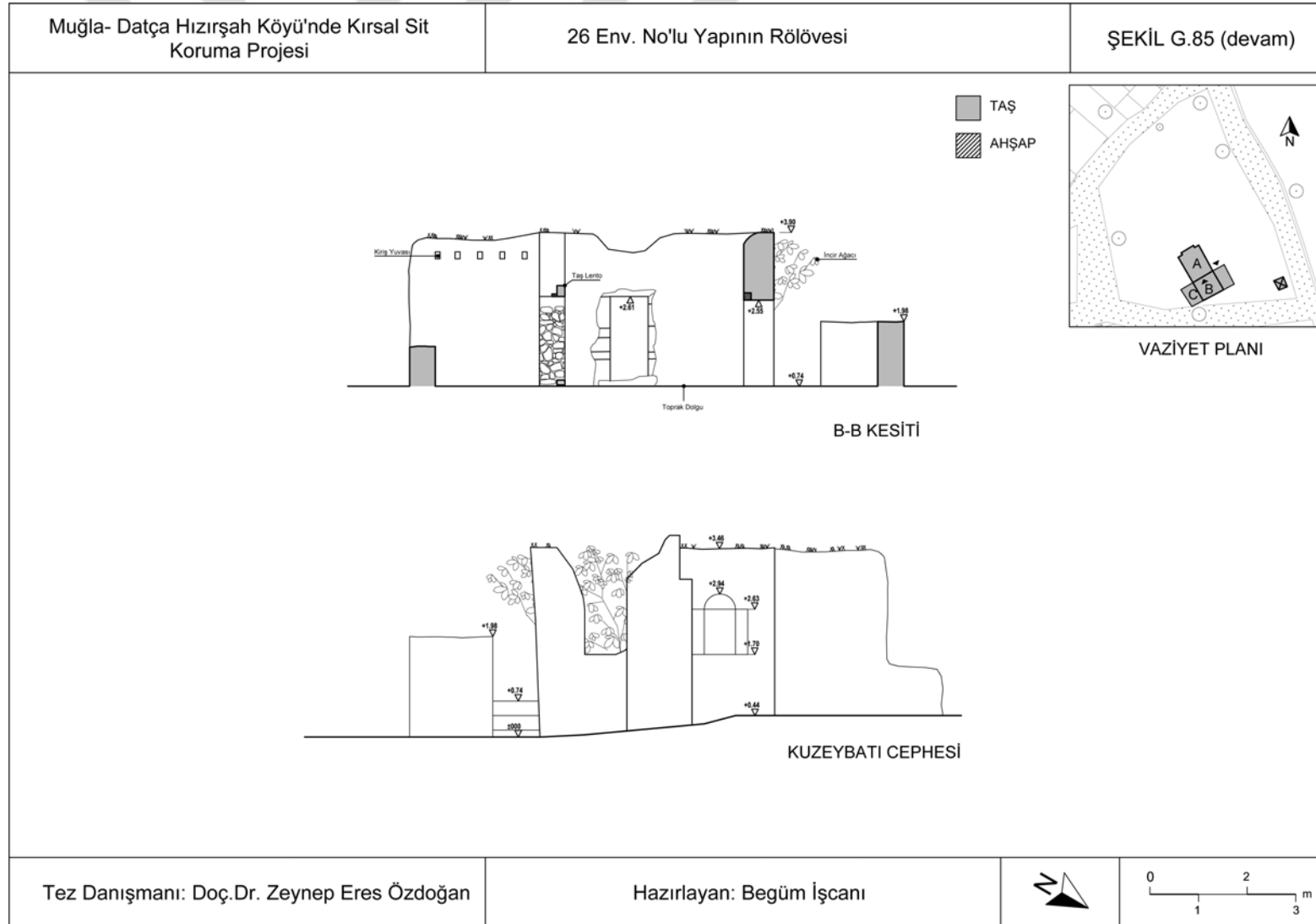
Şekil G.85 (devam) : 26 Env. No'lu Konutun Rölövesi.
