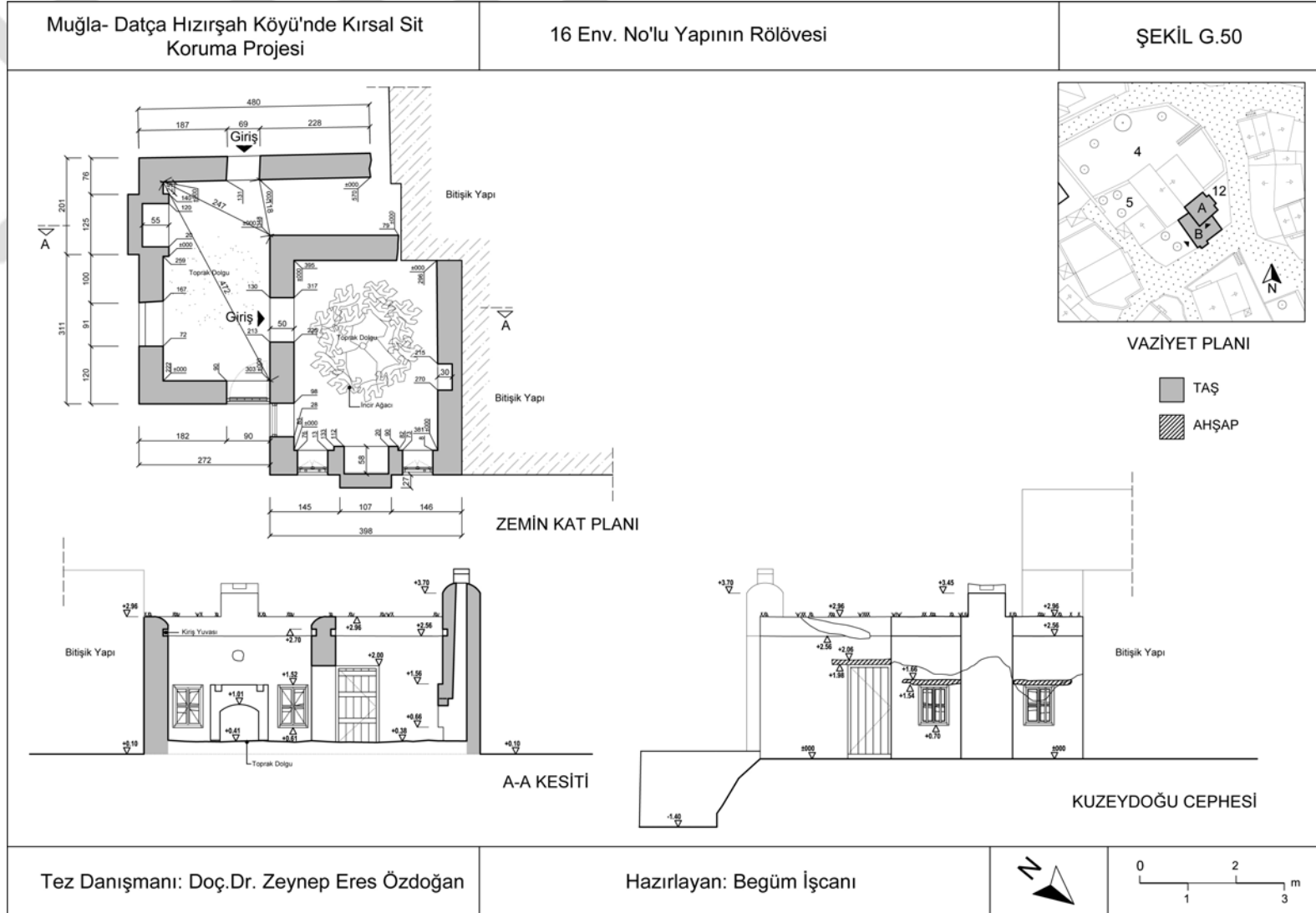
Şekil G.50 : 16 Env. No'lu Konutun Rölövesi.
