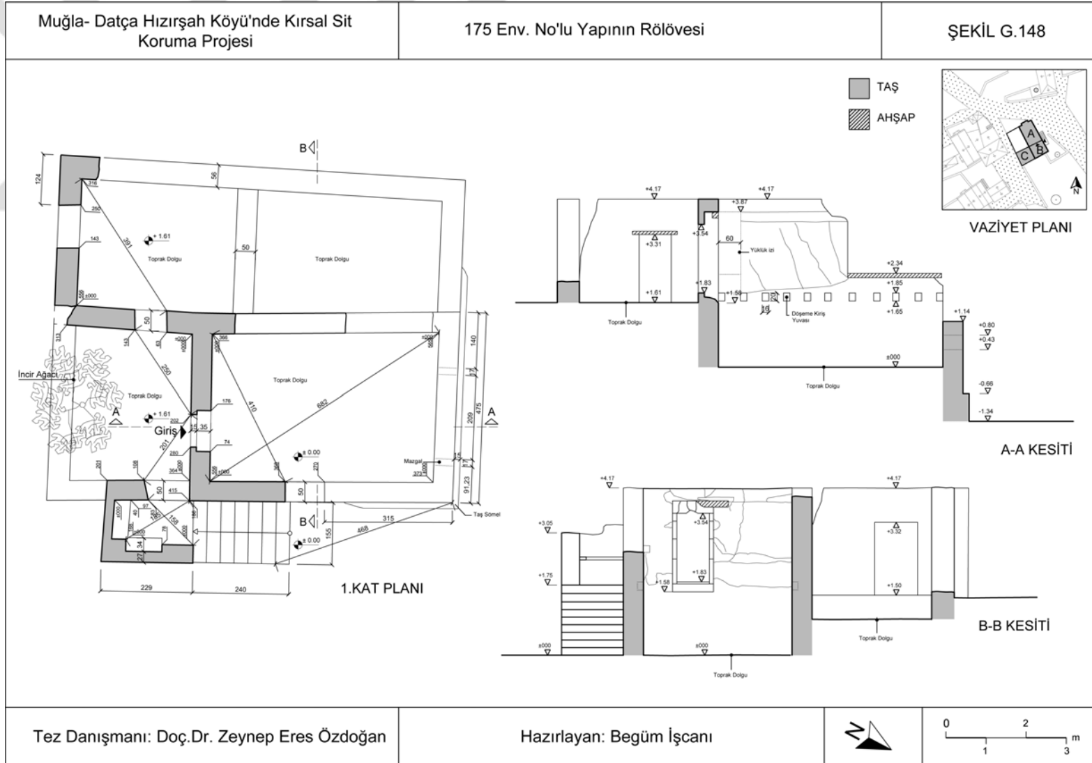
Şekil G.148 : 175 Env. No'lu Konutun Rölövesi.
