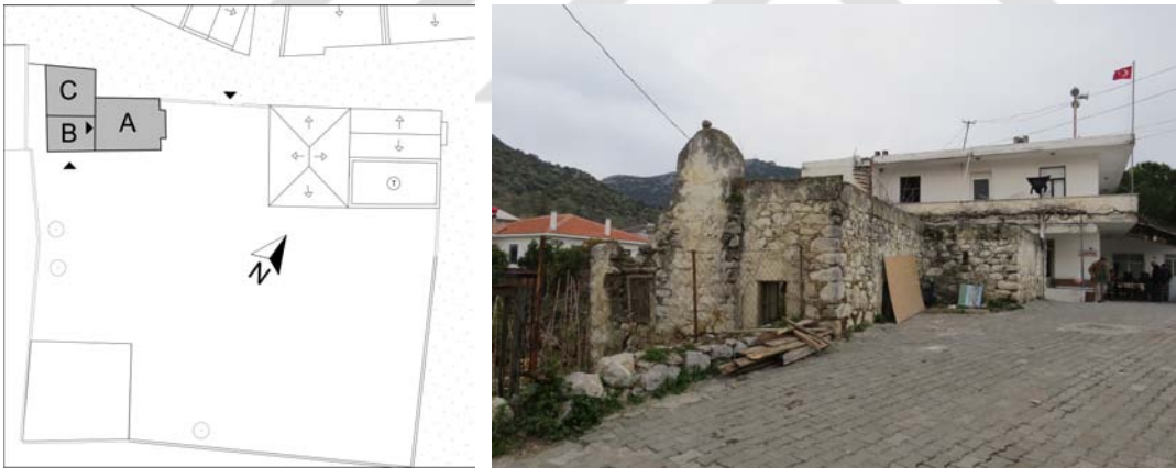
Şekil 5.9 : 101 Env. no'lu yapının vaziyet planı ve kuzeyden yapıya bakış.
