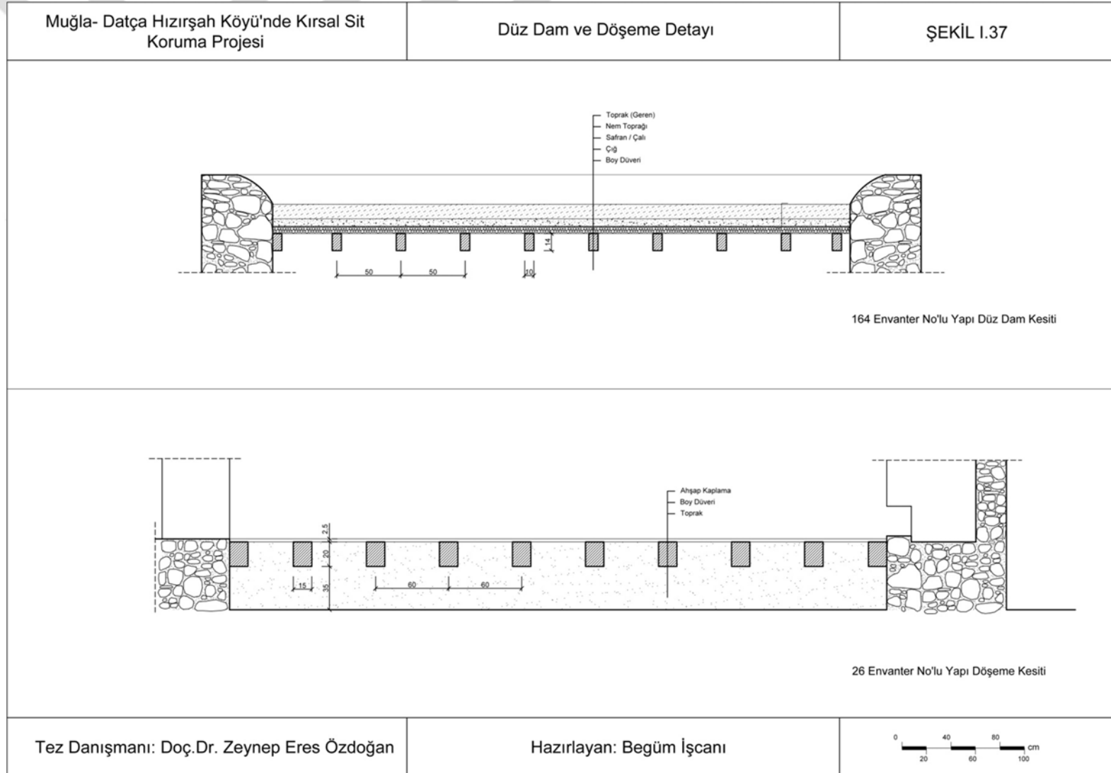
Şekil I.37 : Döşeme ve düz dam detayı.
