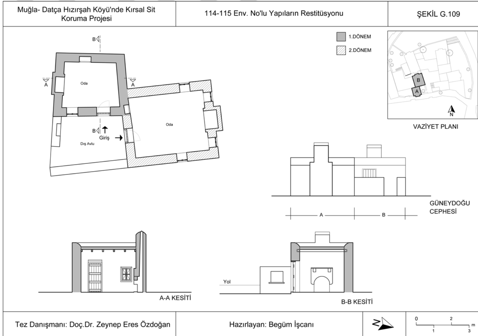
Şekil G.109 : 114 ve 115 Env. No'lu Konutların Restitüsyonu.
