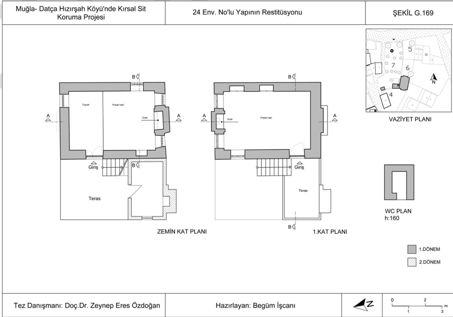
Şekil G.169 : 24 Env. No'lu Konutun Restitüsyonu.
