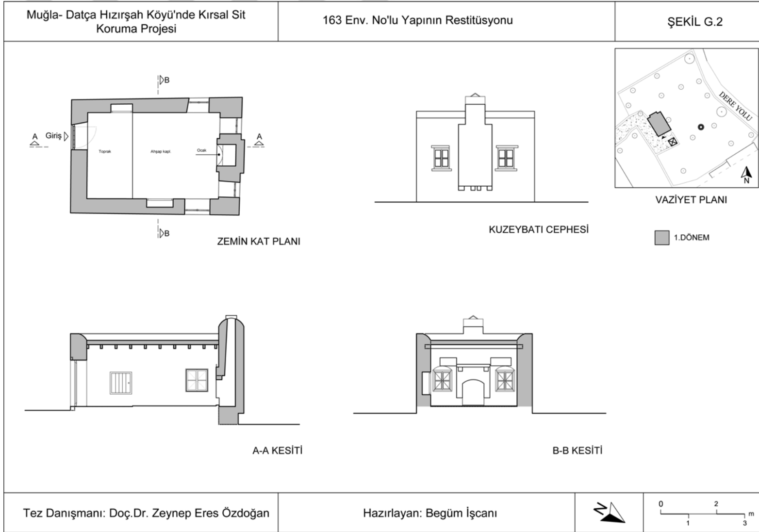
Şekil G.2 : 163 Env. No'lu Konutun Restitüsyonu.
