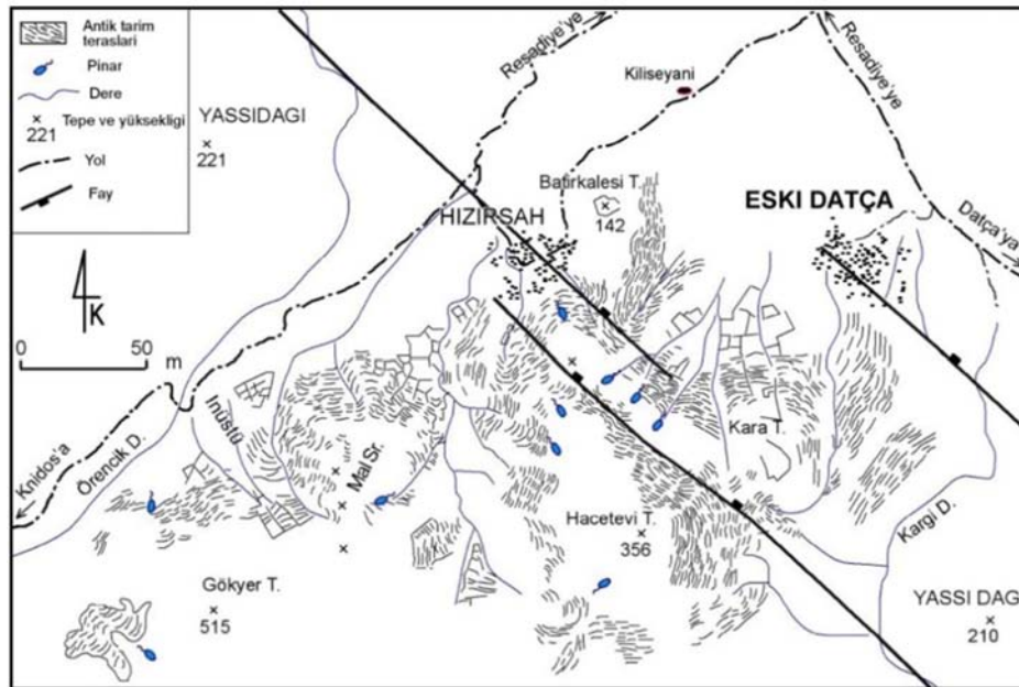
Şekil 3.4 : Hızırşah'ın güneyindeki antik tarım teraslarının planı (Dirik vd., 2003, Şekil 5.1).
