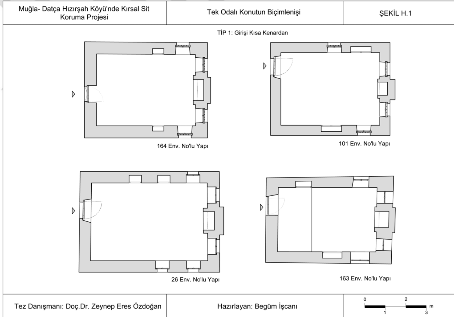
Şekil H.1 : Girişi kısa kenardan tek odalı konutun plan biçimlenişi.
