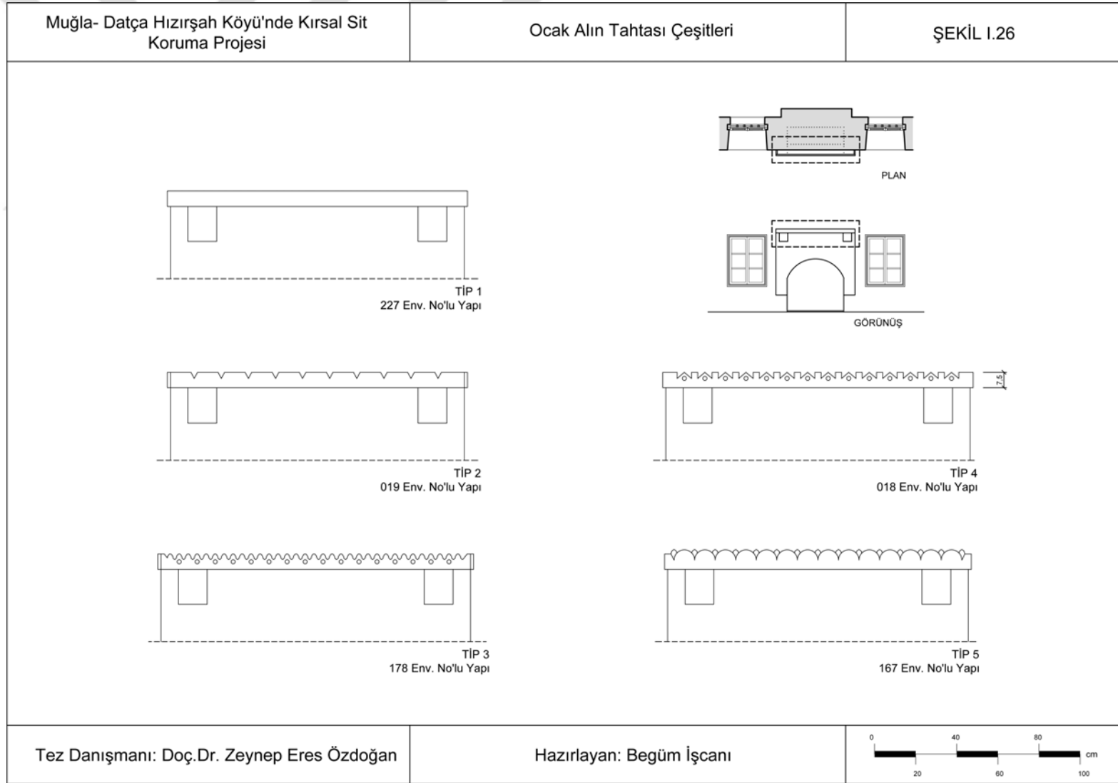
Şekil I.26 : Ocak alın tahtası çeşitleri.
