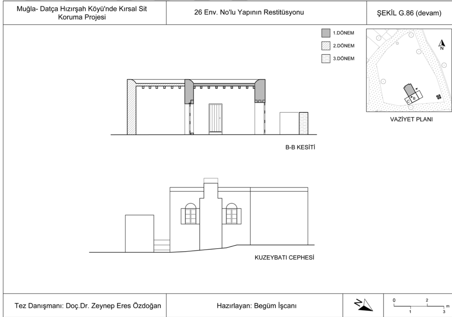
Şekil G.86 (devam) : 26 Env. No'lu Konutun Restitüsyonu.
