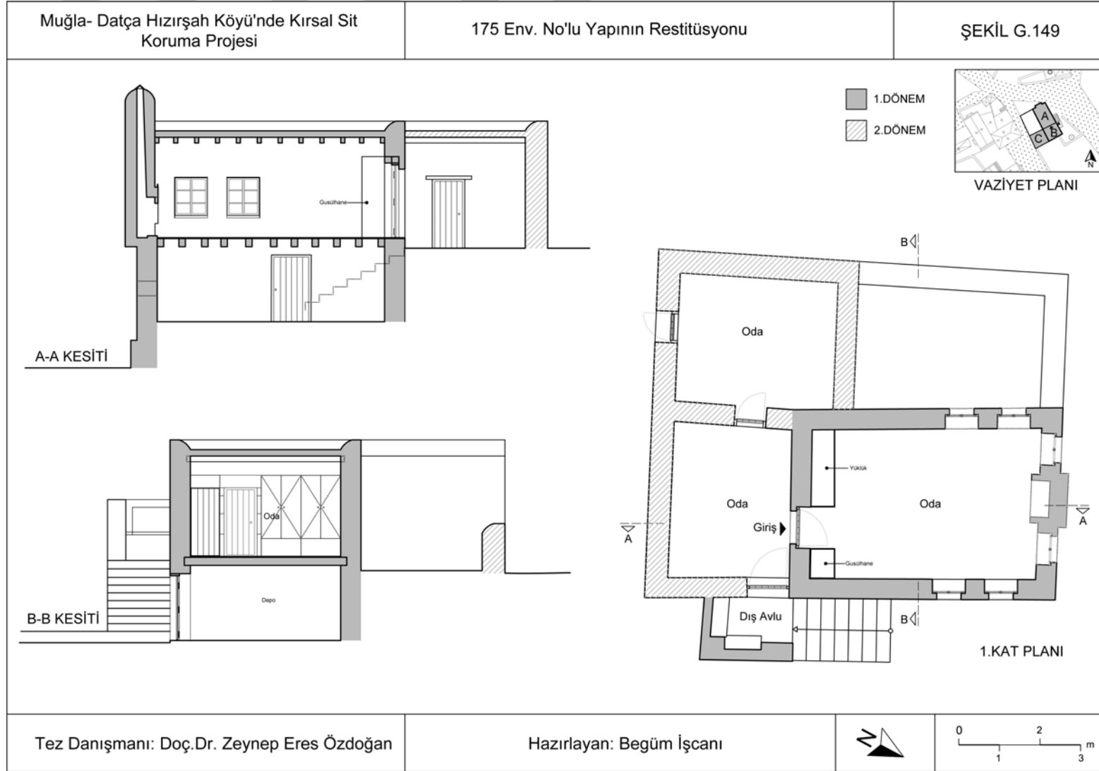
Şekil G.149 : 175 Env. No'lu Konutun Restitüsyonu.
