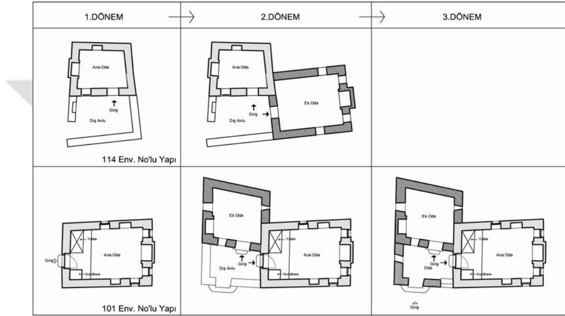
Şekil 5.16 : Tek odalı planın gelişimi.
