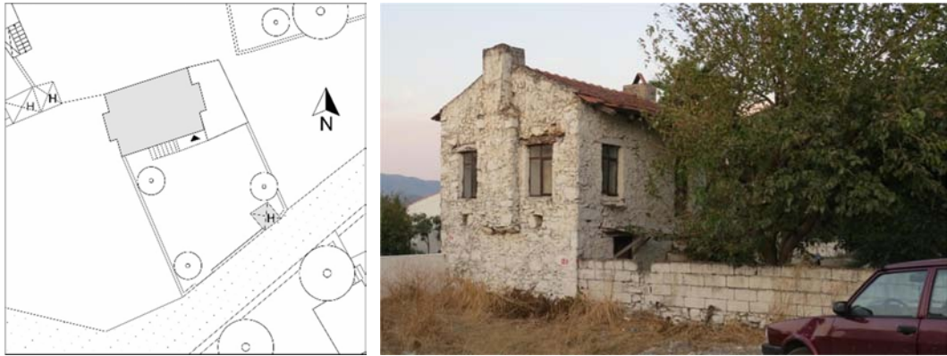
Şekil 5.15 : 164 Env. no'lu yapının vaziyet planı ve kuzeybatı cephesi.
