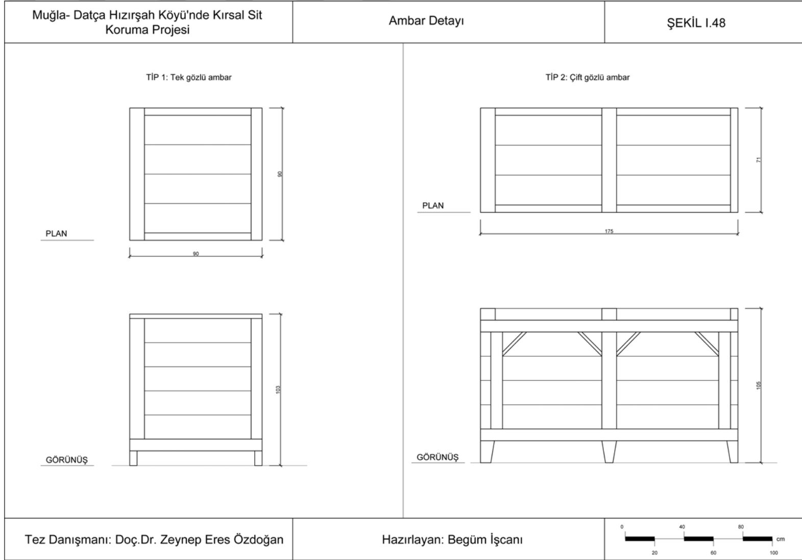
Şekil I.48 : Tek ve çift gözlü Ambar detayı.
