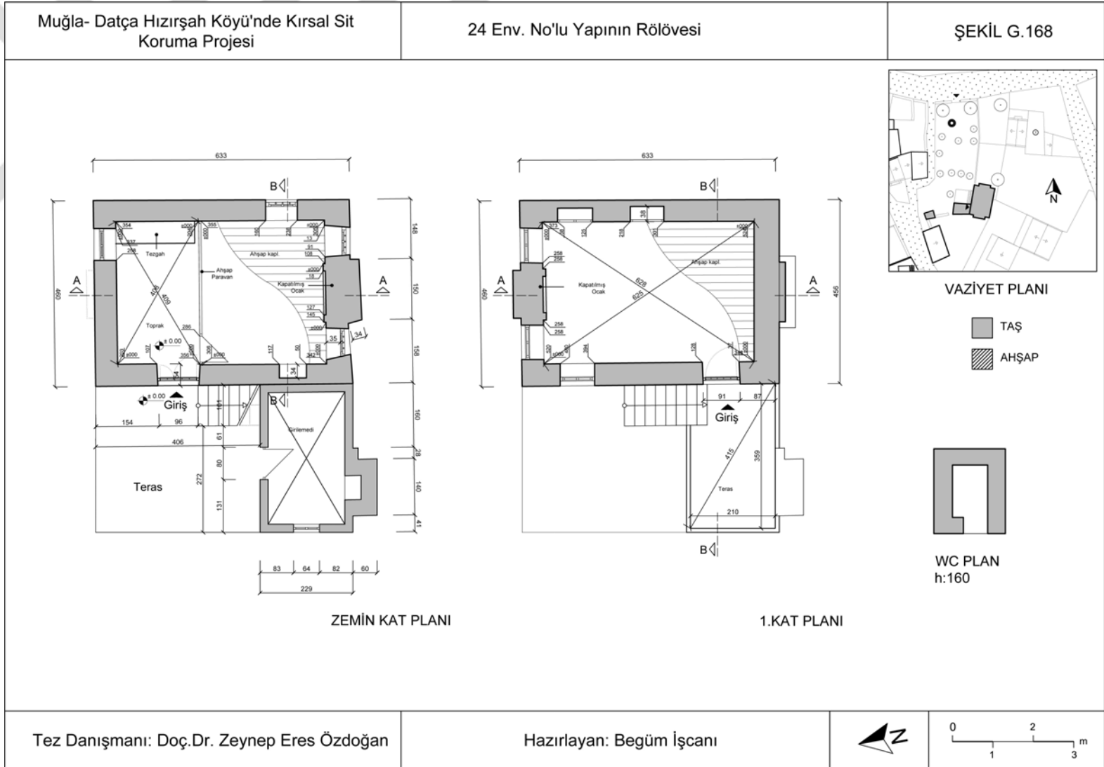
Şekil G.168 : 24 Env. No'lu Konutun Rölövesi.
