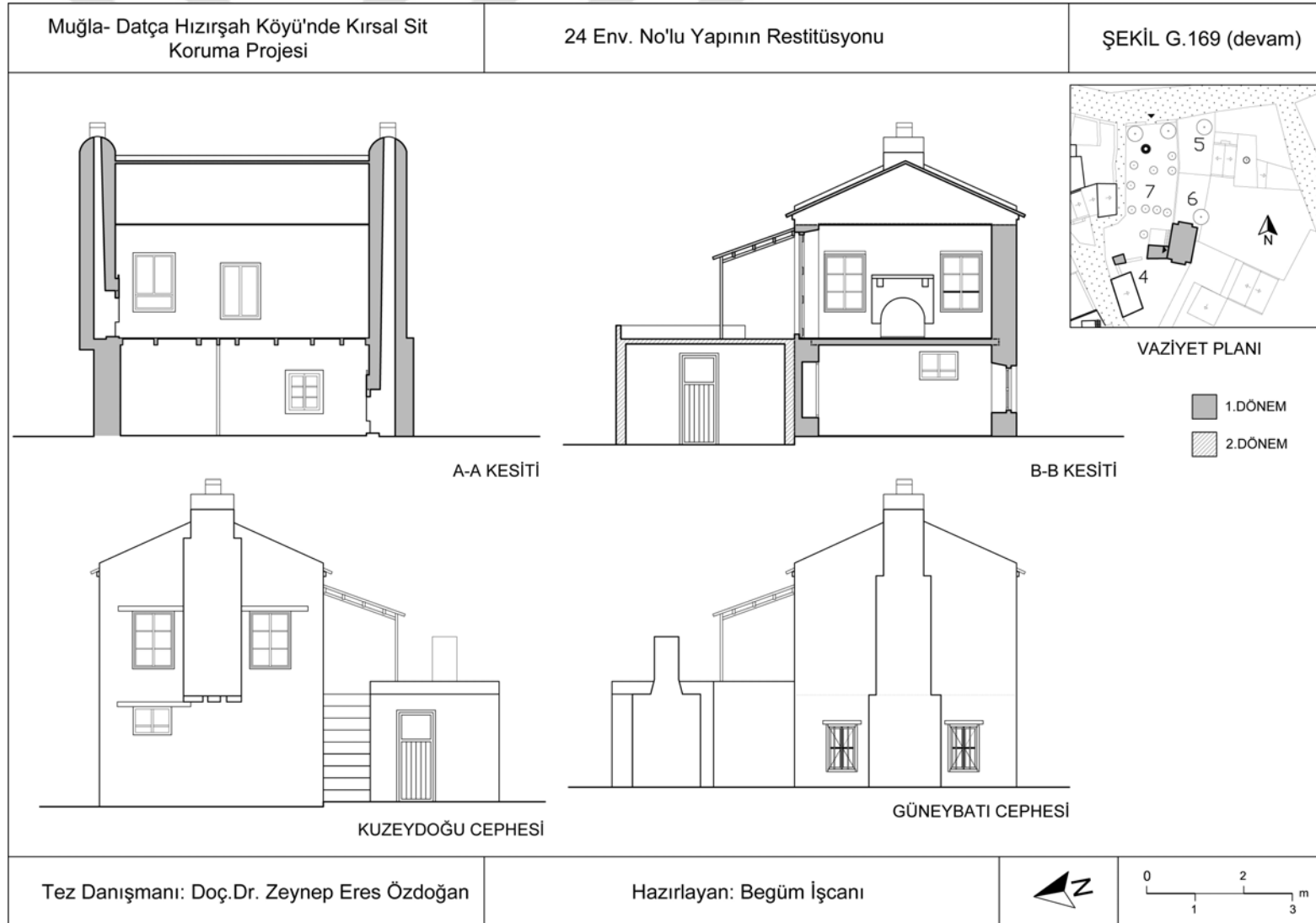
Şekil G.169 (devam) : 24 Env. No'lu Konutun Restitüsyonu.
