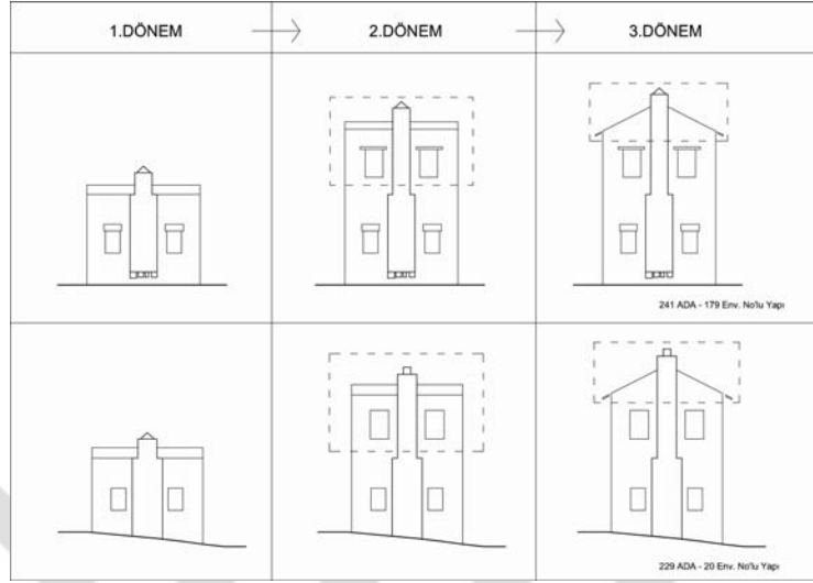
Şekil 5.19 : Tek katlı yapılara ikinci kat ve beşik çatı eklenmesi.
