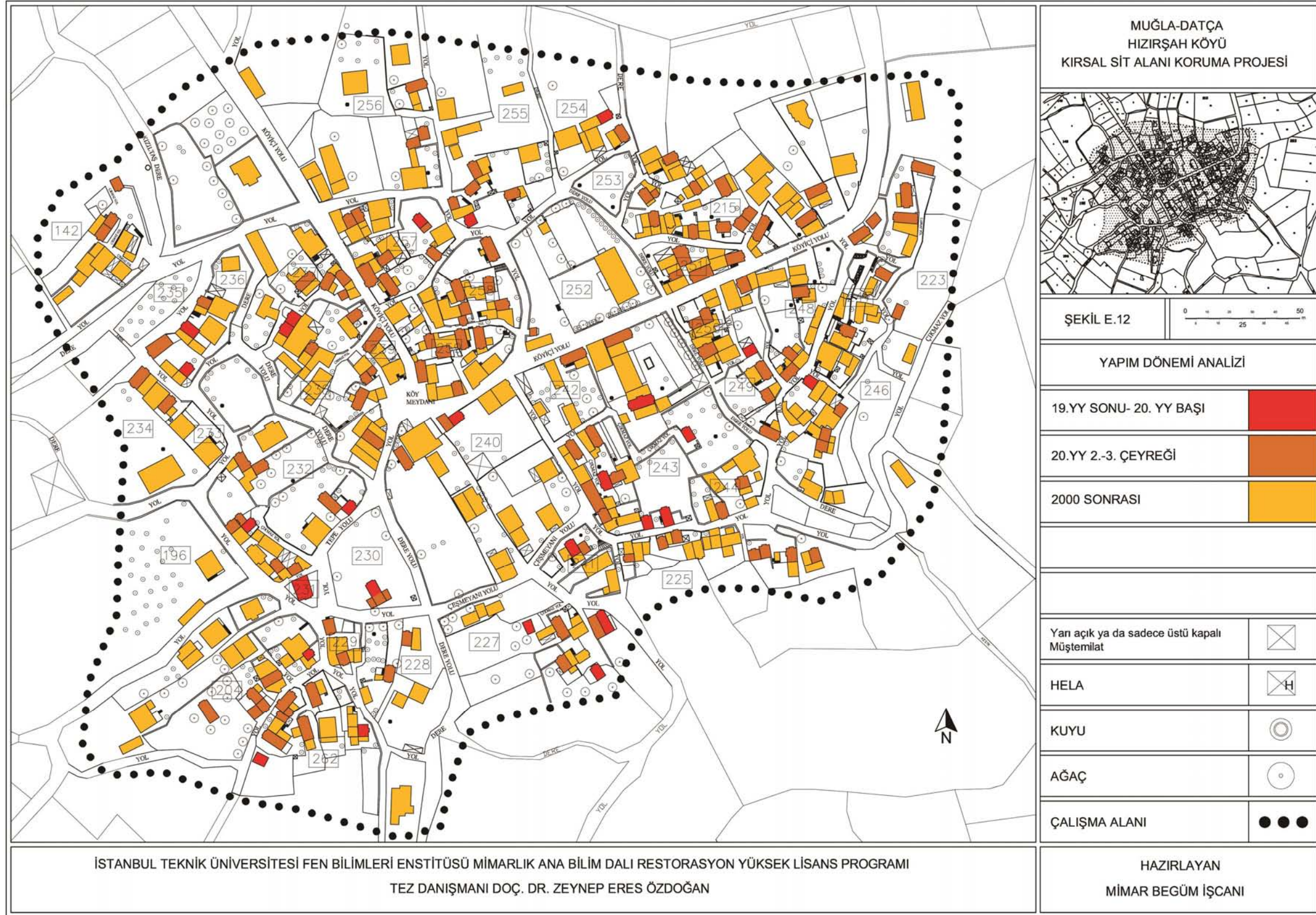
Şekil E.12 : Yapım Dönemi Analizi.
