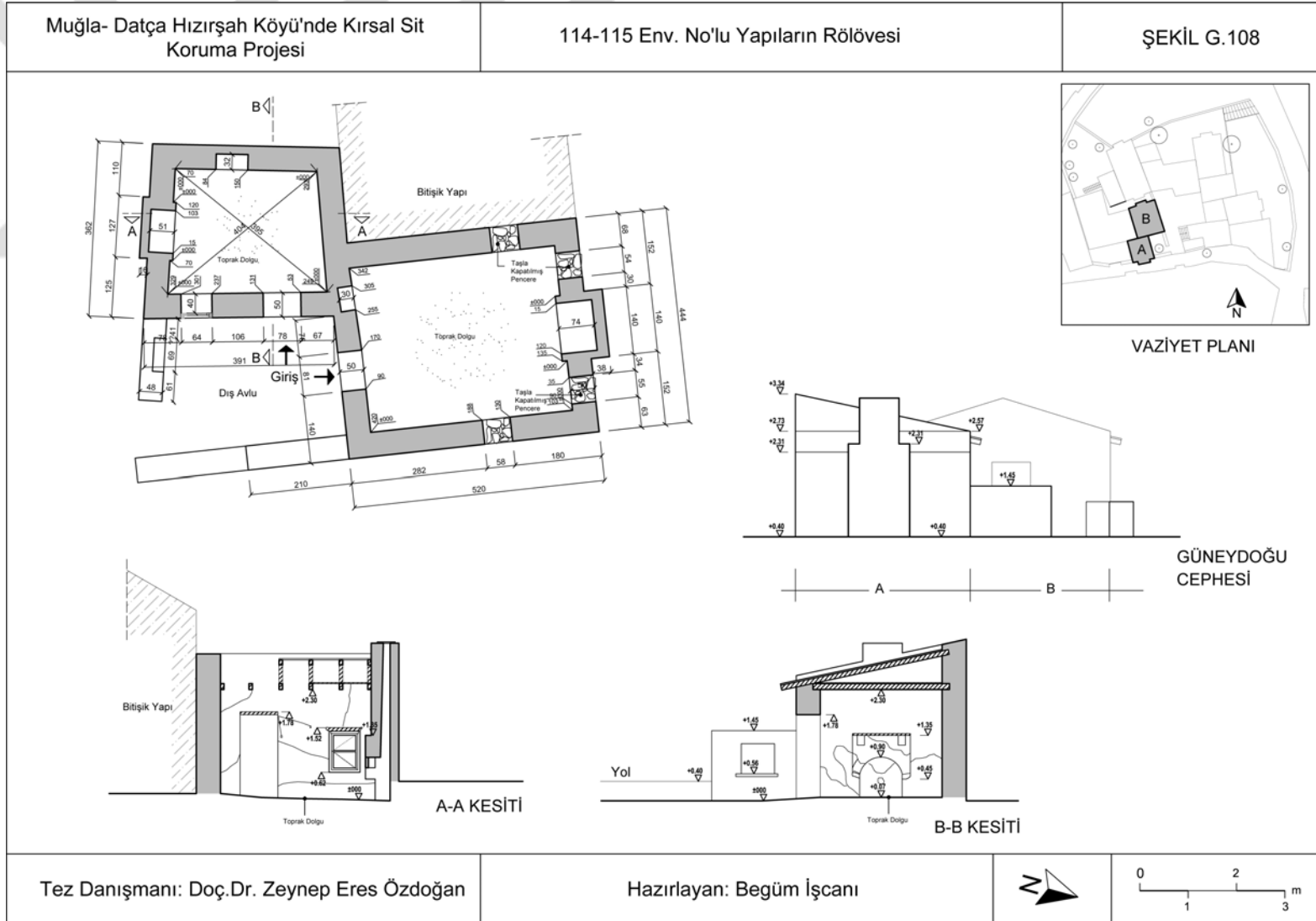
Şekil G.108 : 114 ve 115 Env. No'lu Konutların Rölövesi.
