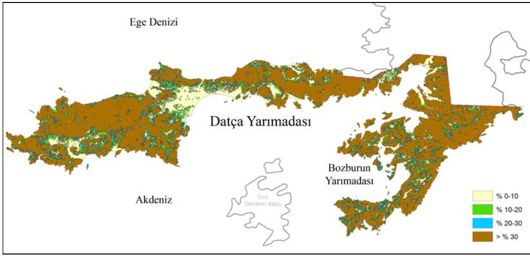
Şekil A.5 : Datça- Bozburun Yarımadası'nda arazilerin eğim durumu (Url-6, CDP Araştırma Raporu'ndan düzenlenmiştir, 2014, s.112).
