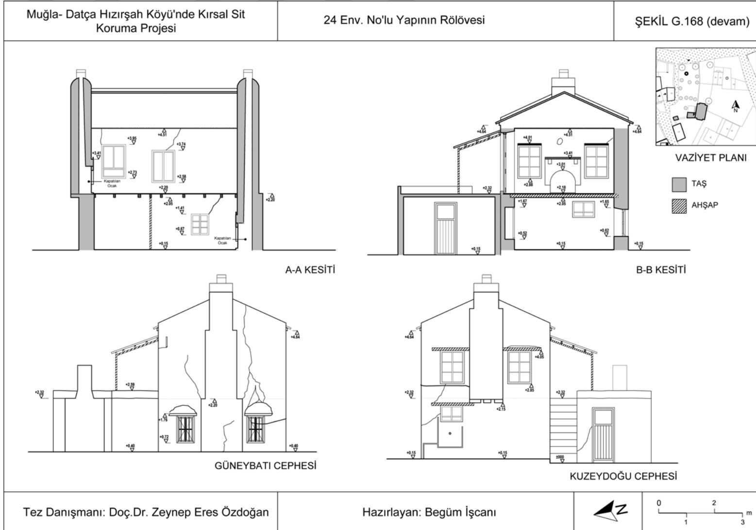
Şekil G.168 (devam) : 24 Env. No'lu Konutun Rölövesi.
