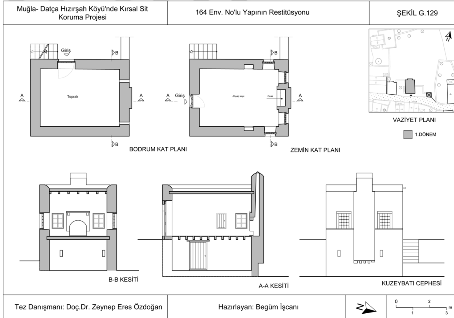
Şekil G.129 : 164 Env. No'lu Konutun Restitüsyonu.
