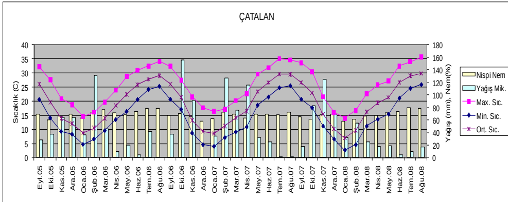
Şekil 3.3. Çatalan'a ait Eylül 2005-Ağustos 2008 iklim verileri.
