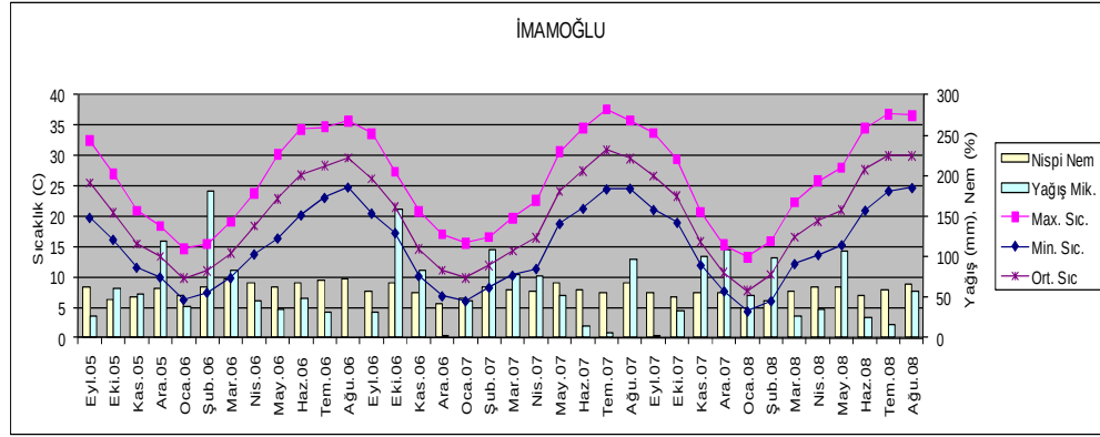
Şekil 3.4. İmamoğlu'na ait Eylül 2005-Ağustos 2008 iklim verileri
