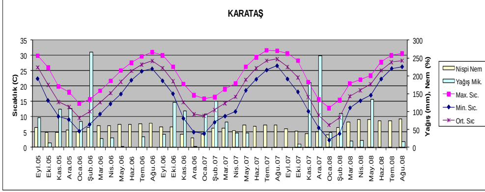
Şekil 3.2. Karataş'a ait Eylül 2005-Ağustos 2008 iklim verileri.
