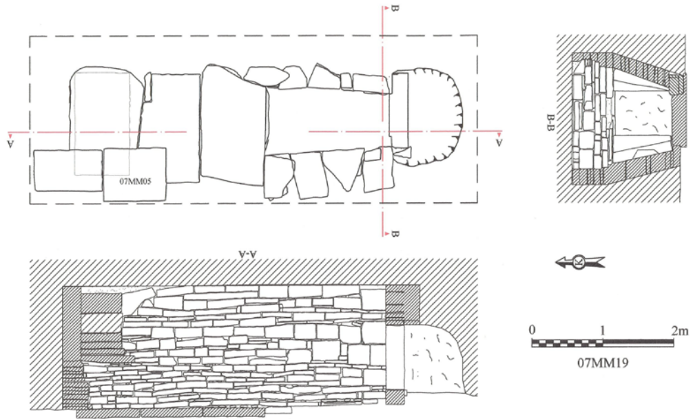
Çizim 6: 07MM19
