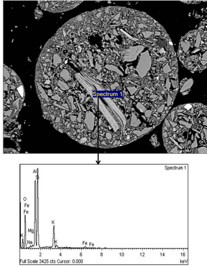
Şekil 5.36. Granüllerin yapısında yer alan lifli (tabakalı) kristallere ait temsili EDX analizi
