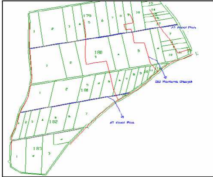
Şekil 3.4. Toplulaştırmalı sulama planlaması.
