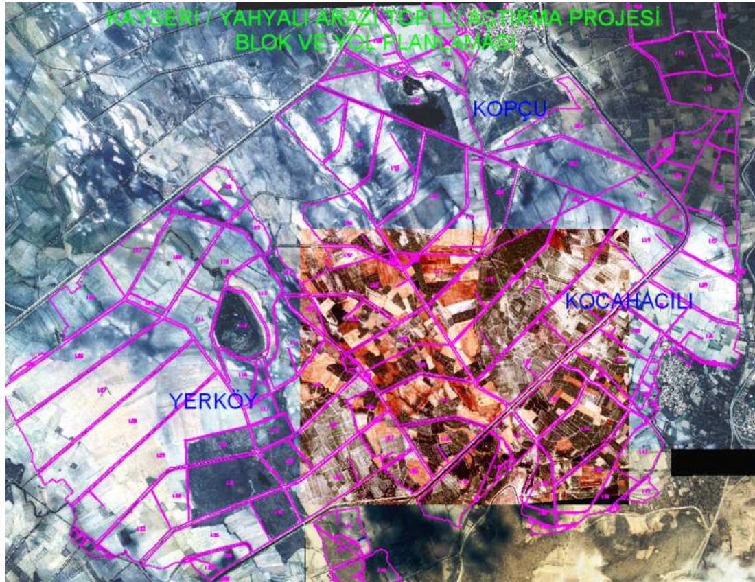
Şekil 5.21. Blok ve yol planlaması.
