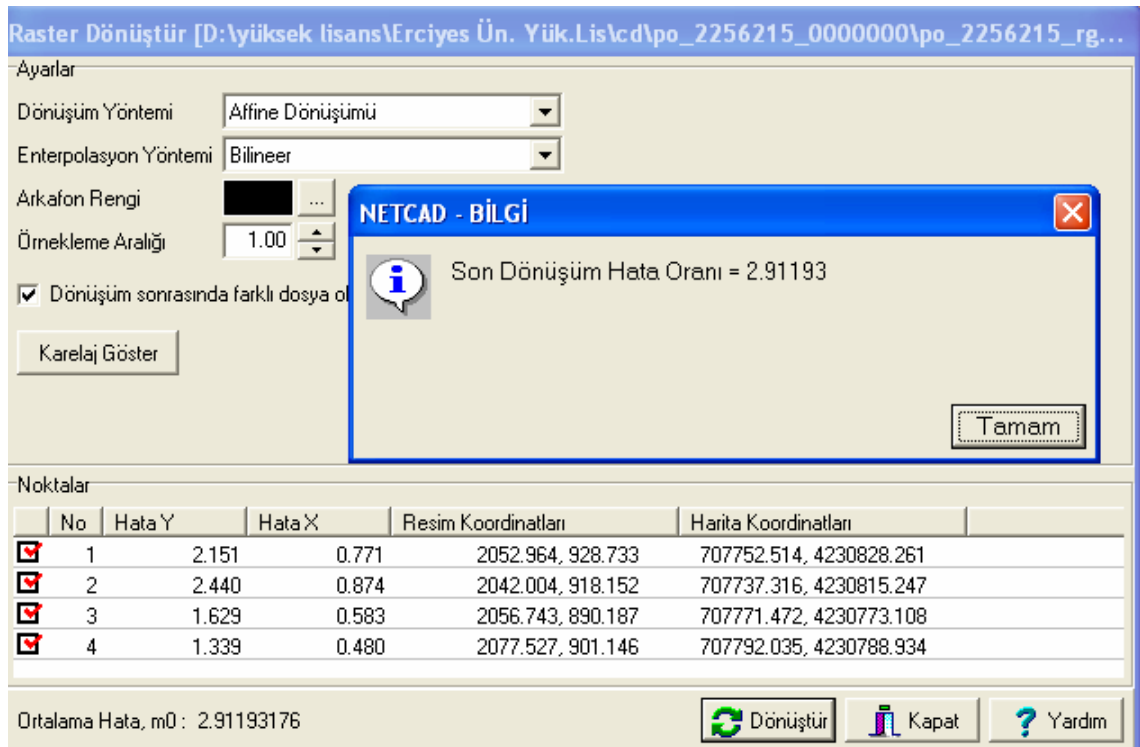
Şekil 5.7. Affine dönüşümü.
