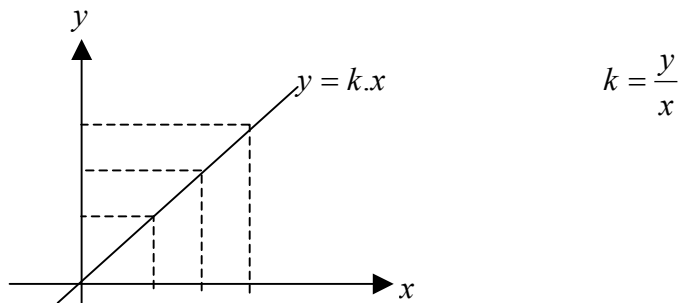
Şekil 1.4.2.1. Doğru Orantı Grafiği
