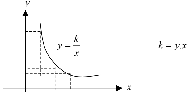
Şekil 1.4.2.2 Ters Orantı Grafiği
