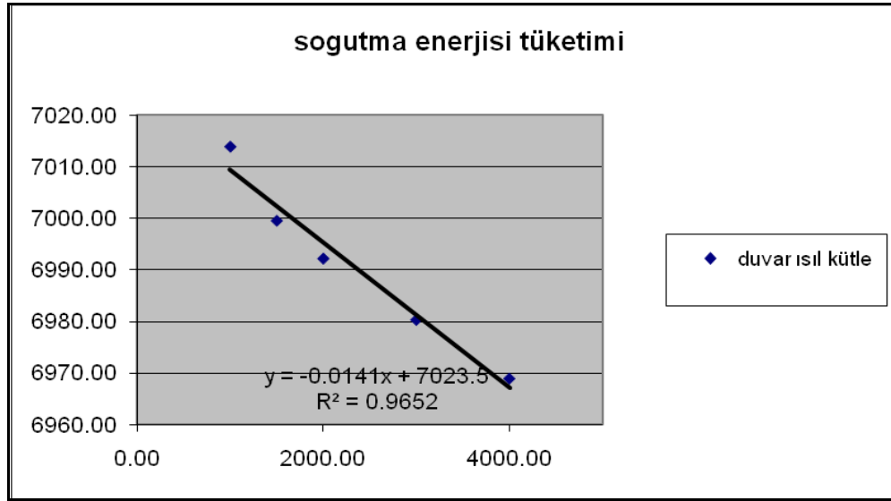
Şekil 3.20. Duvarda yer alan ısıt kütle ile soğutma enerjisi tüketimi arasındaki doğrusal ilişki.
