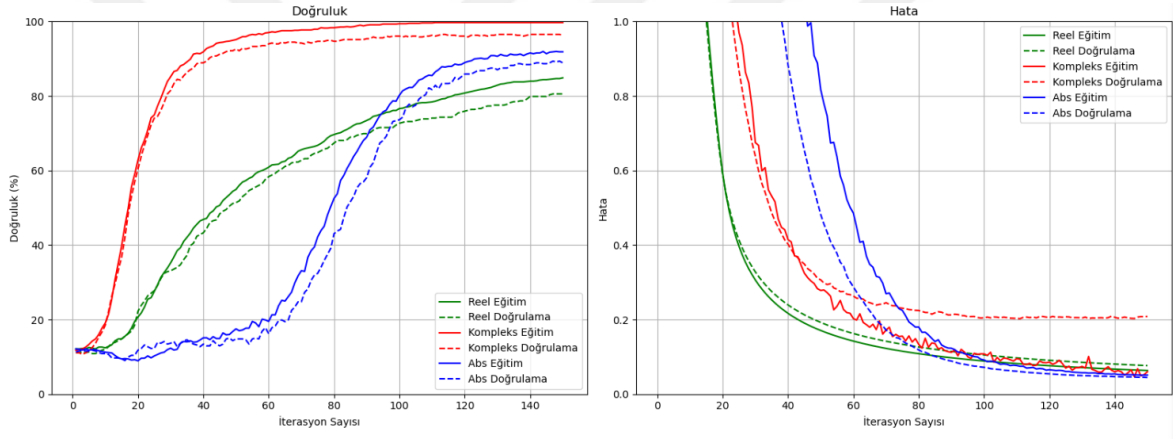
Şekil 6. 6: Digits veri setinin \frac{9}{8} alfa değeri için KarşıFANN yönteminin a) doğruluk ve b) hata grafikleri
