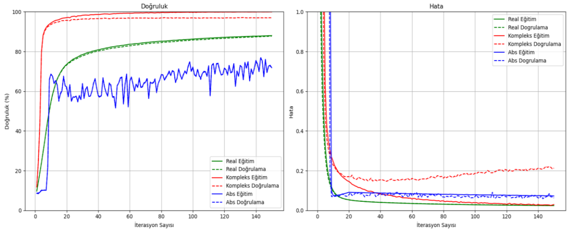
Şekil 6. 8: MNIST Rotation 45^\circ veri setinin 9/8 alfa değeri için KarcıFANN yönteminin a) Doğruluk ve b) Hata grafikleri
