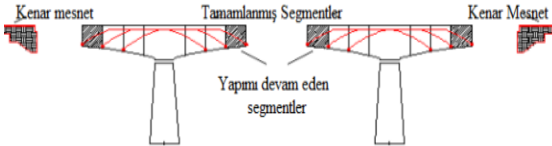
Şekil 1.15. Köprü üstyapısını oluşturan dilimlerin inşasına ait şematik gösterim
