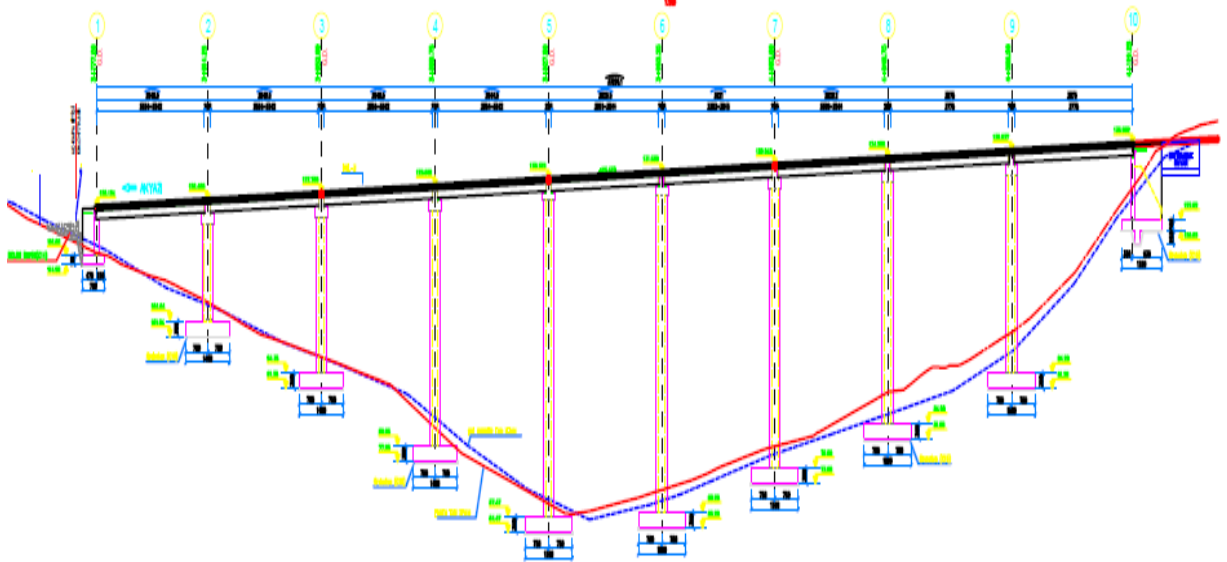
Şekil 2.20. Karşıyaka viyadüğü anayol kesit planı
