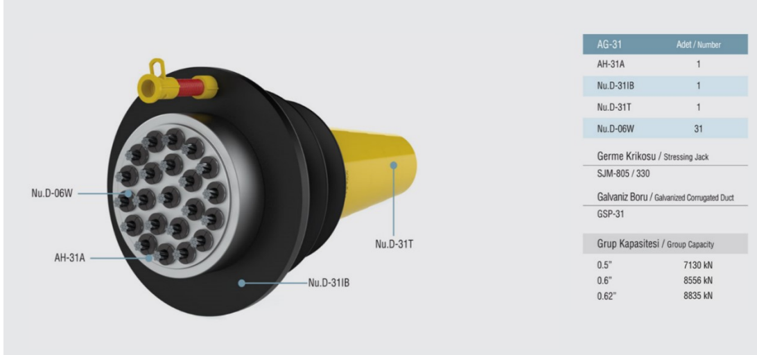
Şekil 1.30. 31'li halat düzenine sahip halat plakası
