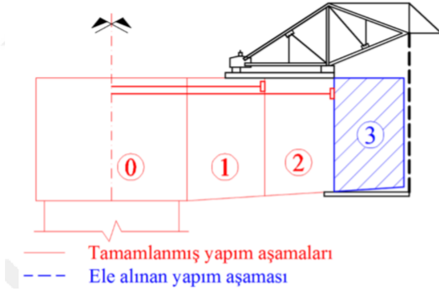
Şekil 1.22. Dilimsel dengeli konsol üstyapısının şematik olarak yapım aşamaları-2
