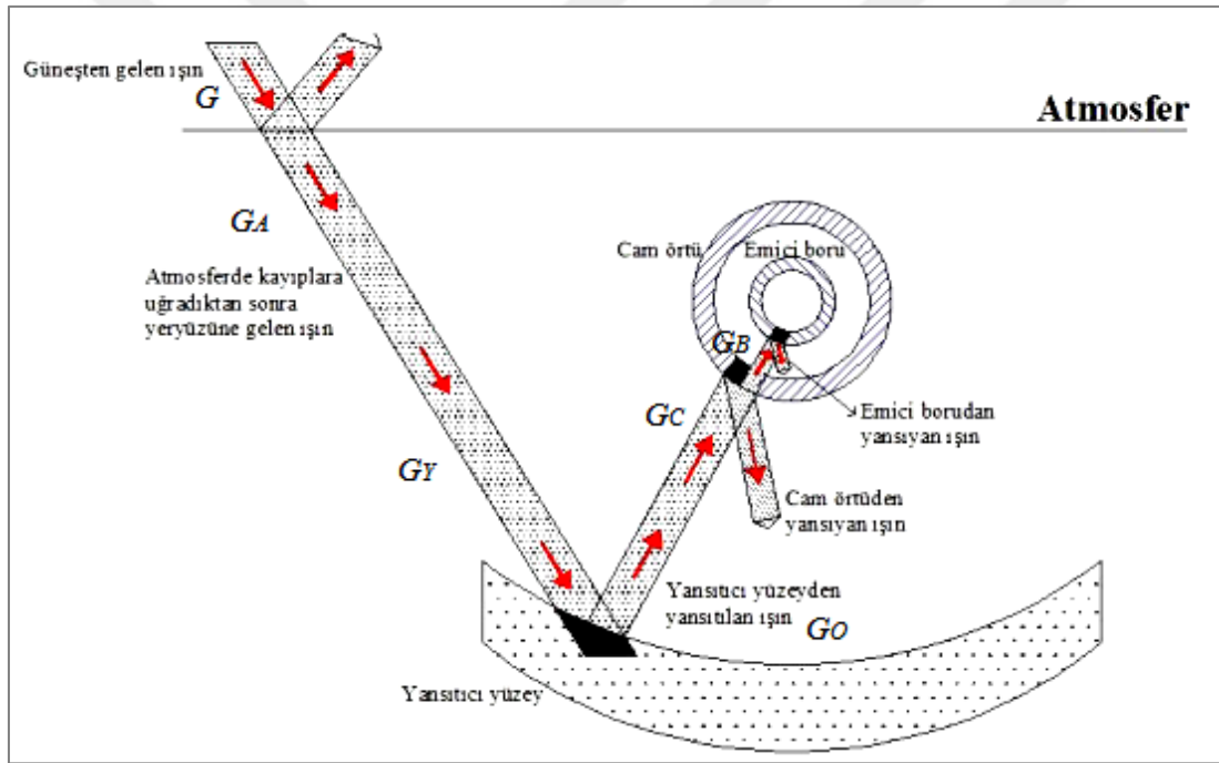
Şekil 5.3. Parabolik oluk tipi güneş kolektöründe güneş ışınlarının transferi (Cicibıyık, 2012)
