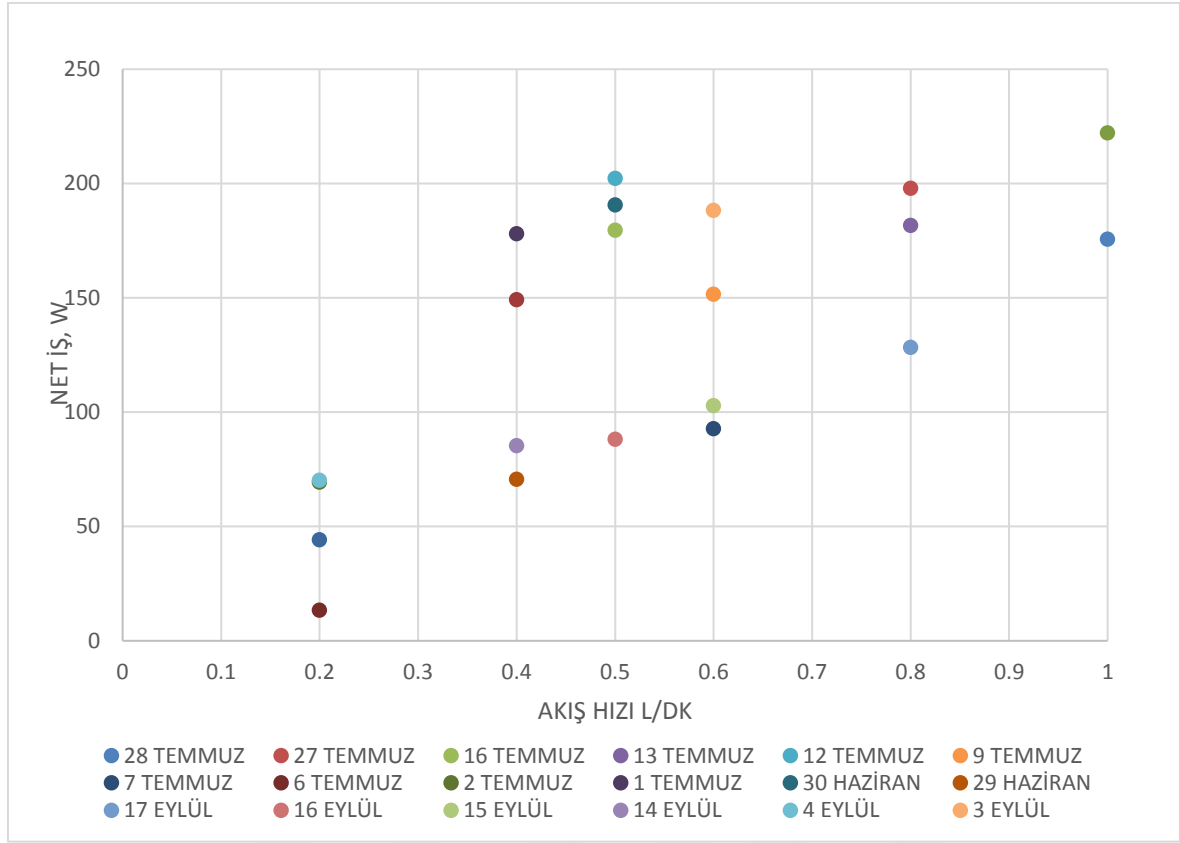
Şekil 6.17. İzobütan için farklı akış hızlarında net iş miktarı
