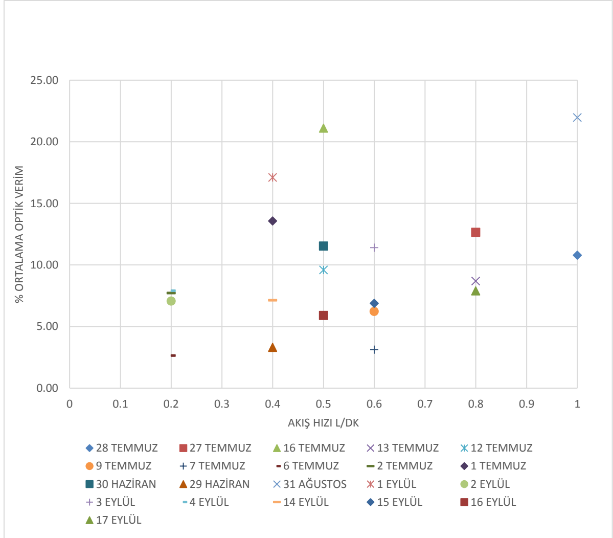
Şekil 6.14. Akış hızına bağlı ortalama optik verim değişimi
