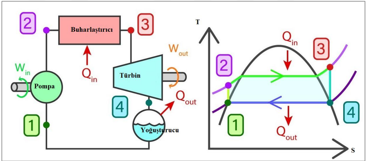
Şekil 4.9. Genel Rankine çevrimi (URL-17)
