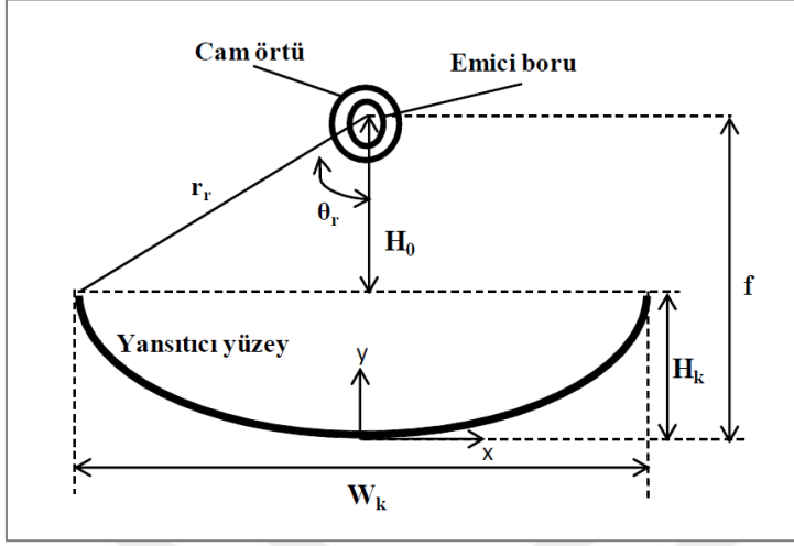
Şekil 4.5. Parabolik oluk tipi güneş kolektörü tasarım parametreleri (Cicibıyık, 2012)
