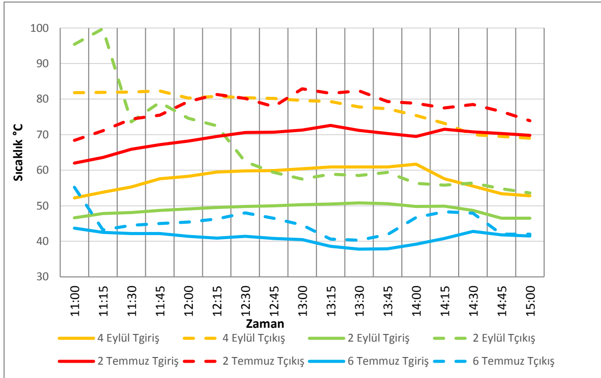
Şekil 6.5. 0,2 L/dk akış hızında gliserin emici boru giriş ve çıkış sıcaklıkları
