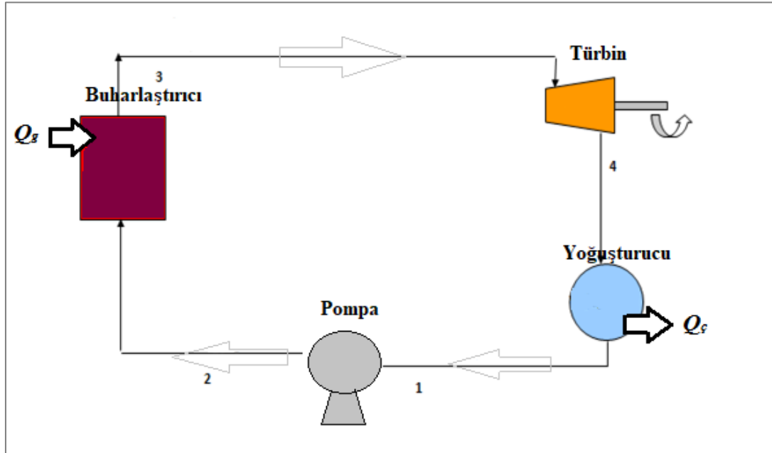
Şekil 5.8. Organik Rankine çevrimi gösterimi
