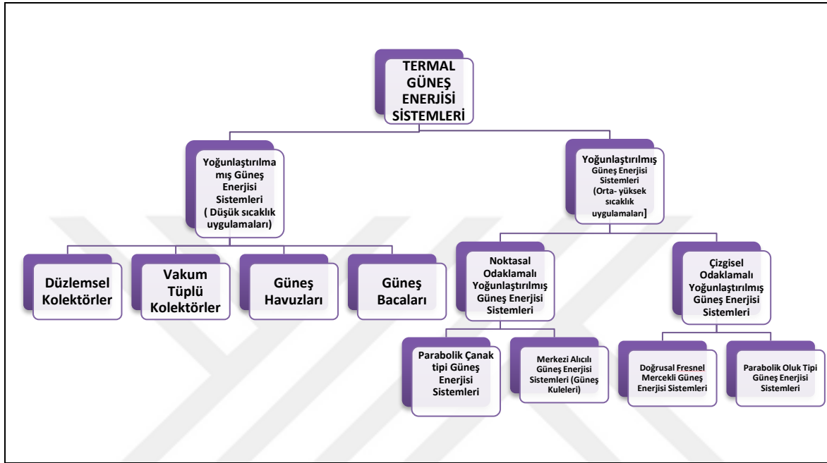
Şekil 3.2. Termal güneş enerjisi sistemleri
