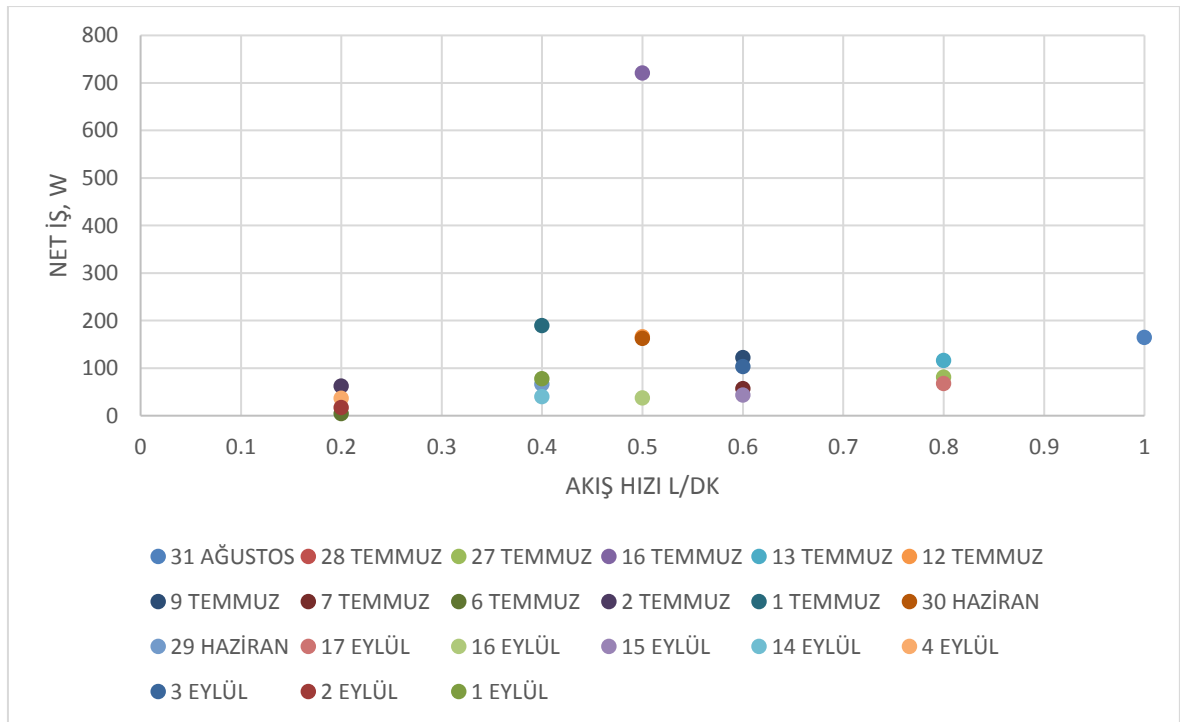
Şekil 6.18. Pentan için farklı akış hızlarında net iş miktarı
