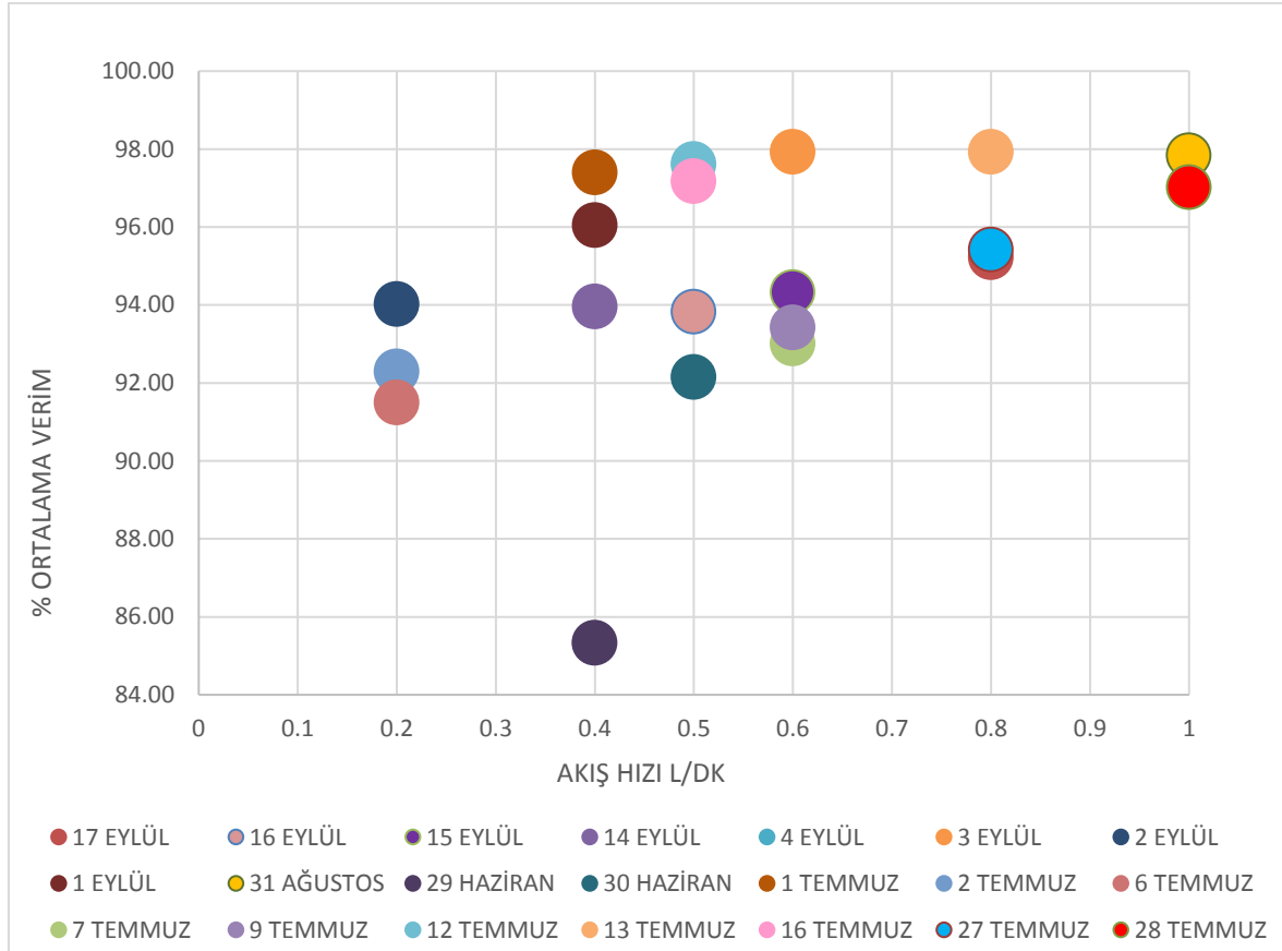
Şekil 6.13. Akış hızına göre ortalama termal verim değerleri
