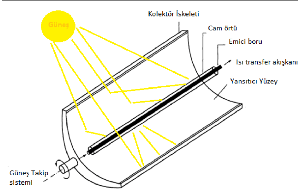
Şekil 4.1. Parabolik oluk tipi güneş enerjisi sistemi
