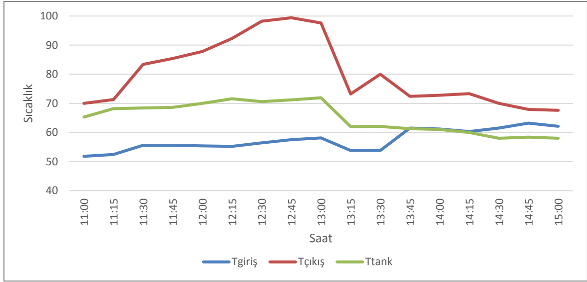
Şekil 6.3. 1 Eylül 2020 tarihli 0,4 L/dk akış hızlı deneysel çalışma sıcaklık değişim grafiği
