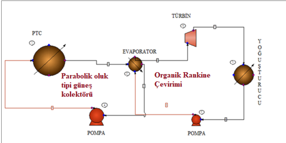
Şekil 6.2. Parabolik oluk tipi güneş enerjisi sistemi ile kombine edilmiş organik Rankine çeviriminin şematik gösterimi
