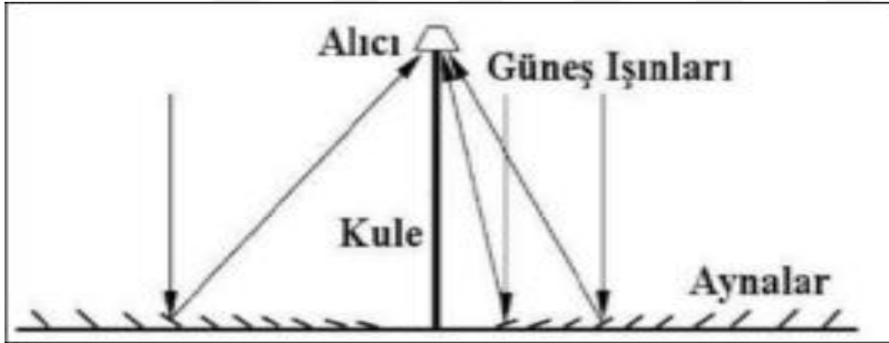
Şekil 3.10. Doğrusal Fresnel kolektör çalışma prensibi (Üçgül ve Ergün, 2012)
