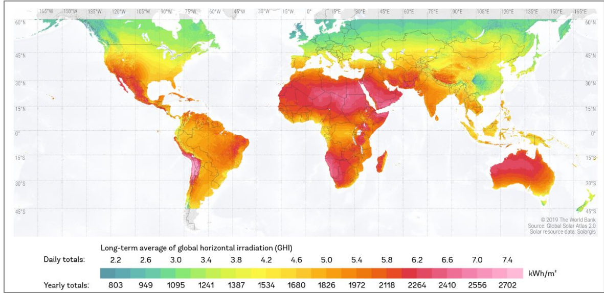
Şekil 2.3. Dünyanın toplam ışınlama haritası (URL-5)
