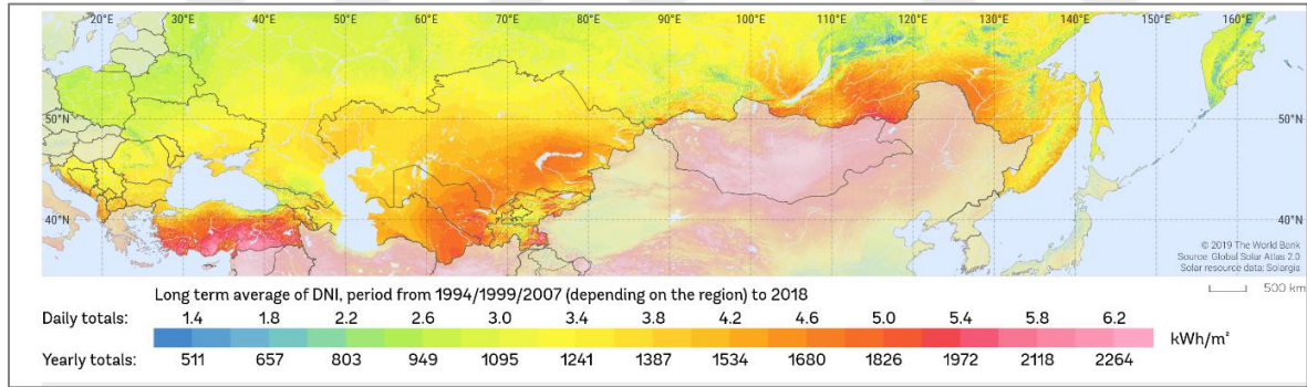
Şekil 2.4. Avrupa ve orta Asya direk ışınlama haritası (URL-5)
