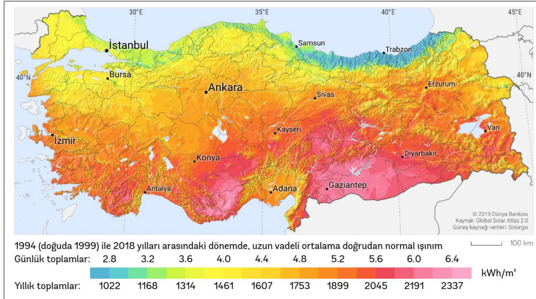
Şekil 2.5. Türkiye’de direkt ışıınım haritası (URL-5)
