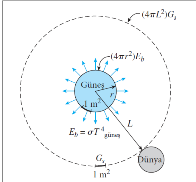
Şekil 2.1. Güneş ile dünya arasında gerçekleşen ışıınım (Çengel, 2015)
