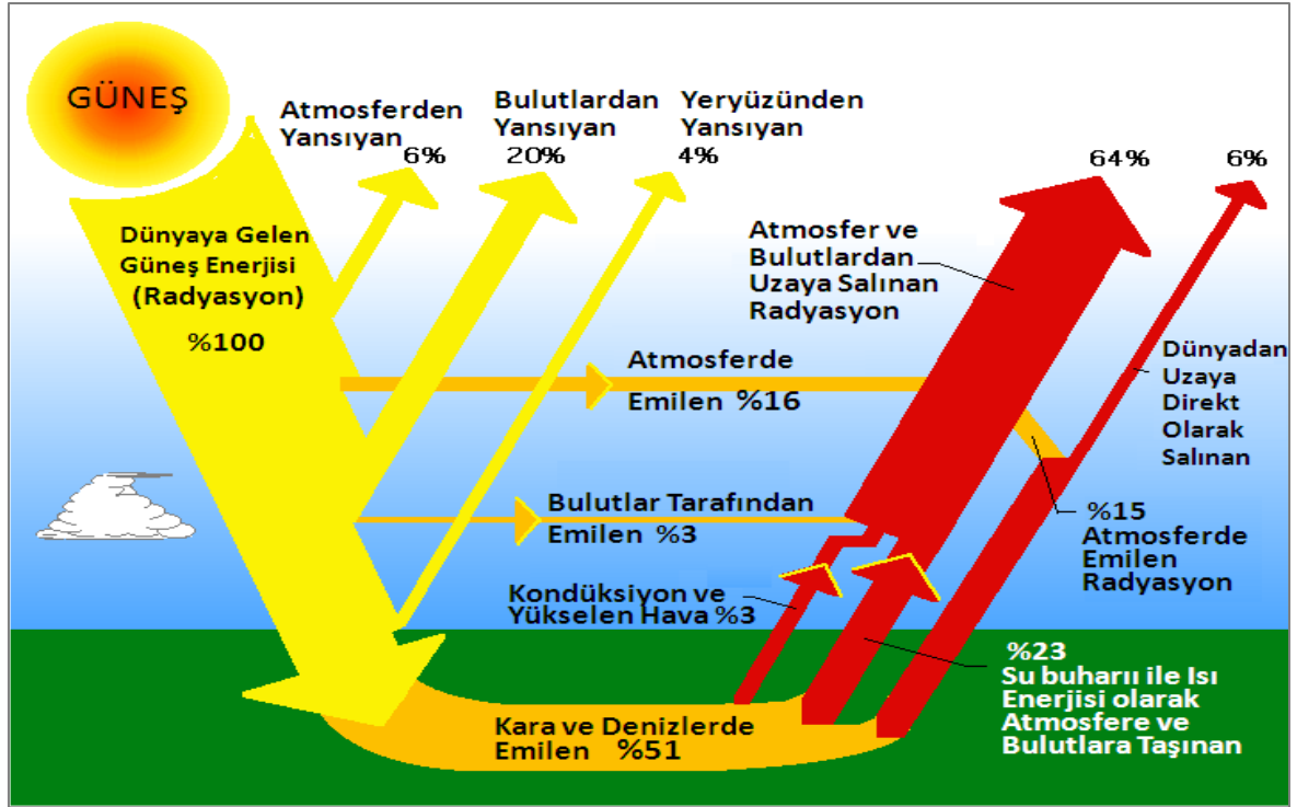
Şekil 5.2. Güneş ışınlarının yeryüzüne gelene kadar uğradığı kayıplar
