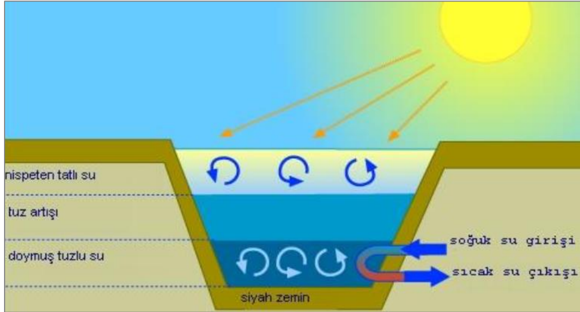
Şekil 3.5. Güneş havuzu (URL-11)
