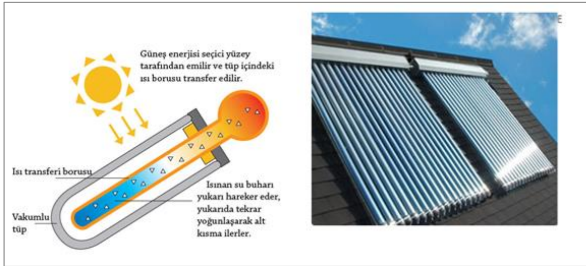
Şekil 3.4. Vakum tüplü güneş kolektörü ve vakumlu cam tüp (URL-10)
