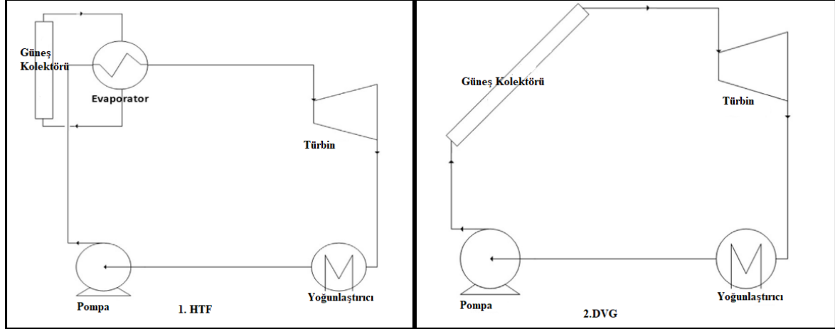
Şekil 4.8. 1. Isı transfer akışkanı konfigürasyonu, 2. Direkt buhar üretim konfigürasyonu gösterimi (Aboelwafa ve diğ., 2018)
