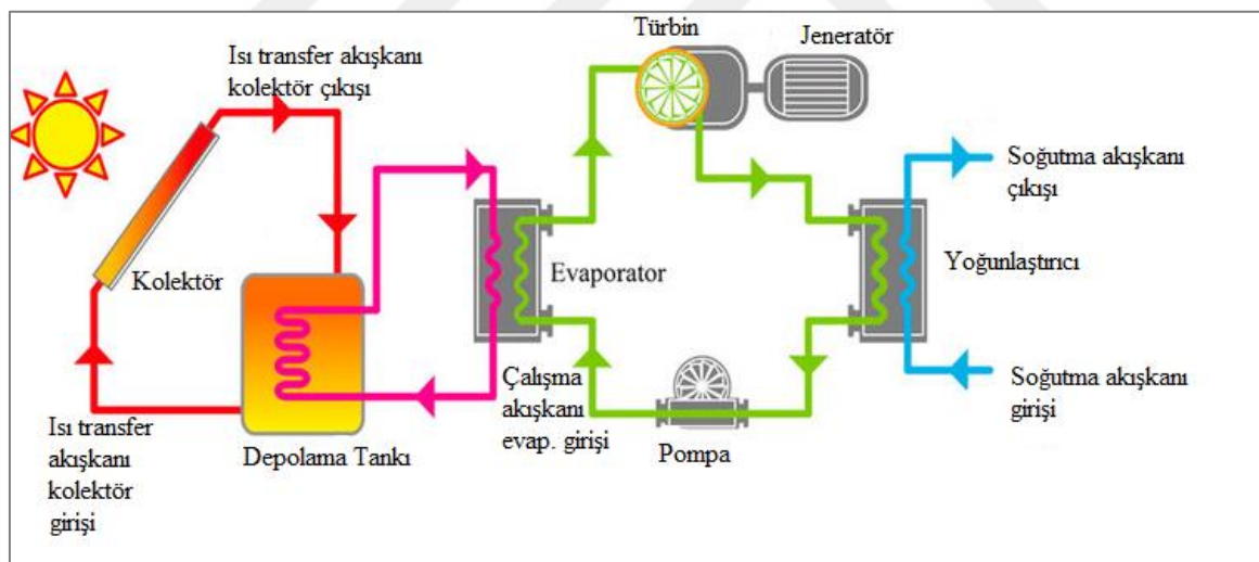
Şekil 4.3. Güneş enerjisinden güç üretimi şeması (URL-14)
