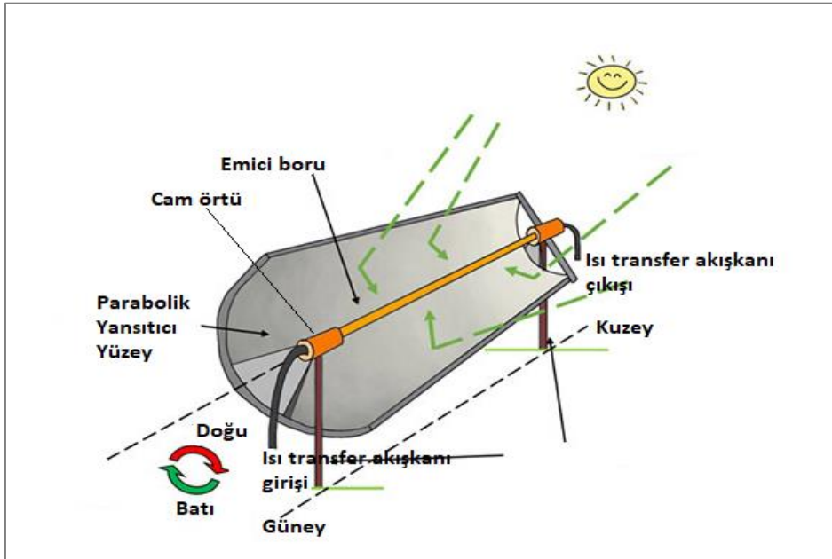
Şekil 3.12. Parabolik oluk tipi güneş enerjisi sistemi
