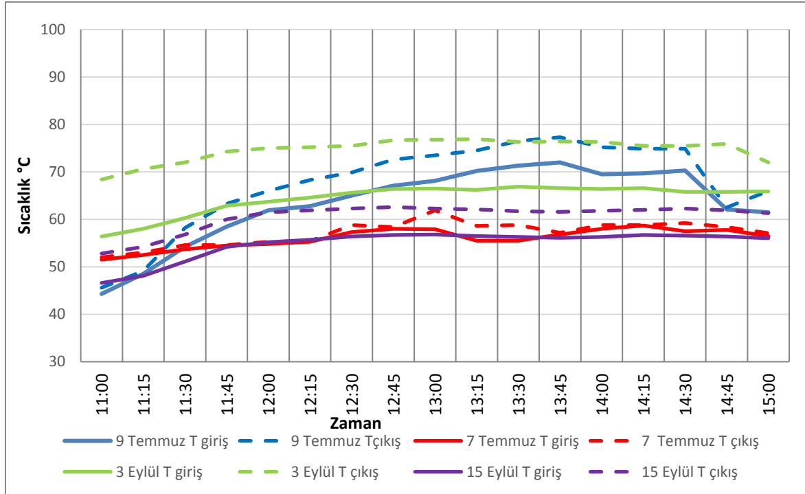
Şekil 6.8. 0,6 L/dk akış hızında gliserin emici boru giriş ve çıkış sıcaklıkları
