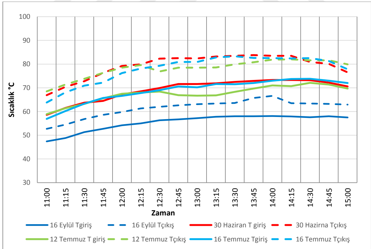
Şekil 6.7. 0,5 L/dk akış hızında gliserin emici boru giriş ve çıkış sıcaklıkları
