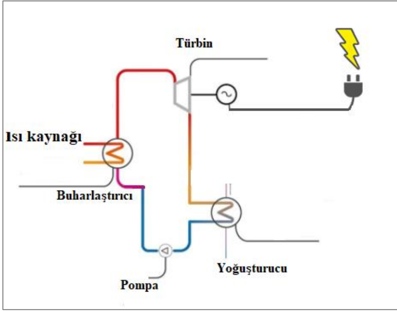
Şekil 4.10. Organik Rankine çevrimi genel gösterimi (URL-18)
