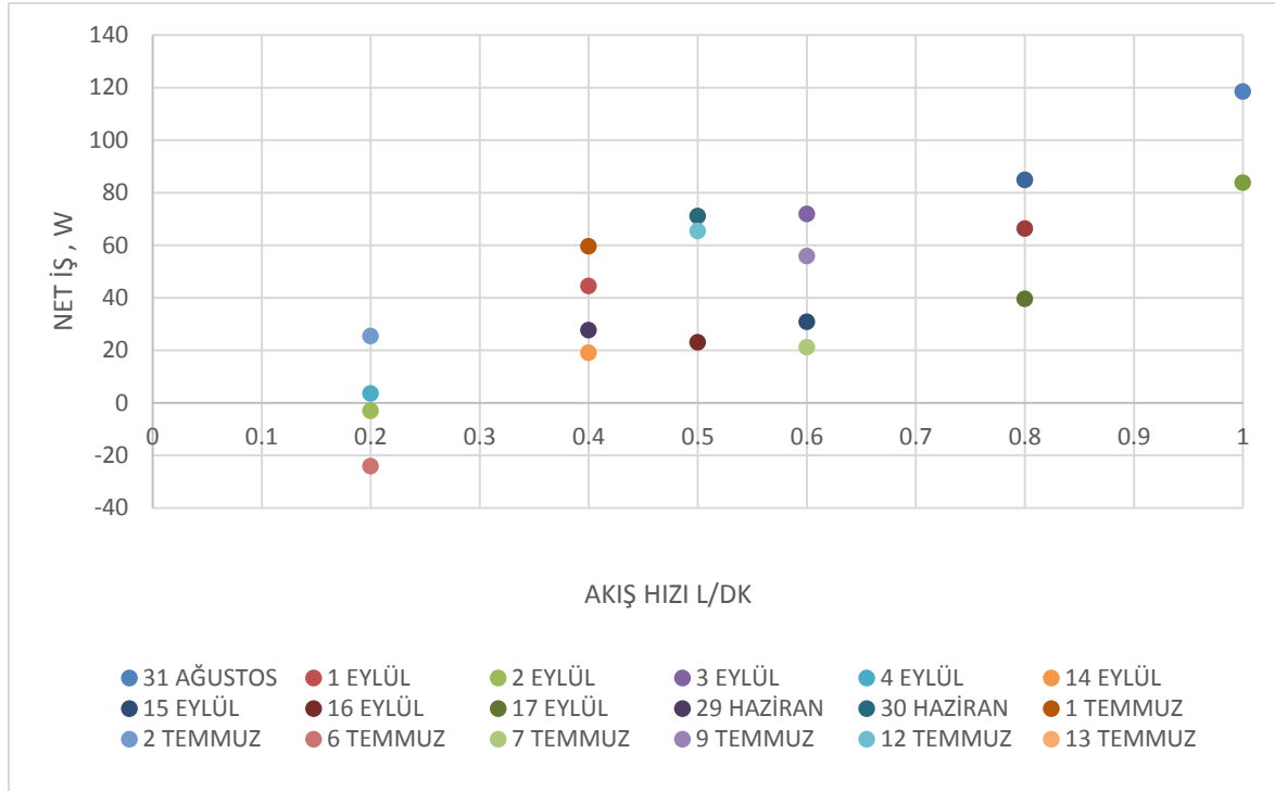
Şekil 6.15. R134a için farklı akış hızlarında net iş miktarı
