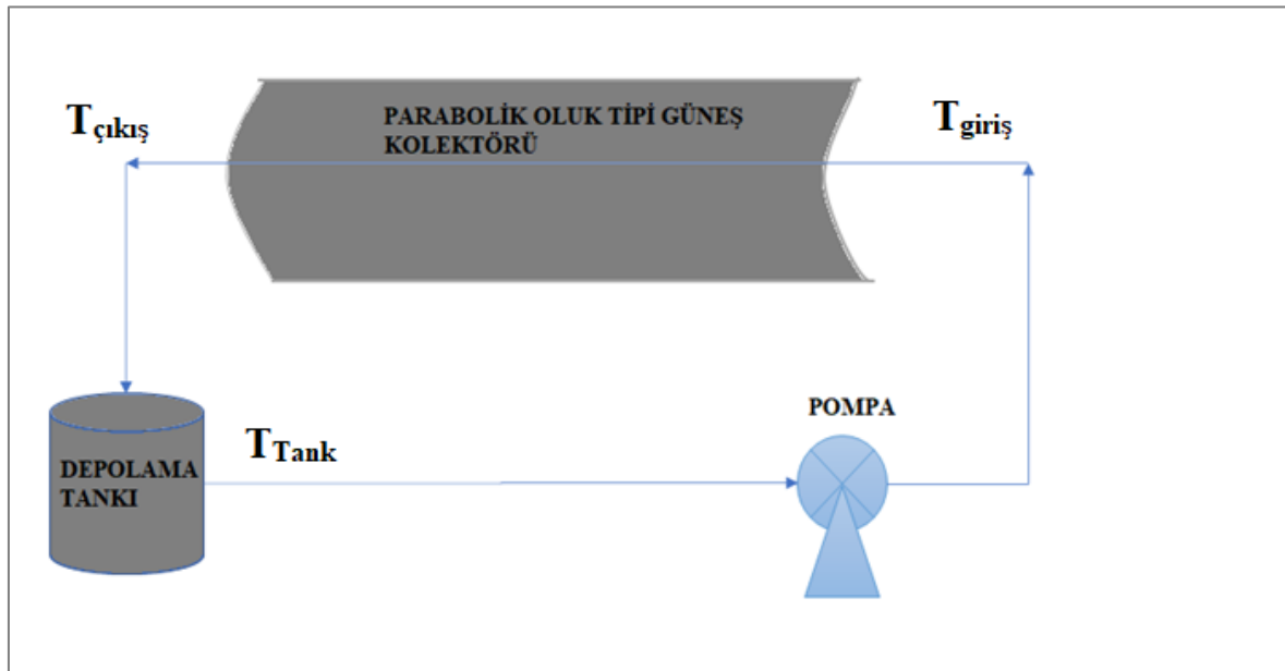
Şekil 6.1. Deneysel çalışma sisteminin şematik gösterimi
