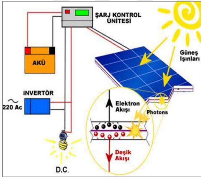
Şekil 3.1. Fotovoltaik sistemlerde elektrik üretimi akış diyagramı (URL-8)
