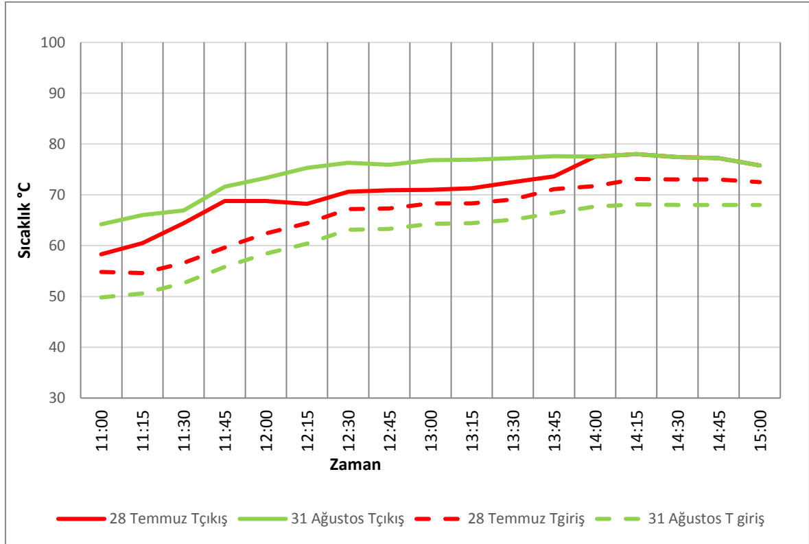
Şekil 6.10. 1,0 L/dk akış hızında gliserin emici boru giriş ve çıkış sıcaklıkları
