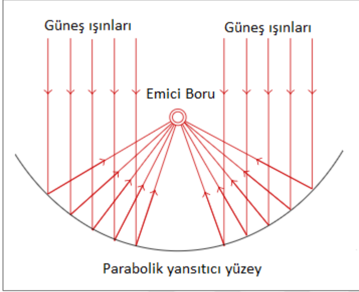
Şekil 4.2. Parabolik yzeyin gneş ışınlarını emici boruya yoğunlaştırılması
