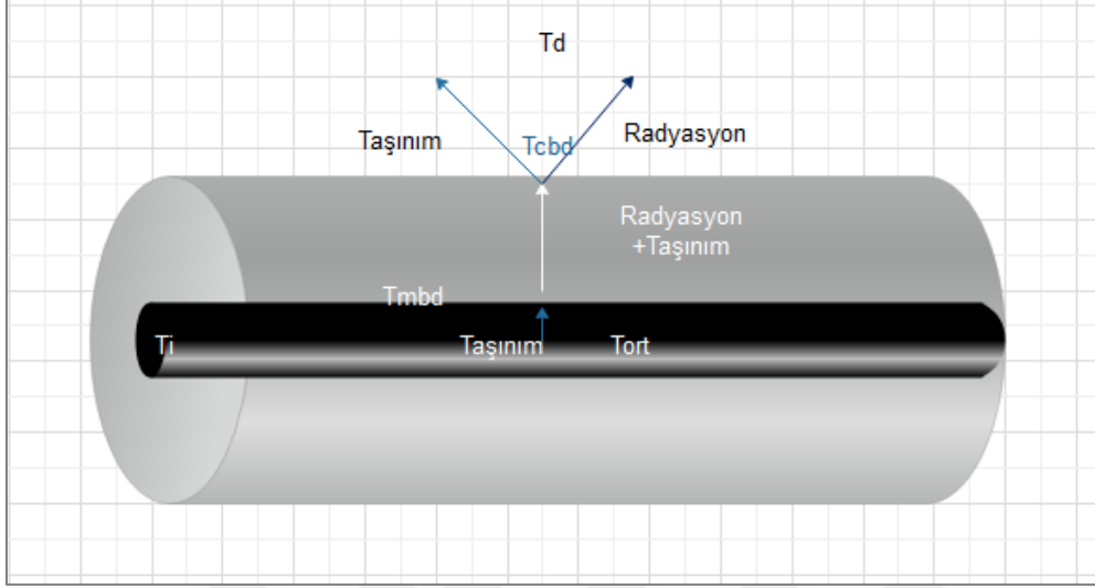
Şekil 5.6. Parabolik oluk tipi güneş kolektöründe ısı transferi termal direnç akımı gösterimi
