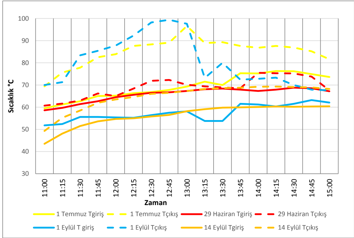
Şekil 6.6. 0,4 L/dk akış hızında gliserin emici boru giriş ve çıkış sıcaklıkları
