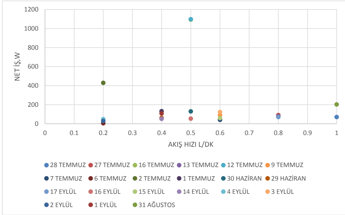
Şekil 6.19. İzopentan için farklı akış hızlarında net iş miktarı
