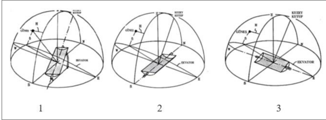
Şekil 4.4. Parabolik oluk tipi güneş kolektörü için konumlandırma türleri. 1. Kutupsal konumlandırma 2. Kuzey-güney konumlandırma 3. Doğu-batı konumlandırma gösterimi
