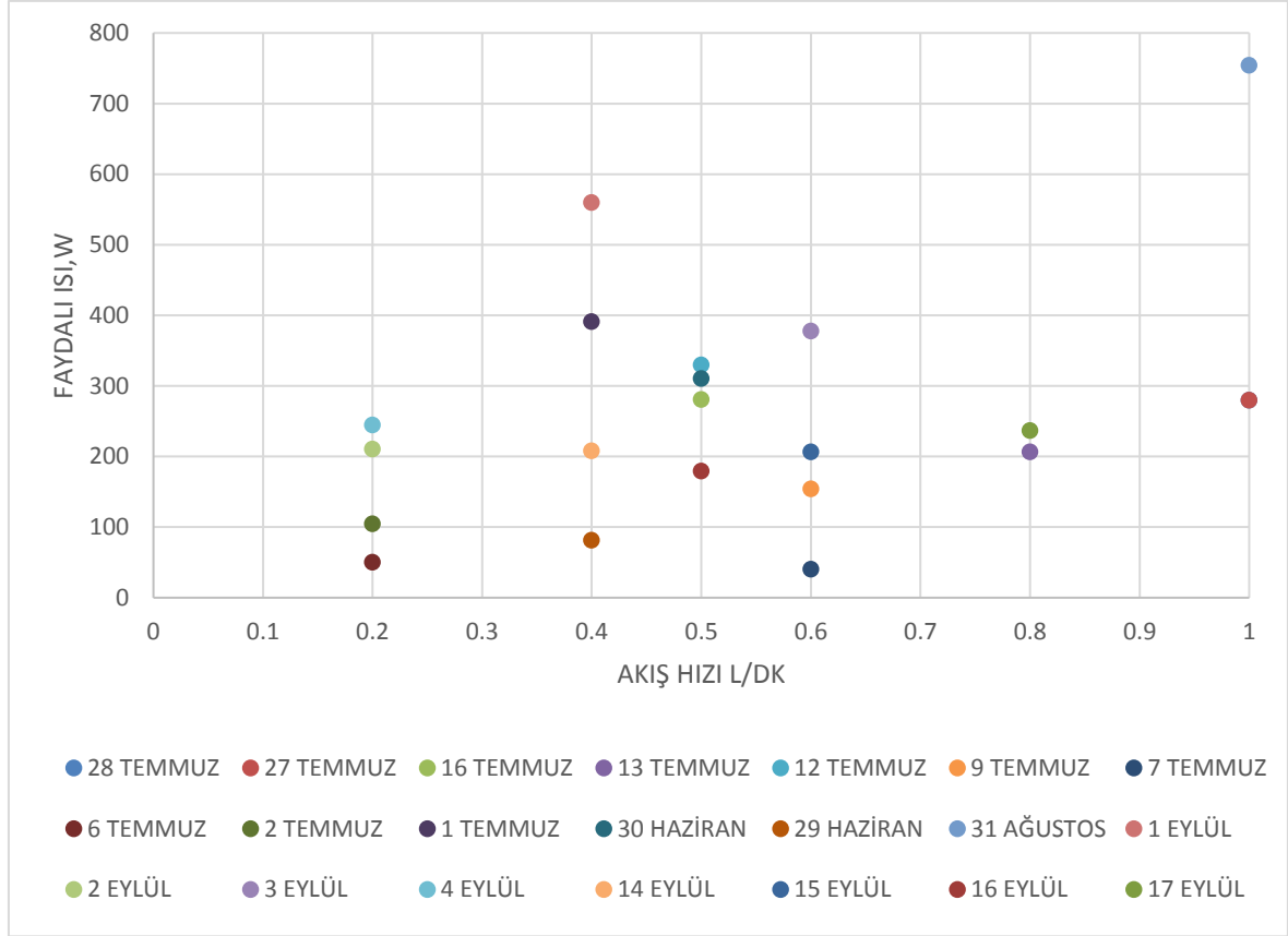
Şekil 6.12. Farklı akış hızlarında hesaplanan faydalı ısı miktarı
