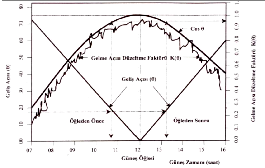
Şekil 5.4. Gelme açısı düzeltme faktörünün geliş açısına göre değişimi (Duffie ve Beckman, 2006)
