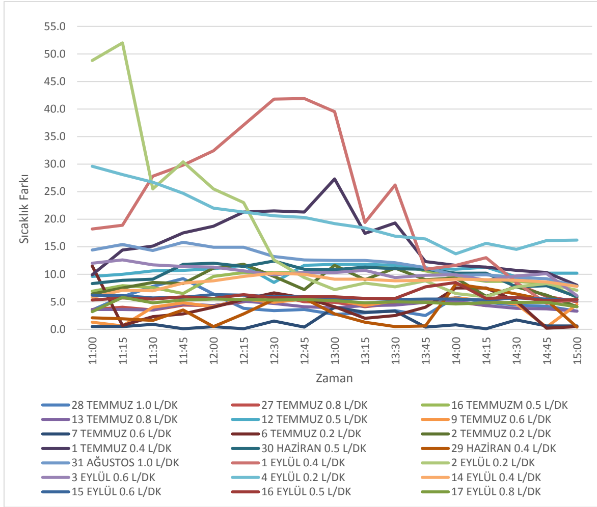
Şekil 6.11. Farklı akış hızlarında gün içerisinde oluşan sıcaklık farkları
