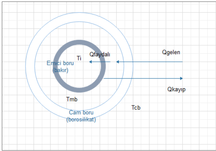
Şekil 5.5. Parabolik oluk kolektörde ısı transfer akışkanından çevreye olan ısı transfer şeması
