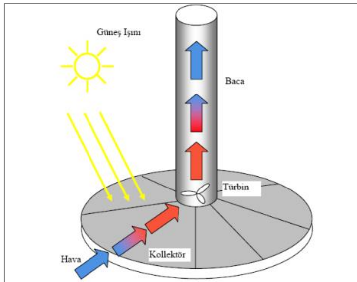
Şekil 3.6. Güneş bacası (Gün ve Kurban, 2011)
