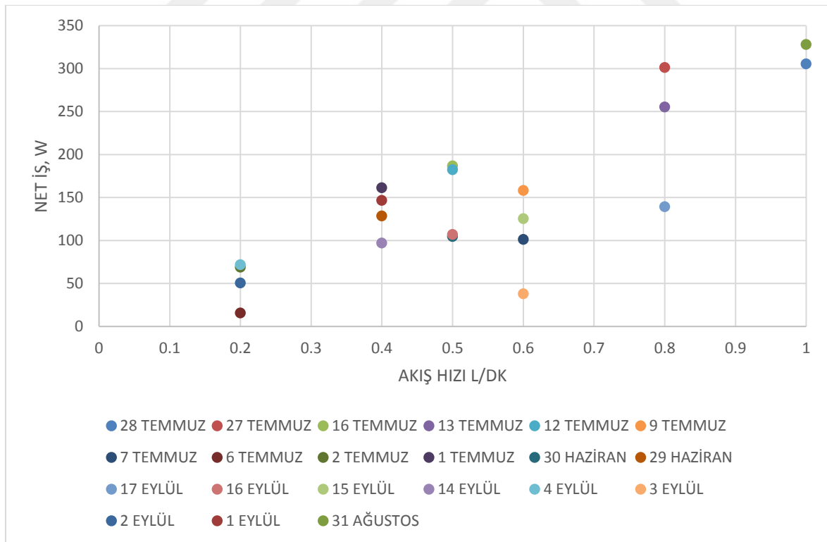
Şekil 6.16. Bütan için farklı akış hızlarında net iş miktarı
