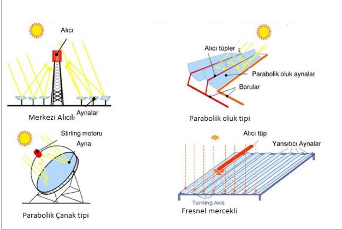
Şekil 3.7. Yoğunlaştırılmış güneş enerjisi sistemleri (URL-13)
