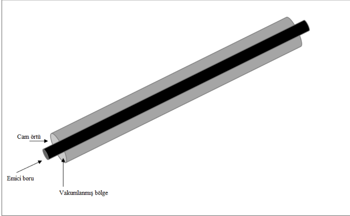
Şekil 4.6. Cam örtü ve emici boruyu içeren toplayıcı kısım
