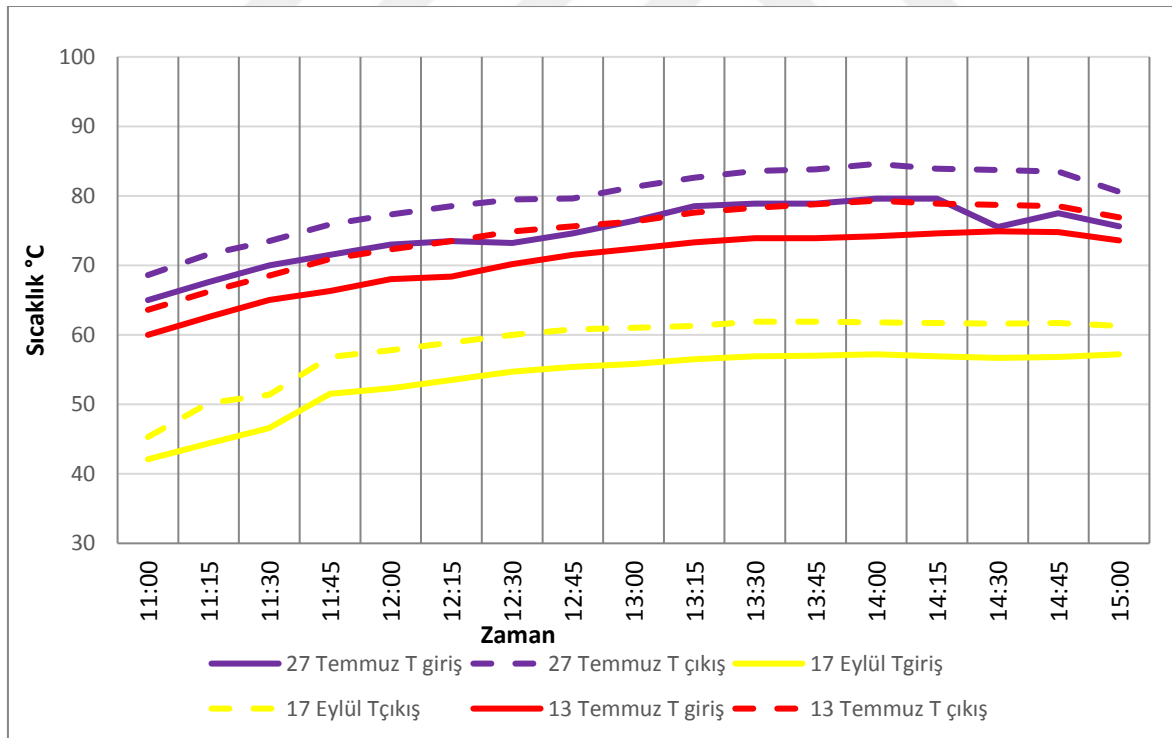
Şekil 6.9. 0, L/dk akış hızında gliserin emici boru giriş ve çıkış sıcaklıkları
