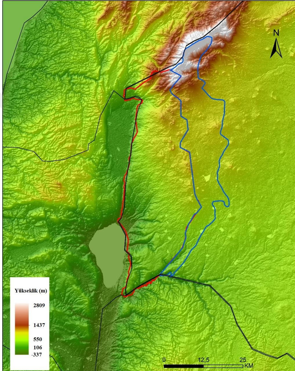
Şekil 2. Golan tepelerinin Sayısal Yükseklik Modeli Haritası.
