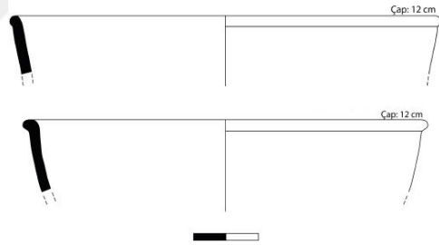
Şekil 35: DSA TİP 16 ve Tarsus benzeri örneği (Jones, 1950: fig. 188, E).
