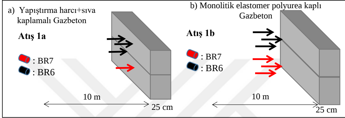
Şekil 3.1. Gazbeton duvarın geniş iki kısa yüzeyine atışın şematik gösterimi
