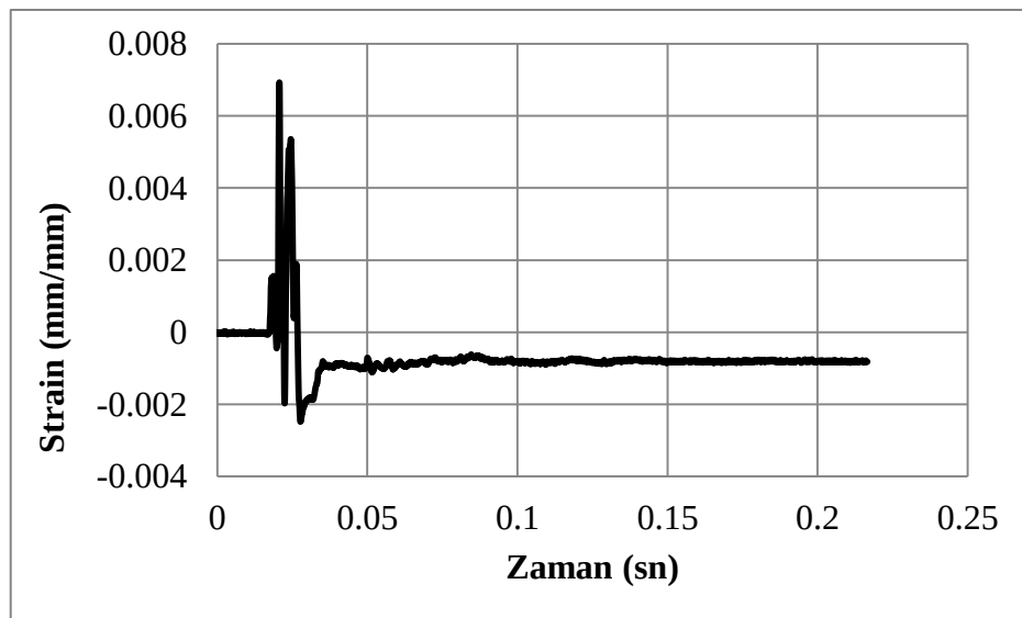
Şekil 4.19. C50sDi deney numunesine ait birim deformasyon-zaman grafiği
