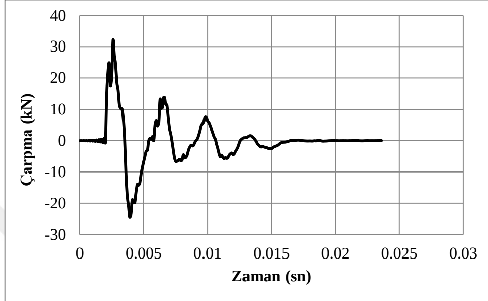
Şekil 4.28. C100sOr deney numunesine ait darbe yükü/zaman grafiği
