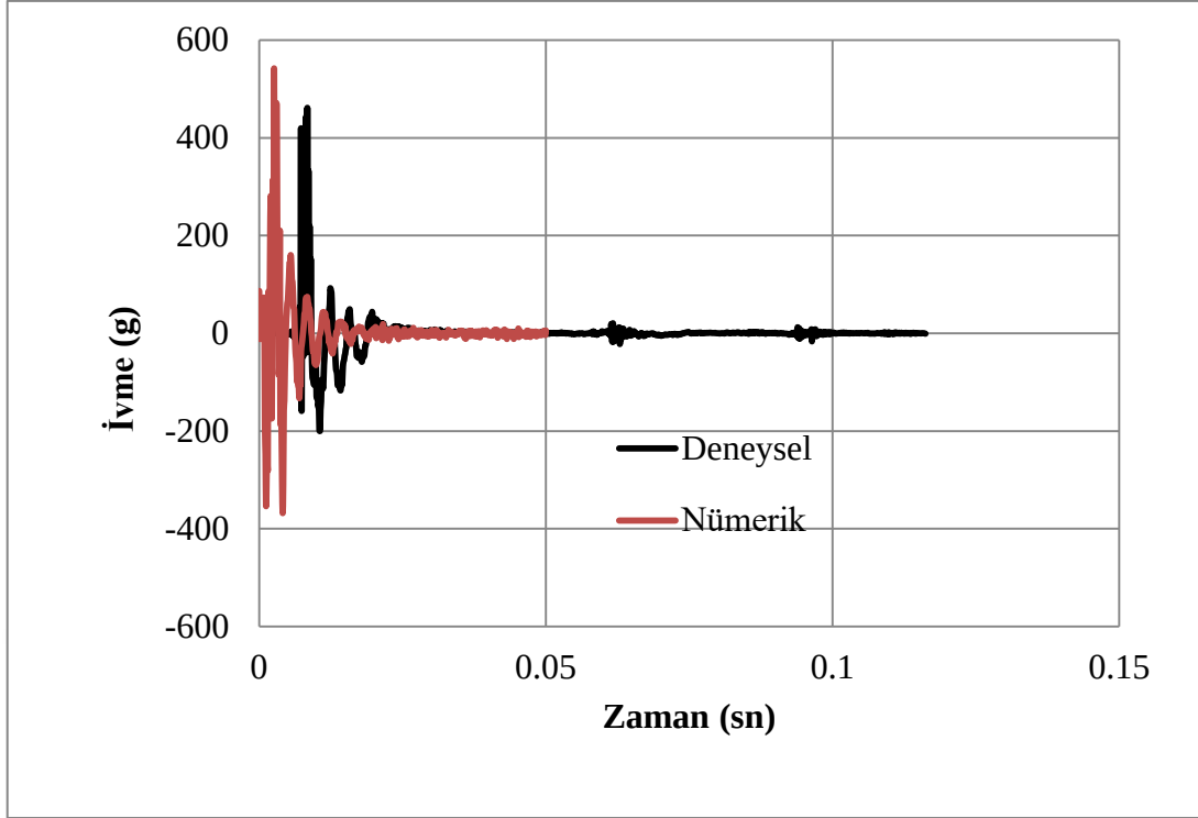
Şekil 4.10. C50dOr ivme-zaman grafik değerleri
