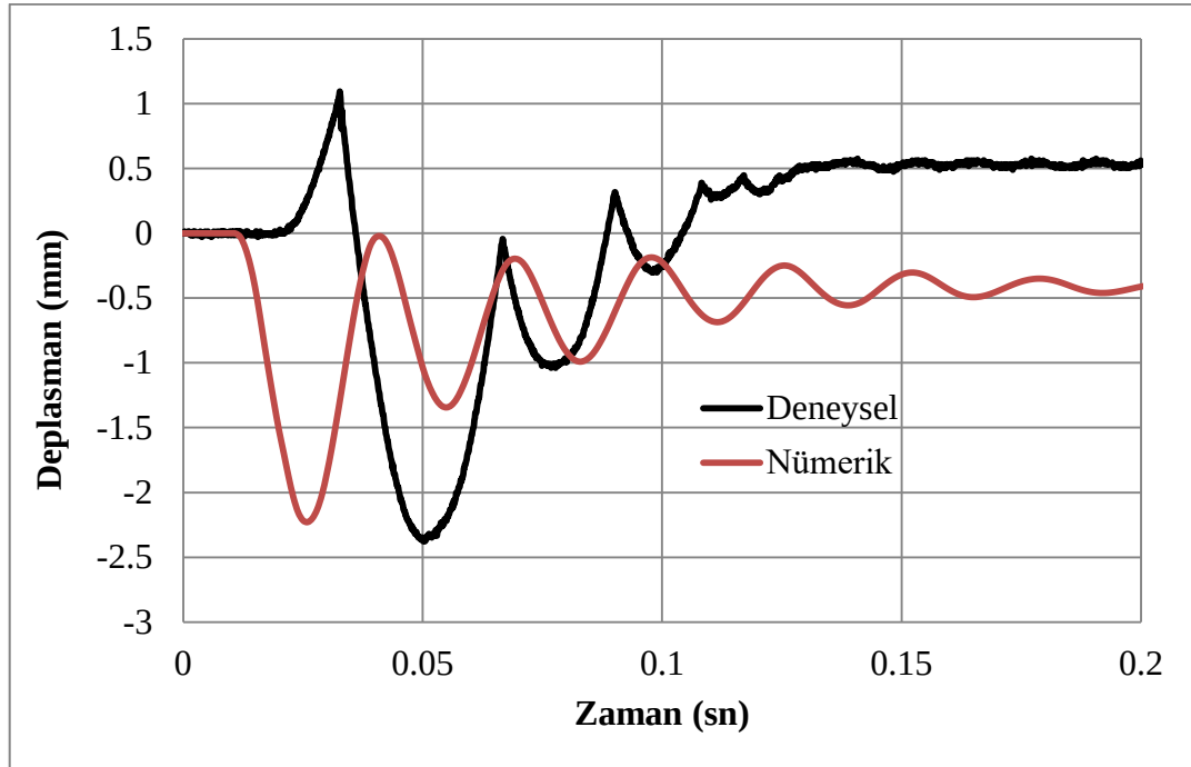
Şekil 4.6. C50sOr yer değıştirme-zaman grafik değerleri
