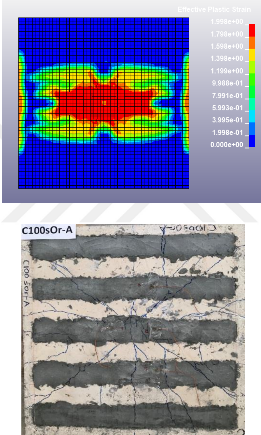
Şekil 4.67. C100sOr-A numunesinin deney sonrası çatlak dağılımı
