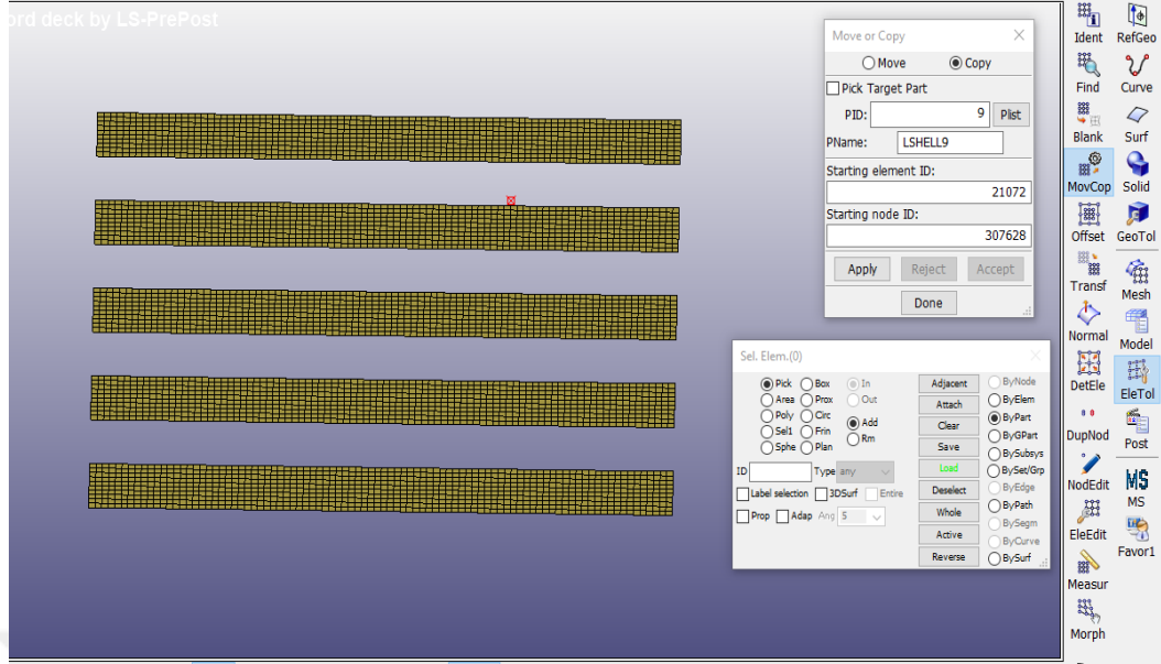
Şekil 3.43. TRM şeritlerin mesh işlemlerinin tek part haline getirilmesi
