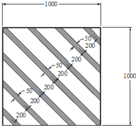
50 mm TRM Diyagonal Tek Yön
