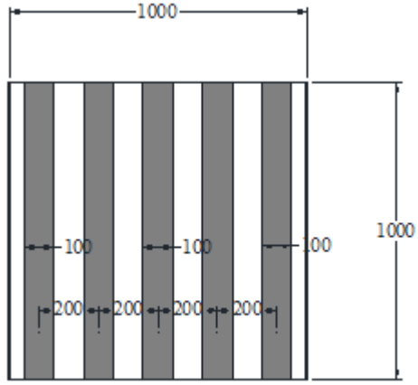
100 mm TRM Ortogonal Tek Yön
