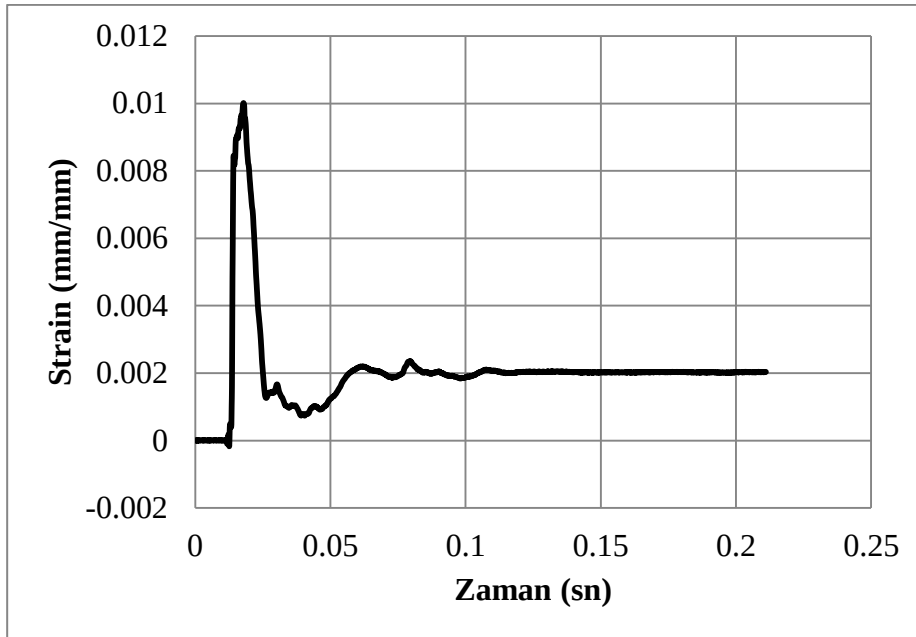
Şekil 4.69. C100sOr-A deney numunesine ait birim deformasyon-zaman grafiği
