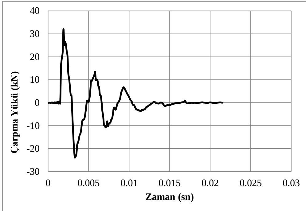
Şekil 4.83. C100dDi-A deney numunesine ait darbe yükü/zaman grafiği
