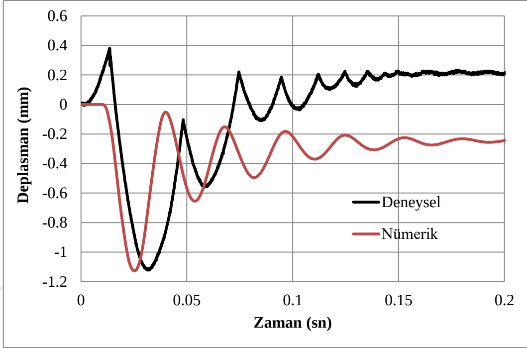
Şekil 4.21. C50dDi yer değiştirme-zaman grafik değerleri
