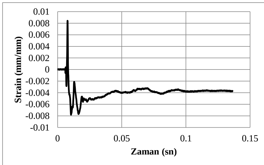
Şekil 4.14. C50dOr deney numunelerine ait birim deformasyon-zaman grafiği
