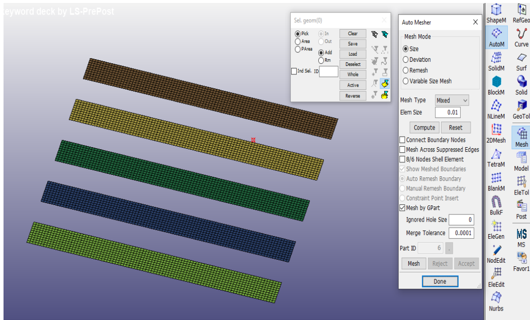
Şekil 3.42. TRM şeritlerin sonlu elemanlara (mesh) bölünme işlemi
