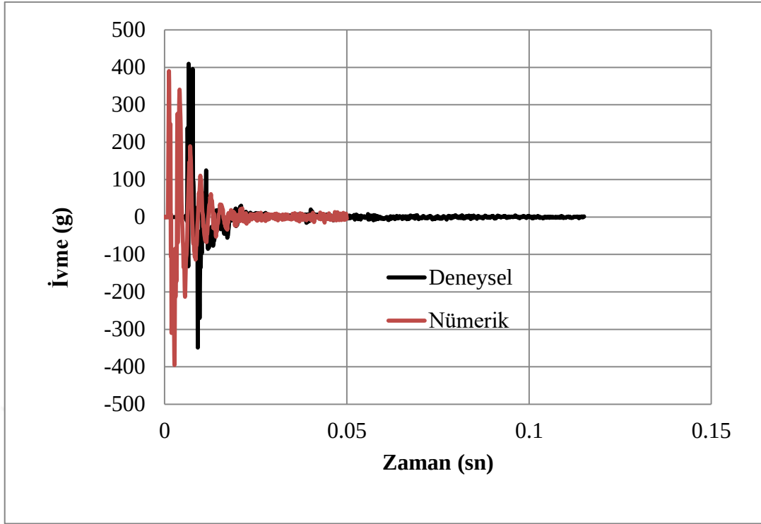
Şekil 4.15. C50sDi ivme-zaman grafik değerleri
