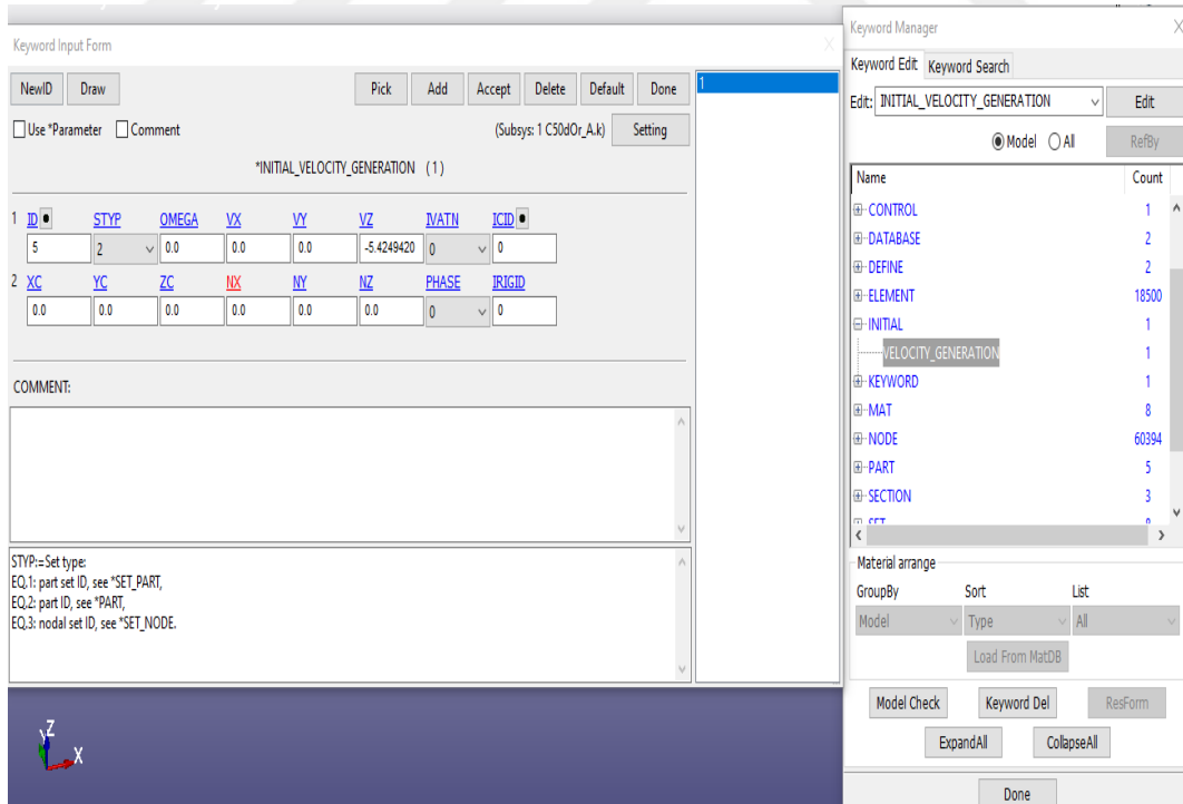
Şekil 3.45. Sisteme yük atamasının yapılması
