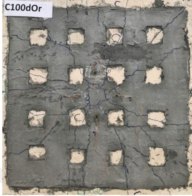
Şekil 4.32. C100dOr numunesinin deney sonrası çatlak dağılımı
