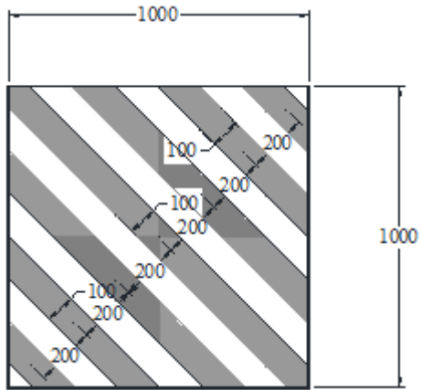
100 mm TRM Diyagonal Tek Yön
