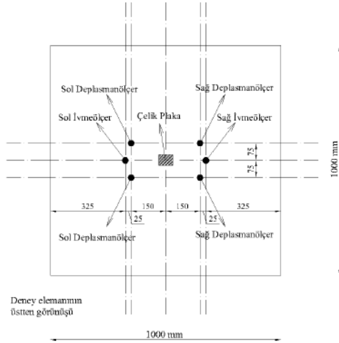
Şekil 3.29. Çelik plaka, ivme ve deplasman ölçü aletlerin yerleşim detayı
