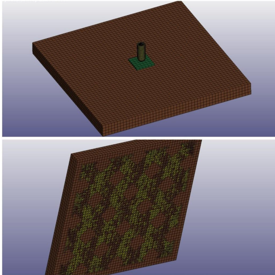
Şekil 3.44. Sonlu elemanlara bölünme işlemlerin genel görünümü
