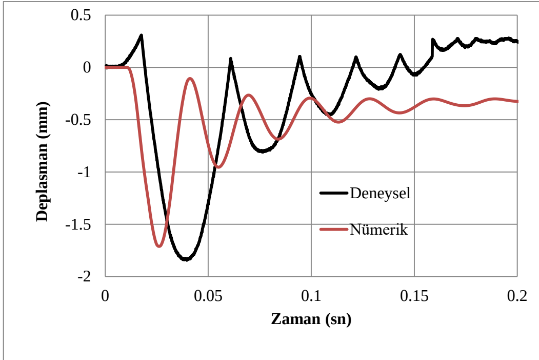
Şekil 4.11. C50dOr yer değiştirme-zaman grafik değerleri
