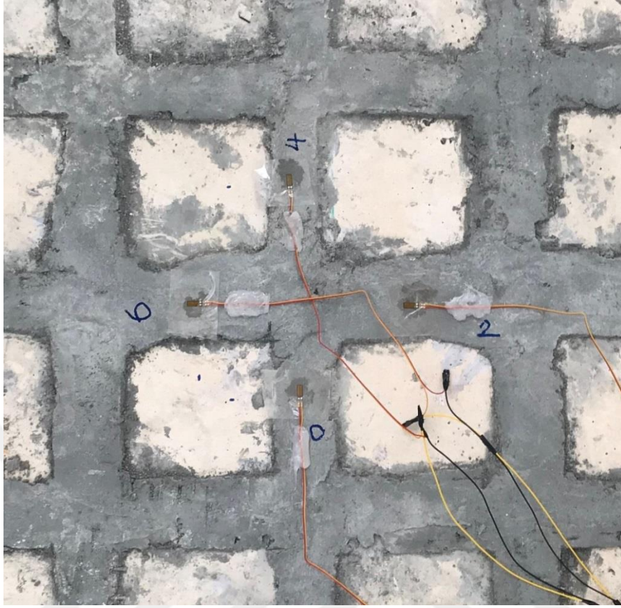
Şekil 3.11. Strain-gauge montajı
