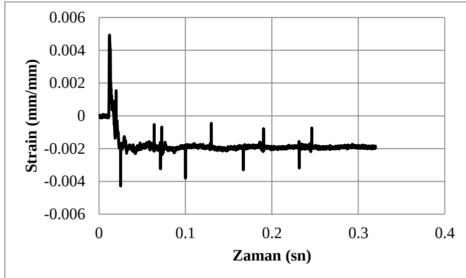
Şekil 4.79. C100sDi-A deney elemanına ait birim deformasyon-zaman grafiği
