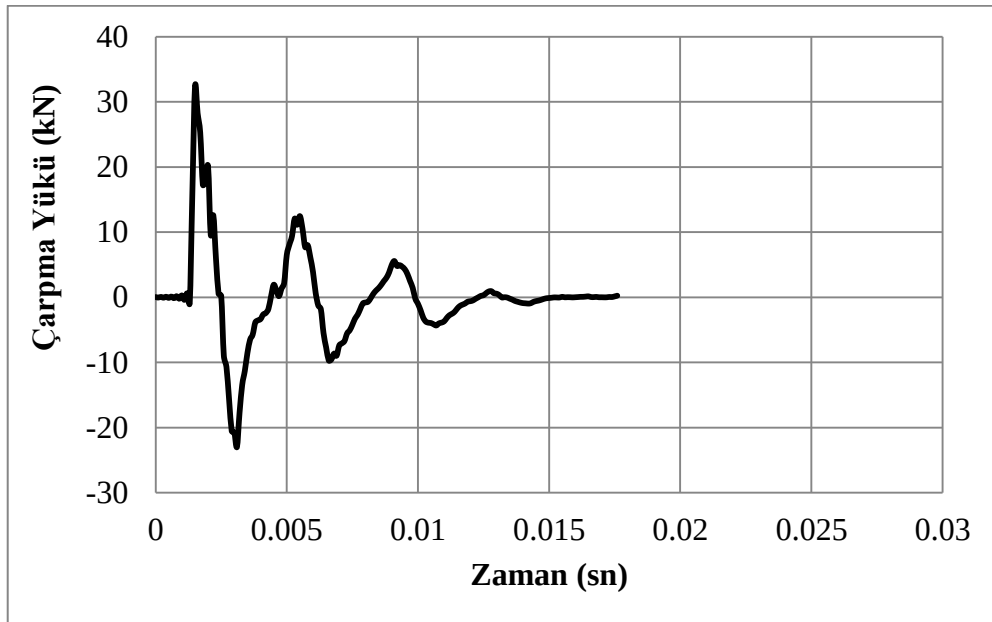
Şekil 4.73. C100dOr-A deney numunesine ait darbe yükü/zaman grafiği
