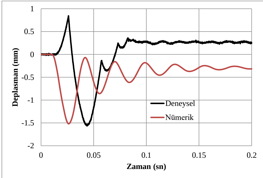
Şekil 4.16. C50sDi yer değıştirme-zaman grafik değerleri
