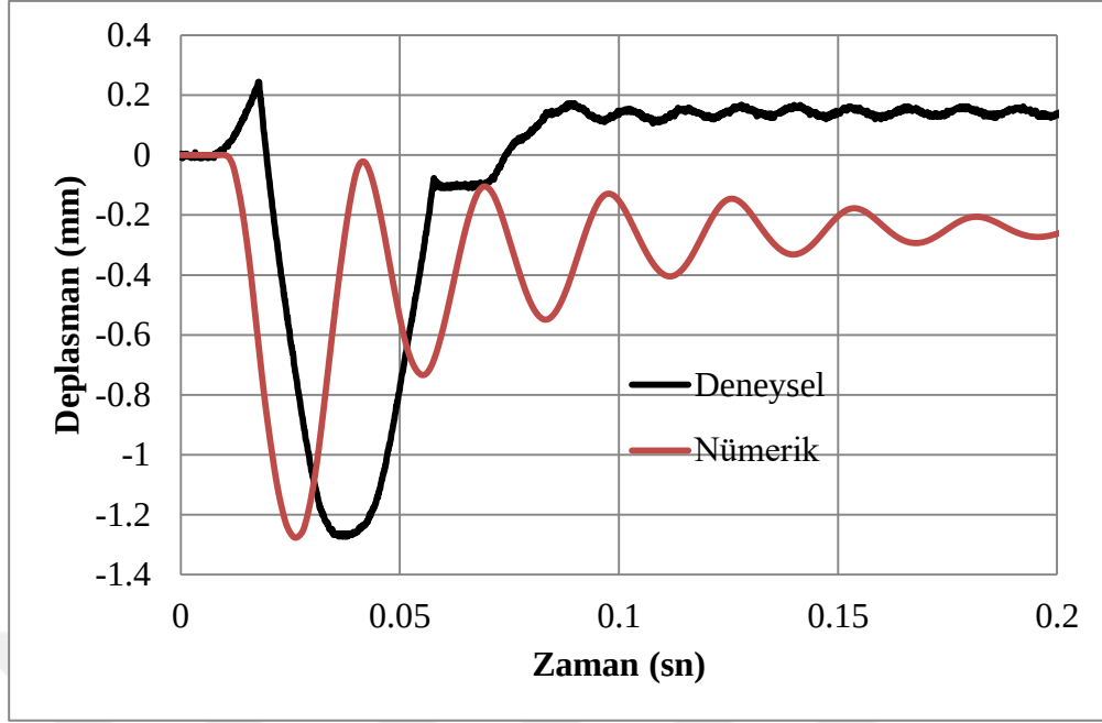
Şekil 4.31 C100dOr yer değiştirme-zaman grafik değerleri
