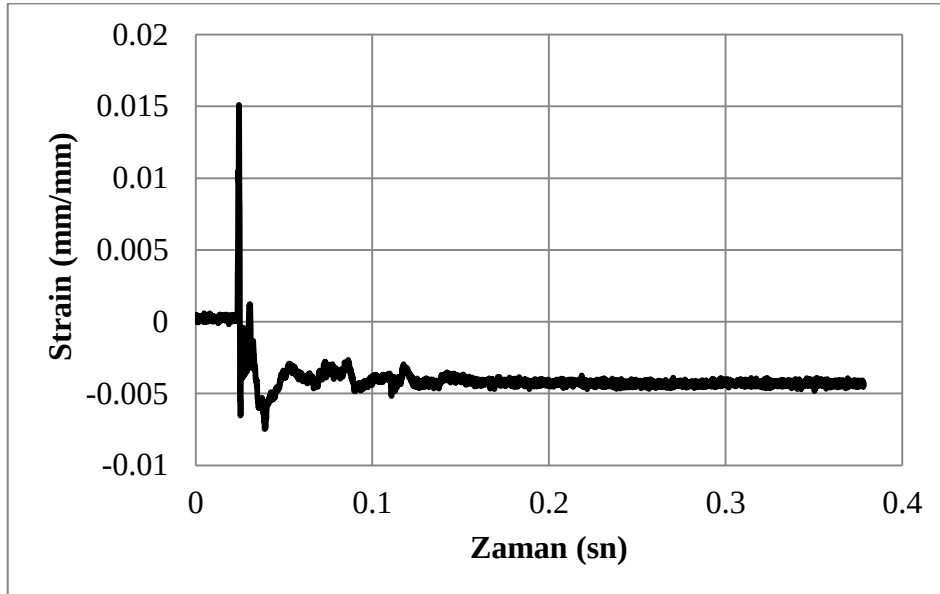
Şekil 4.9. C50sOr deney numunelerine ait birim deformasyon-zaman grafiği
