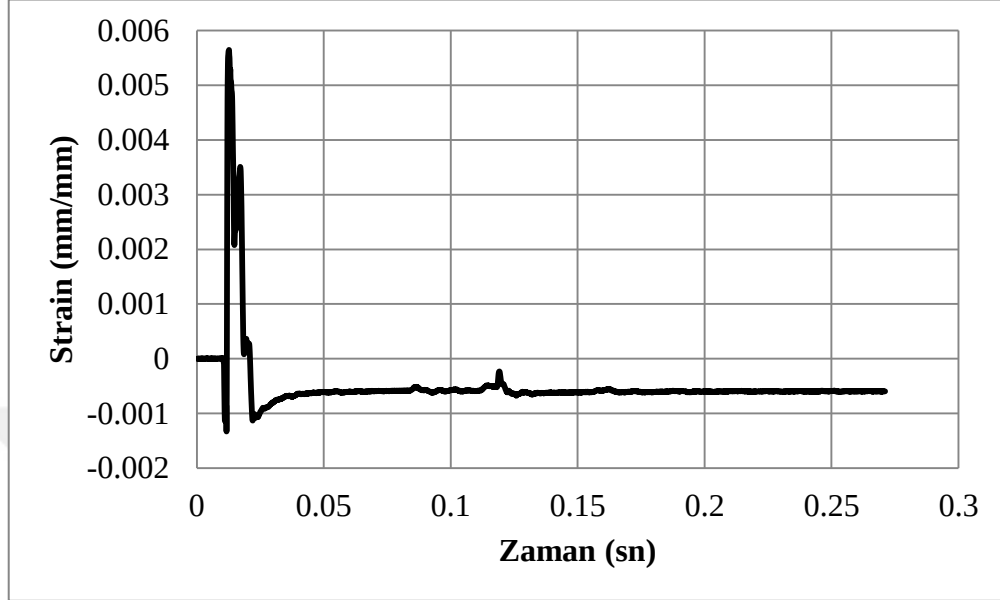
Şekil 4.74. C100dOr-A deney numunesine ait birim deformasyon-zaman grafiği
