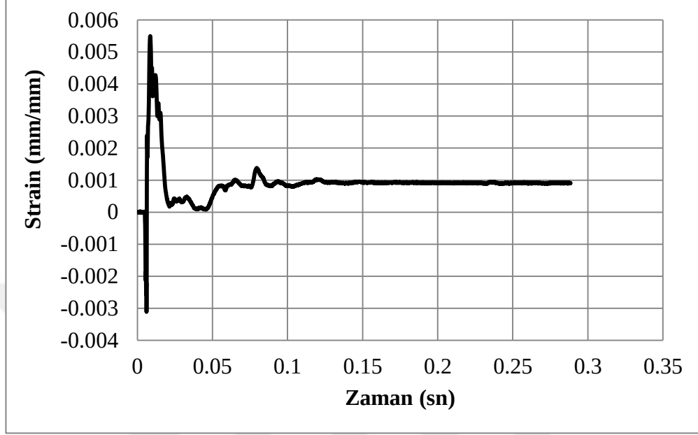
Şekil 4.24. C50dDi deney numunesine ait birim deformasyon-zaman grafiği
