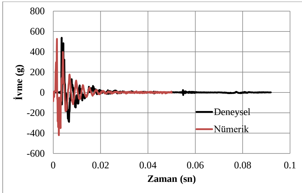
Şekil 4.30. C100dOr ivme-zaman grafik değerleri
