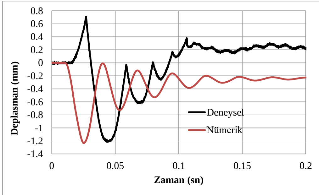
Şekil 4.56. C50sDi-A yer değiştirme-zaman grafik değerleri
