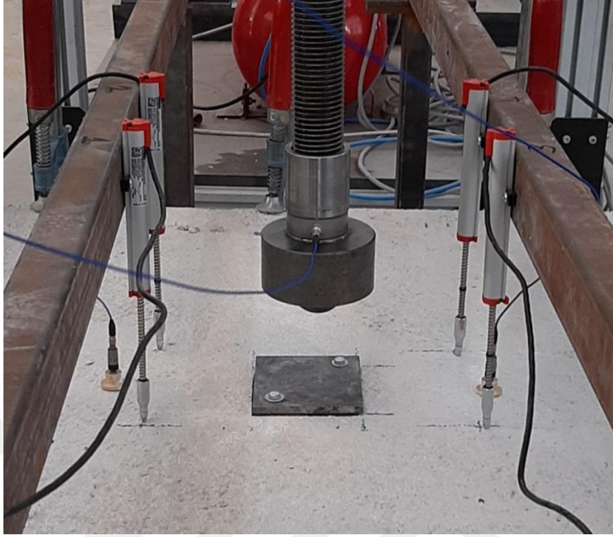
Şekil 3.3. Plaka - kauçuk montaj
