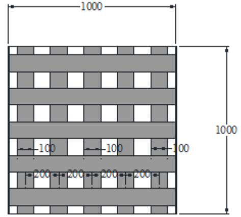
100 mm TRM Ortogonal Çift Yön
