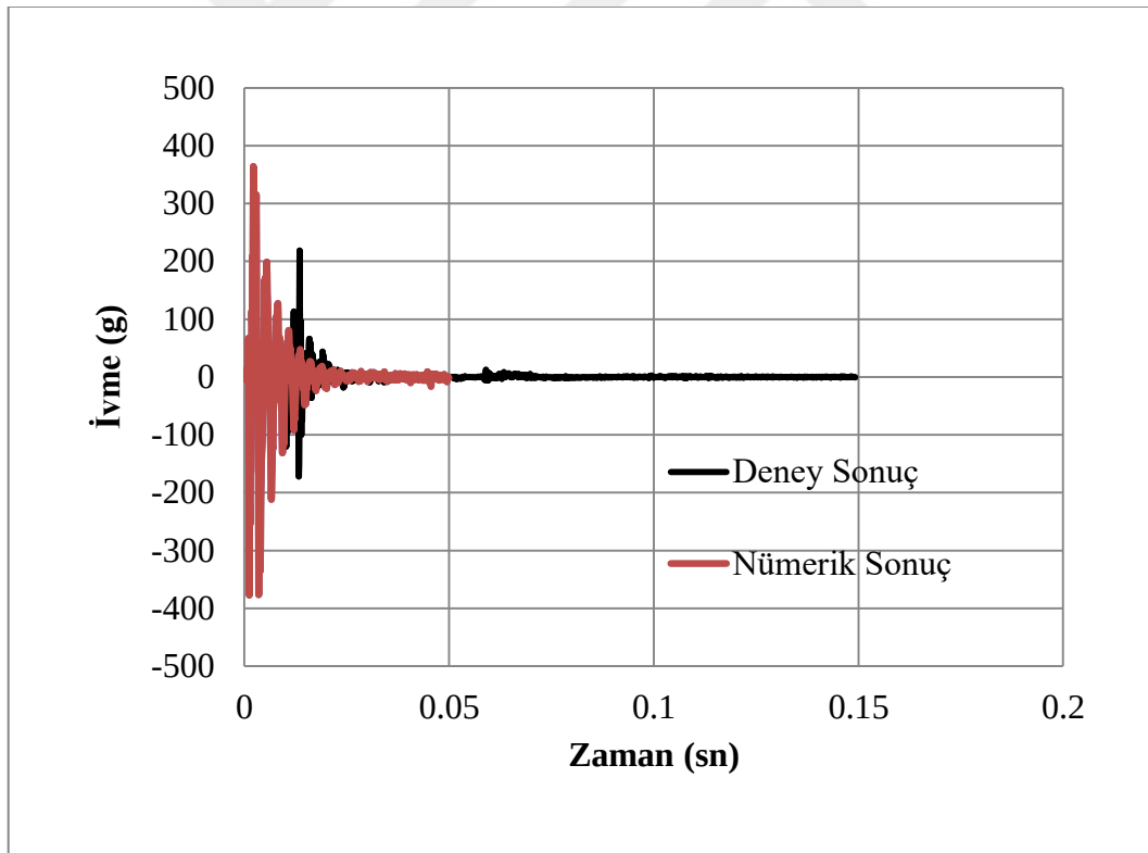
Şekil 4.1. Referans ivme-zaman grafik değerleri
