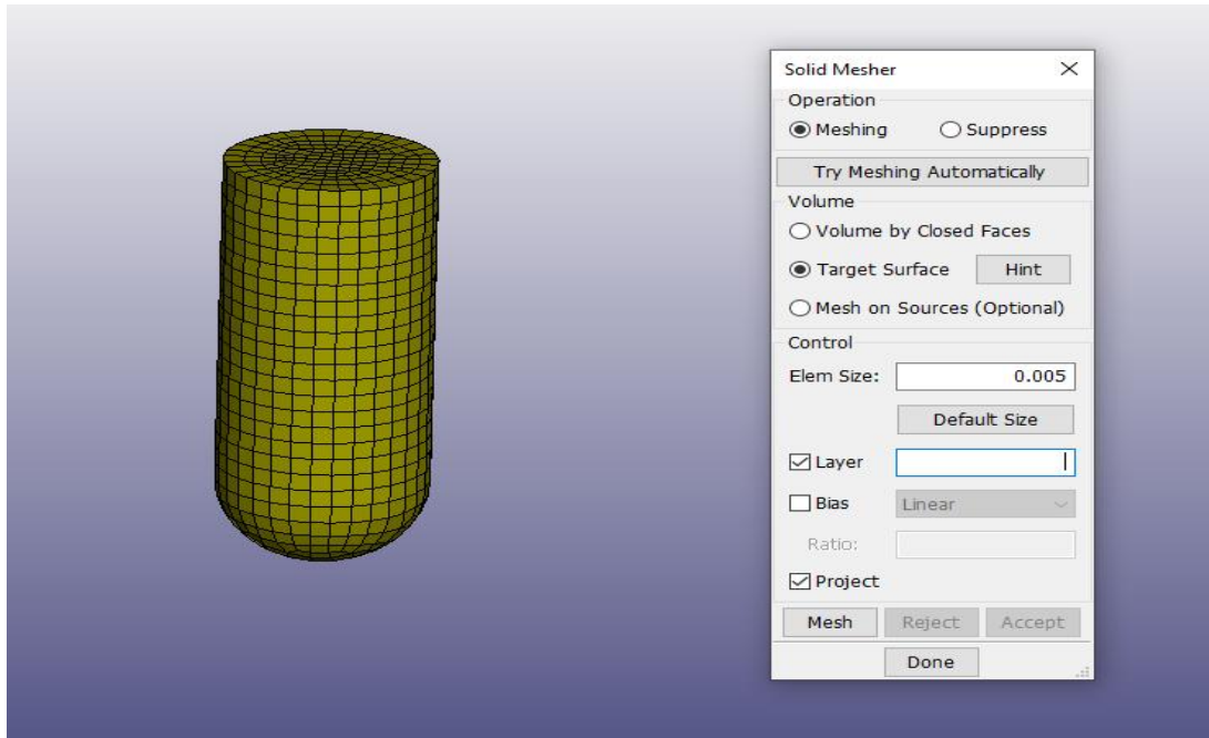
Şekil 3.41. Çelicin sonlu elemanlara bölünme işlemi
