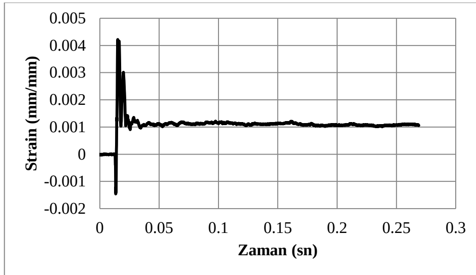
Şekil 4.39. C100sDi deney numunesine ait birim deformasyon-zaman grafiği
