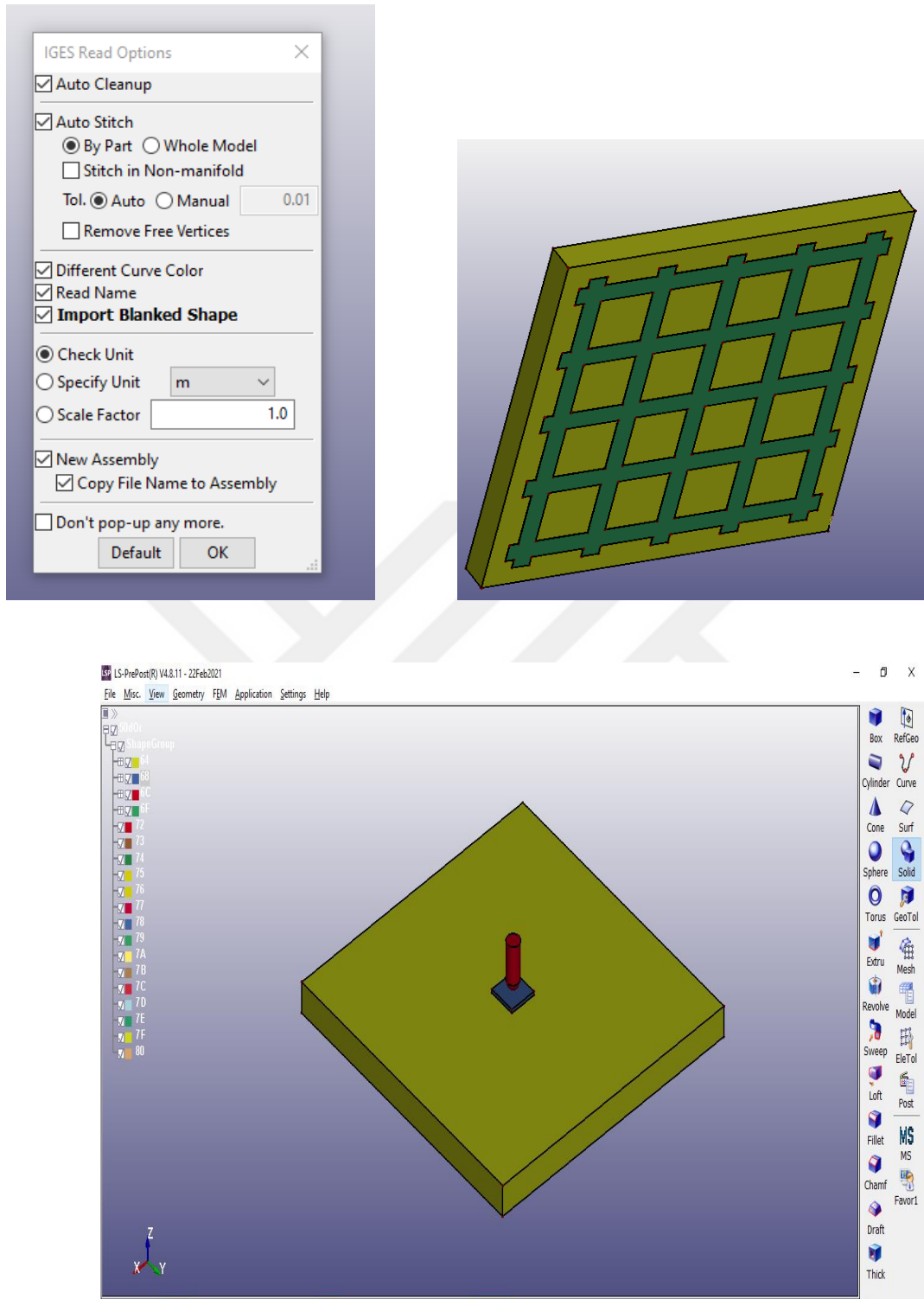
Şekil 3.31. Deneysel modelin LS DYNA programında oluşturulması
