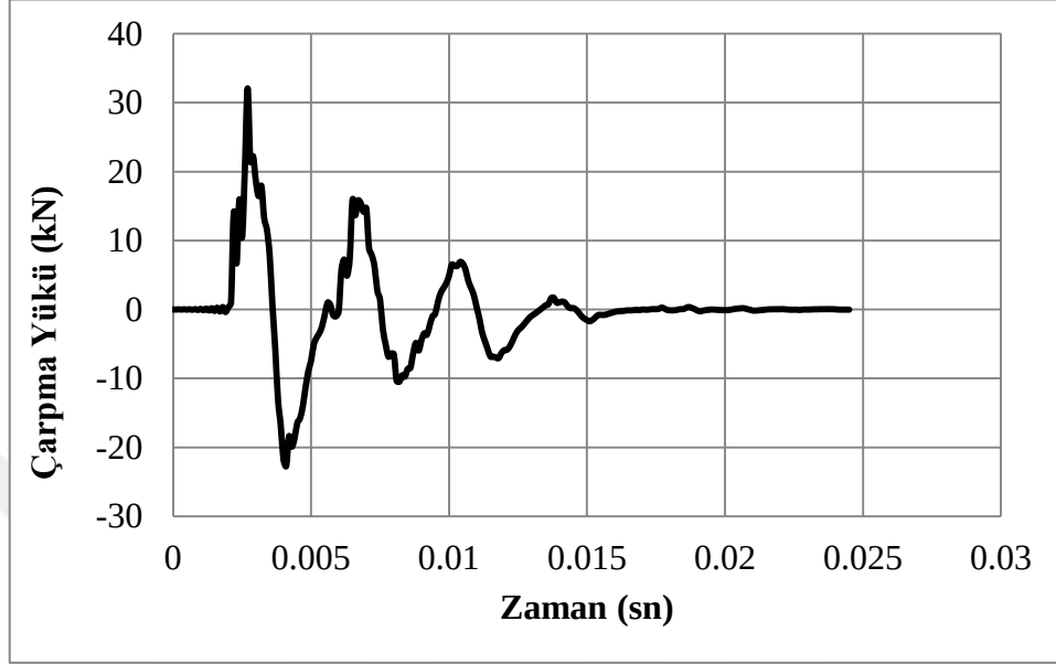
Şekil 4.13. C50dOr deney numunelerine ait darbe yükü/zaman grafiği
