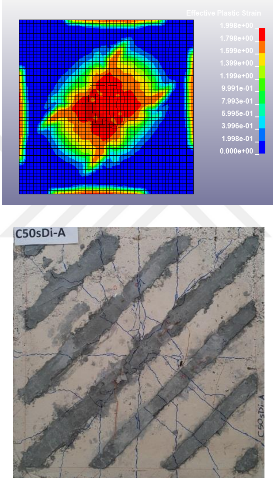
Şekil 4.57. C50sDi-A numunesinin deney sonrası çatlak dağılımı
