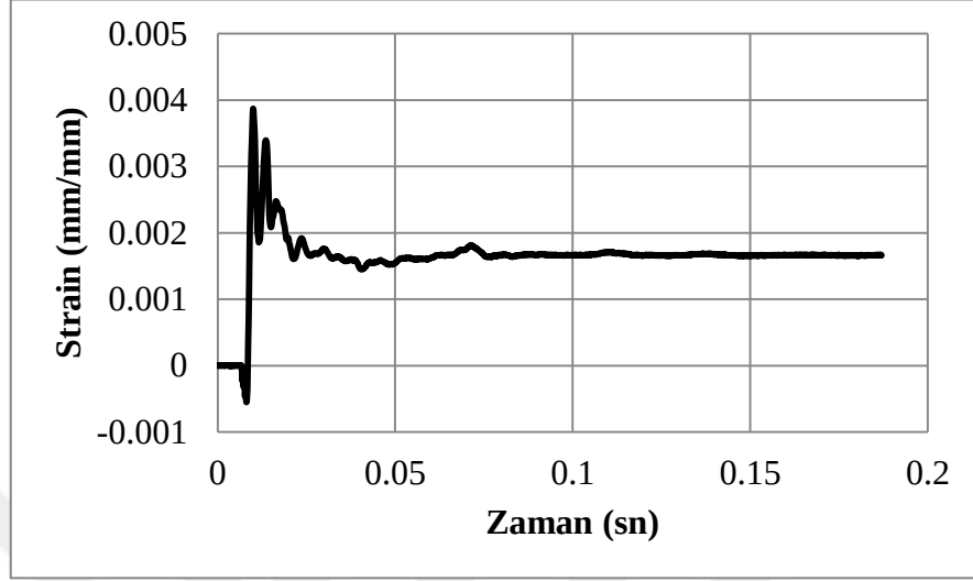
Şekil 4.84. C100dDi-A deney numunesine ait birim deformasyon-zaman grafiği
