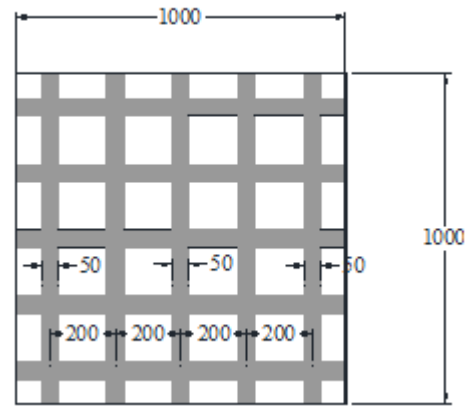
50 mm TRM Ortogonal Çift Yön
