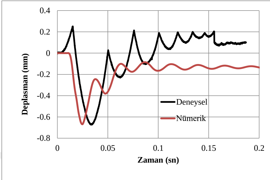
Şekil 4.81. C100dDi-A yer değiştirme-zaman grafik değerleri
