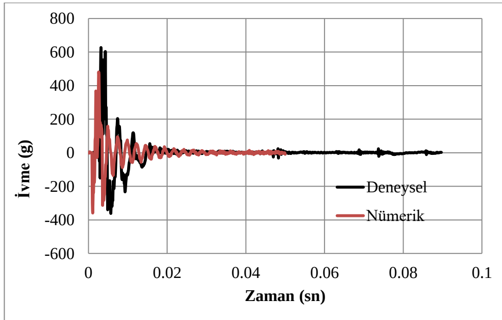
Şekil 4.70. C100dOr-A ivme-zaman grafik değerleri
