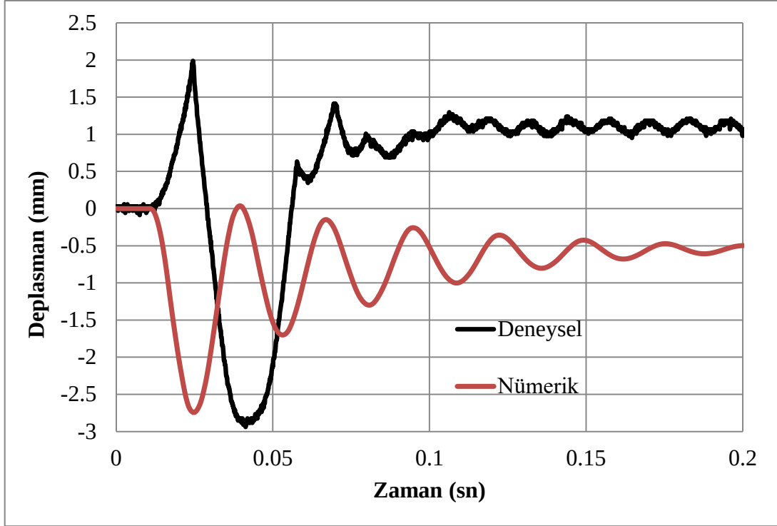
Şekil 4.2. Referans yer değiştirme-zaman grafik değerleri
