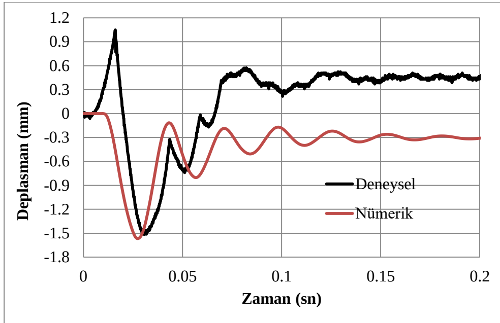
Şekil 4.46. C50sOr-A yer değiştirme-zaman grafik değerleri
