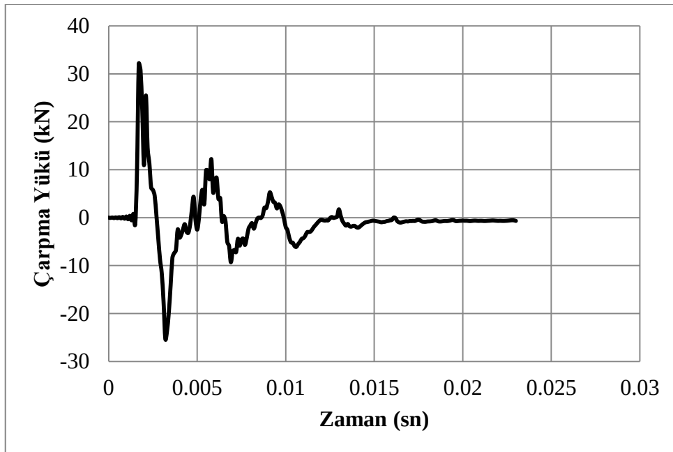
Şekil 4.33. C100dOr deney numunesine ait darbe yükü/zaman grafiği
