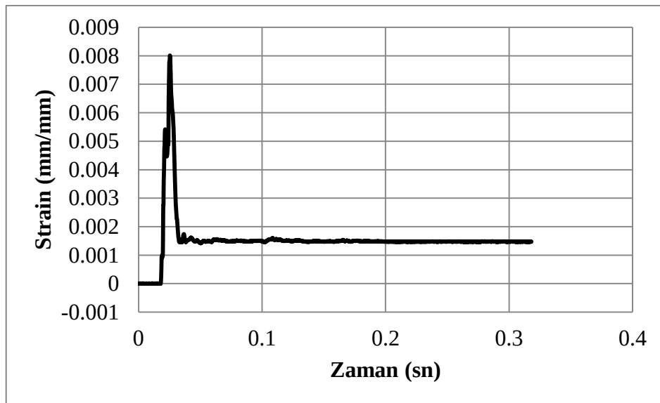
Şekil 4.59. C50sDi-A deney numunesine ait birim deformasyon-zaman grafiği
