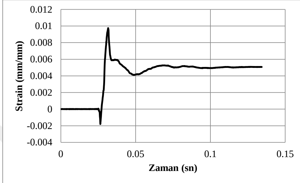
Şekil 4.54. C50dOr-A deney numunesine ait birim deformasyon-zaman grafiği
