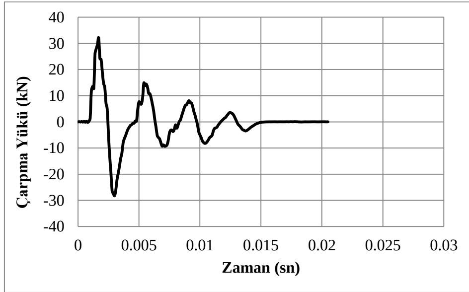
Şekil 4.53. C50dOr-A deney numunesine ait darbe yükü/zaman grafiği
