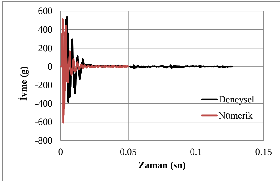
Şekil 4.20. C50dDi ivme-zaman grafik değerleri
