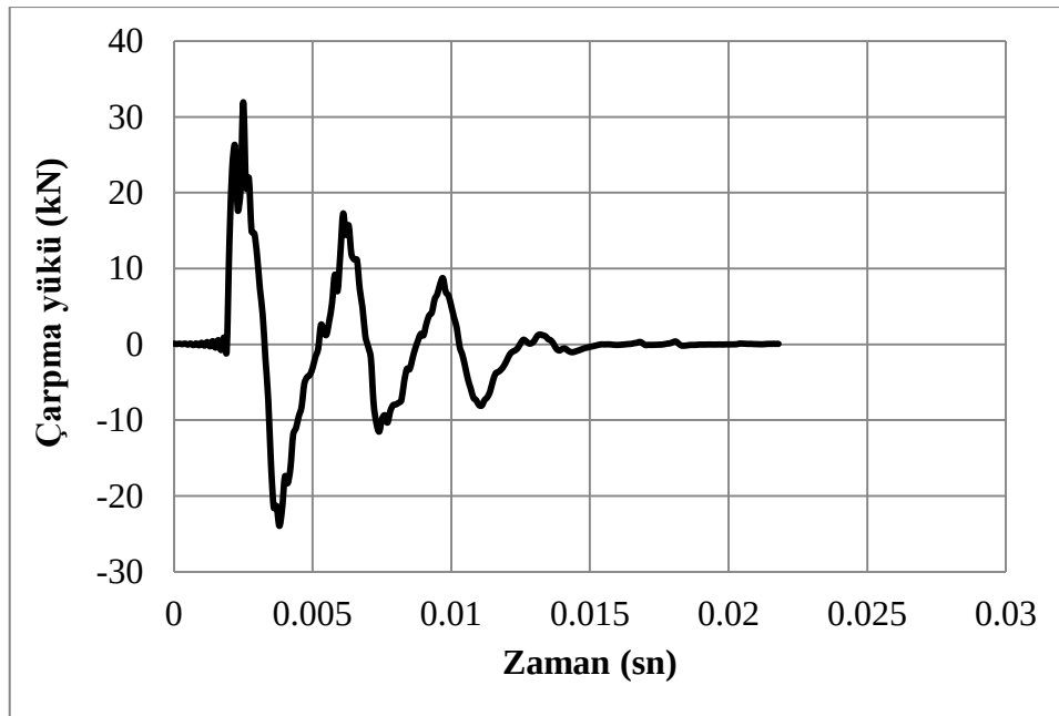
Şekil 4.43. C100dDi deney numunesine ait darbe kuvveti/zaman grafiği
