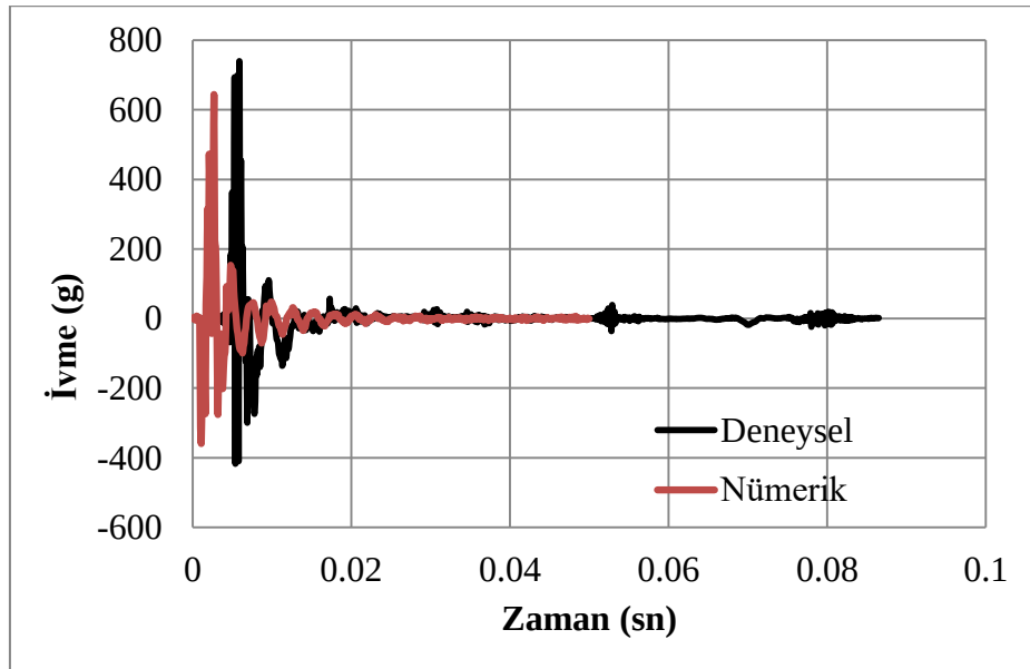
Şekil 4.80. C100dDi-A ivme-zaman grafik değerleri
