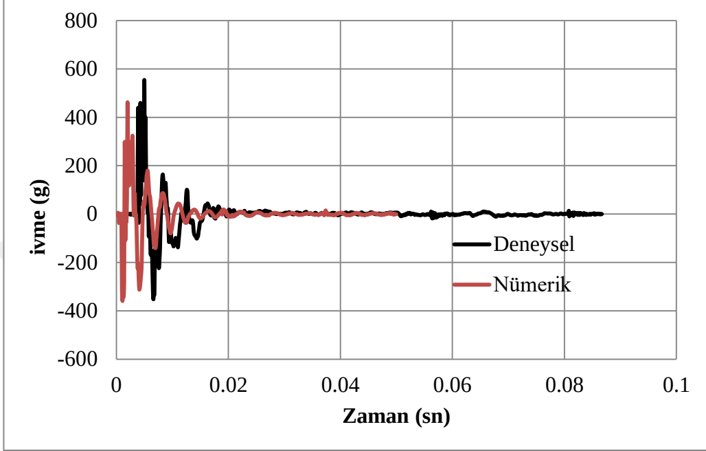
Şekil 4.75. C100sDi-A ivme-zaman grafik değerleri
