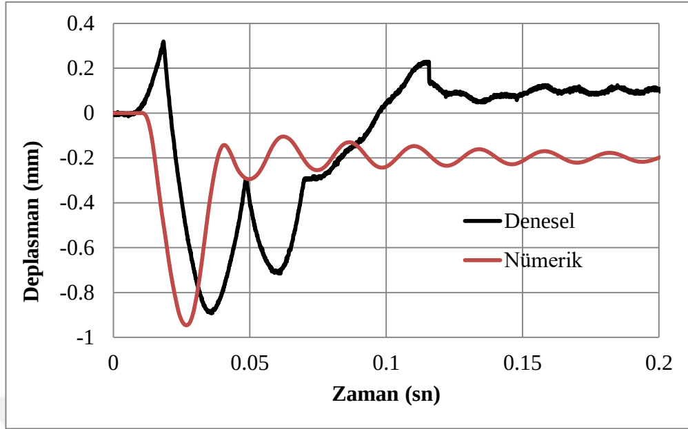
Şekil 4.71. C100dOr-A yer değıştirme-zaman grafik değeri
