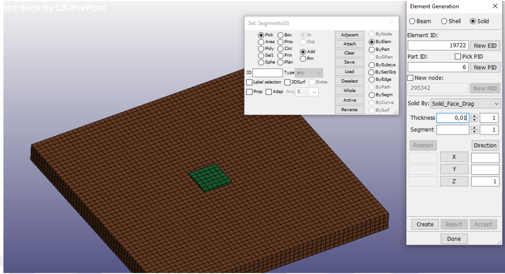
Şekil 3.40. Çelik plakanın sonlu elemanlara bölünme işlemi
