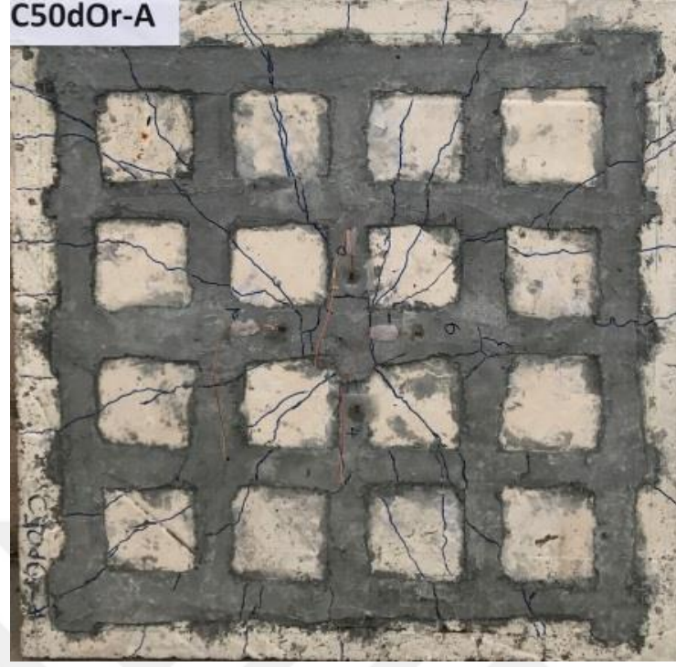
Şekil 4.52. C50dOr-A numunesinin deney sonrası çatlak dağılımı
