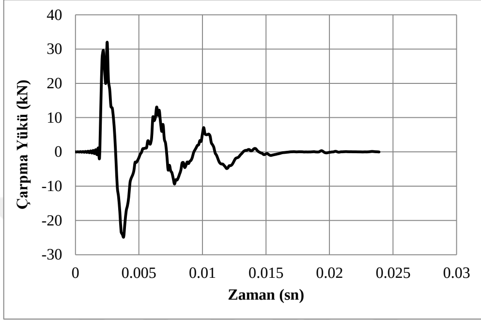
Şekil 4.38. C100sDi deney numunesine ait darbe yükü/zaman grafiği
