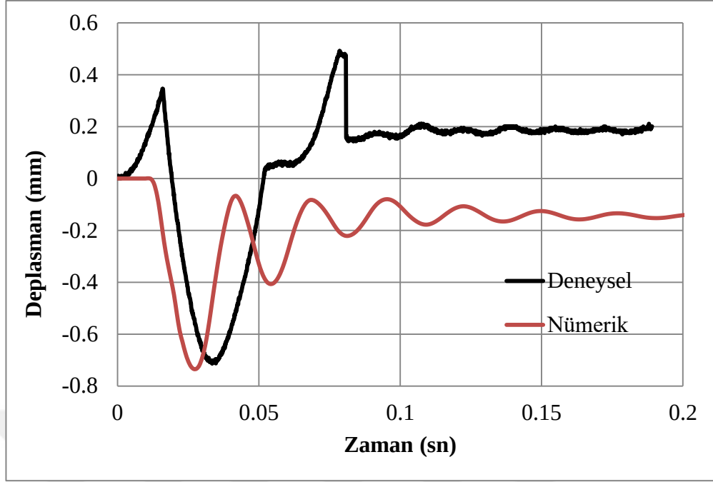
Şekil 4.61. C50dDi-A yer değiştirme-zaman grafik değerleri
