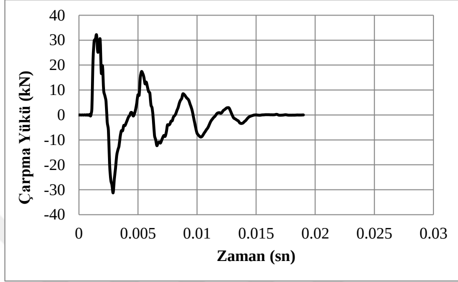
Şekil 4.68. C100sOr-A deney numunesine ait darbe yükü/zaman grafiği
