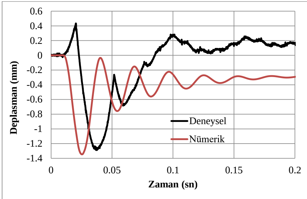
Şekil 4.36. C100sDi yer değiştirme-zaman grafik değerleri
