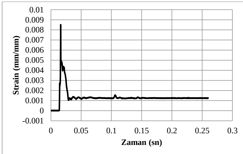
Şekil 4.29. C100sOr deney numunesine ait birim deformasyon-zaman grafiği
