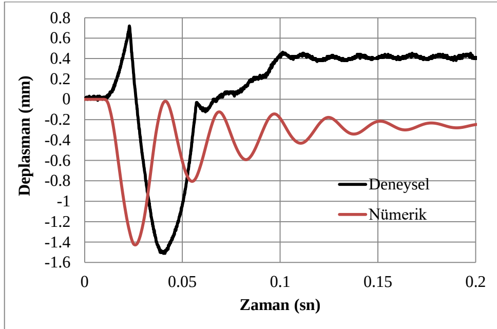
Şekil 4.26. C100sOr yer değiştirme-zaman grafik değerleri
