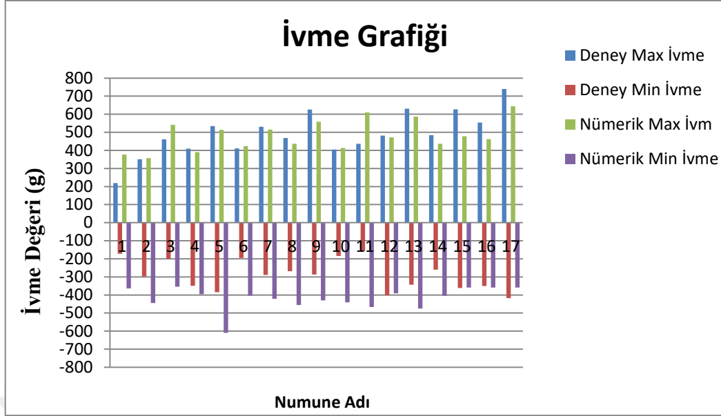
Şekil 4.85. Deney ile sayısal analiz sonuçlarının ivme grafiği
