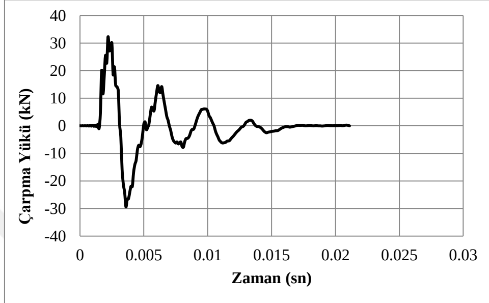
Şekil 4.18. C50sDi deney numunesine ait darbe yükü/zaman grafiği
