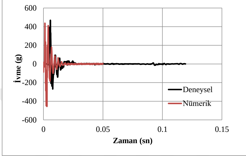
Şekil 4.35. C100sDi ivme-zaman grafik değerleri
