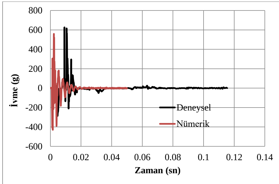
Şekil 4.40. C100dDi ivme-zaman grafik değerleri
