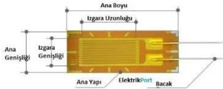
Şekil 3.10. Strain-gauge yapısı
