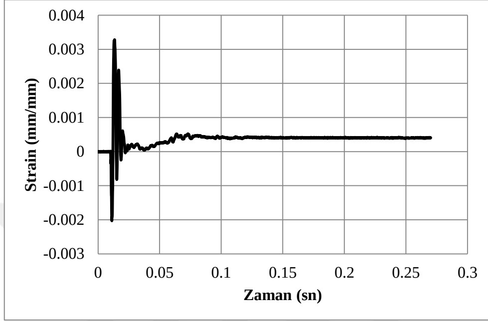
Şekil 4.44. C100dDi deney numunesine ait birim deformasyon-zaman grafiği
