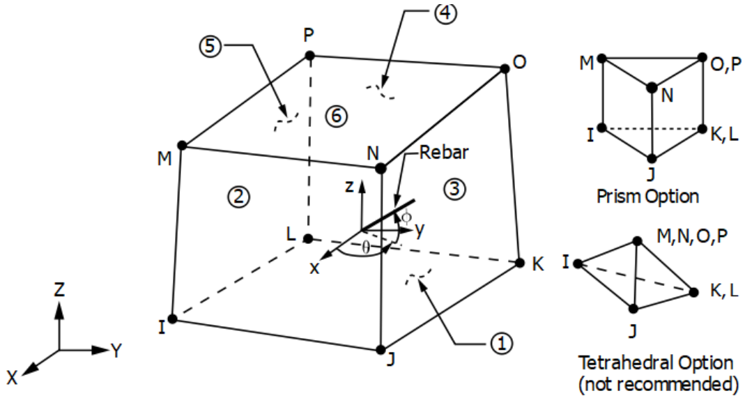
Şekil 3.32. Tetrahedron 10 noktalı şekil elemanı
