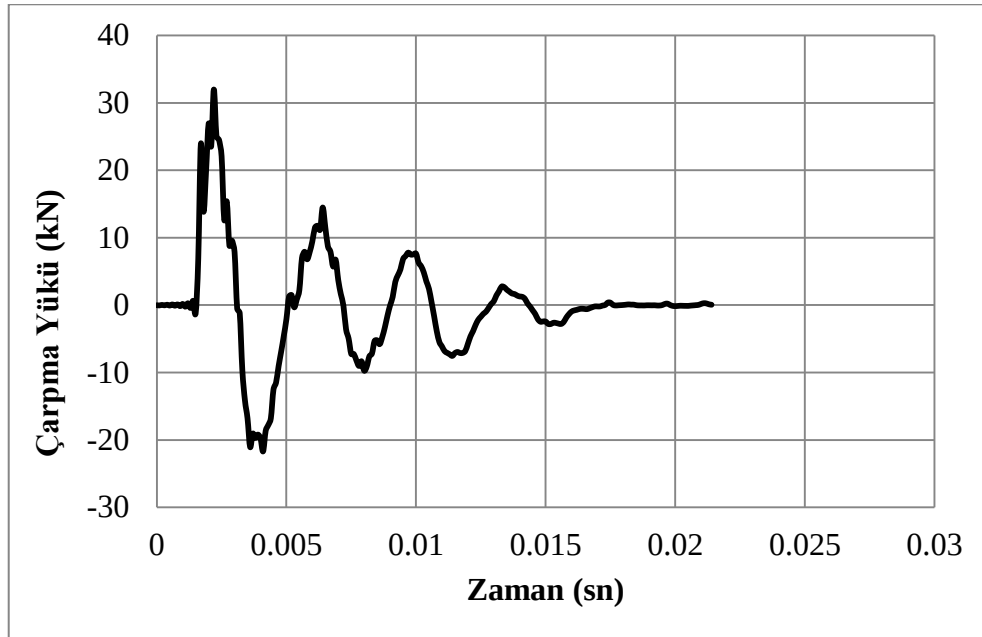
Şekil 4.63. C50dDi-A deney numunesine ait darbe yükü/zaman grafiği
