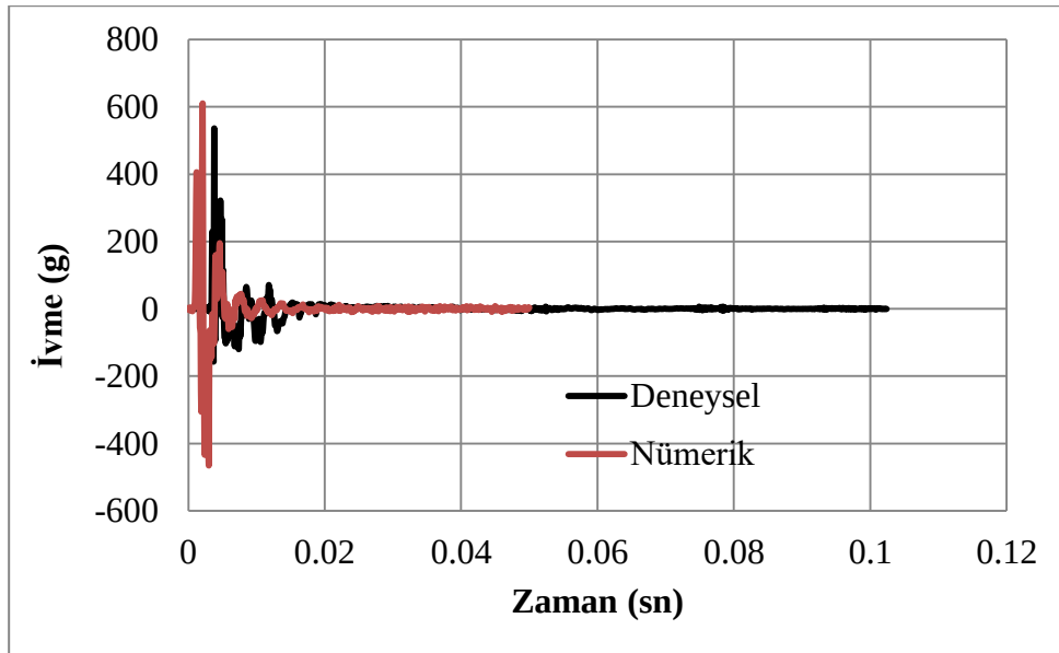
Şekil 4.50. C50dOr-A ivme-zaman grafik değerleri
