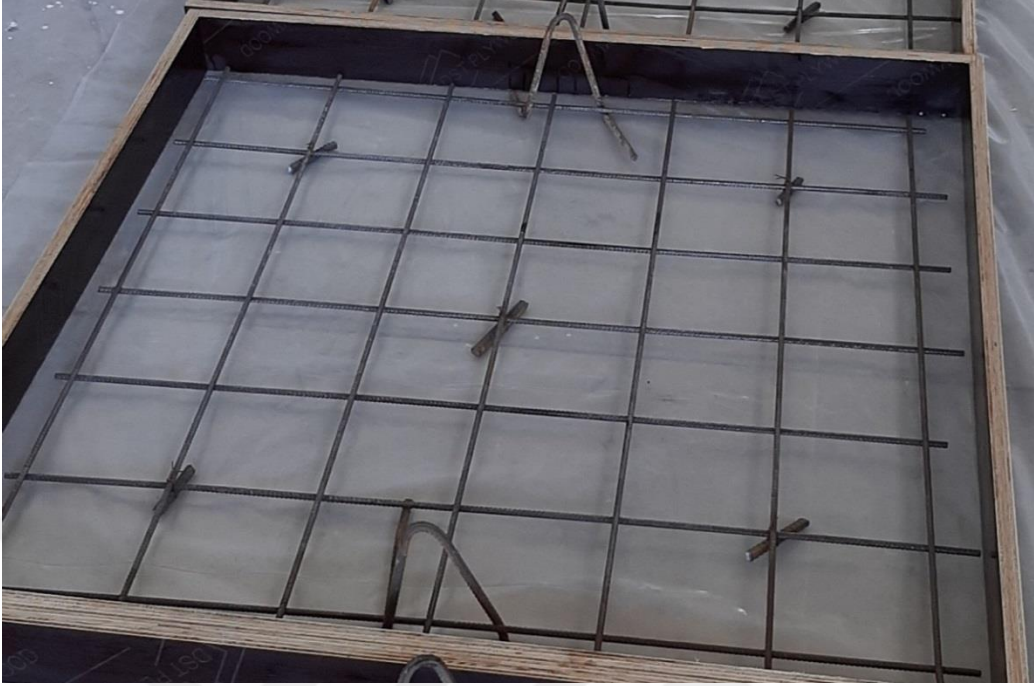
Şekil 3.17. Donatı çeliği
