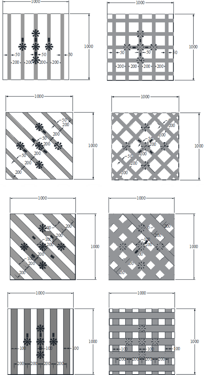
Şekil 3.25. 50 mm ve 100 mm genişliğinde TRM şeritlerin ankraj yerleri
