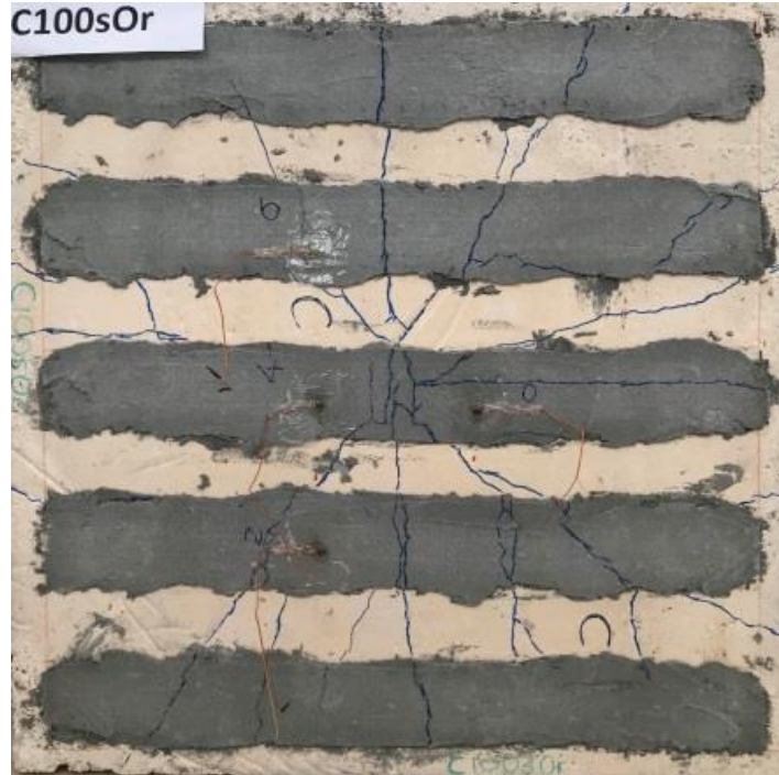
Şekil 4.27. C100sOr numunesinin deney sonrası çatlak dağılımı
