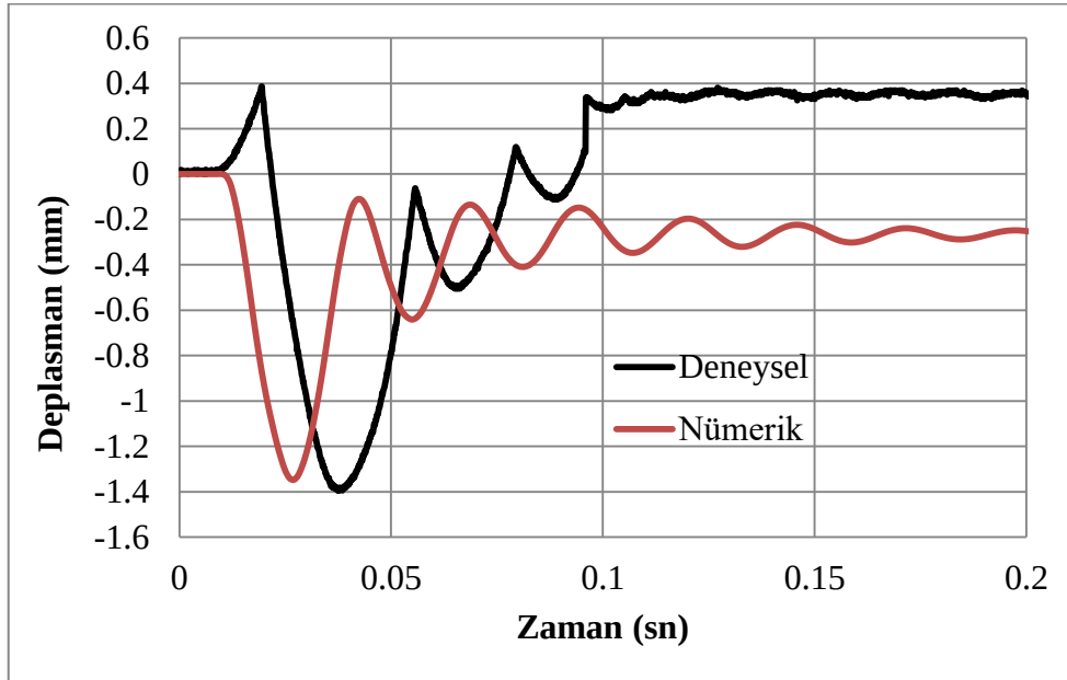
Şekil 4.66. C100sOr-A yer değiştirme-zaman grafik değerleri
