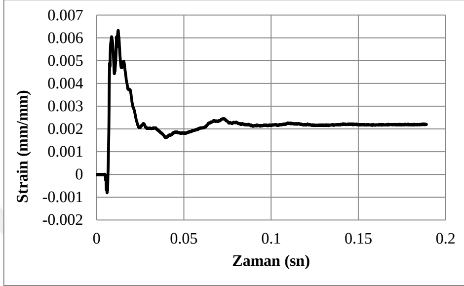
Şekil 4.64. C50dDi-A deney numunesine ait birim deformasyon-zaman grafiği
