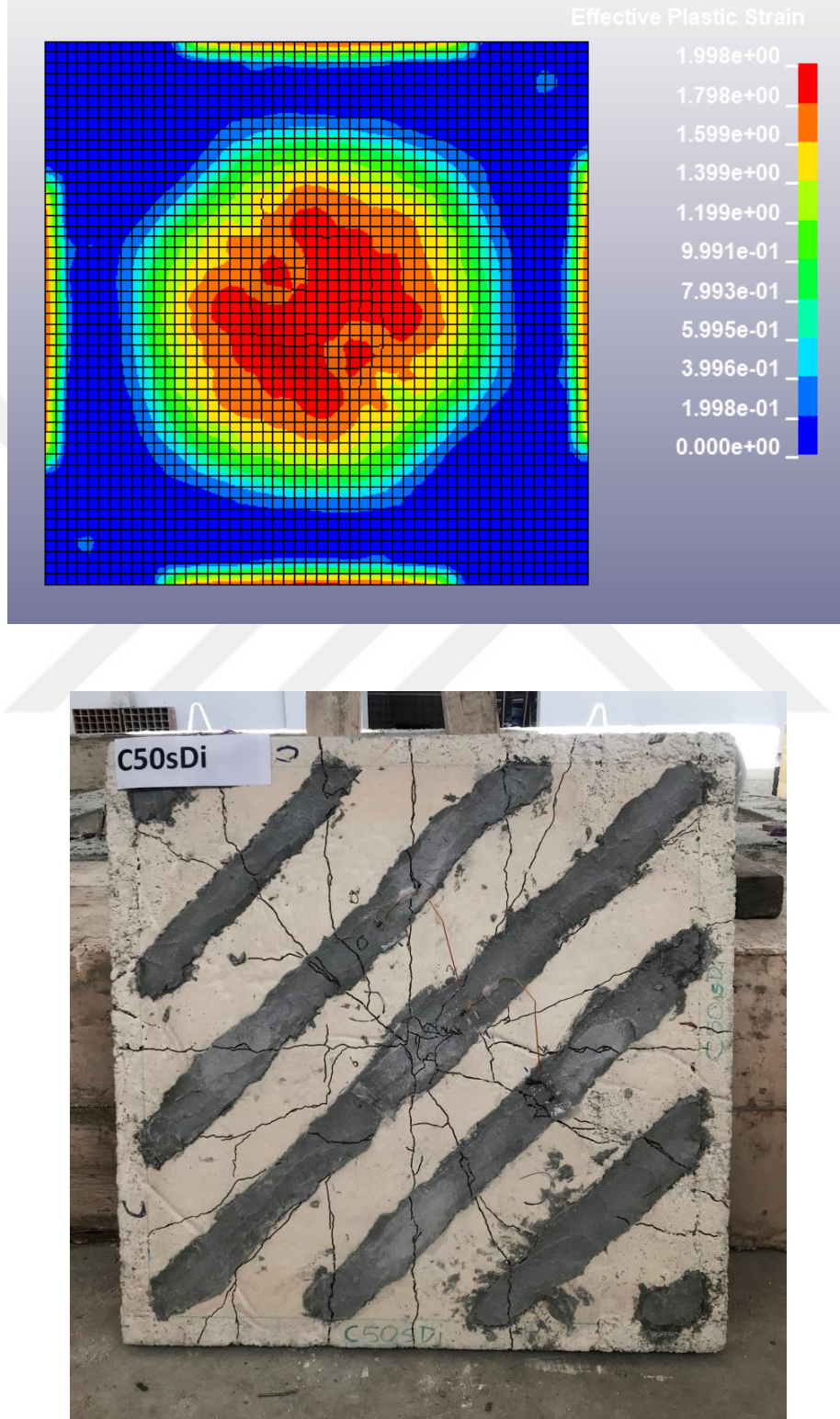
Şekil 4.17. C50sDi numunesinin deney sonrası çatlak dağılımı
