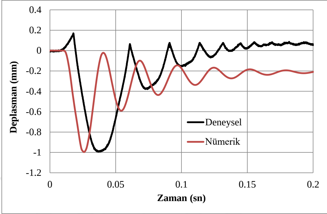
Şekil 4.41. C100dDi yer değiştirme-zaman grafik değerleri
