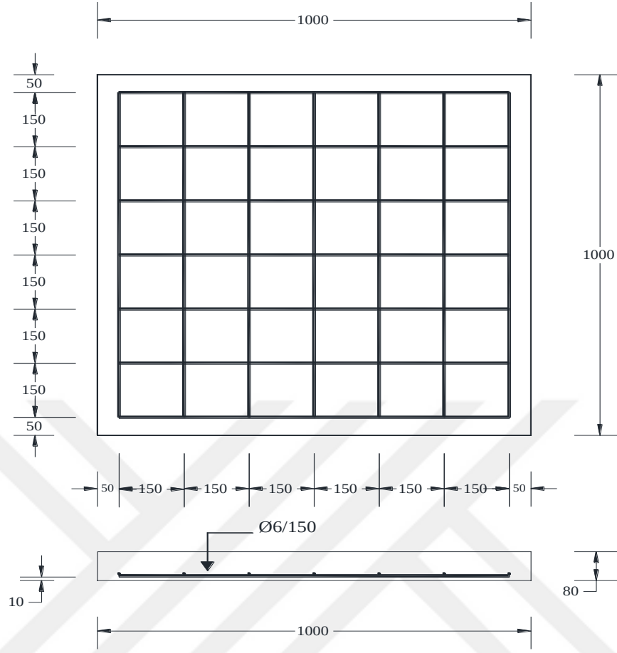
Şekil 3.21. Betonarme döşemenin detayları
