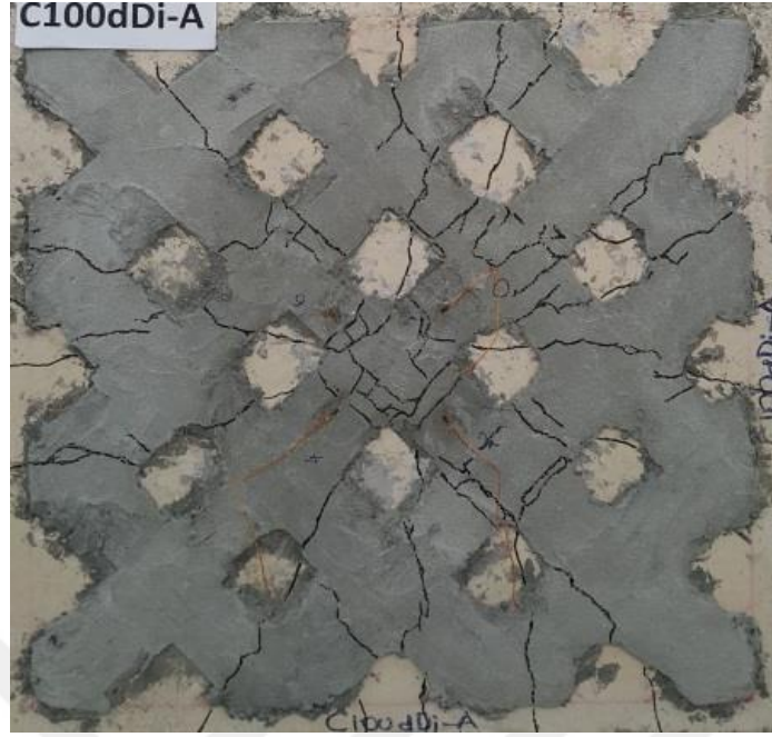
Şekil 4.82. C100dDi-A numunesinin deney sonrası çatlak dağılımı
