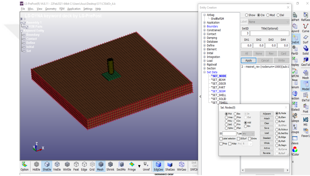
Şekil 3.46. Mesnet noktalara bir grup oluşturulması
