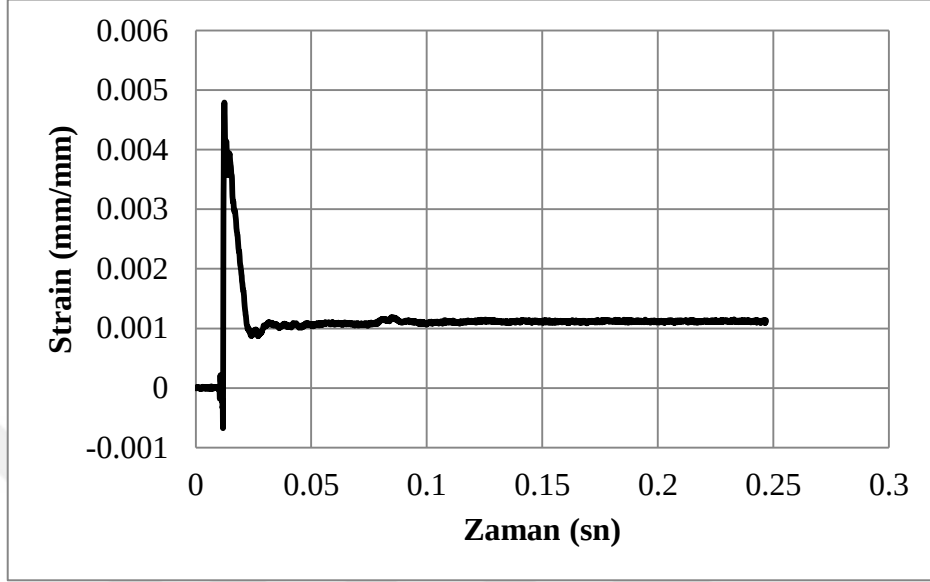
Şekil 4.34. C100dOr deney numunesine ait birim deformasyon-zaman grafiği
