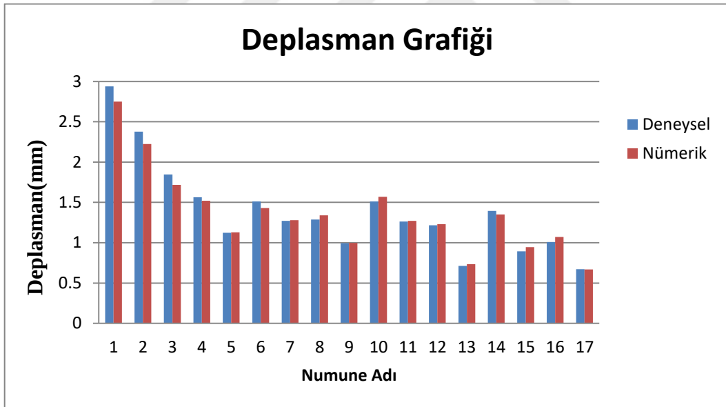
Şekil 4.86. Deney ile sayısal analiz sonuçlarının deplasman grafiği
