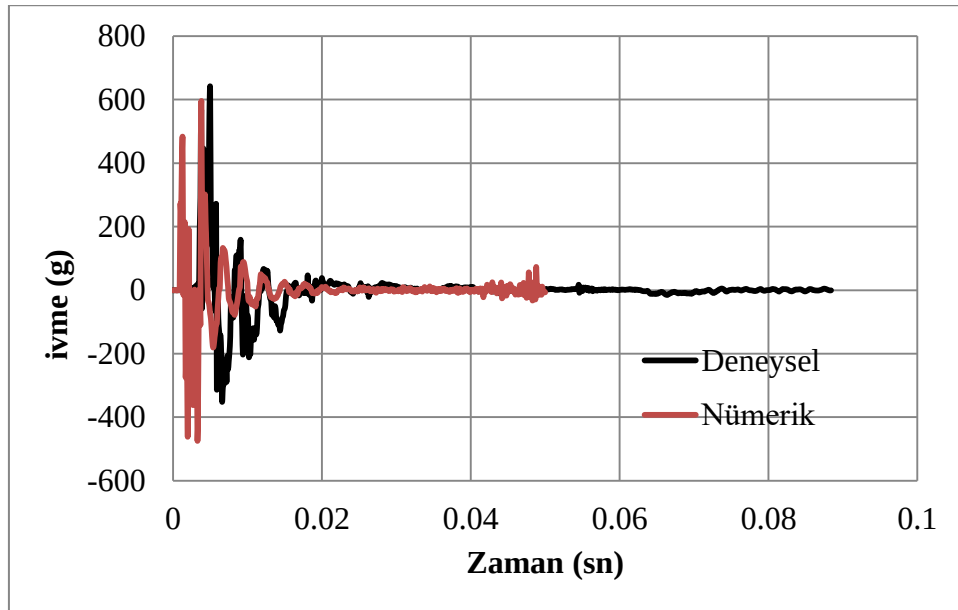
Şekil 4.60. C50dDi-A ivme-zaman grafik değerleri
