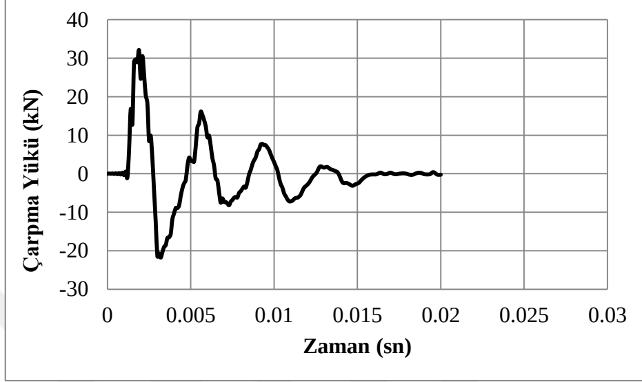
Şekil 4.78. C100sDi-A deney elemanına ait darbe yükü/zaman grafiği
