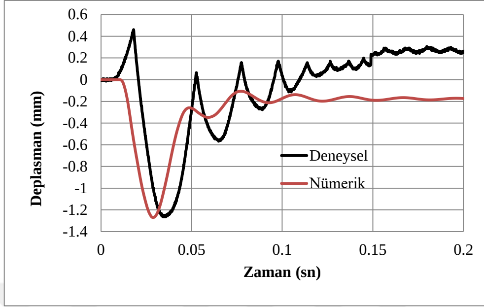
Şekil 4.51. C50dOr-A yer değiştirme-zaman grafik değerleri
