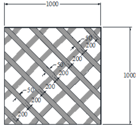
50 mm TRM Diyagonal Çift Yön
