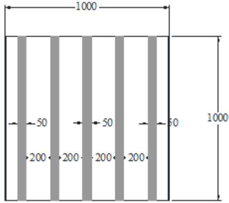
50 mm TRM Ortogonal Tek Yön
