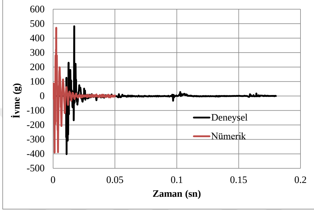
Şekil 4.55. C50sDi-A ivme-zaman grafik değerleri
