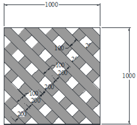
100 TRM Diyagonal Çift Yön
