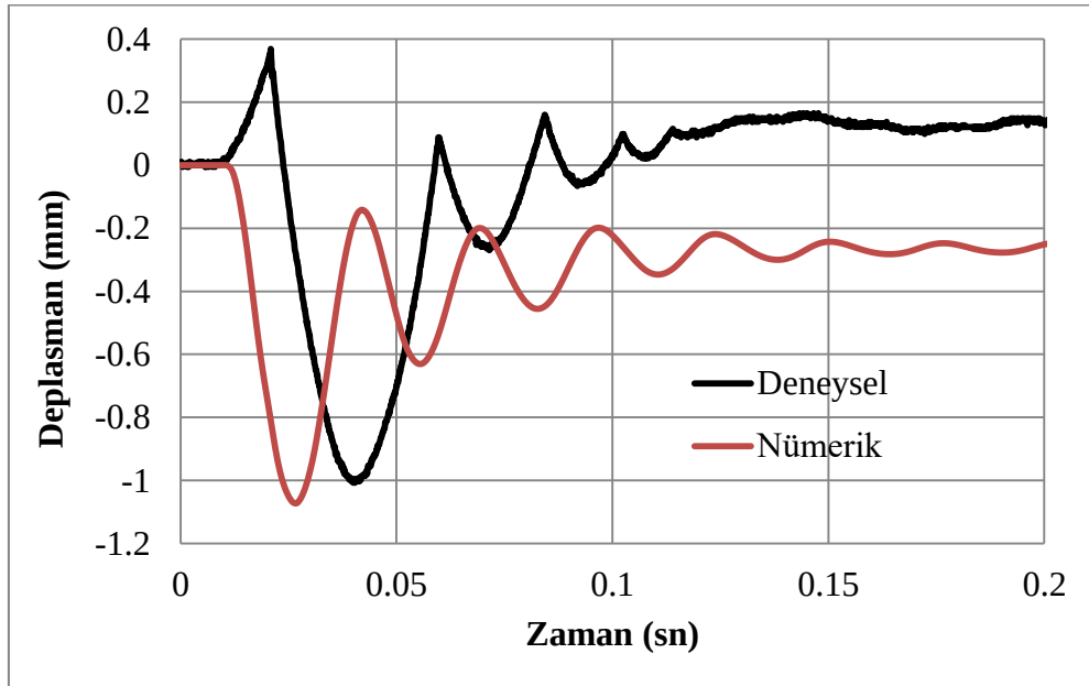
Şekil 4.76. C100sDi-A yer değiştirme-zaman grafik değerleri
