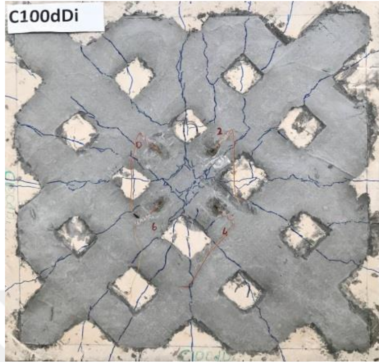
Şekil 4.42. C100dDi numunesinin deney sonrası çatlak dağılımı
