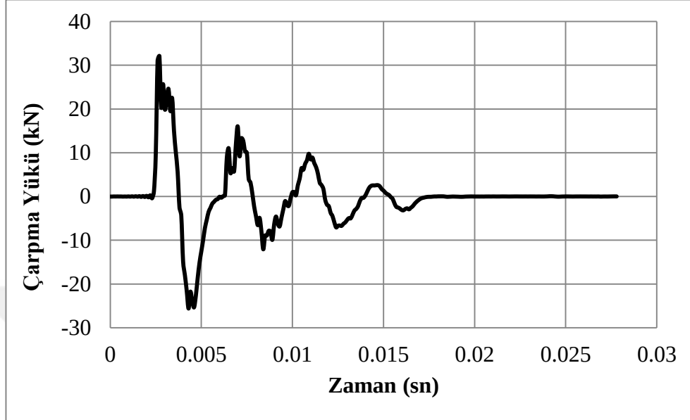
Şekil 4.58. C50sDi-A deney numunesine ait darbe yükü/zaman grafiği
