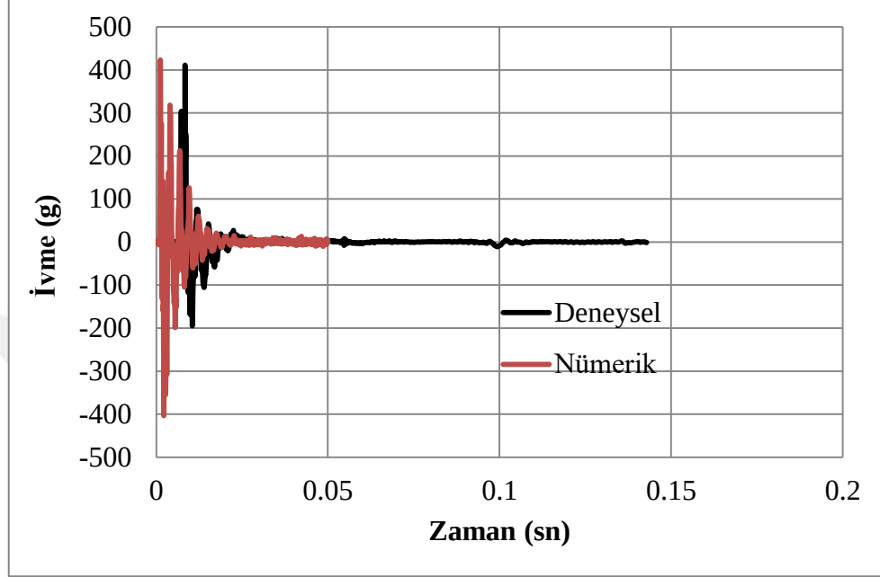
Şekil 4.25. C100sOr ivme-zaman grafik değerleri
