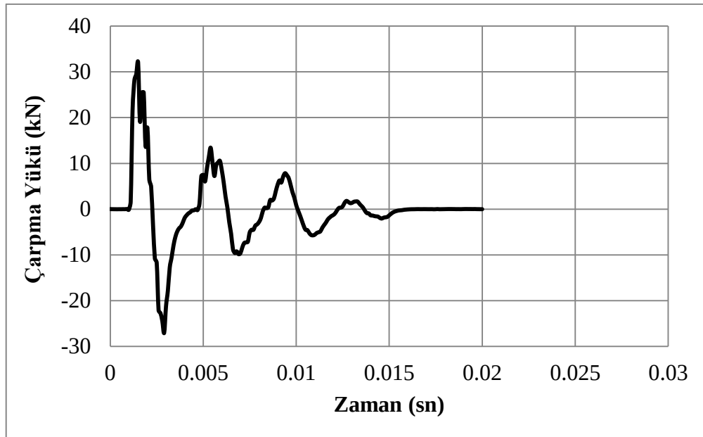
Şekil 4.23. C50dDi deney numunesine ait darbe yükü/zaman grafiği
