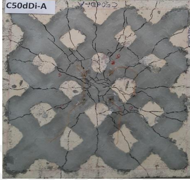
Şekil 4.62. C50dDi-A numunesinin deney sonrası çatlak dağılımı
