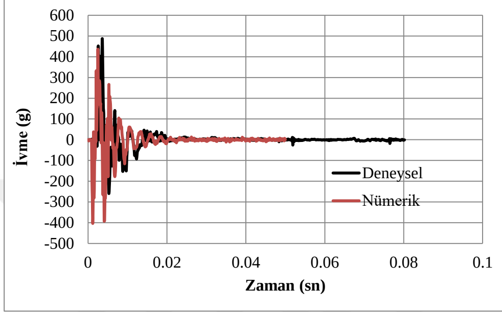
Şekil 4.65. C100sOr-A ivme-zaman grafik değerleri
