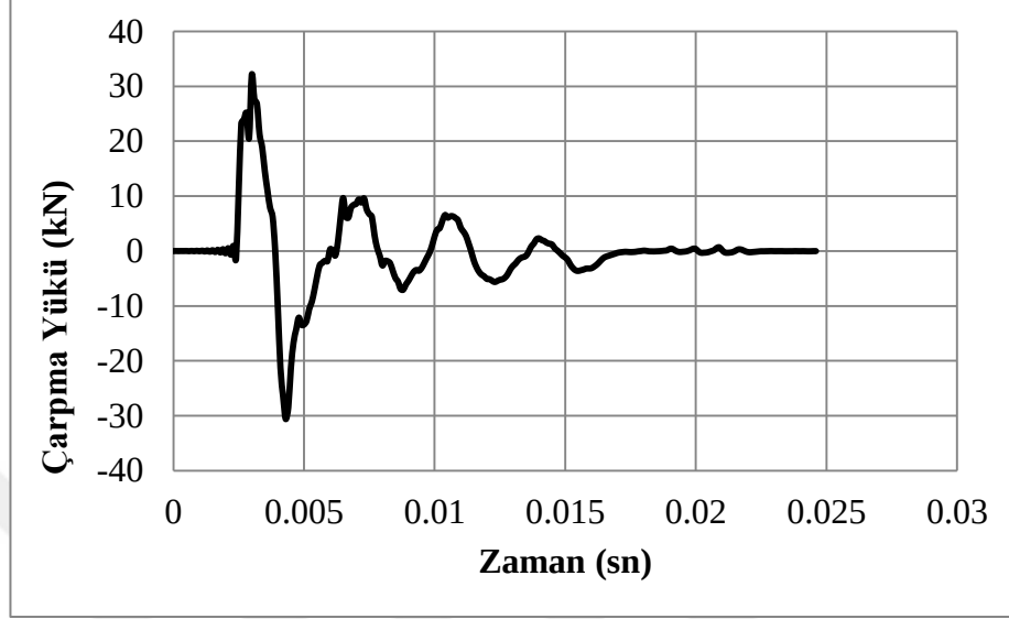
Şekil 4.8. C50sOr deney numunelerine ait darbe yükü/zaman grafiği
