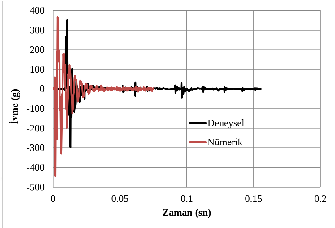
Şekil 4.5. C50sOr ivme-zaman grafik değerleri
