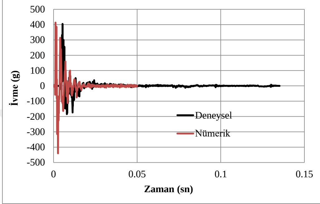
Şekil 4.45. C50sOr-A ivme-zaman grafik değerleri
