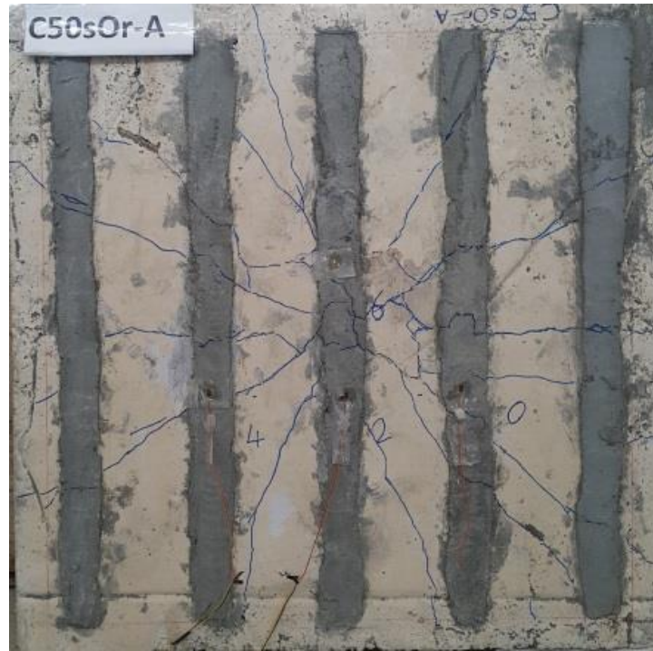
Şekil 4.47. C50sOr-A numunesinin deney sonrası çatlak dağılımı
