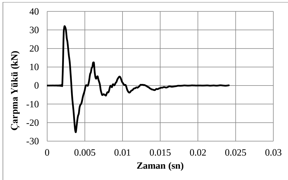
Şekil 4.4. Referans deney numunelerine ait darbe yükü/zaman grafiği
