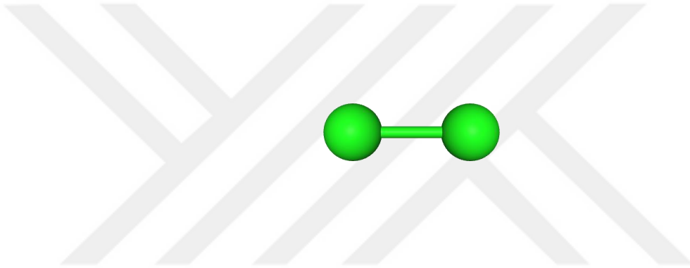
Şekil 1. Klor Gazının ( \text{Cl}_2 ) 3 Boyutlu Kimyasal Yapı Modeli
