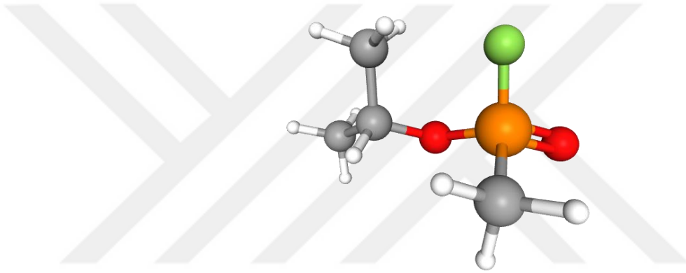
Şekil 9. Sarin Molekülünün ( C_4H_{10}FO_2P ) 3 Boyutlu Kimyasal Yapı Modeli
