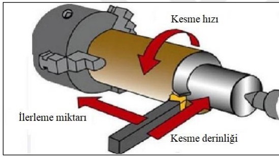
Şekil 3.9. Torna tezgahında kesme hızı, ilerleme miktarı ve kesme derinliği yönleri (Kaya, 2019)
