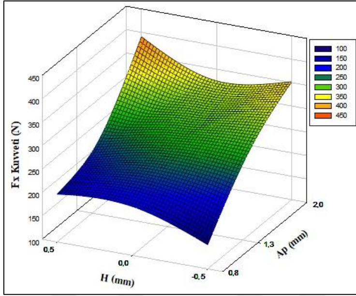
Şekil 9.15. Pozitif takımda F_x için H - A_p etkisi
