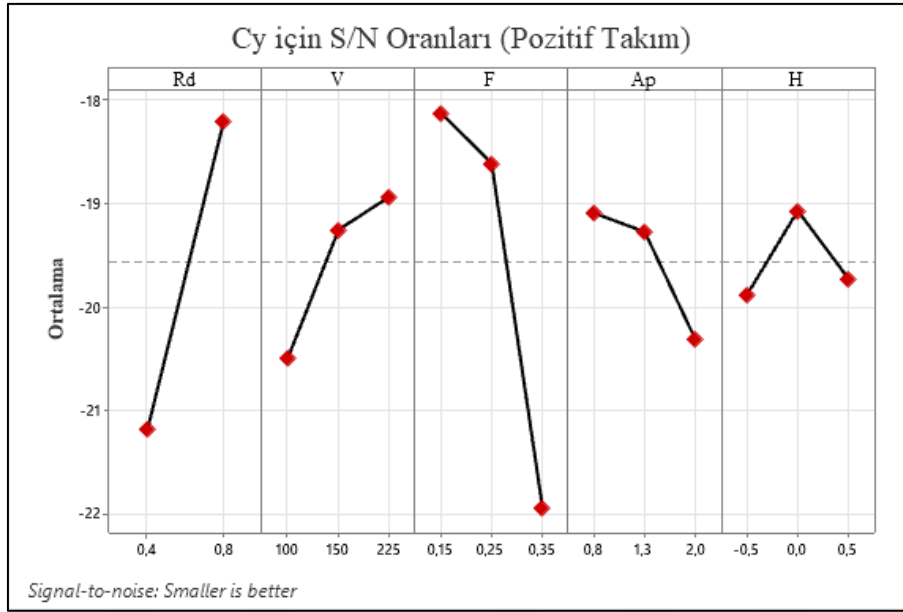
Şekil 9.47. Pozitif takımın faktörlerin Cy için S/N oranları
