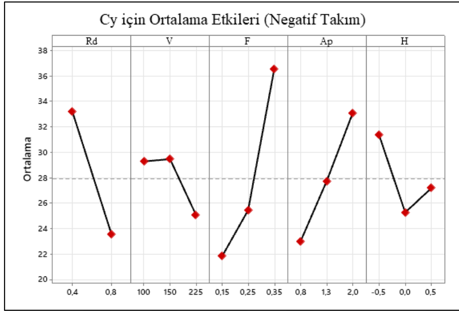
Şekil 9.41. Negatif takımın faktörlerin Cy için ortalama etkileri
