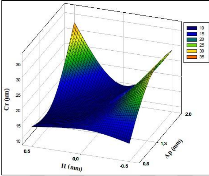
Şekil 9.34. Negatif takımında Cr için H-Ap etkileşimi
