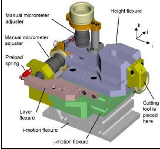
řekil 7.2. Mikron hassasiyette ayar saėlayan takım tutucu (Bono ve Hibbard, 2007)
