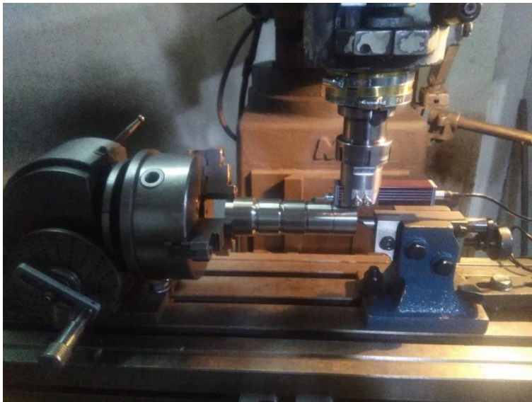
Resim 8.11. Yüzey pürüzlülük ölçümü
