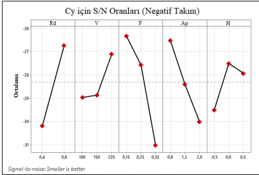
Şekil 9.42. Negatif takımda faktörlerin Cy için S/N oranları
