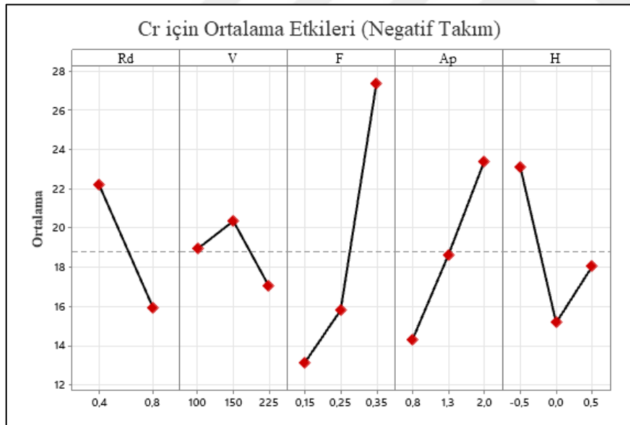
Şekil 9.31. Negatif takımda faktörlerin Cr için ortalama etkileri
