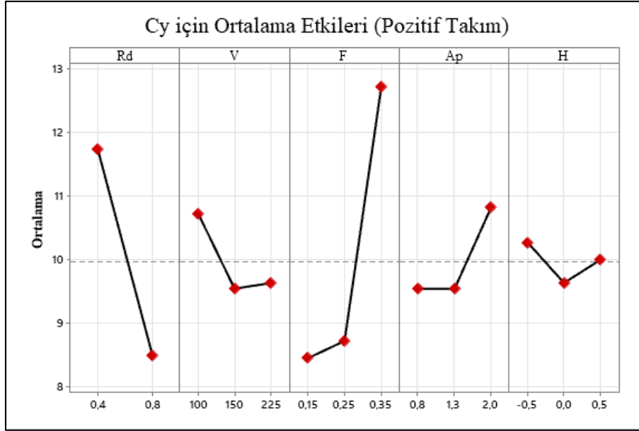
Şekil 9.46. Pozitif takımda faktörlerin Cy için ortalama etkileri
