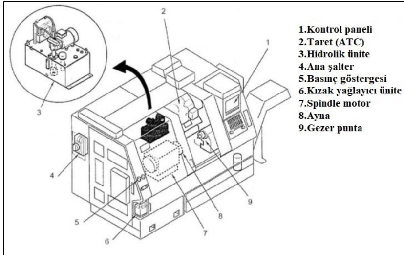
Şekil 3.5. CNC torna ve kısımları (Aksu, 2021)
