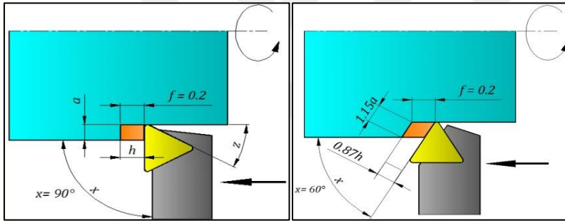
Şekil 3.13. Yanaşma açısına bağlı talaş kesiti (Yaldız, 2010)
