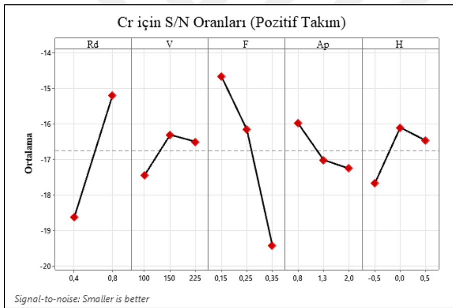
Şekil 9.37. Pozitif takımda faktörlerin Cr için S/N oranları
