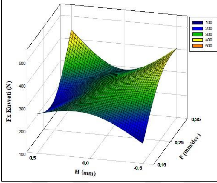
Şekil 9.4. Negatif takımında F_x için H - F etkisi
