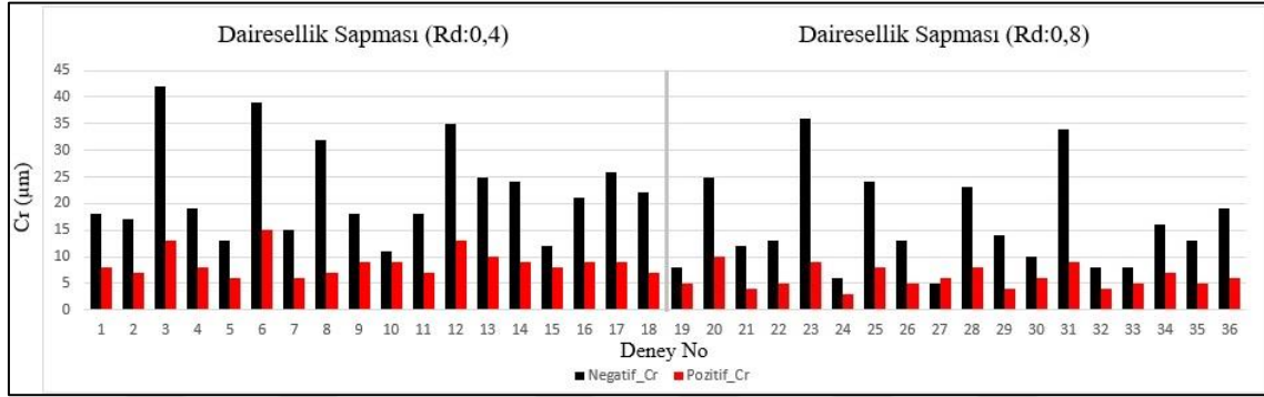
Şekil 9.59. Kesici takıma bağlı dairesellik sapma değerleri (Cr)
