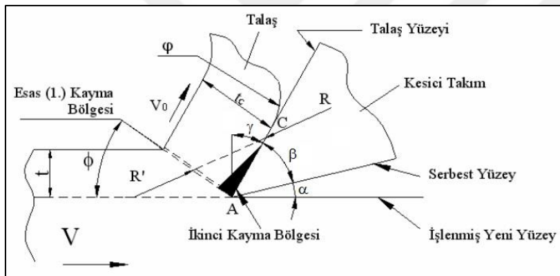
Şekil 3.10. Kesici takım açıları (Şahin, 2000)
