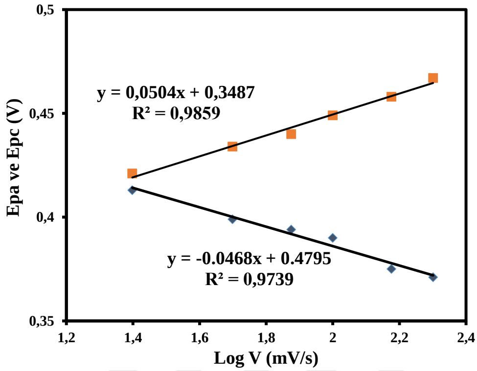
Şekil 7.21. 0,025, 0,05, 0,075, 0,1 0,150 ve 0,2 Vs-1 tarama hızlarında 30 \mu M rutin'e ait dönüşümlü voltamogramlar (Epa ve Epc)-log v grafiği
