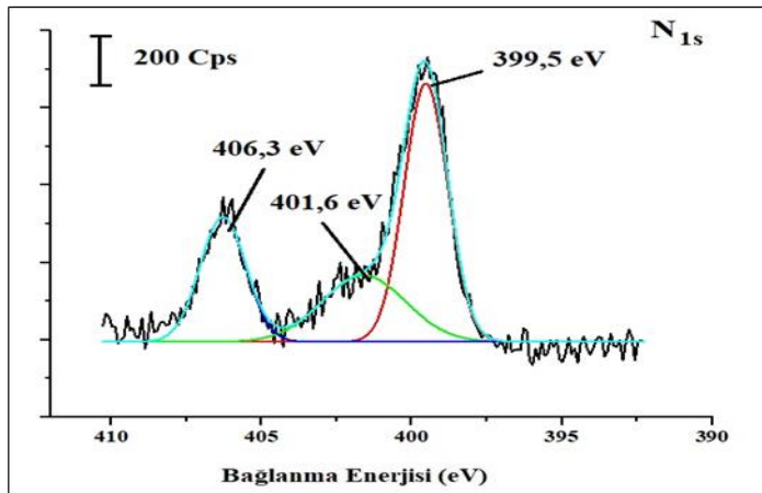
Şekil 7.12. 8-NQ/KGE yüzeyleri için N1s kısmi tarama XPS spektrumu
