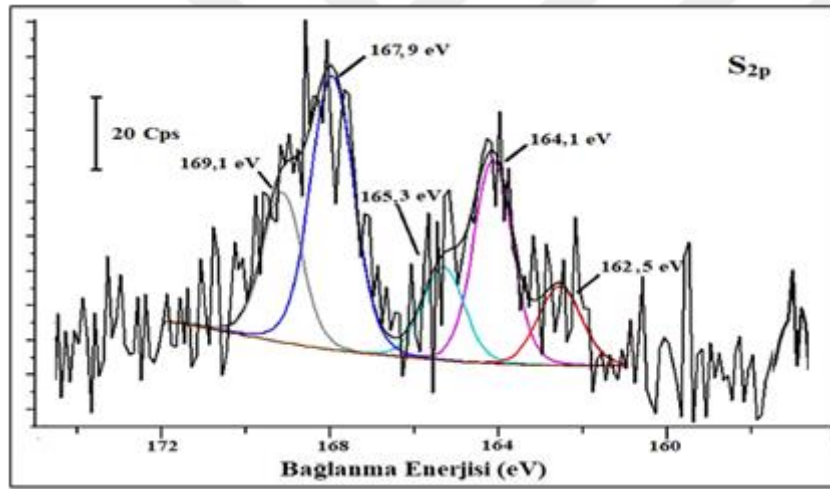
Şekil 7.9. 2-MBT/KGE yüzeyleri için S_{2p} kısmi tarama XPS spektrumu
