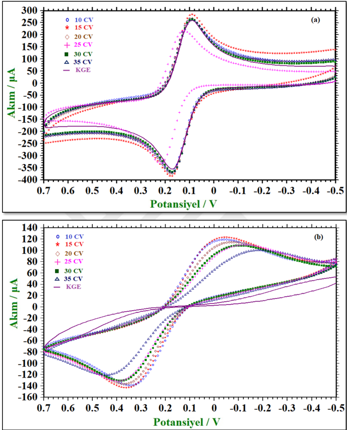
Şekil 7.4. 8-NQ/KGE ve KGE yüzeylerin, a ) 1,0 \times 10^{-3} M Ferrosenin 0,1 M TBATFB içeren asetonitrildeki çözeltisinde b) 1,0 \times 10^{-3} M Ferrisiyanürün 0,1 M KCl çözeltisinde elde edilen dönüşümlü voltamogramları
