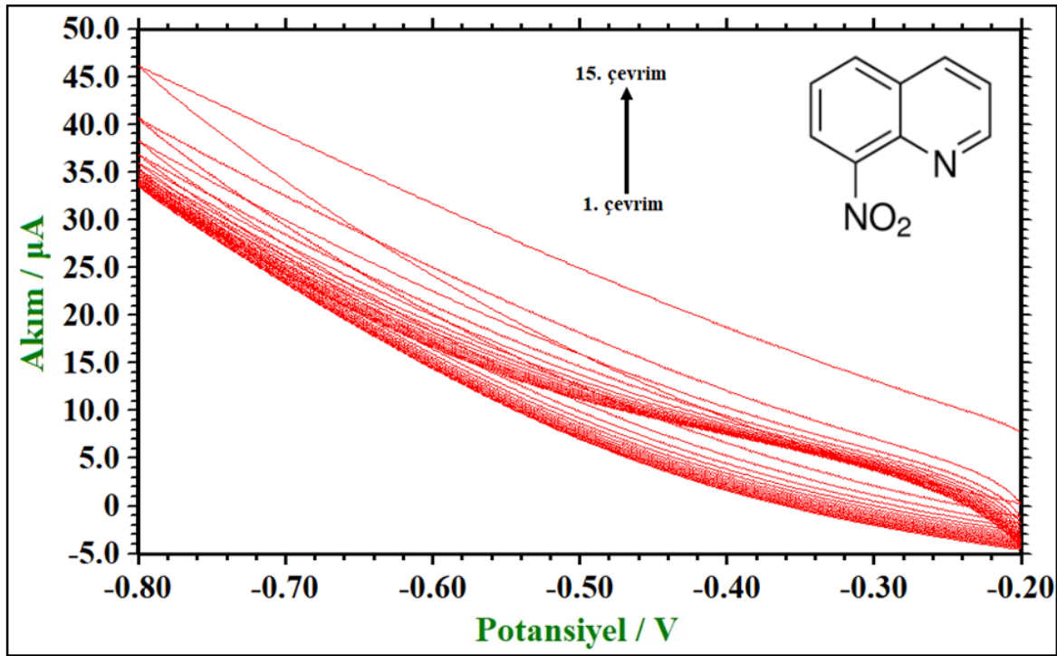
Şekil 7.2. 1,0 \times 10^{-3} M 8-NQ molekülünün içeren etanol ortamında KGE yüzeyin modifikasyon voltamogramı
