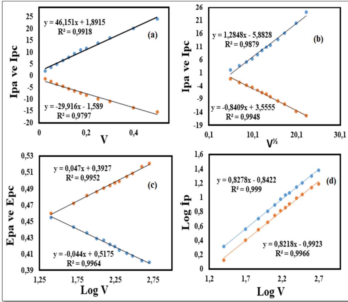
Şekil 7.24. 0,025, 0,05, 0,075, 0,1, 0,125, 0,150, 0,175, 0,2, 0,250, 0,300, 0,400, 0,500 \text{Vs}^{-1} tarama hızlarında : (a). I_{pa} ve I_{pc} vs. v 'nin grafiği. (b). I_{pa} ve I_{pc} vs. v^{1/2} 'nin grafiği; (c). E_{pa} ve E_{pc} vs \text{Log } v grafiği ve (d). \text{Log } I_{pa} ve \text{Log } I_{pc} vs \text{Log } v grafikleri.
