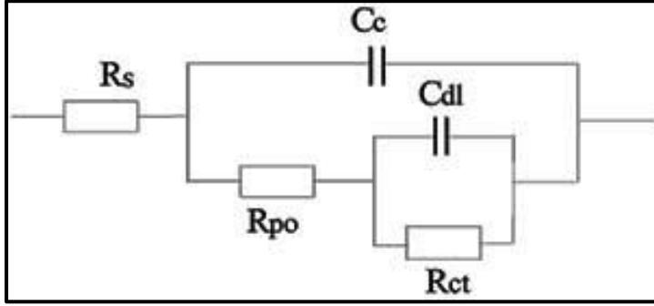
Şekil 3.23. Başarısız bir kaplama için eşdeğer devre [12]
