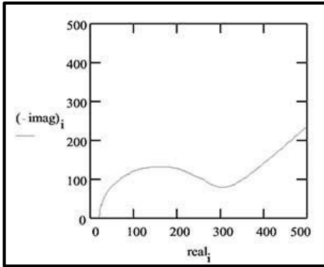
Şekil 3.21. Karışık kontrol devresi için Nyquist şeması [12].
