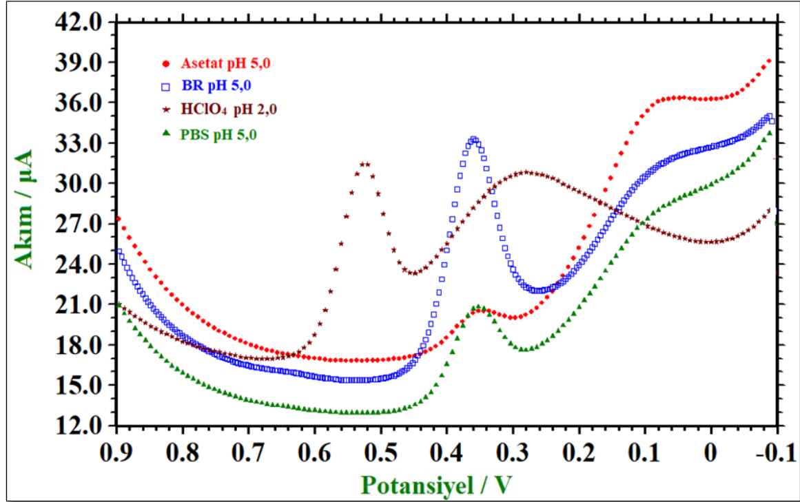
Şekil 7.25. 2-MBT/KGE ile farklı destek elektrolit ortamlarında 0,1 M pH 5 asetat, PBS, Briton-Robinson (BR) tamponları ve 0,1 M pH 2 perklorik asit 30 \mu\text{M} rutine ait DPV voltamogramları
