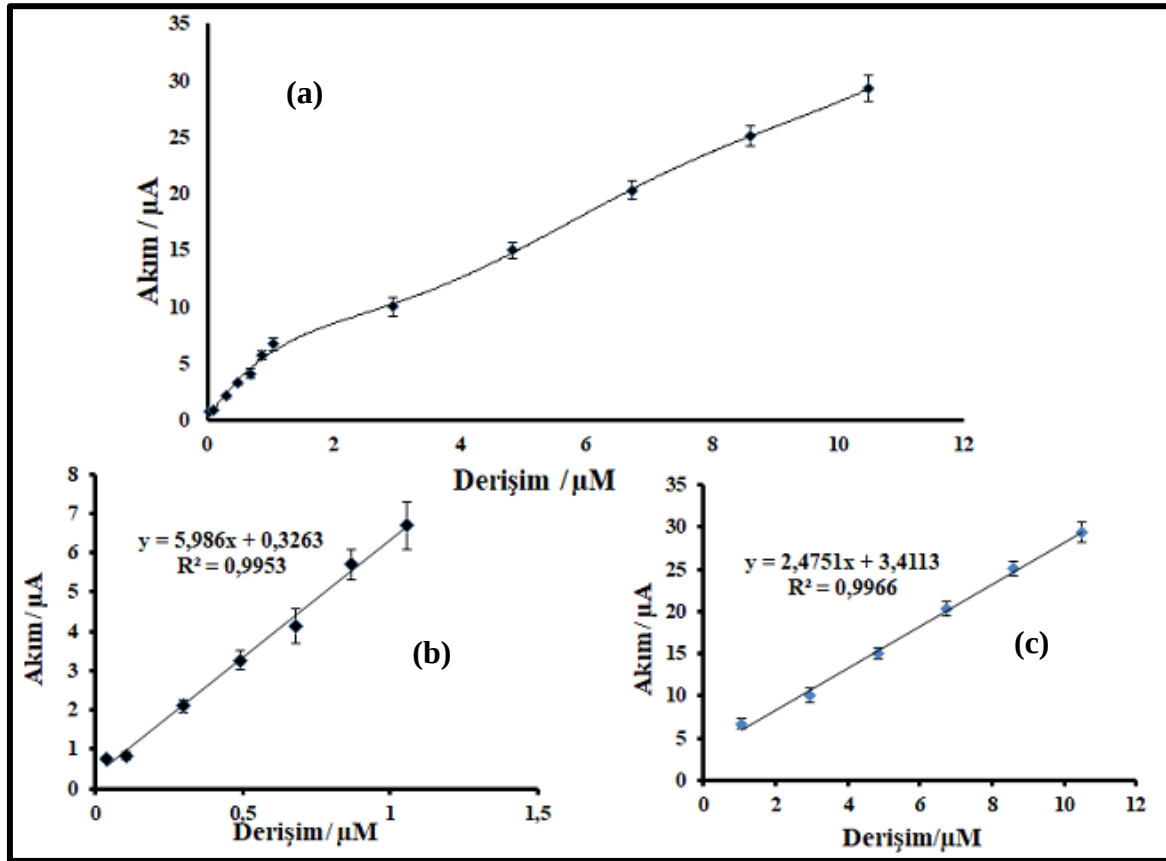
Şekil 7.32. 2-MBT/KGE elektrodu ile pH 4,5 BR ortamına standart rutin ilaveleriyle elde edilen a) kalibrasyon grafiği, b) 0,039-1,1 \mu\text{M} aralığında doğrusal çalışma aralık grafiği c) 1,1-10,5 \mu\text{M} aralığında doğrusal çalışma aralık grafiği.
