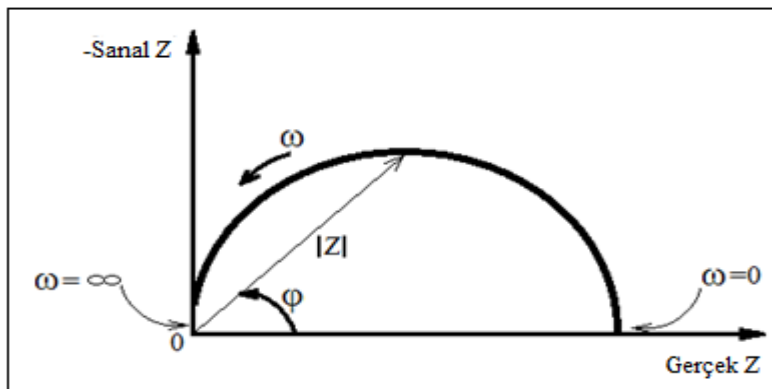
Şekil 3.8. İmpedans vektörlü Nyquist grafiği [12].
