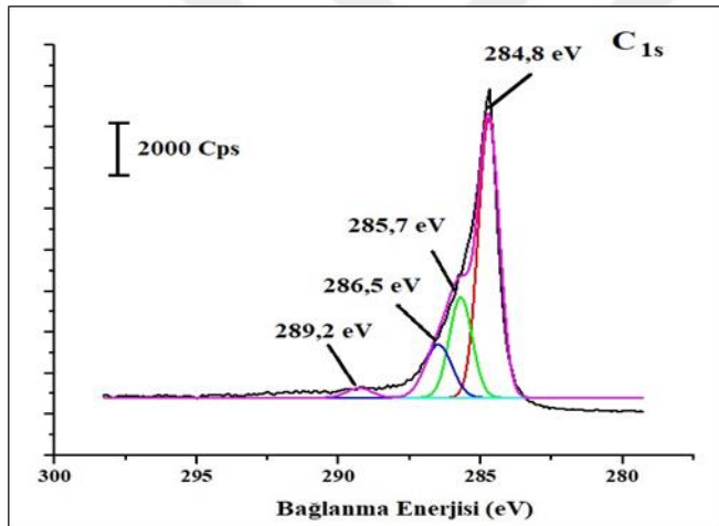
Şekil 7.11. 8-NQ/KGE yüzeyleri için C1s kısmi tarama XPS spektrumu
