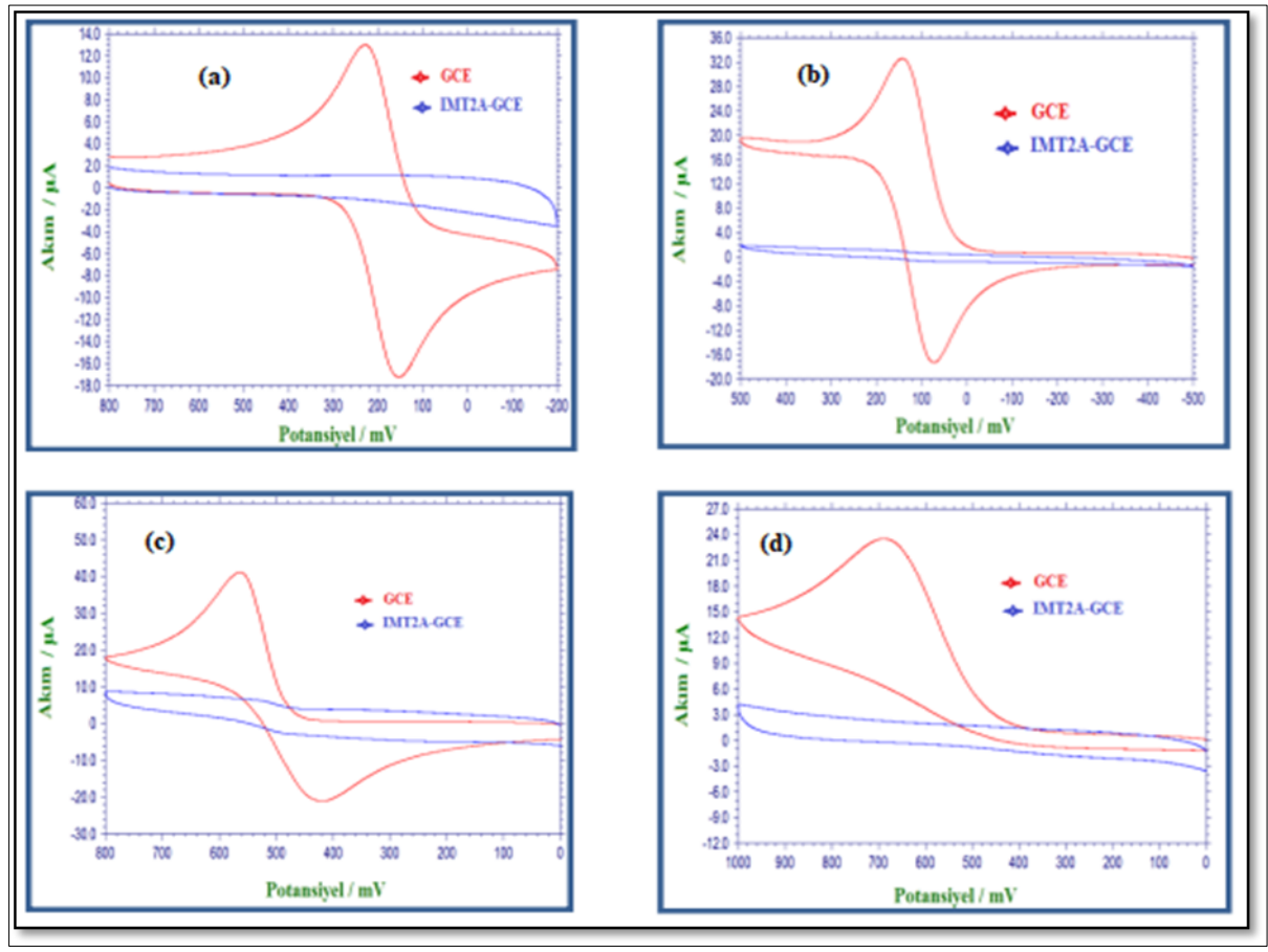
Şekil 3.4. GCE ve IMT2A-GCE yüzeylerinin a) 1,0 \times 10^{-3} M ferrisiyanürün, 0,1 M KCl çözeltisinde b) 1,0 \times 10^{-3} M ferrosenin, 0,1 M TBATFB içeren MeCN çözeltisinde c) 1,0 \times 10^{-3} M DA'nın, 0,1 M H_2SO_4 çözeltisinde d) 1,0 \times 10^{-3} M AA'nın, 0,1 M H_2SO_4 çözeltisinde CV voltamogramları [12].
