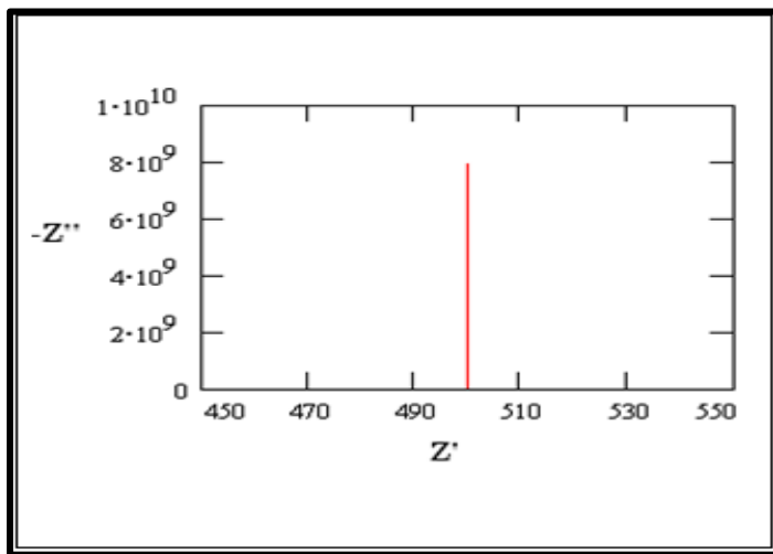
Şekil 3.13. Kaplama için tipik Nyquist grafiği [12].
