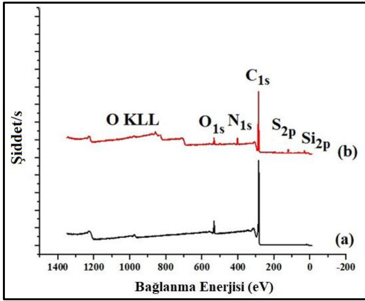
Şekil 7.6. (a) Yalın KGE ve (b) 2-MBT/KGE'nin XPS genel tarama spektrumu
