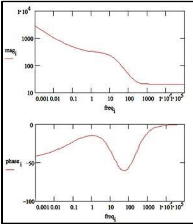
Şekil 3.22. Karma kontrol devresi için Bode grafiği [12].
