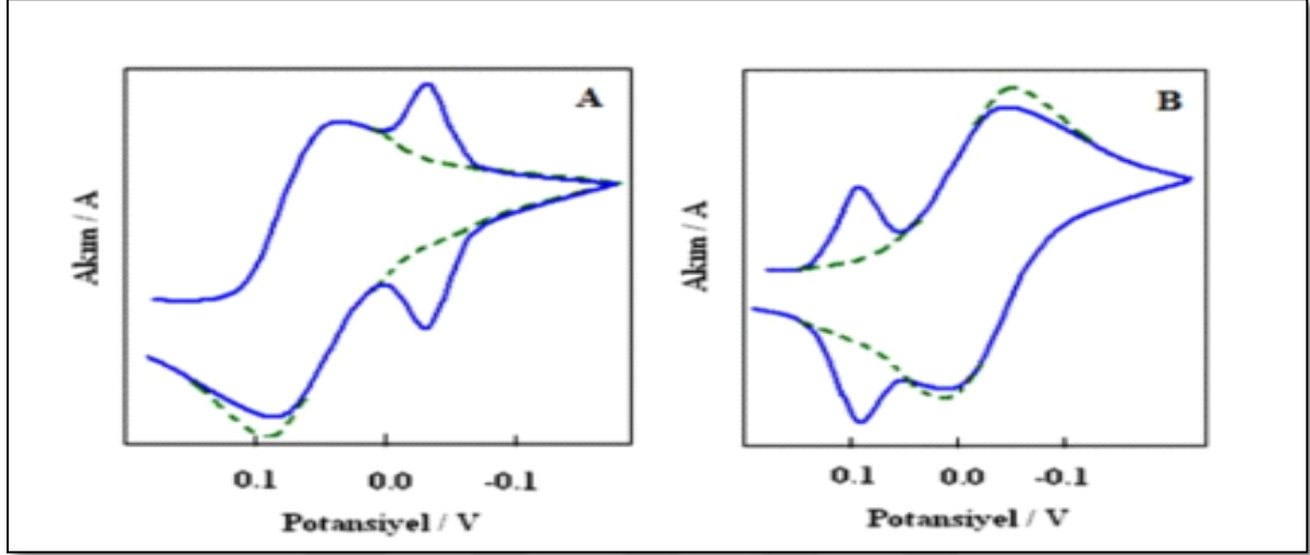
Şekil 2.6. Durgun elektrot yüzeyine adsorplanmış maddelerin voltamogramları, (A) reaktantın kuvvetli adsorpsiyonunda, (B) Ürünün kuvvetli adsorpsiyonunda gözlenen voltamogramlar [7].
