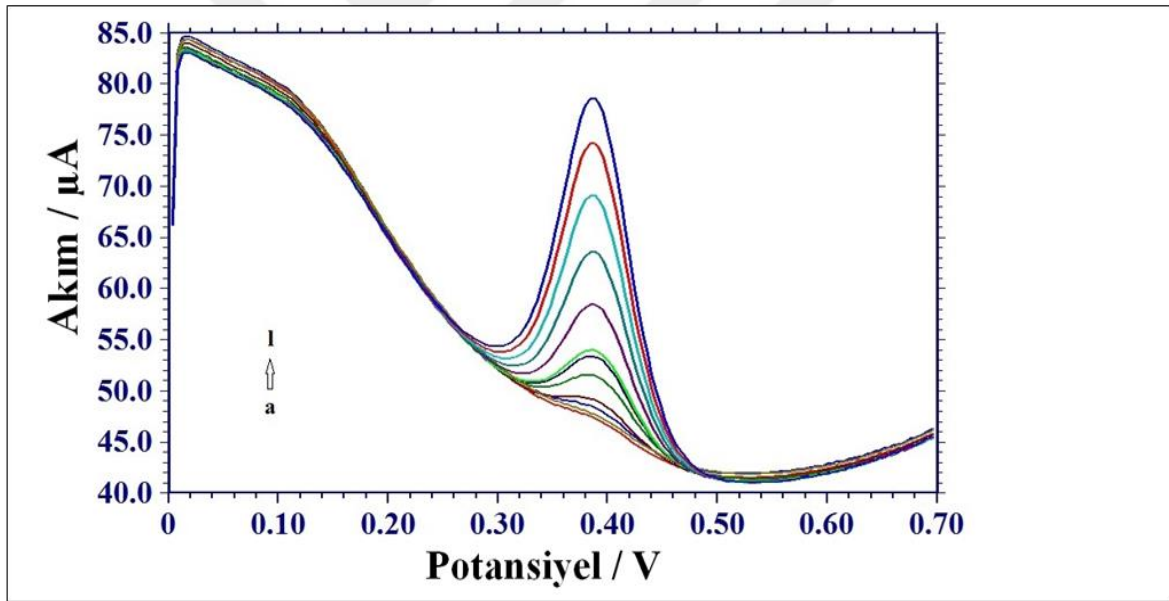
Şekil 7.31. 2-MBT/KGE elektrodu ile pH 4,5 BR ortamına standart rutin eklemeleriyle elde edilen DPV voltamogramları (tarama hızı 100mV/s) rutin derişimi ( \mu\text{M} ) 0,039, 0,107, 0,298, 0,490, 0,679, 0,869, 1,06, 2,96, 4,85, 6,73, 8,61 ve 10,05 (a \rightarrow i)
