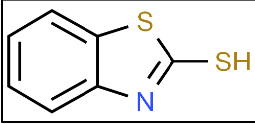
Şekil 6.1. 2-MBT molekül yapısı
