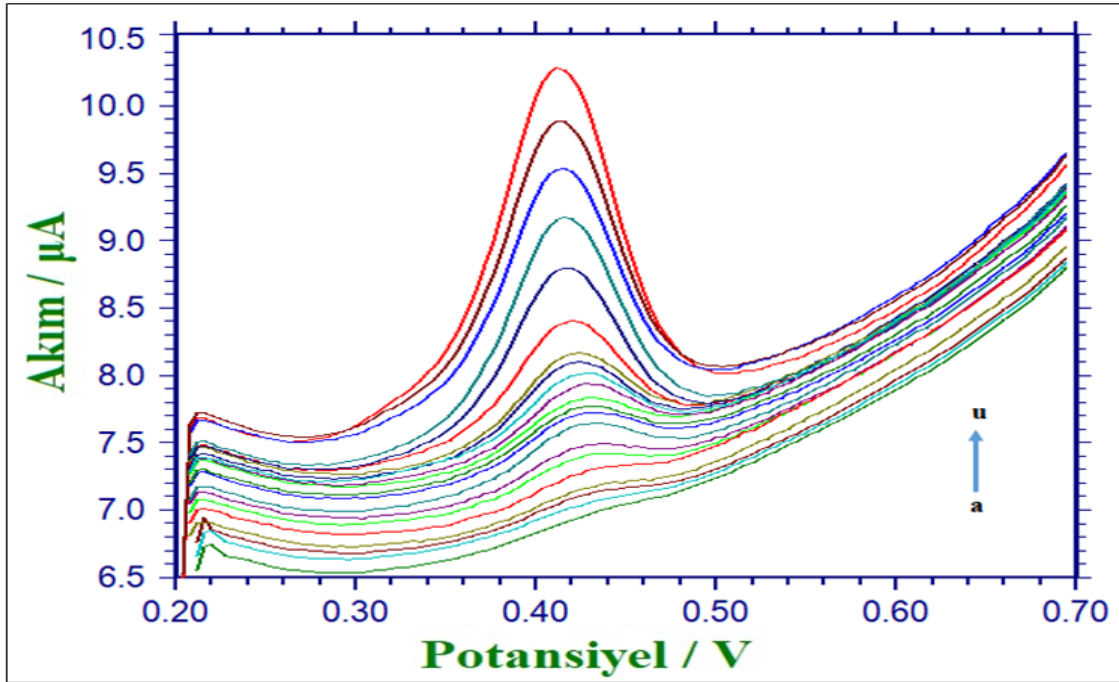
Şekil 7.33. 8-NQ/KGE elektrodu ile pH 3,0 BR ortamına standart Rutin eklemeleriyle elde edilen DPV voltamogramları (tarama hızı 100mV/s) Rutin derişimi ( \mu\text{M} ) 0,0155, 0,0301, 0,0592, 0,0882, 0,1068, 0,312, 0,4895, 0,5848, 0,6791, 0,7747, 0,8691, 0,9638, 1,058, 2,257, 4,105, 6,734, 8,612, 10,5, 14,03, 17,89, 19,73 (a \rightarrow u)
