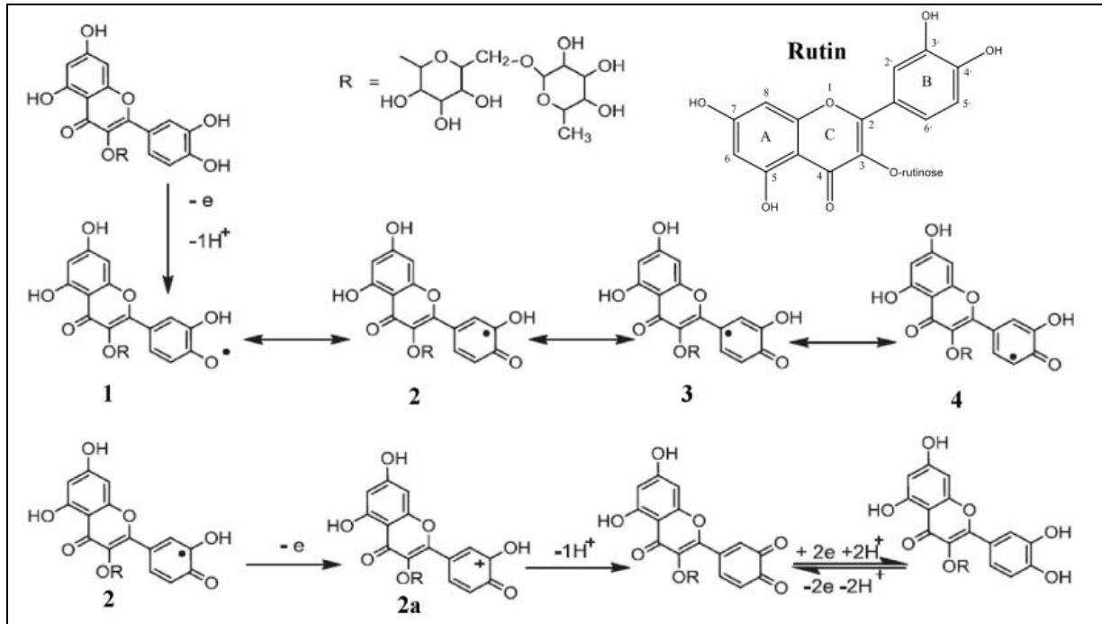
Şekil 7.22. 2-MBT/KGE'de rutin'in yükseltgenme mekanizması
