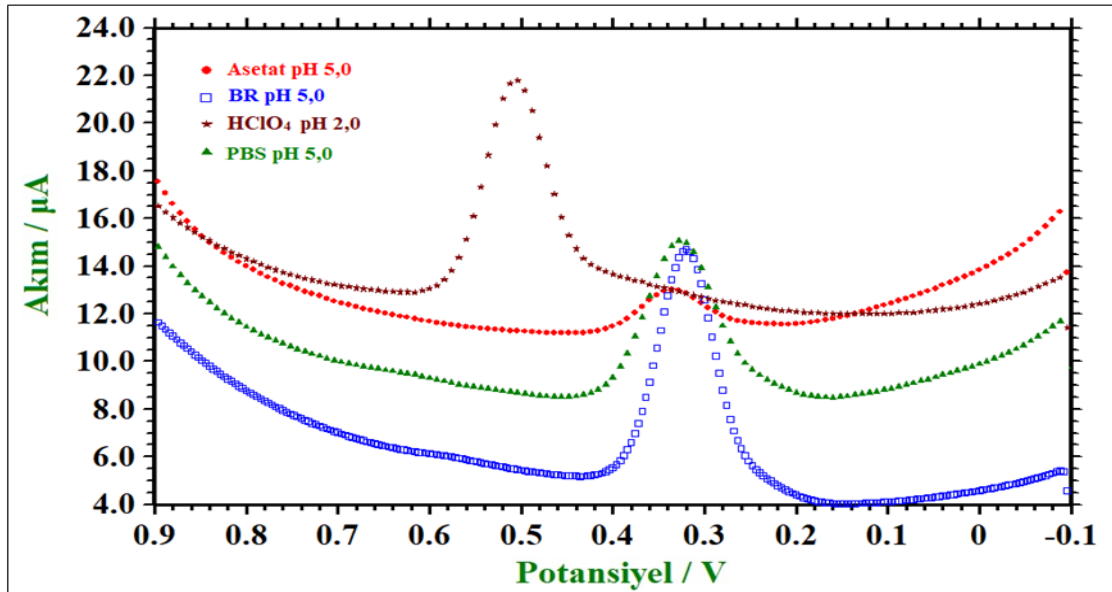
Şekil 7.28. 8-NQ/KGE ile farklı destek elektrolit ortamlarında 0,1 M pH 5 asetat , PBS, Briton-Robinson (BR) tamponları ve 0,1 M pH 2 perklorik asit 30 \mu\text{M} rutine ait DPV voltamogramları
