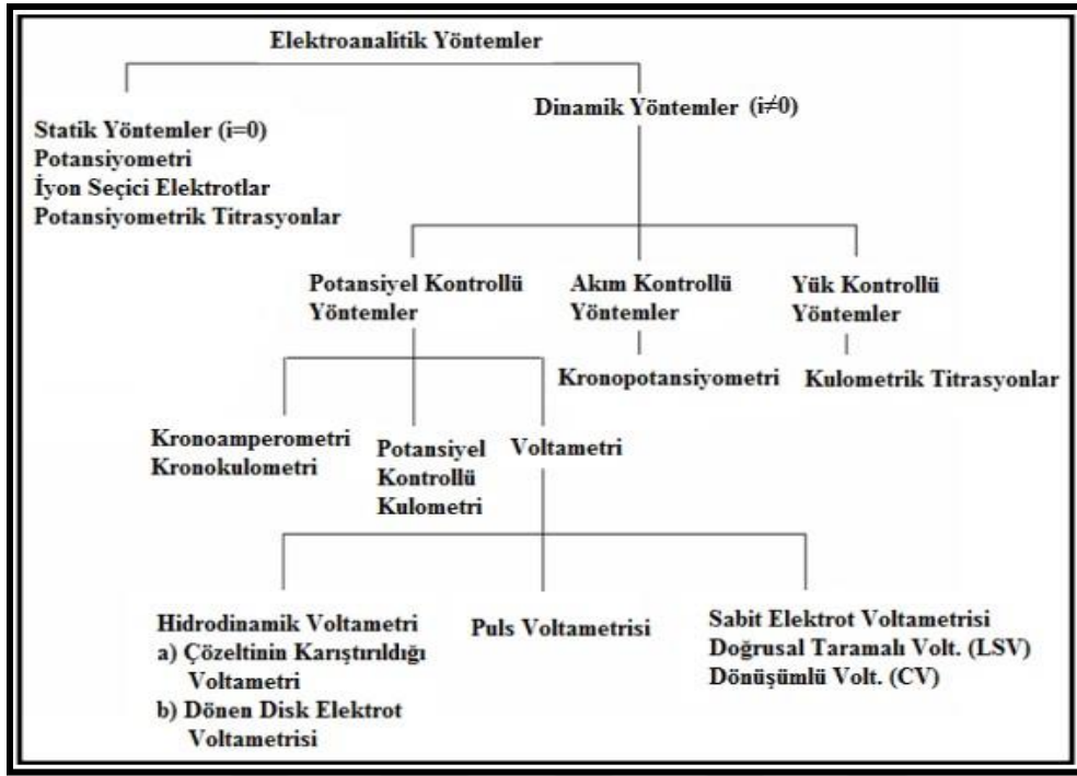
Şekil 2.1. Elektroanalitik yöntemlerin şematik olarak sınıflandırılması [11].
