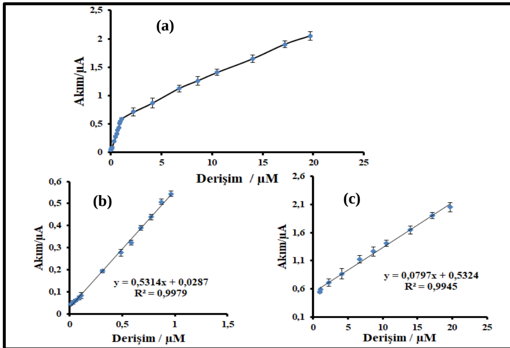
Şekil 7.34. 8-NQ/KGE elektrodu ile pH 3,0 BR ortamına standart Rutin ilaveleriyle elde edilen a) kalibrasyon grafiğı, b) 0,0155-0,96 \mu\text{M} aralığında doğrusal çalışma aralık grafiğı c) 0,96-19,73 \mu\text{M} aralığında doğrusal çalışma aralık grafiğı.
