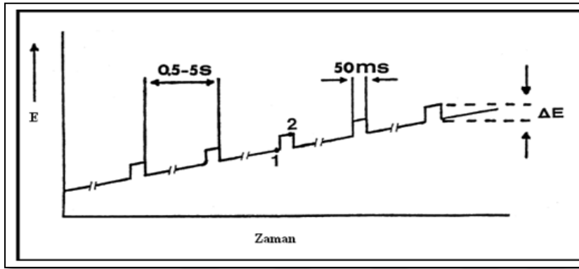
Şekil 2.8. DPV için uyarma sinyal grafiği [15].
