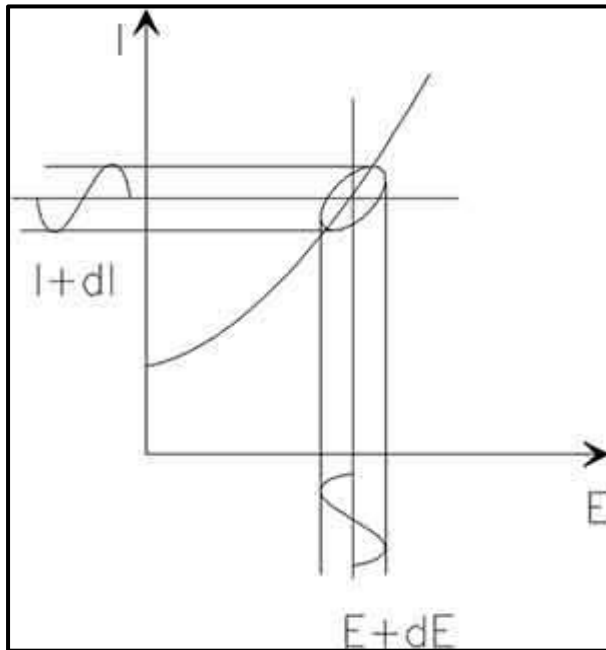
Şekil 3.7. Lissajous figürünün kökeni [12].
