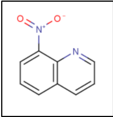
Şekil 6.2. 8-NQ molekül yapısı
