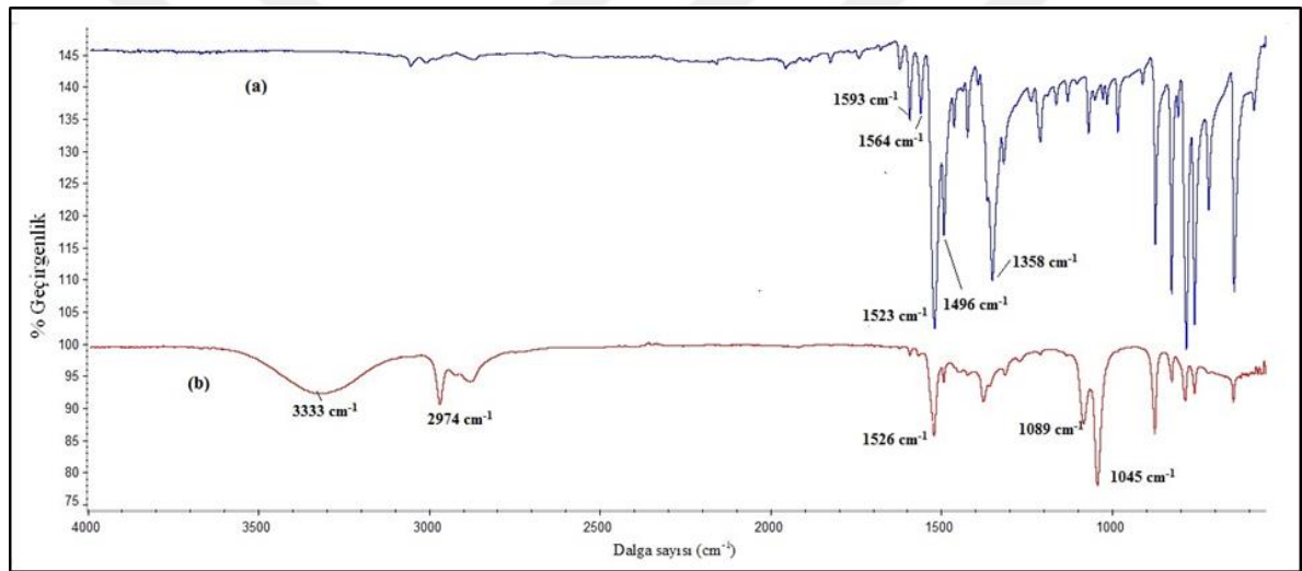
Şekil 7.15. (a) katı 8-NQ ve (b) KGE üzerindeki 8-NQ filminin FTIR spektrumu
