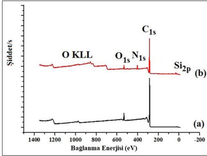
Şekil 7.10. (a) Yalın KGE ve (b) 8NQ/KGE'nin XPS genel tarama spektrumu
