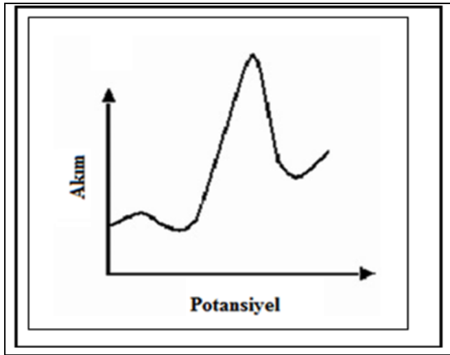
Şekil 2.9. DPV'ye ait voltamogram [15].
