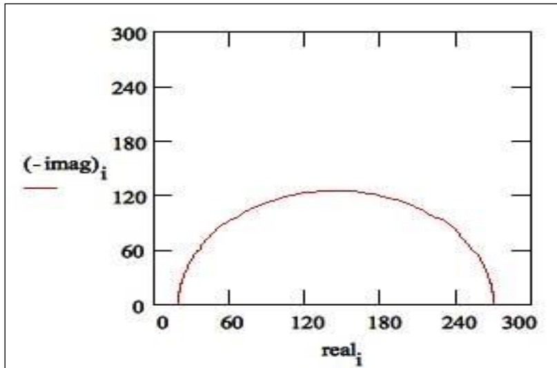
Şekil 3.16. 1 mm/yıl korozyon oranı için Nyquist grafiği [12].
