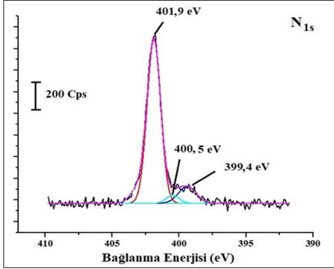
Şekil 7.8. 2-MBT/KGE yüzeyleri için N_{1s} kısmi tarama XPS spektrumu
