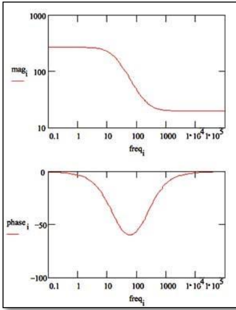
Şekil 3.17. 1 mm/yıl korozyon oranı için Bode grafiği [12].
