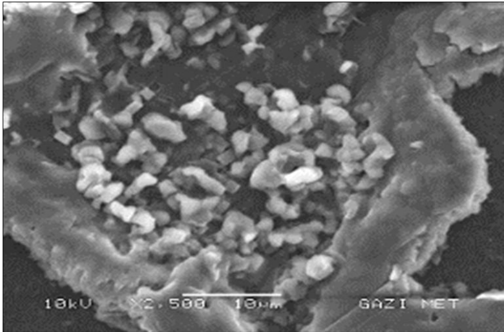
Şekil 7.17. 2-MBT/KGE yüzeyinin SEM fotoğrafı
