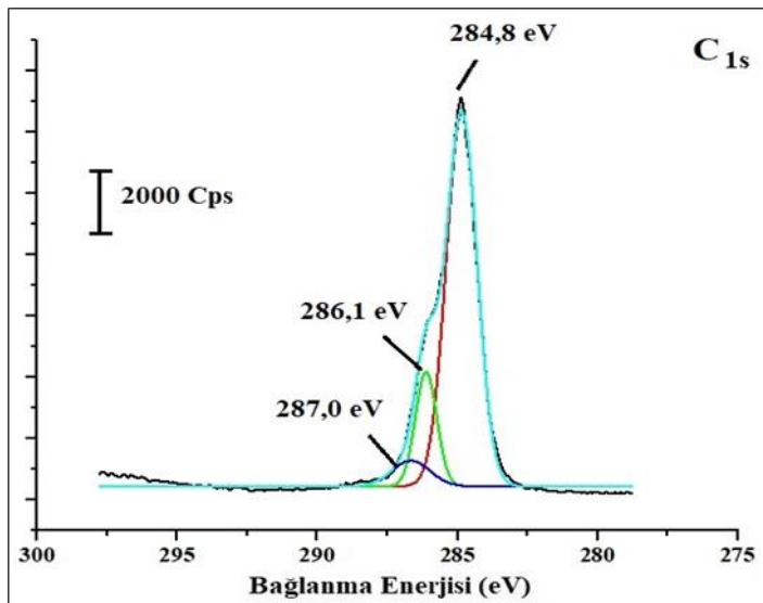
Şekil 7.7. 2-MBT/KGE yüzeyleri için C 1s kısmi tarama XPS spektrumu
