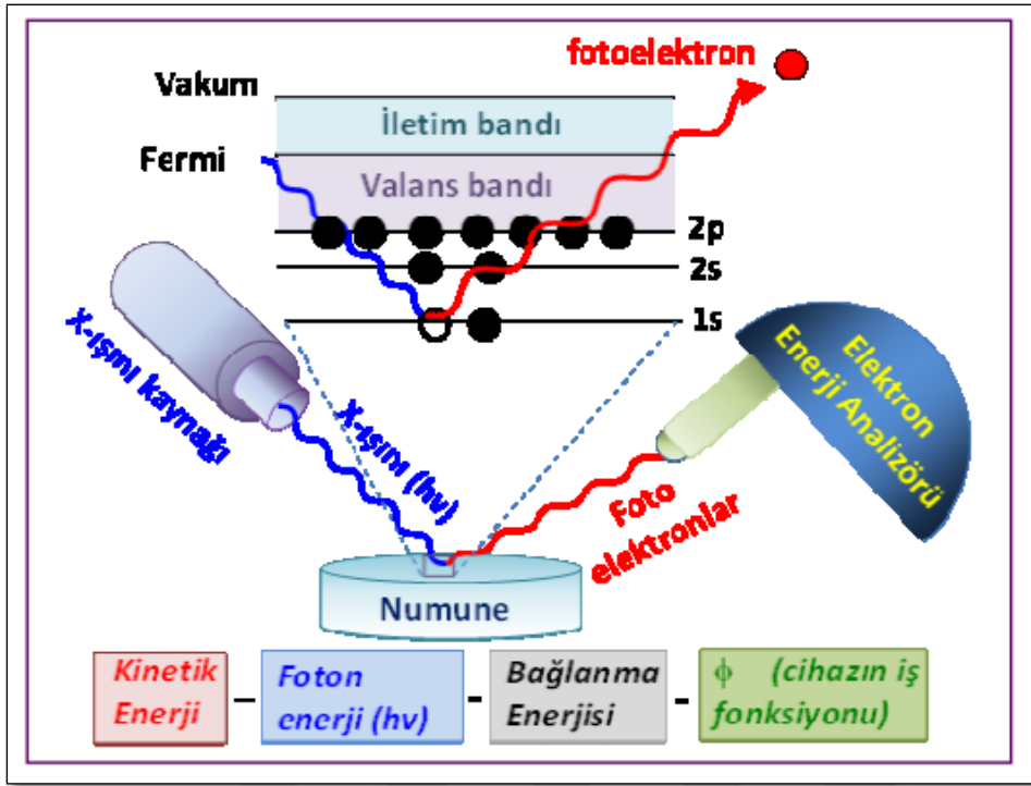
Şekil 3.26. XPS tekniğinin şematik gösterimi [74]
