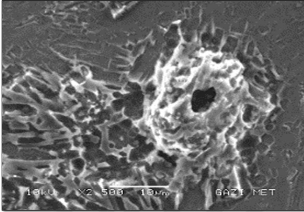
Şekil 7.18. 8-NQ/KGE yüzeyinin SEM fotoğrafı
