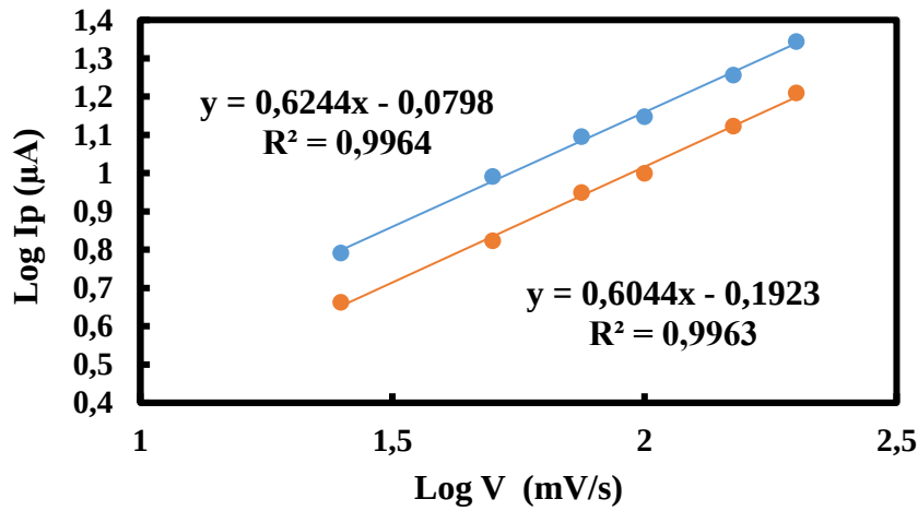
Şekil 7.20. 30 µM içeren rutin molekülünün log Ip-log v grafiği
