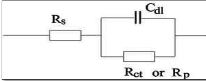
Şekil 3.15. Basitleştirilmiş randles hücre şematik diyagramı [12].
