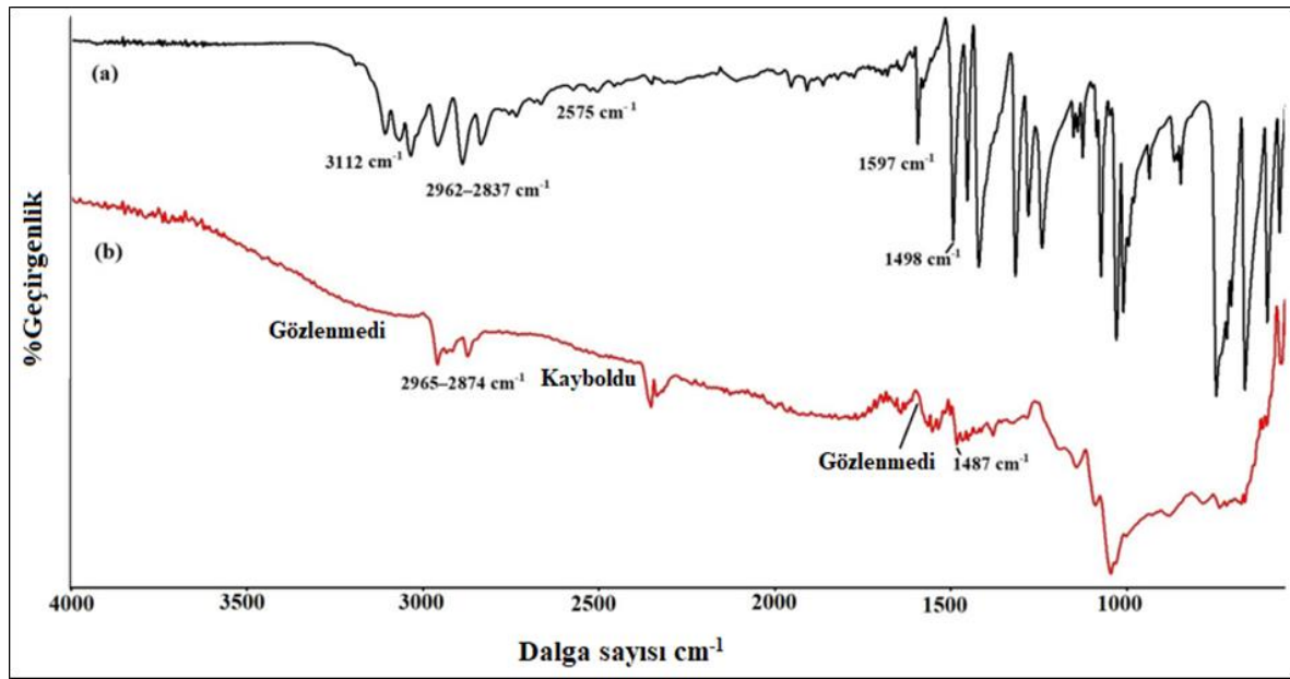
Şekil 7.14. (a) katı 2-MBT ve (b) KGE üzerindeki 2-MBT filminin FTIR spektrumu
