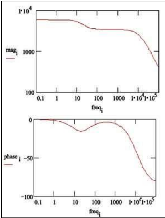
Şekil 3.25. Başarısız bir kaplama için Bode grafiği [12].
