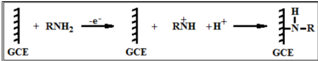
Şekil 3.2. GCE elektrodunun amin yükseltgenmesi ile modifikasyonu
