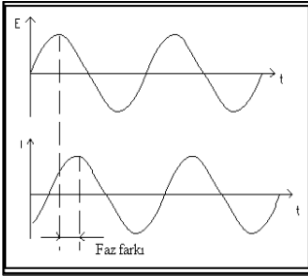
Şekil 3.6. Lineer sistemde sinüzoidal akım tepkisi [12].
