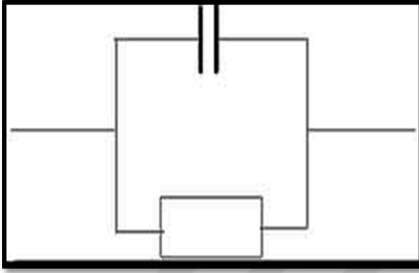
Şekil 3.9. Tek zaman sabitli basit eşdeğer devre [12].
