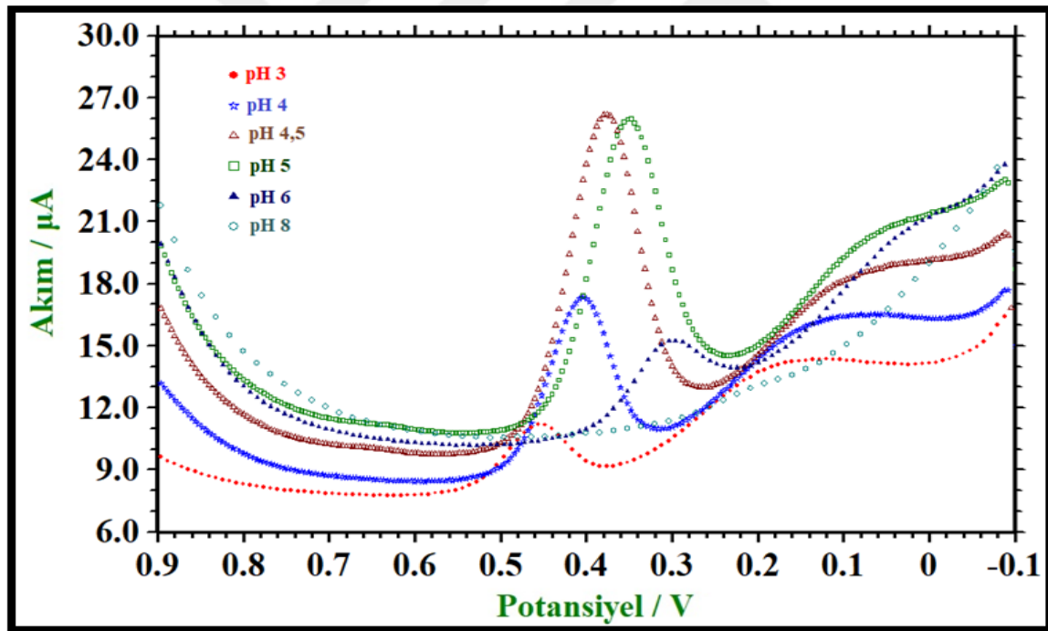
Şekil 7.26. 2-MBT/KGE elektrotları ile 30 \mu\text{M} rutin in BR tamponu ortamında pH değerleri 3,0, 4,0, 4,5, 5,0 6,0 ve 8,0 olan destek elektrolit ortamında alınmış DPV voltamogramları
