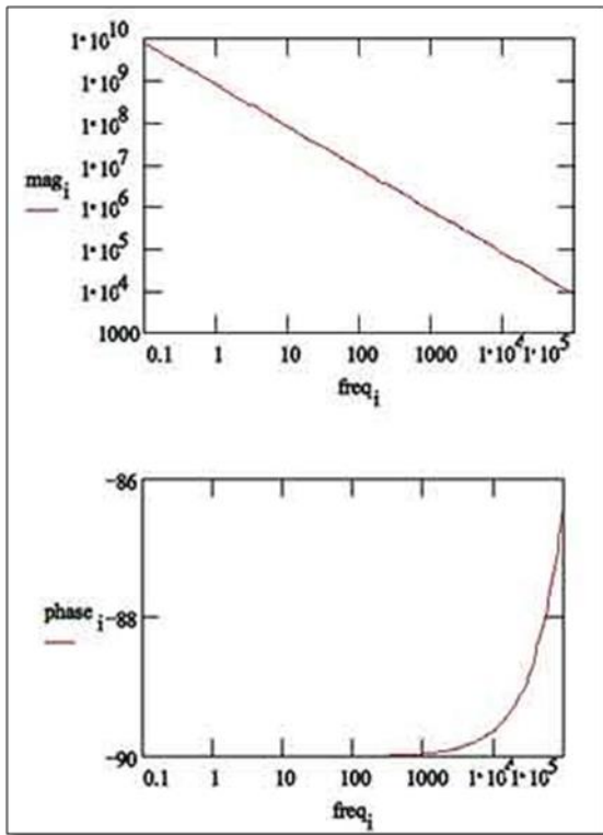
Şekil 3.14. Kaplama için tipik Bode grafiği [12].
