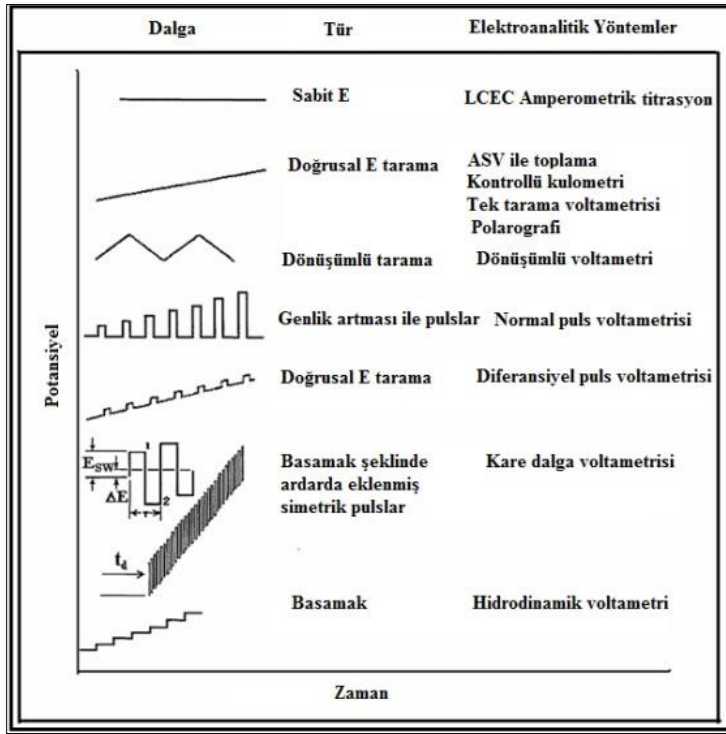
Şekil 2.2. Bazı genel voltametrik yöntemler için potansiyel uyarma sinyalleri [11].
