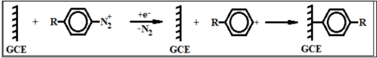
Şekil 3.1. GCE elektrodunun diazonyum tuzu indirgenmesi yöntemi ile modifikasyonu
