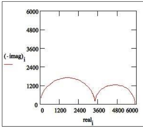
Şekil 3.24. Başarısız bir kaplama için Nyquist grafiği [12].
