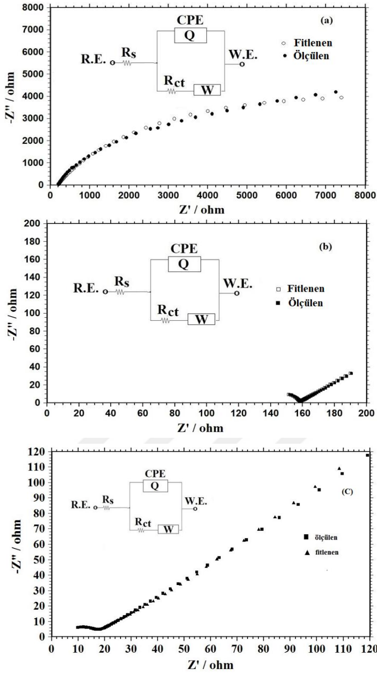
Şekil 7.5. a) Yalın KGE b) 2-MBT/KGE ve c) 8-NQ/KGE yüzeylerin 1,0 \times 10^{-3} M [\text{Fe}(\text{CN})_6]^{3-/4-} redoks çiftini içeren 0,1 M KCl çözeltisinde Nyquist grafiği, eşdeğer devre modeli ve simülasyonları
