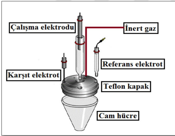
Şekil 2.3. Voltametrik ölçümlerde kullanılan bir hücrenin sistematik diyagramı [11].
