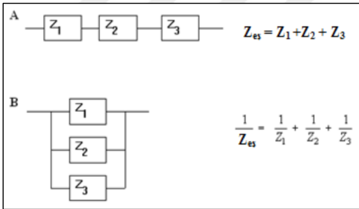
Şekil 3.11. A) Seri ve B) Paralel bağlı impedans elemanlarının ve eşdeğer impedans ( Z_{es} ) hesaplamalarının gösterilişi [12].
