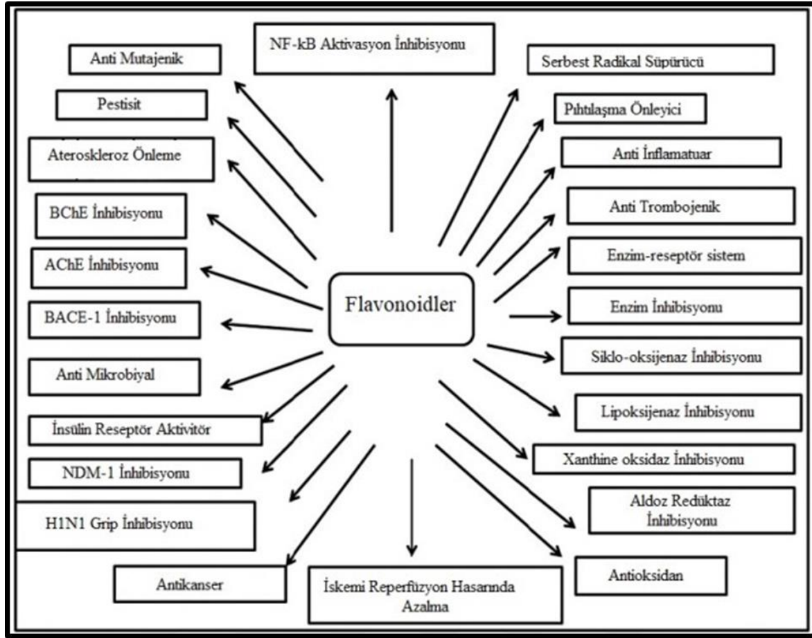
Şekil 4.2. Çeşitli biyoaktivitelerdeki flavonoidlerin insan sağlığı ve tarımdaki rolünün toplu gösterimi. BChE, bütirilkolinesteraz ; AChE, asetilkolinesteraz; BACE-1, \beta aktif bölge bölünme enzimi - 1; NDM-1, New Delhi (Yeni Delhi) metallo- \beta -laktamaz-1; H1N1, haemagglutinin 1 neuraminidase 1 [90].
