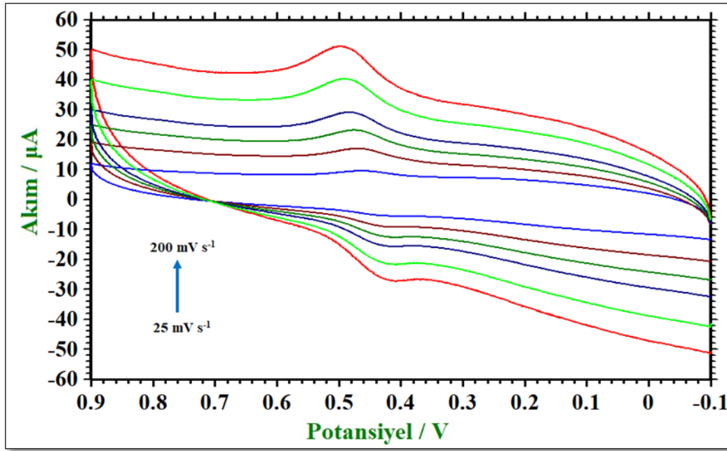
Şekil 7.19. 30 µM rutin içeren pH=4,5 BR ortamında artan tarama hızları ile 2-MBT/KGE elektrodu kullanılarak alınmış dönüşümlü voltamogramlar
