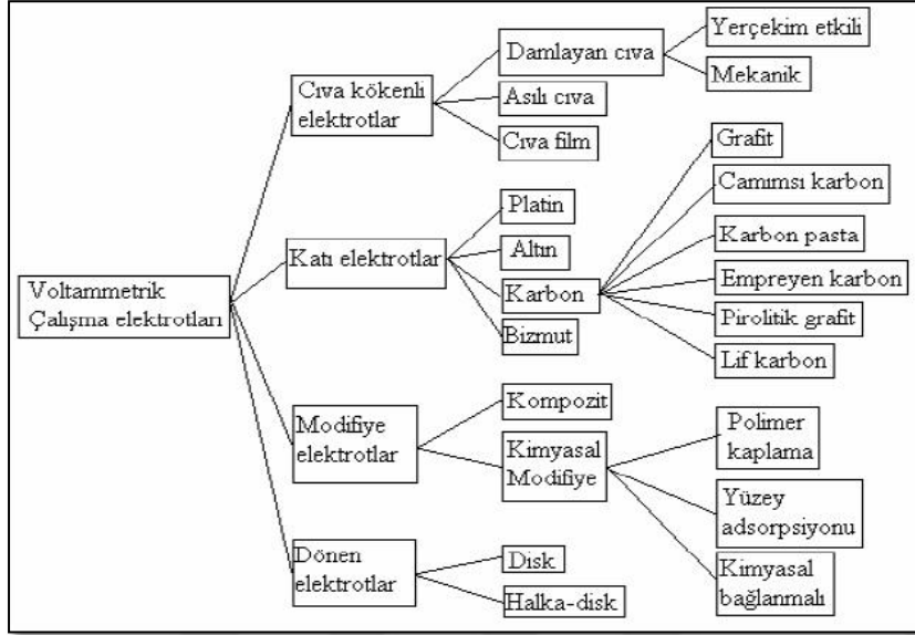
Şekil 2.10. Voltammetrik çalışma elektrotlarının genel sınıflandırılması [15].
