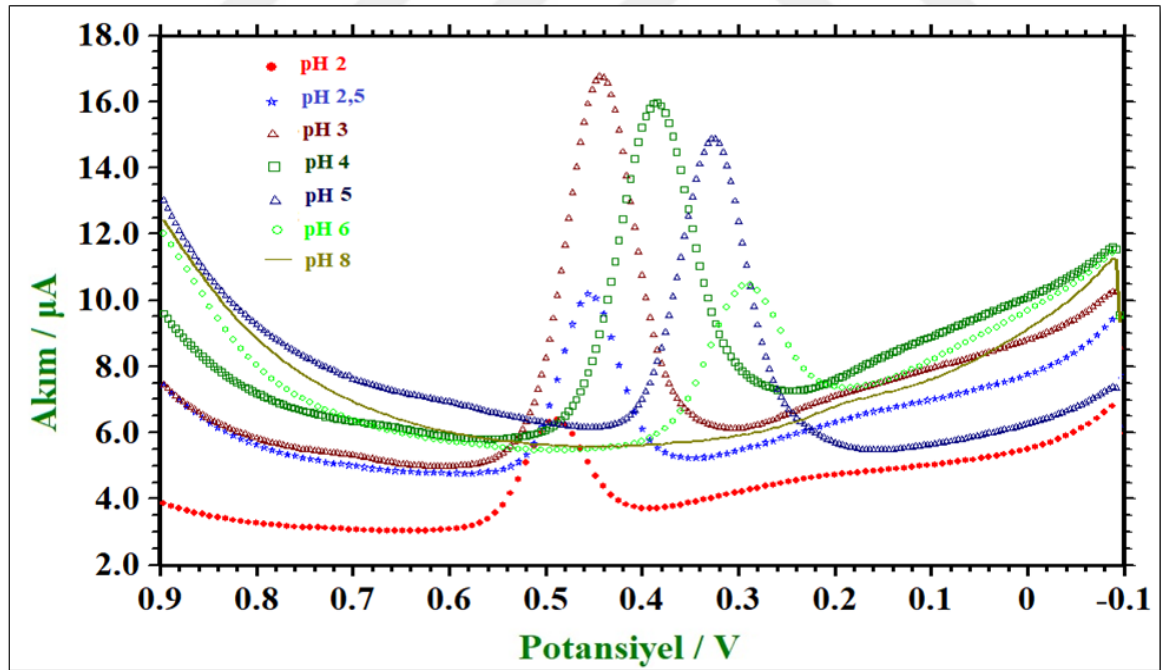
Şekil 7.29. 2 -NQ/KGE elektrotları ile 30 \mu\text{M} Ru M Rutinin BR tamponu ortamında pH değerleri 2,0, 2,5, 3,0, 4,0, 5,0 6,0 ve 8,0 olan destek elektrolit ortamında alınmış DPV voltamogramları
