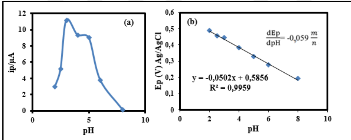
Şekil 7.30. 8-NQ/KGE'de (a) i_p -pH ve (b) E_p -pH şekilleri
