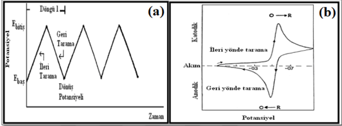
Şekil 2.4. (a) CV deneyinde zamanla uygulanan potansiyelin değişimi ve (b) Tersinir O + ne^- \rightarrow R redoks tepkimesi için elde edilen akım potansiyel eğrisi [7].
