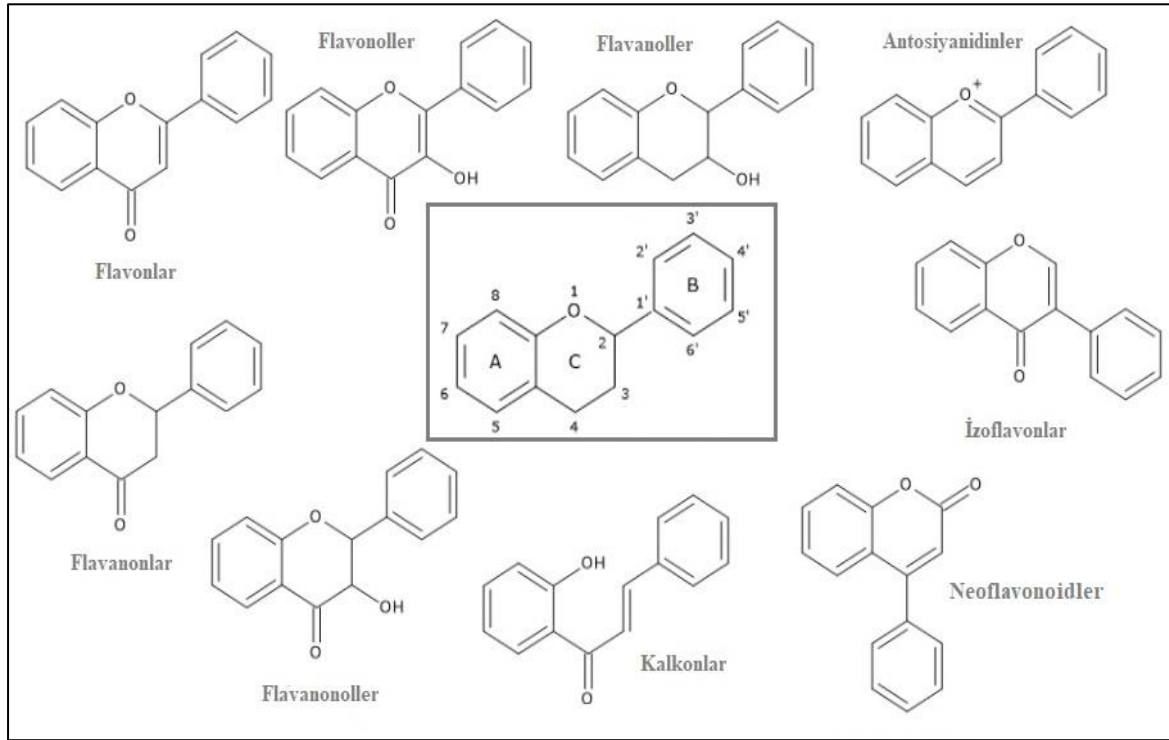
Şekil 4.1. Flavonoidlerin temel iskelet yapısı ve sınıfları [90].
