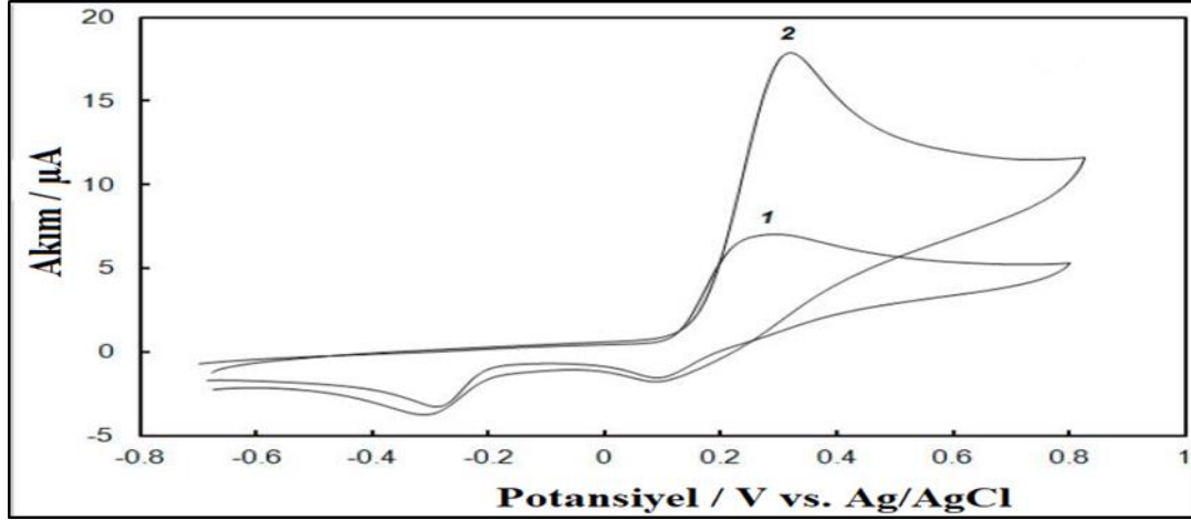
Şekil 3.5. DA'nın, a) yalın Au ve b) MCM-48/Au yüzeyindeki davranışı tarama hızı:100 mV/s, DKE [72].
