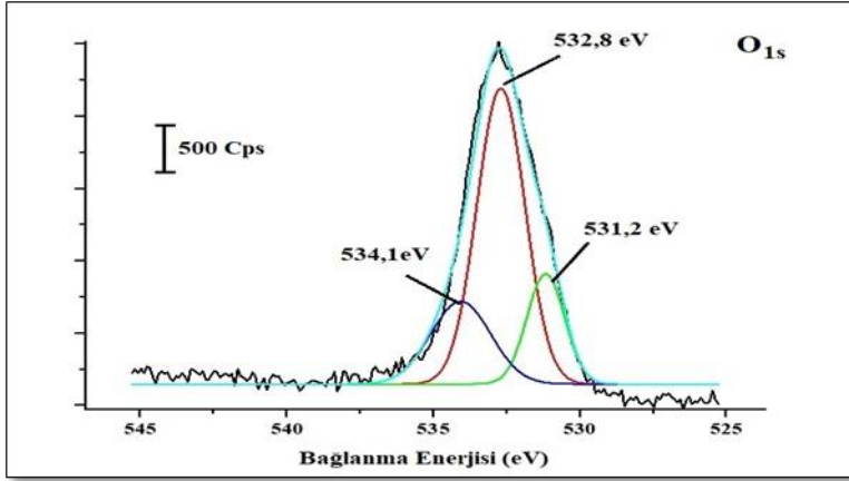
Şekil 7.13. 8-NQ/KGE yüzeyleri için O1s kısmi tarama XPS spektrumu
