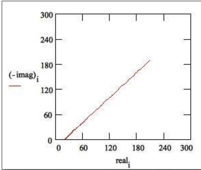
Şekil 3.18. Warburg impedansı için Nyquist grafiği [12].
