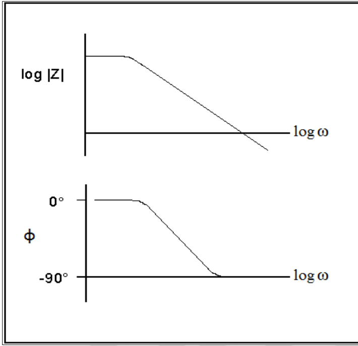
Şekil 3.10. Tek zaman sabitli bode grafiği [12].
