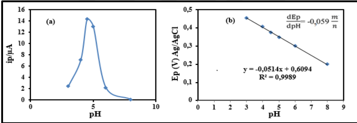
Şekil 7.27. 2-MBT/KGE'de (a) i_p -pH ve (b) E_p -pH şekilleri
