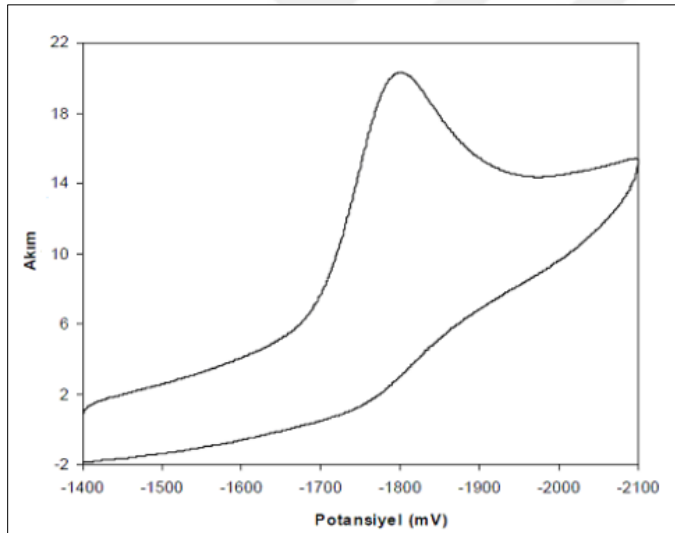
Şekil 2.5. Tersinmez reaksiyon voltamogramı [20]
