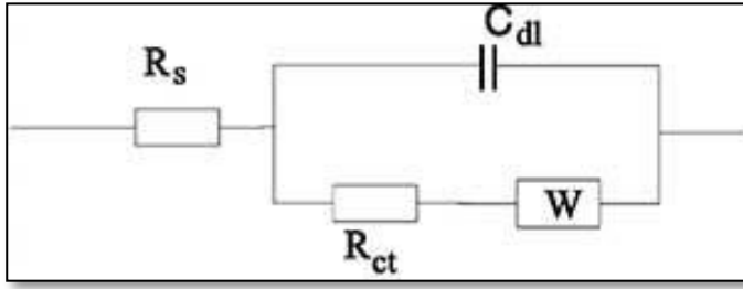
Şekil 3.20. Randles hücresi: karışık kinetik ve yük transfer kontrollü eşdeğer devre [12].
