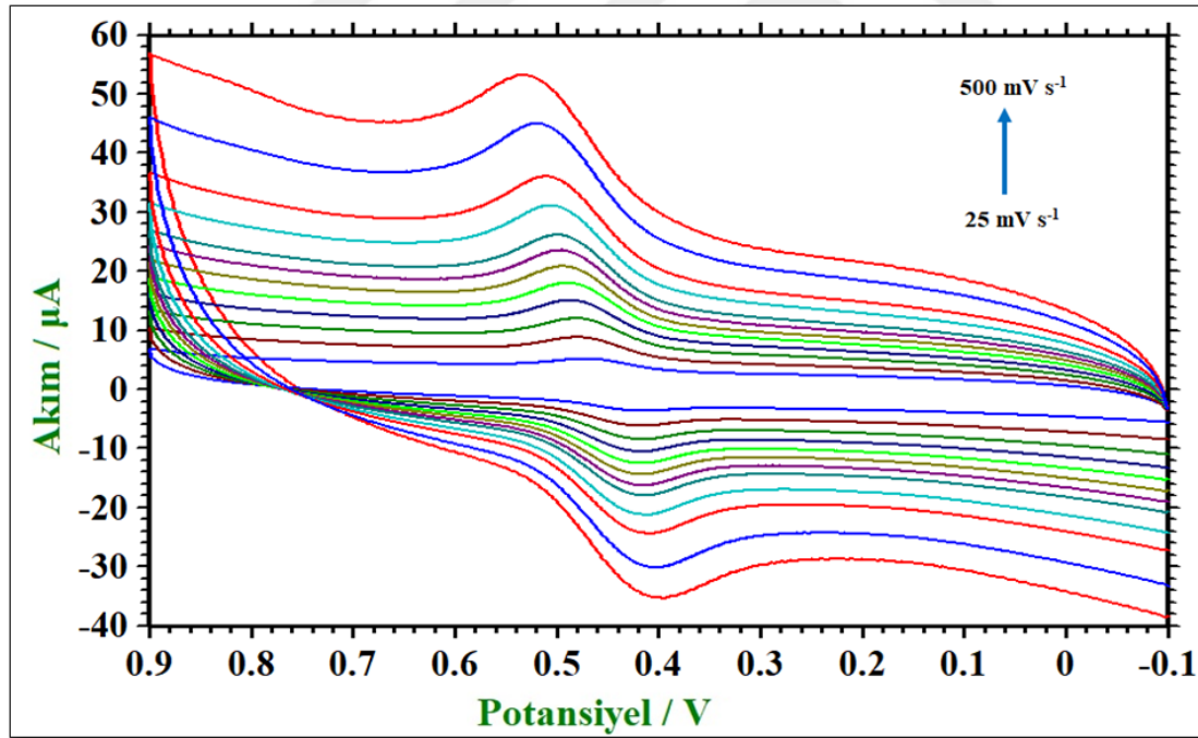
Şekil 7.23. 30 \mu M rutin içeren pH=3,0 BR ortamında artan tarama hızları ile 8-NQ/KGE elektrodu kullanılarak alınmış dönüşümlü voltamogramlar
