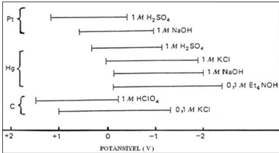
Şekil 2.11. Farklı destek elektrolit ortamlarında Pt, Hg ve C elektrotlar için çalışılabilir potansiyel aralıkları [12].
