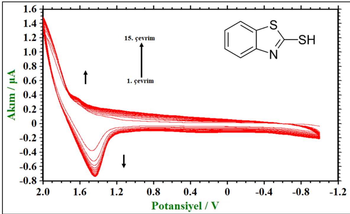
Şekil 7.1. 1,0 \times 10^{-3} 2-MBT molekülünü 0,1 M TBATFB içeren MeCN çözeltisinde yüzeyin modifikasyon voltamogramı
