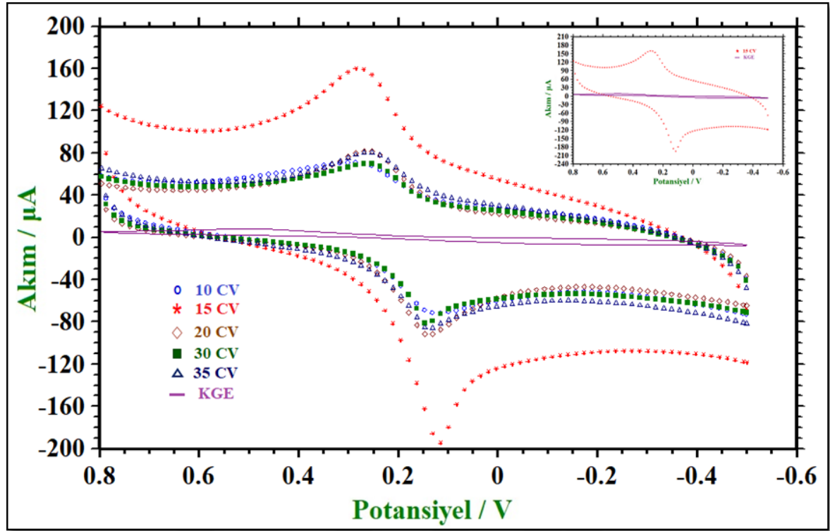
Şekil 7.3. 2-MBT/KGE ve KGE yüzeylerin, 1,0 \times 10^{-3} \text{ M} ferrisiyanür/ferrosiyanür redoks 0,1 \text{ M KCl} çözeltisinde elde edilen dönüşümlü voltamogramları
