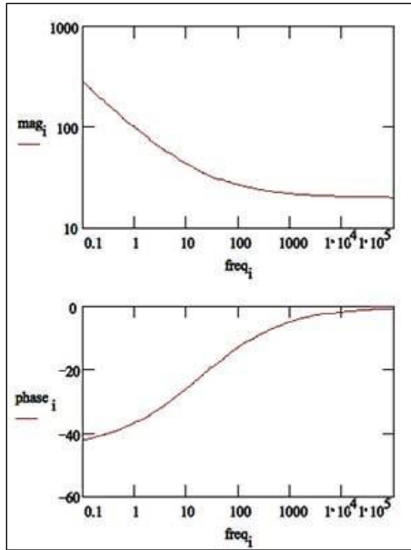
Şekil 3.19. Warburg impedansı için Bode grafiği [12].
