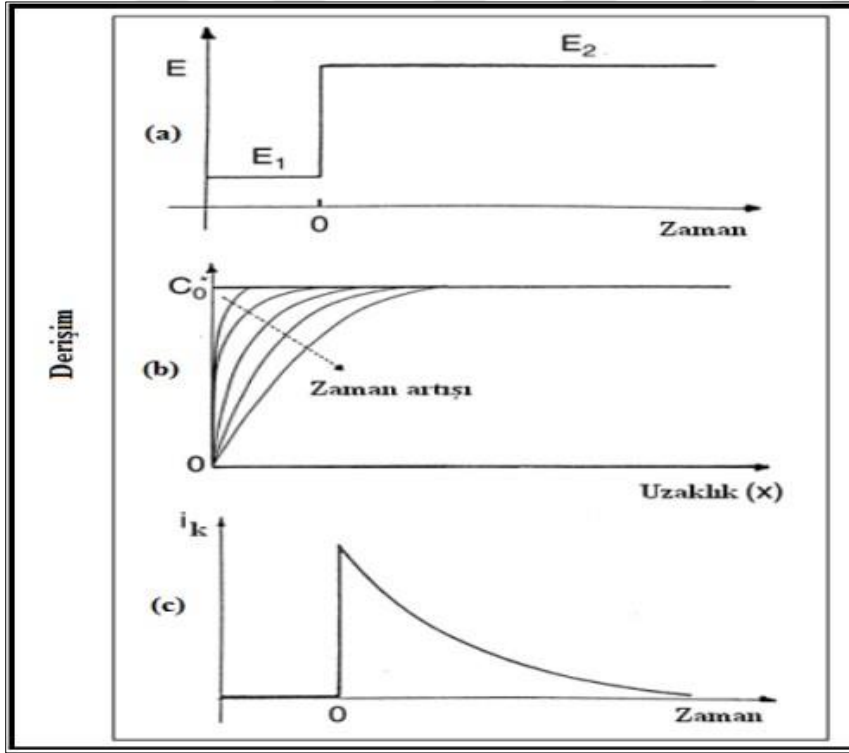
Şekil 2.7. CA ile yapılan çalışmalarda a) E_1 potansiyeline sahip bir yüzeye, belli bir zaman diliminde E_2 potansiyelinin uygulanması b) Derişim profilinin zamanla değişimi c) uygulanan potansiyelde akım-zaman değişimi [12].
