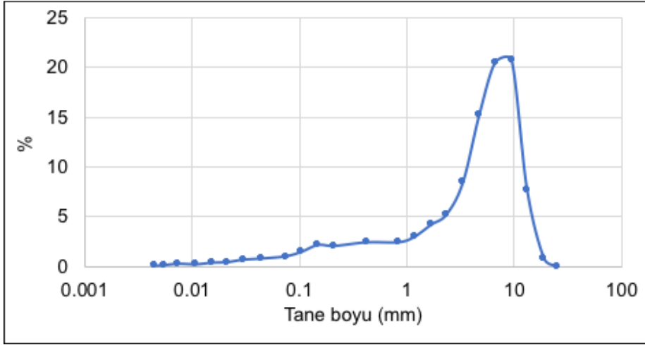
Şekil 20. Bilyalı değirmen için hesaplanan tek tane kırılma fonksiyonu
