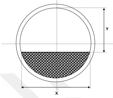
Şekil 22. Değirmen kesiti
