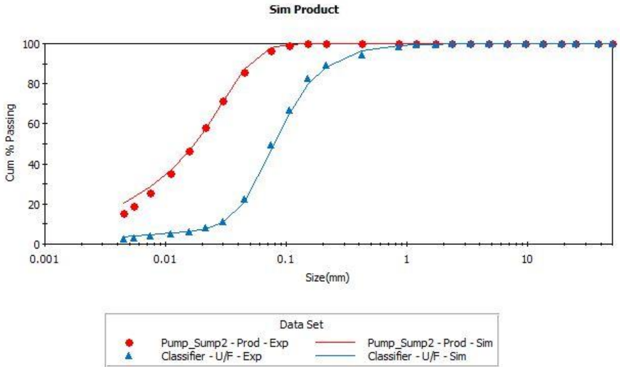
Şekil 73. 4 No'lu Çimento Öğütme Devresi referans koşuluna ait ölçülen ve hesaplanan boyut dağılımları
