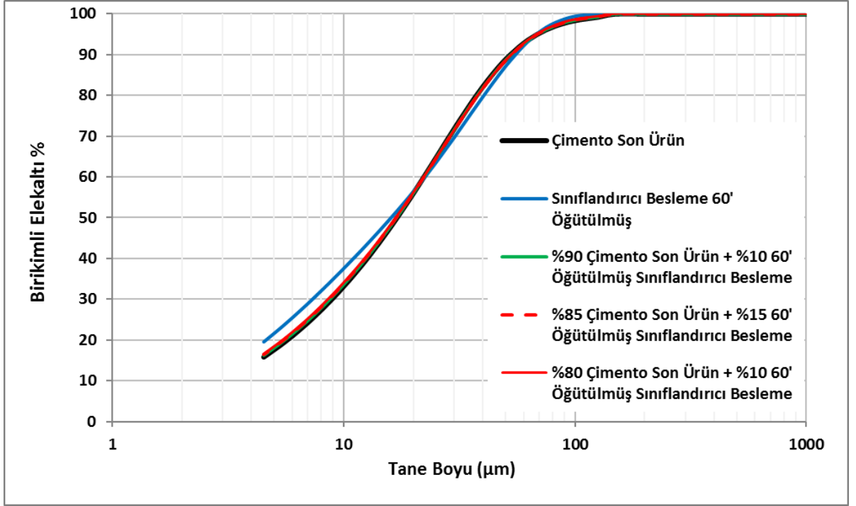
Şekil 51. 4 No’lu Çimento Öğütme Devresi’ne ait hazırlanan karışımların tane boyu dağılımları (sınıflandırıcı besleme ve çimento son ürün)
