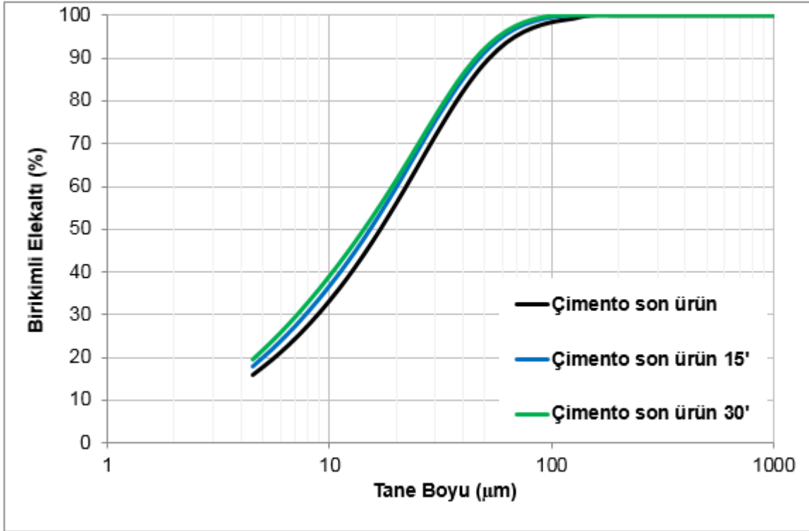
Şekil 38. 4 No'lu Çimento Öğütme Devresi, çimento son ürünü boyut dağılımları
