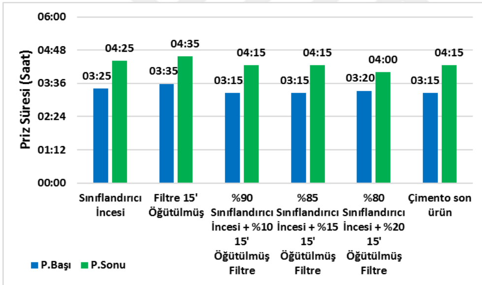
Şekil 50. 4 No'lu Çimento Öğütme Devresi'ne ait hazırlanan karışımların priz süreleri (filtre ve sınıflandırıcı incesi)
