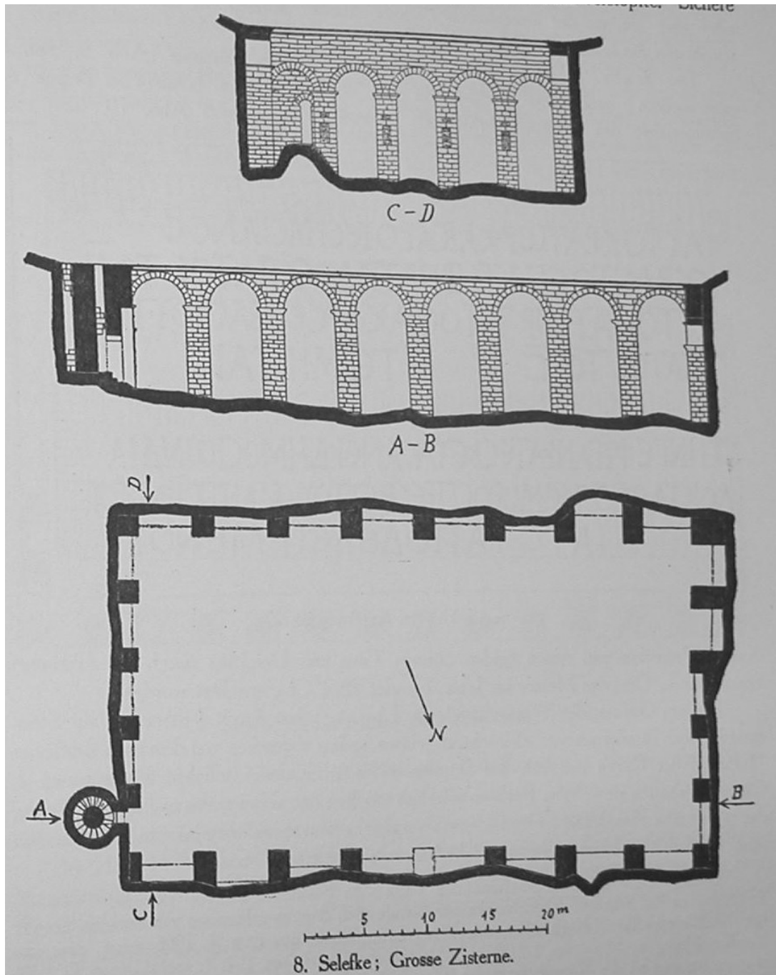
Figür 51: Tekir Ambarı Planı (Keil-Wilhelm 1931,5,Abb.8).
