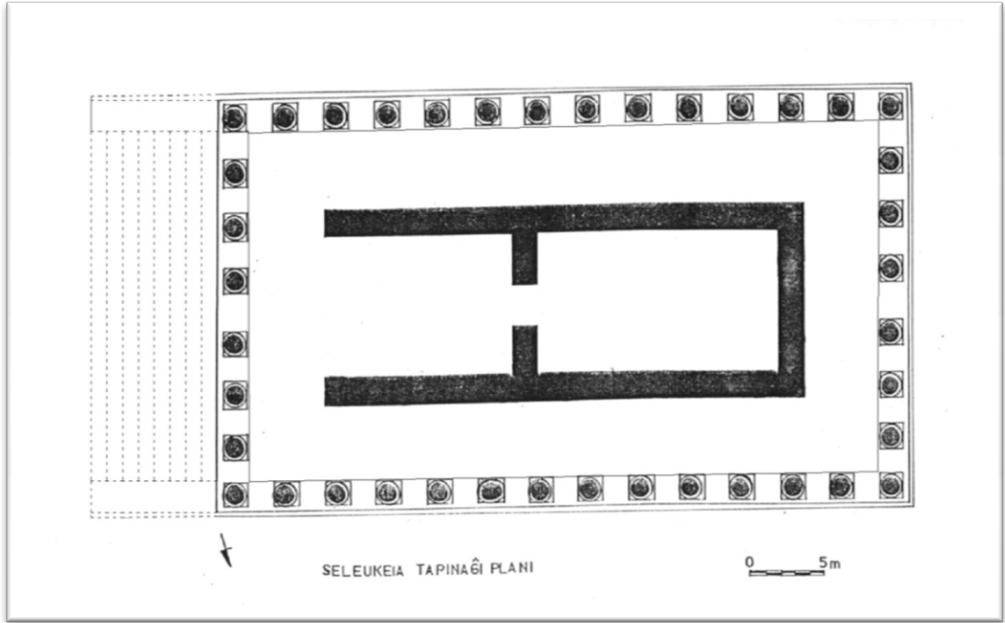
Figür 11: Tapınak Planı (Topçu'dan İşlenerek).
