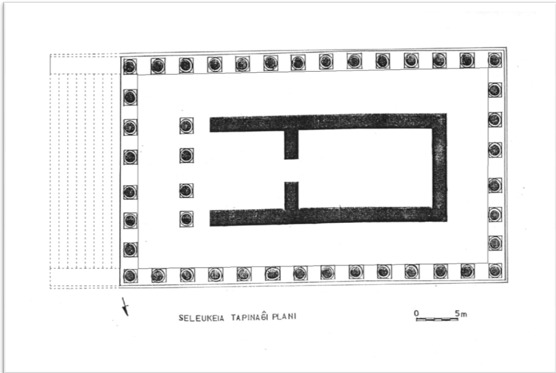
Figür 12: Tapınağın Prostýlos Girişli Planı (Topçu'dan İşlenerek).
