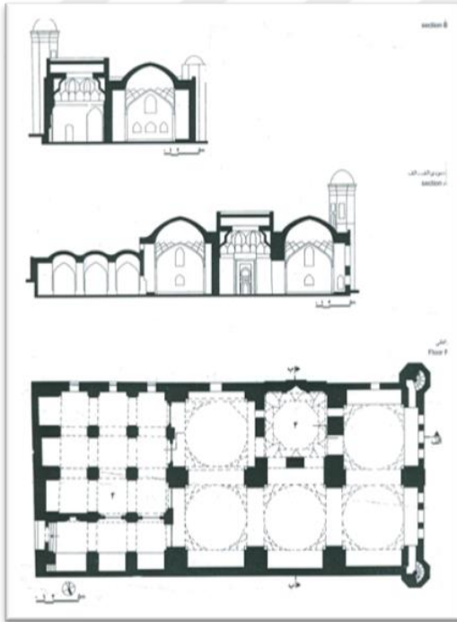
Diyagram 11.1. Marand Camisinin Planı
