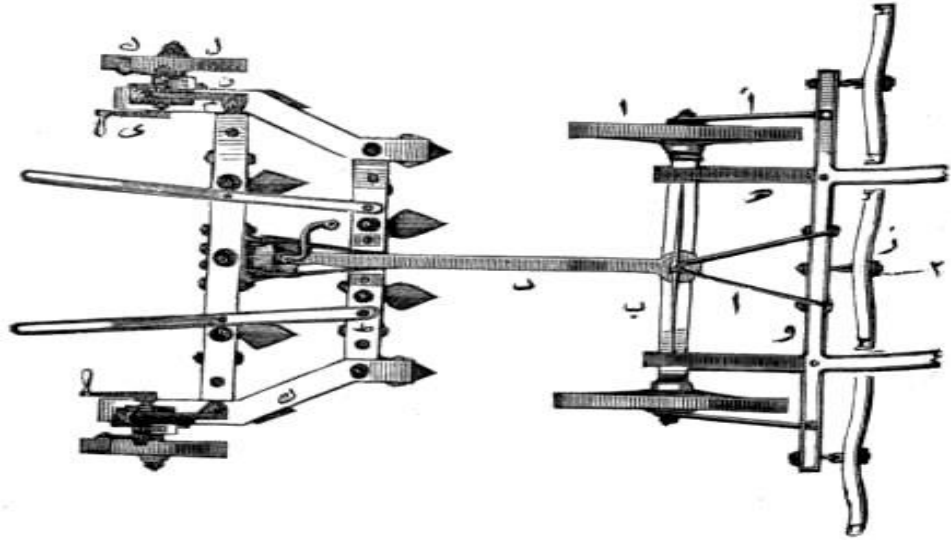
Şekil 115 Sürgü sabanının sathı
