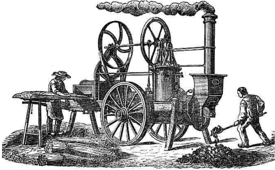
Şekil 276 Renöd ve Lóc vapor döğeni
