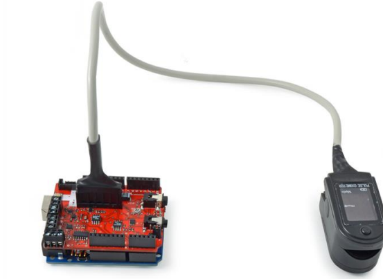
Şekil 3.6. e-Health platform pulse and oxygen in blood sensörü.
