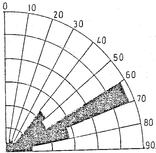
Şekil 22. Beydağı kireçtaşı çatlak düzlemlerinin eğim miktarına ait Gül diyagramı (300 ölçü).
