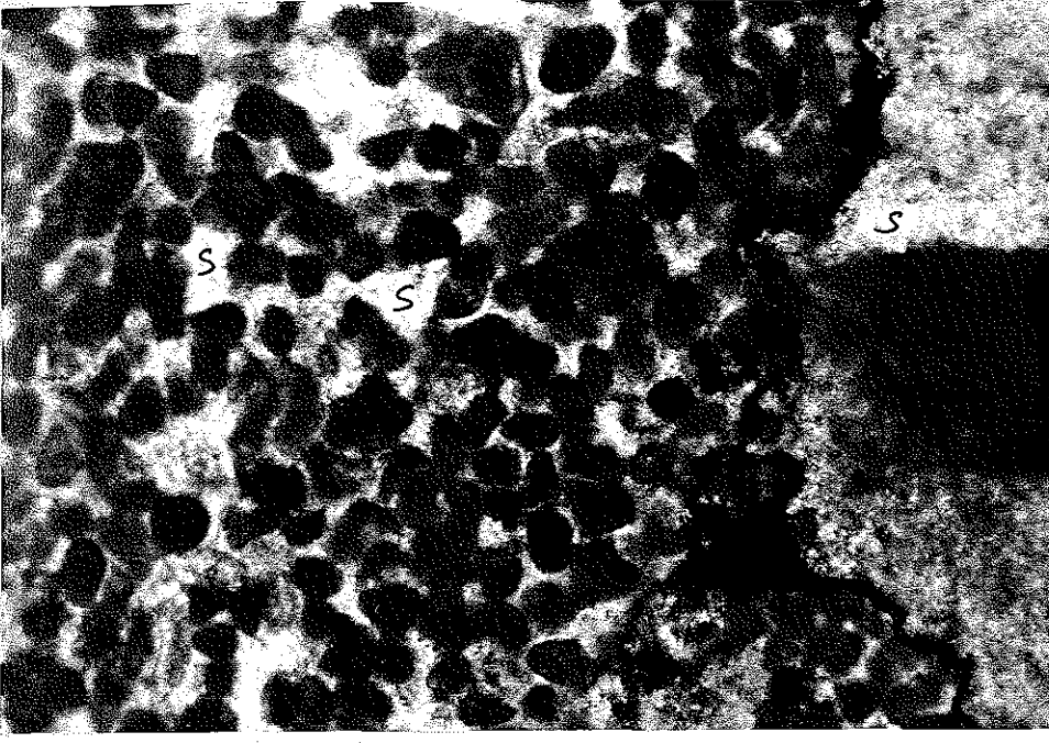
Foto 3. Beydağı kireçtaşlarında Pelsparitik dokunun mikroskobik görüntüsü.
