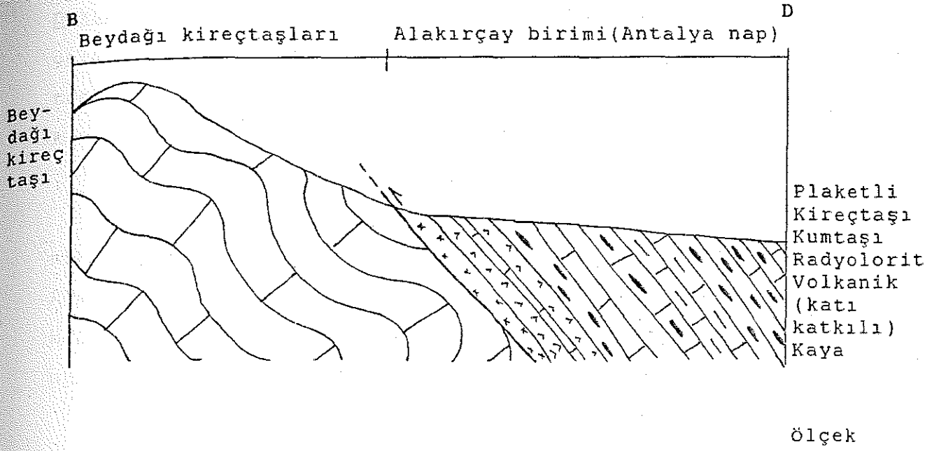
Şekil 10. Güllük Dağı kenarında Beydağı kireçtaşları ile Alakırçay birimini gösteren şematik enine jeolojik kesit.
