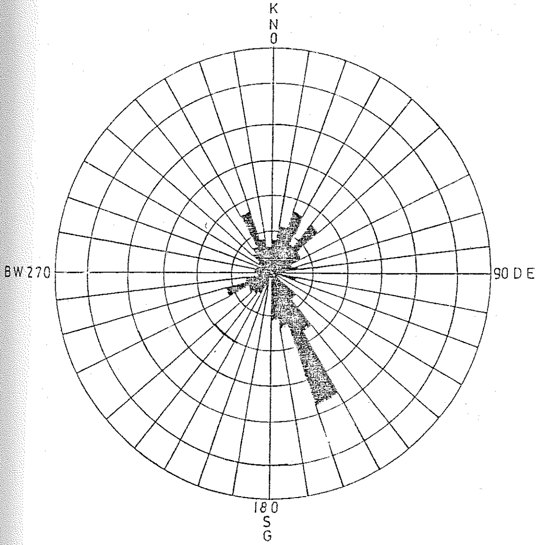
Şekil 23. Beydağı kireçtaşı çatlak düzlemine ait eğim yönü Gül diyagramı (300 ölçü).
