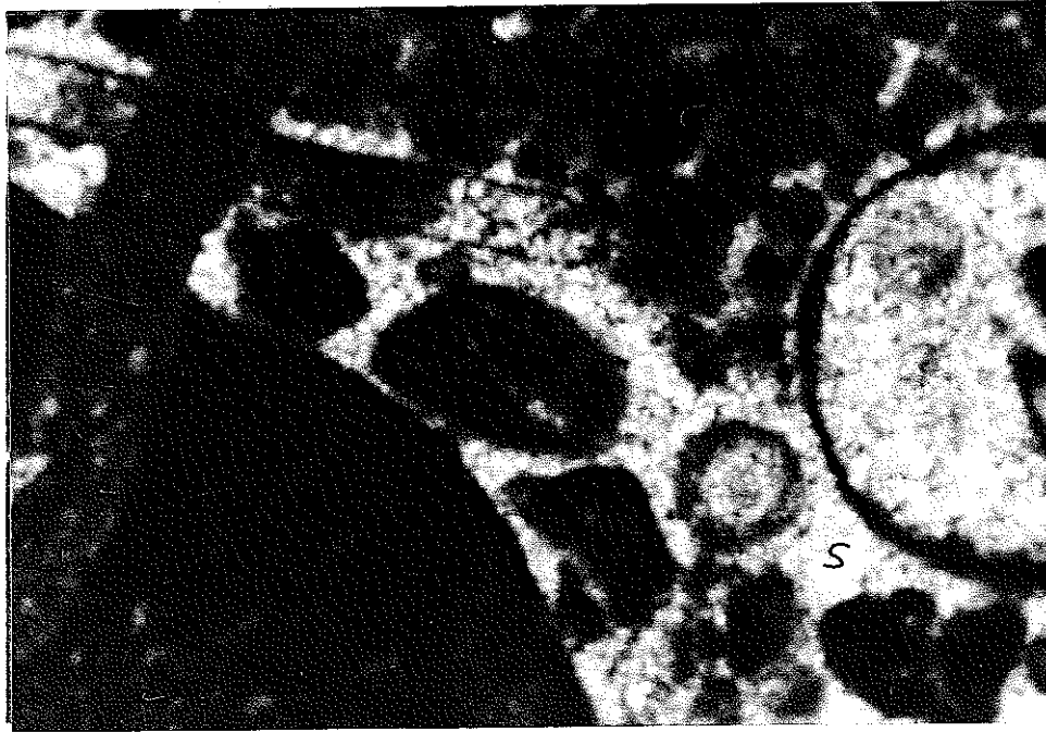
Foto 6. Beydağı kireçtaşında intaklast parçalarının mikroskopik görünüşü
