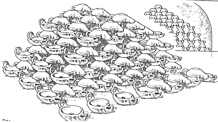
Çizim 4: Fırında Kandil Dizilişi (Çokay, 1996, Lev. 8, Çiz. 3)
