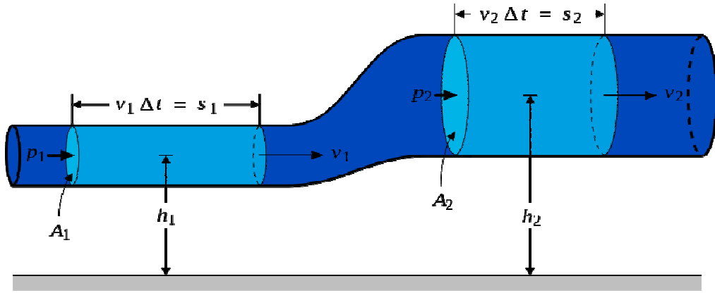
Şekil 1.1: Sürekli akışkanın hız momentum grafiği
