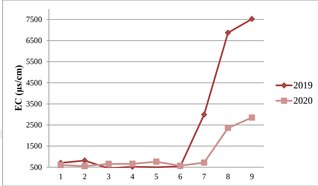
Şekil 4.2. Su örneklerinin EC (µs/cm) düzeylerinin istasyonlara göre değişimi
