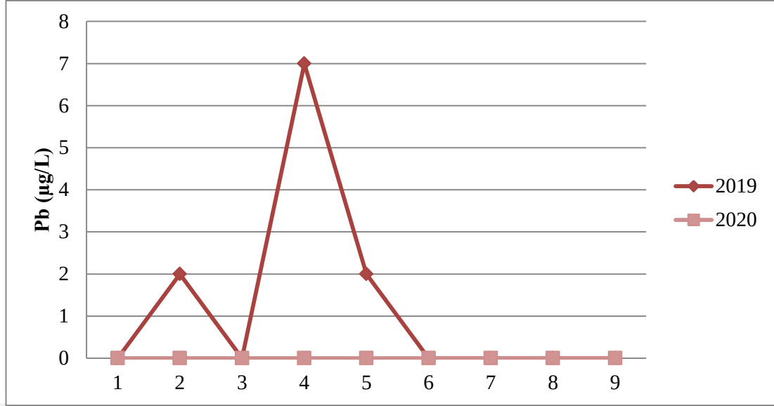
Şekil 4.15. Su örneklerinin kurşun konsantrasyonlarının (µg/L) istasyonlara göre değişimi
