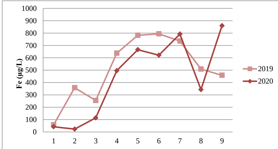
Şekil 4.9. Su örneklerinin demir konsantrasyonlarının (µg/L) istasyonlara göre değişimi
