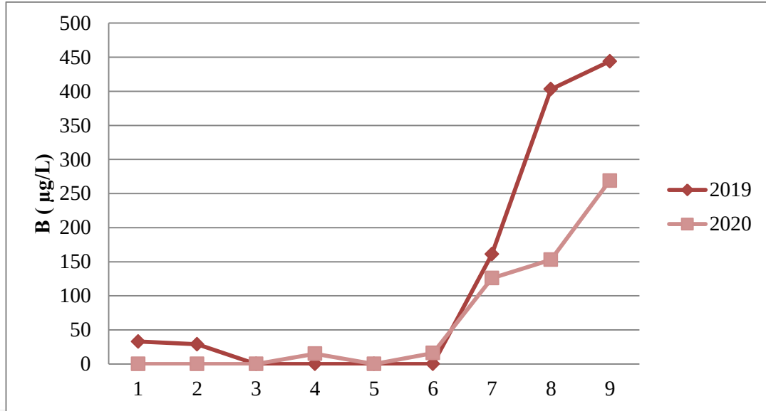
Şekil 4.20. Su örneklerinin bor konsantrasyonlarının (µg/L) istasyonlara göre değişimi
