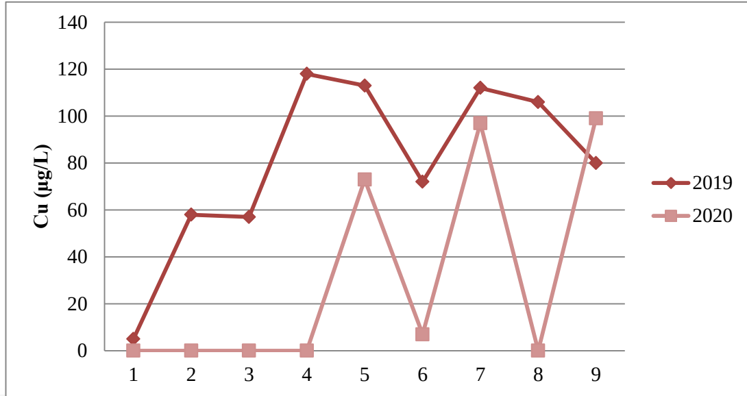
Şekil 4.12. Su örneklerinin bakır konsantrasyonlarının (µg/L) istasyonlara göre değişimi
