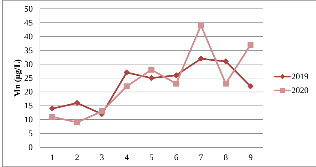
Şekil 4.10. Su örneklerinin mangan konsantrasyonlarının (µg/L) istasyonlara göre değişimi
