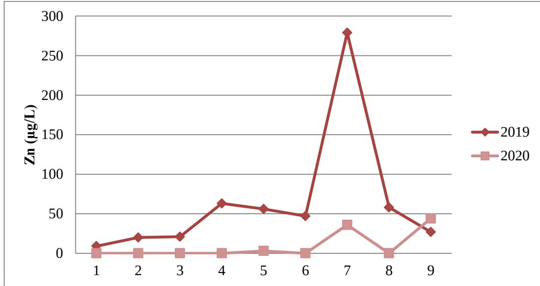
Şekil 4.11. Su örneklerinin çinko konsantrasyonlarının (µg/L) istasyonlara göre değişimi
