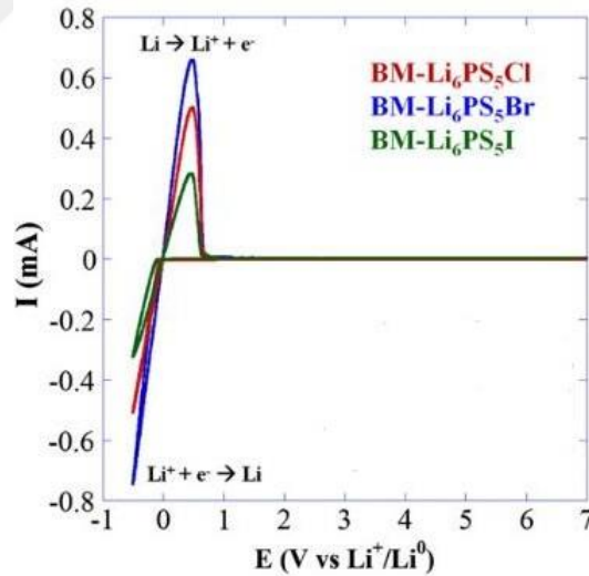
Şekil 3.12. \text{Li}_6\text{PS}_5\text{X} ( \text{X}=\text{Cl}, \text{Br}, \text{I} ) katı elektrolitlerin elektrokimyasal pencere analizi [27].
