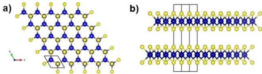
Şekil 5.5. 2H MoS 2 fazının şematik görünümü.
