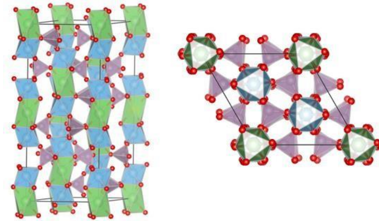
Şekil 3.14. LATP kristal yapısı şematik görünümü.
