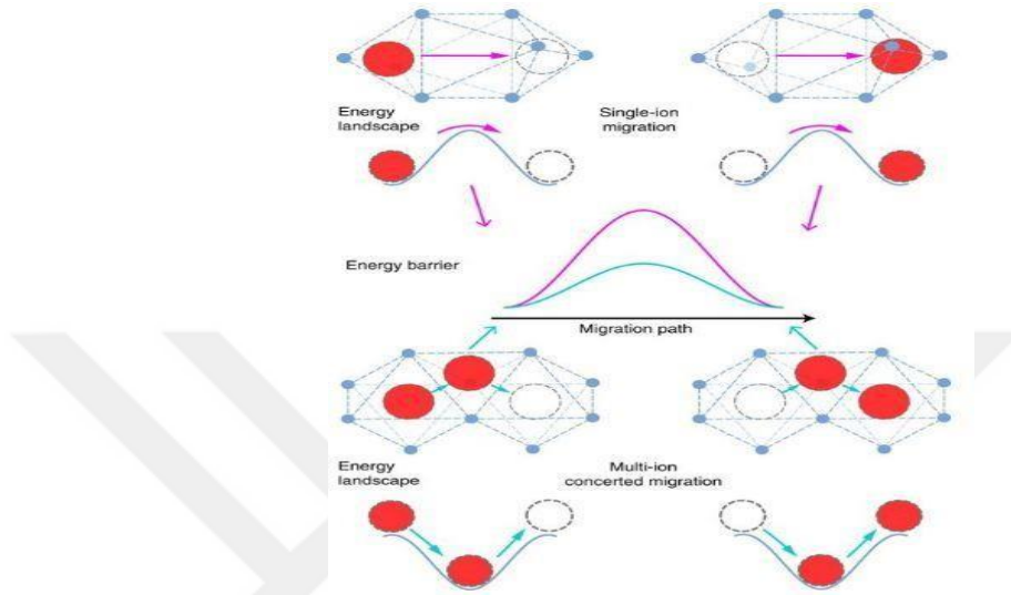
Şekil 4.1. Tek ve birkaç atomun birlikte hareketine ait klasik difüzyon modeli ve ilgili aktivasyon enerji bariyerleri [34].
