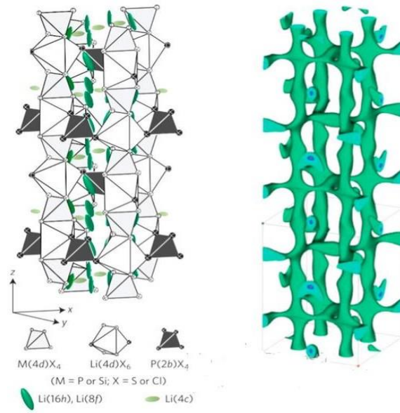
Şekil 3.13. \text{Li}_{9.54}\text{Si}_{11.74}\text{P}_{1.44}\text{S}_{11.7}\text{Cl}_{0.3} katı elektrolitinde kristal yapı ve lityum iyon difüzyon kanalları [29].
