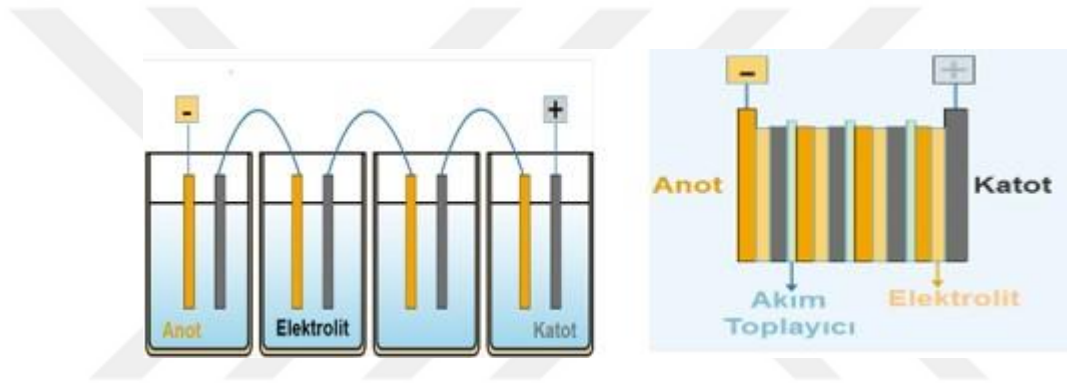
Şekil 3.2. Sıvı ve katı elektrolit içeren pillerin paketlenmesi.
