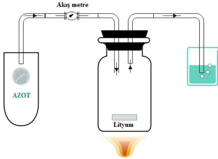
Şekil 5.2. Lityum yüzeyinin nitrürlemesi mekanizması.
