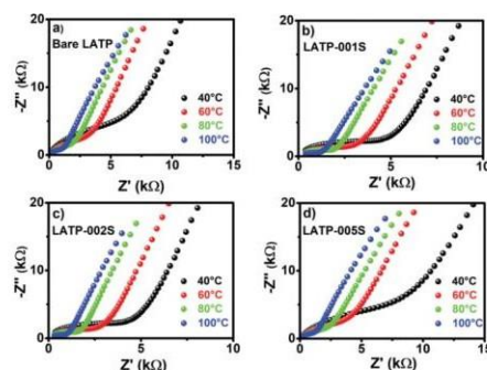
Fig. 7 Nyquist plots for (a) bare-LATP, (b) LATP-001S, (c) LATP-002S and (d) LATP-005S.
