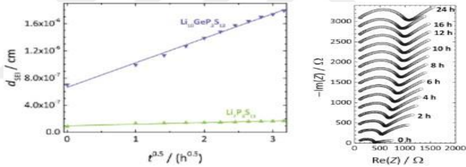
Şekil 3.9. \text{Li}_{10}\text{GeP}_2\text{S}_{12} ve \text{Li}_7\text{P}_3\text{S}_{11} katı elektrolitlerinde zamana bağlı ara yüzey kalınlığının ilerlemesi ve empedans analizi [25].
