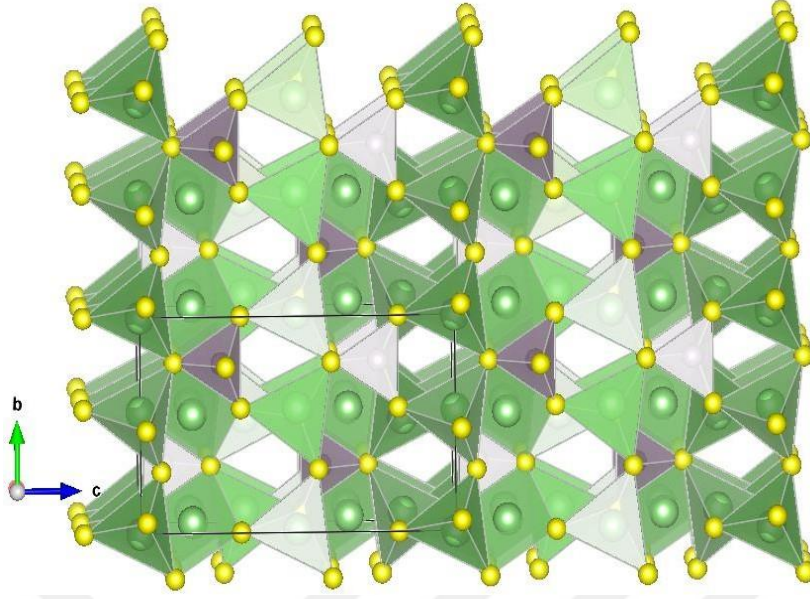
Şekil 3.4. \text{Li}_3\text{PS}_4 kristal yapısı şematik görünümü.
