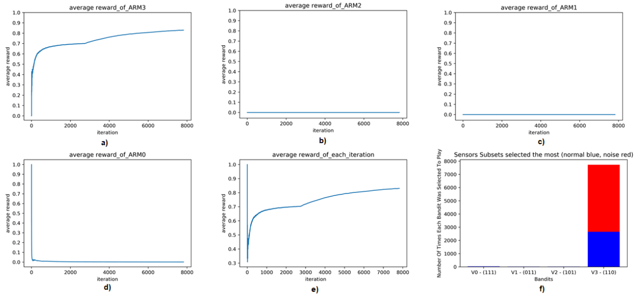
Şekil 4.8. Test 3 için UCB algoritmasında elde edilen grafikler, (a) KOL3 için ortalama ödül grafiği, (b) KOL2 için ortalama ödül grafiği, (c) KOL1 için ortalama ödül grafiği, (d) KOL0 için ortalama ödül grafiği, (e) genel ortalama ödül grafiği, (f) KOL0 , KOL1 , KOL2 ve KOL3 'ün seçilme sayılarının normal ve gürültülü veriye göre değişimi (normal veri mavi renk, gürültülü veri kırmızı renk)
