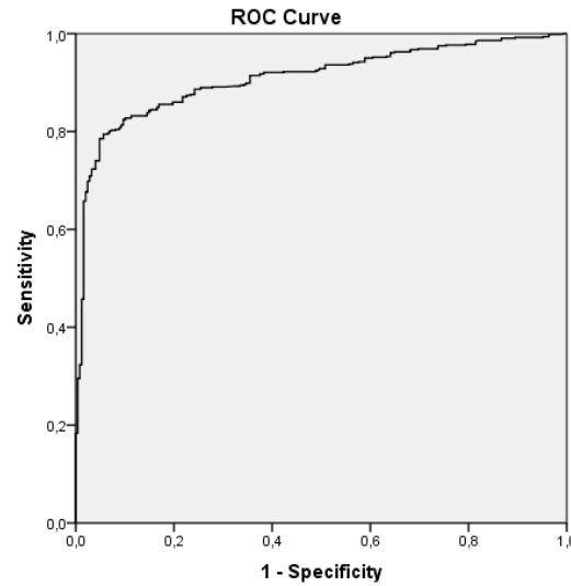
Şekil 4.4. Pozitif gerçek durum “var” için ROC analiz grafiği (Örnek vd.’den, 2020)
