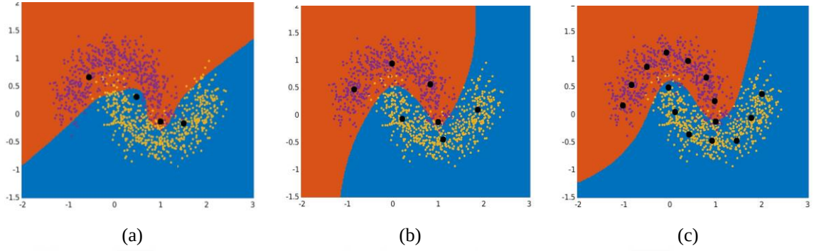
Şekil 5.6 Farklı merkez sayıları ile MCPCC- L_2 karar bölgesi değişimi; merkez sayıları a) 4, b) 7, c) 15; siyah noktalar merkezleri, kırmızı bölge negatif alanı, mavi bölge pozitif alanı temsil etmektedir.
