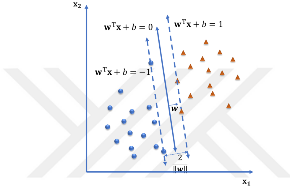
Şekil 2.5 Katı marj SVM sınıflandırma
