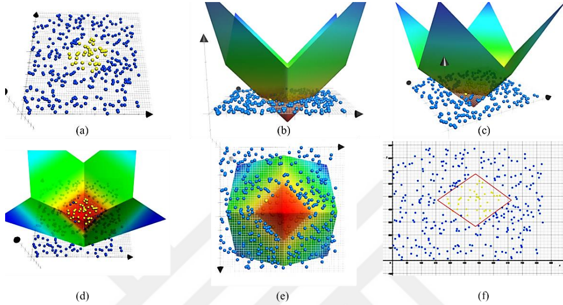
Şekil 2.12 İki sınıfın ayrılması amacıyla PCF fonksiyonu ile koni oluşturulmaktadır. Bu koninin farklı açılardan görünümü (b,c,d,e) ile gösterilmiştir. (f)'te, pozitif (sarı) örnekler, negatif (mavi) örneklerden PCF seviye kümesinden elde edilmiş karar sınırı ile ayrılmıştır (Cevikalp ve Sağlamlar'dan, 2019).
