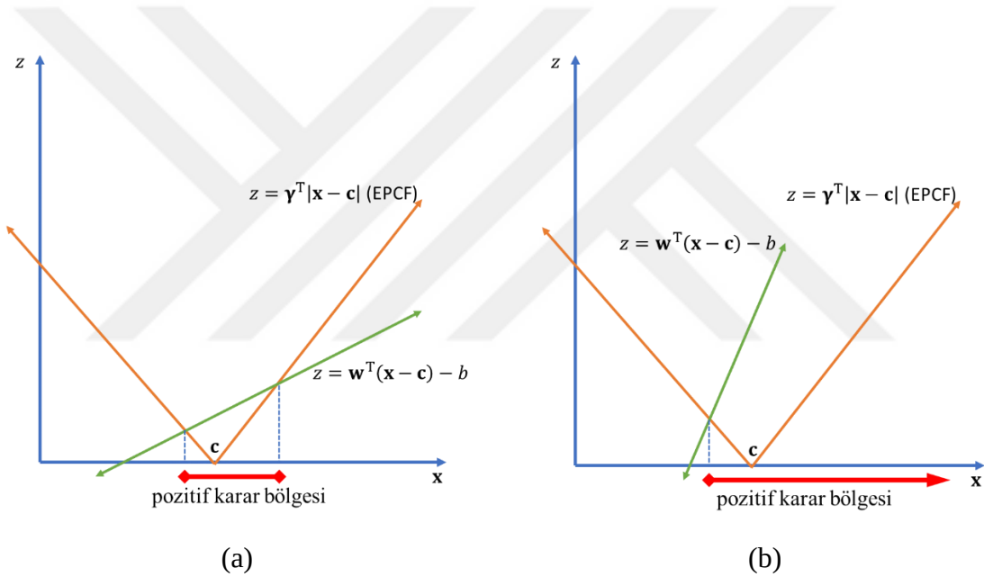
Şekil 4.3 b > 0, \gamma > 0, |w_i| < \gamma_i, i = 1, \dots, d şartları ile z = \mathbf{w}^T(\mathbf{x} - \mathbf{c}) - b hiperdüzlem (yeşil) eğimi koninin (turuncu) yanal yüzeyinin eğiminden daha küçük olur ve pozitif karar bölgesi kompakt sınırlı bir alan oluşturur, b) diğer durumda karar bölgesi sınırlı olmaz, sonsuza uzar.
