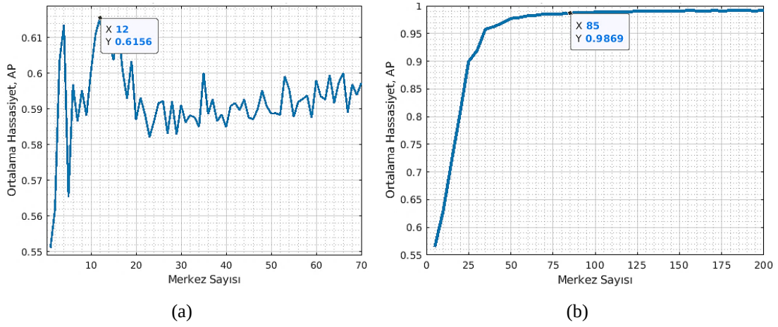
Şekil 5.9 Merkez sayısı değişimi ile ortalama hassasiyet değişimi: a) MCPCC- L_1 , b) MCPCC- L_2
