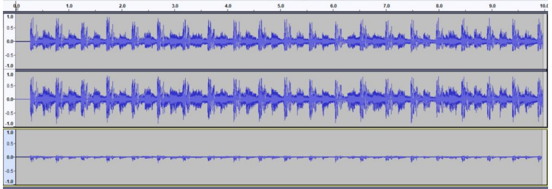
Şekil 8.3 FPGA AM verici sisteminin A2 modüle edici sinyaliyle yapılan test sonuçları: üstte A2 test sinyali, ortada modülasyonu takiben demodülasyonla elde edilen dalga şekli, altta iki sinyalin farkı
