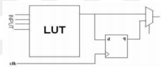
Şekil 3.2. Mantık hücresi
