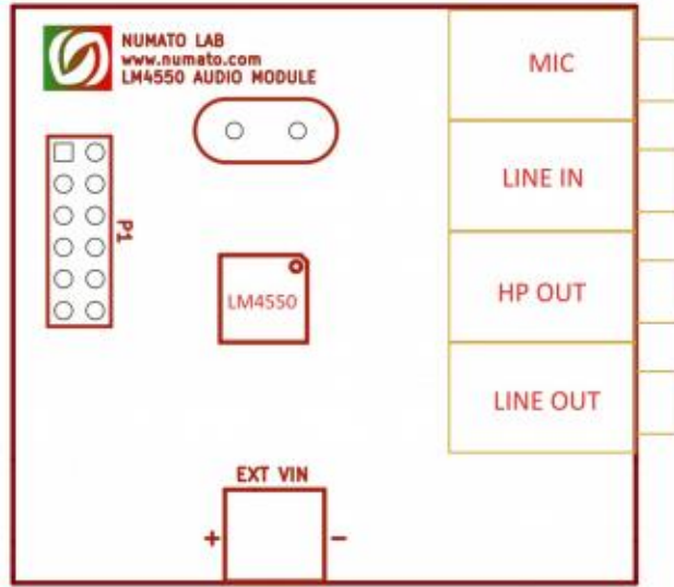
Şekil 7.6. LM4550 bağlantı şeması
