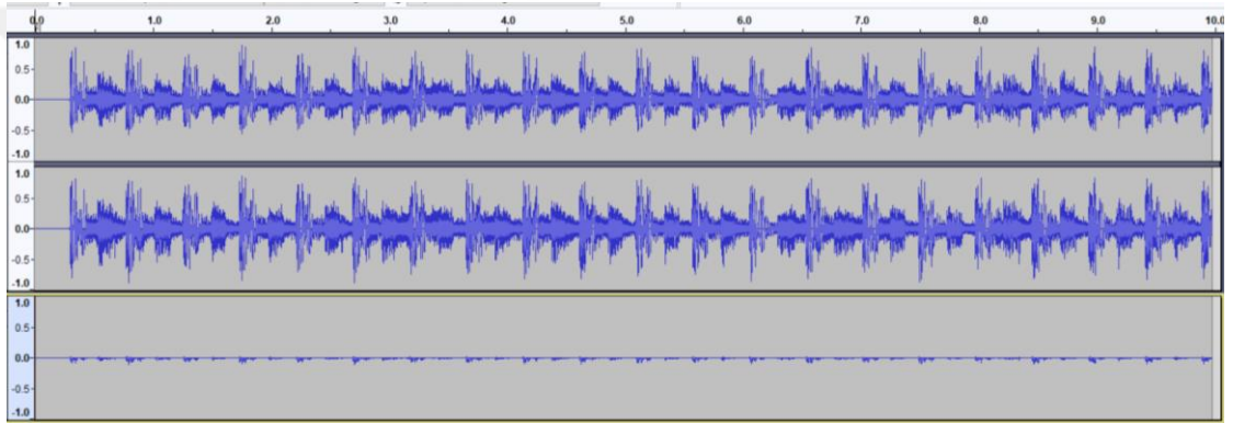
Şekil 8.4 FPGA AM verici sisteminin A2 modüle edici sinyaliyle yapılan simülasyon sonuçları: üstte A2 test sinyali, ortada modülasyonu takiben demodülasyonla elde edilen dalgaşekli, altta iki sinyalin farkı
