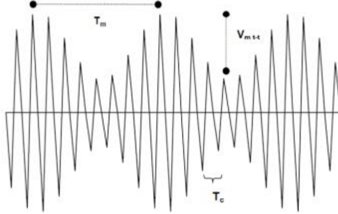
Şekil 4.5. Modüleli işarete bilgi işaretine ait büyüklükler
