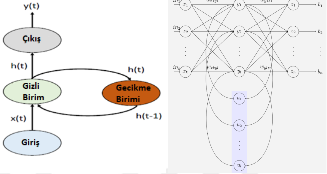
Şekil 4.24: a) Genelleştirilmiş Elman ağ yapısı, b) Katmanlı ağ yapısı.
