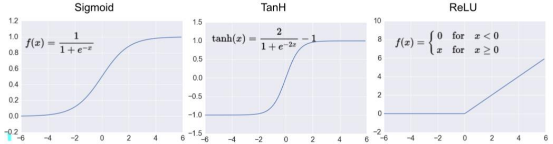
Şekil 4.12: En popüler üç aktivasyon fonksiyonunun grafikleri.
