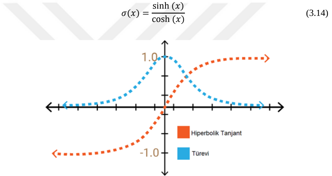
Şekil 3.7: Tanh fonksiyonunun ve türevinin grafiği.
