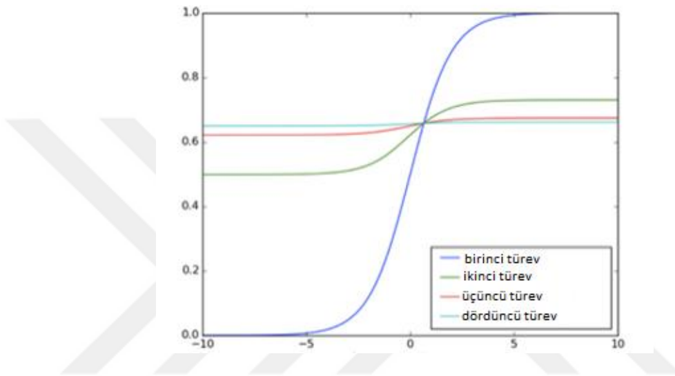
Şekil 4.26: Sigmoid aktivasyon fonksiyonunun türev ve bağlı değişimi.
