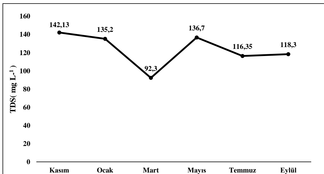
Şekil 4.11. Toplam çözünmüş katı madde değerinin mevsimsel değişimi
