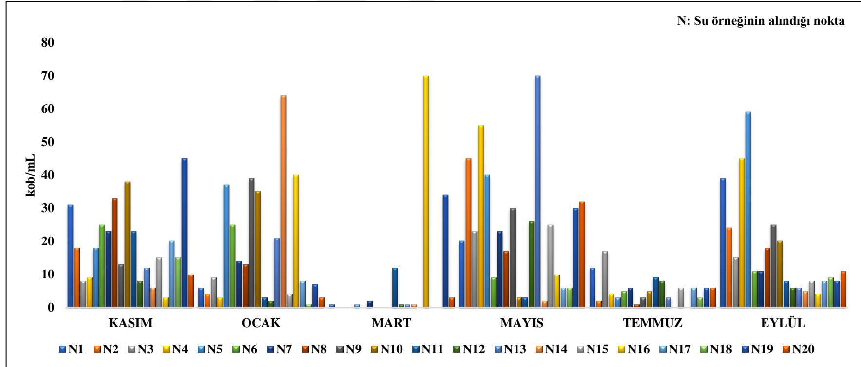
Şekil 4.4. Fekal koliform miktarının aylara göre dağılımı
