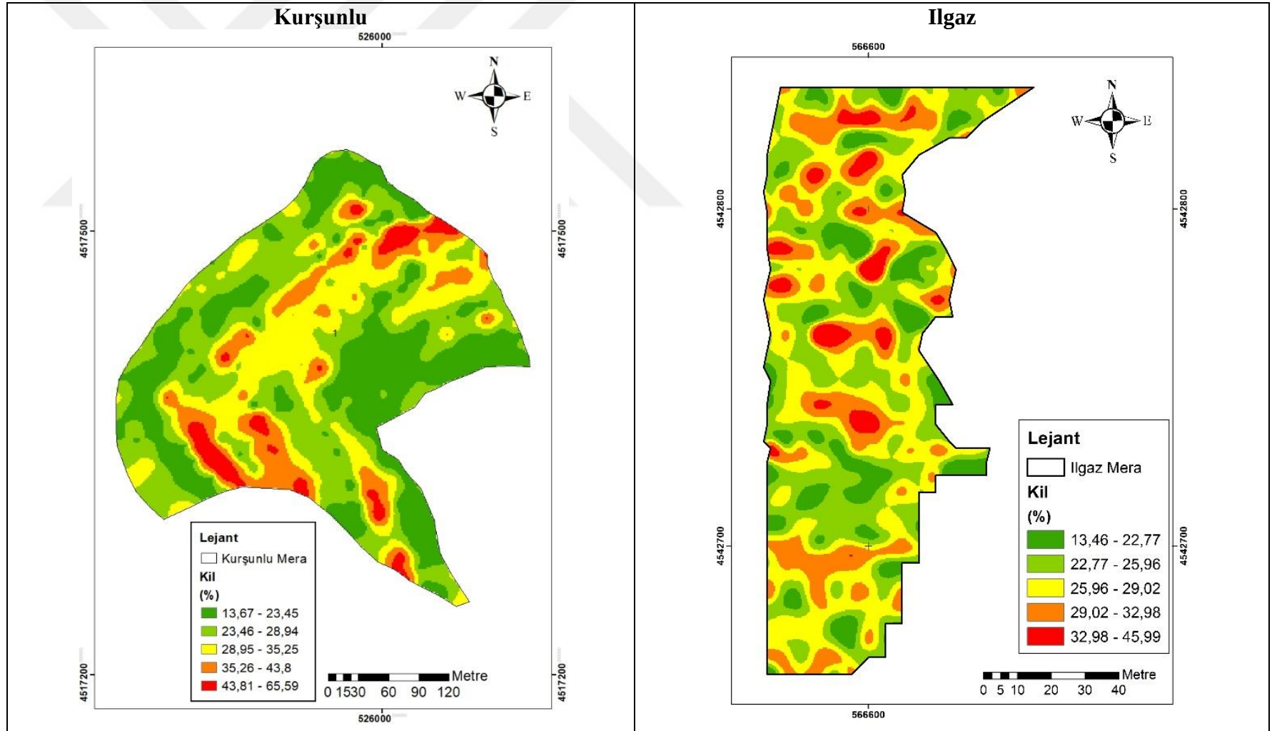
Şekil 4. 6 Kil içeriğinin mera topraklarında uzaysal değişim deseni
