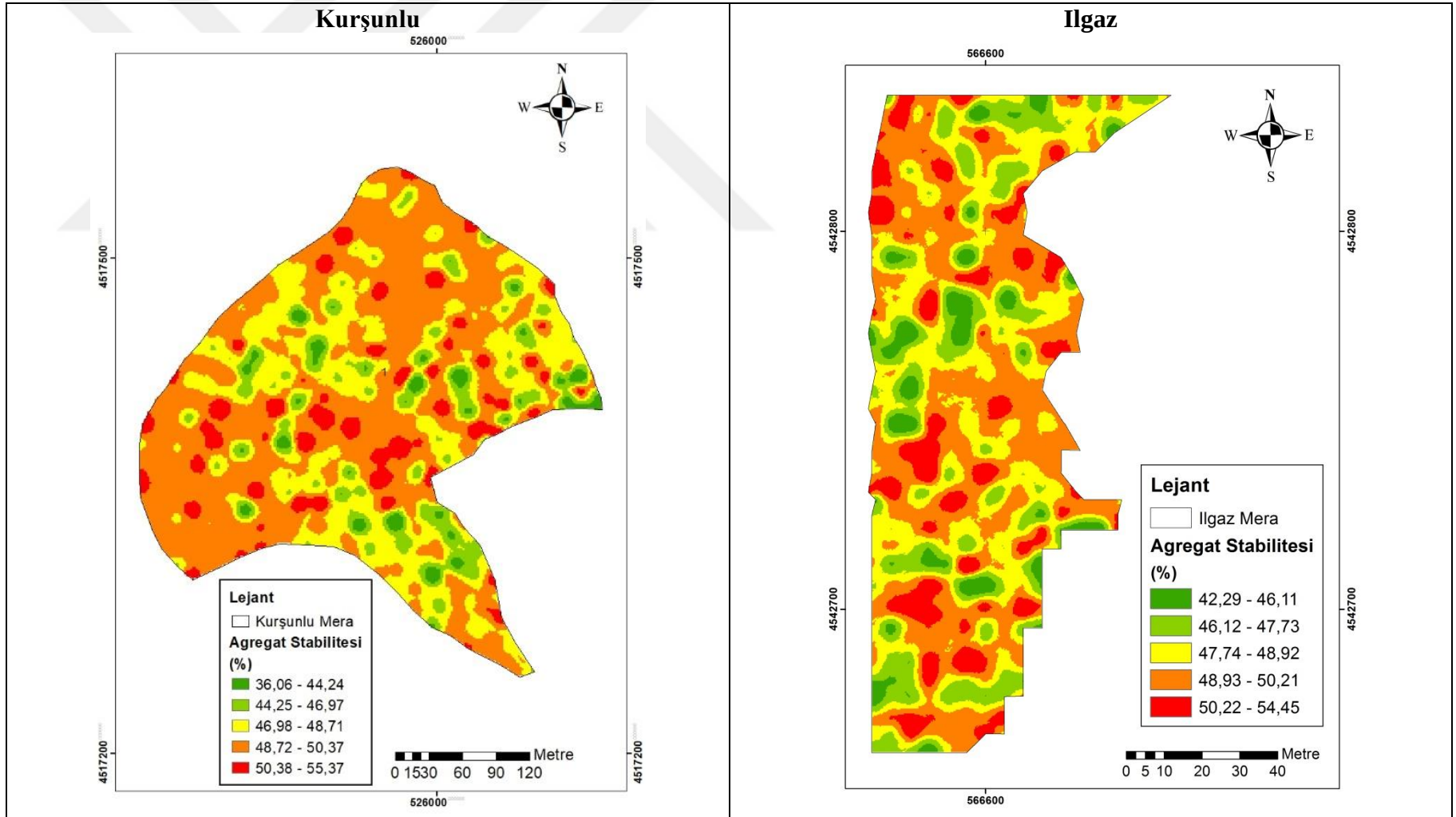
Şekil 4. 30 Agregat stabilitesinin mera topraklarında uzaysal değişim deseni
