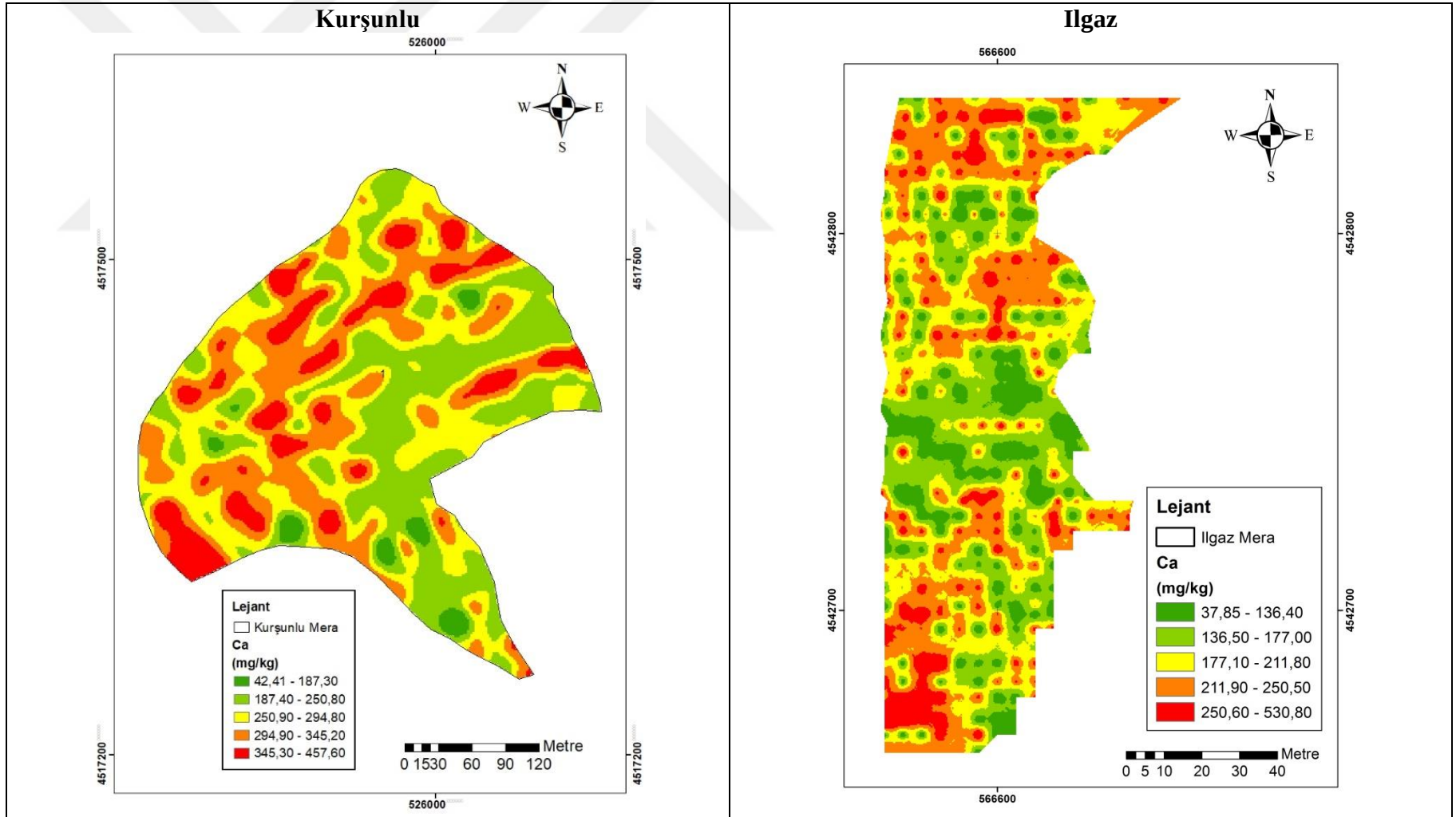
Şekil 4. 57 Kalsiyum (Ca) içeriğinin mera topraklarında uzaysal değişim deseni
