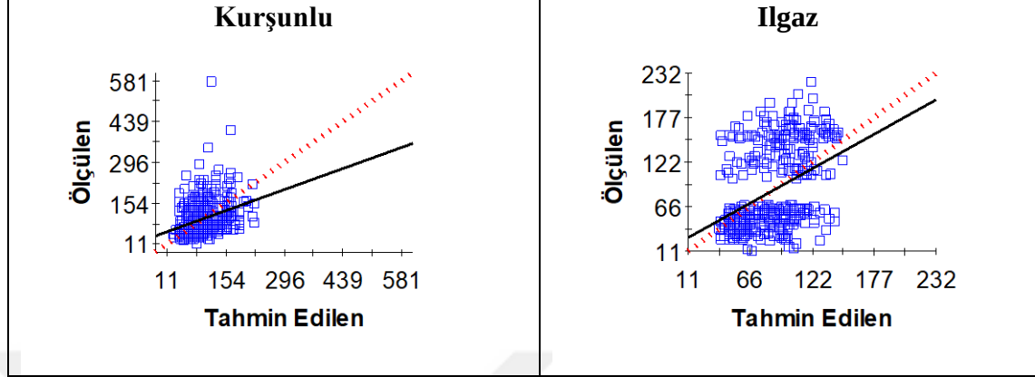
Şekil 4. 53 Mera topraklarının K içeriğine ilişkin çapraz doğrulama grafikleri
