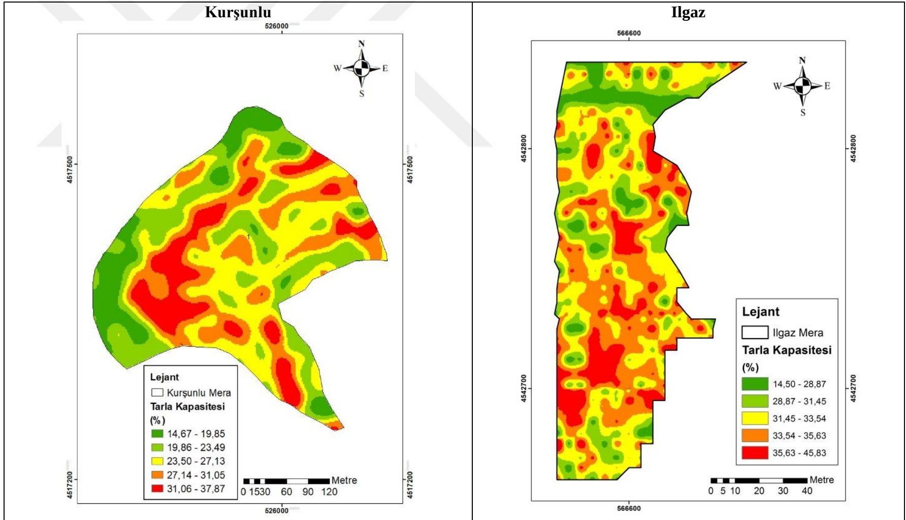
Şekil 4. 21 Tarla kapasitesinin mera topraklarında uzaysal değişim deseni
