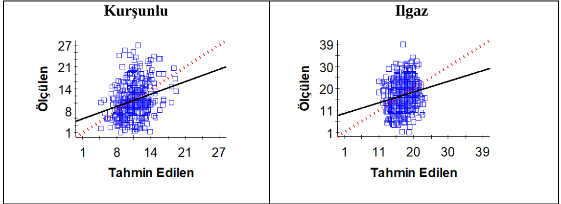
Şekil 4. 26 Mera topraklarının bitkiye yarayışlı su içeriğine ilişkin çapraz doğrulama grafikleri
