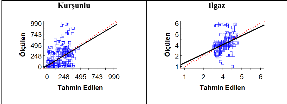
Şekil 4. 50 Mera topraklarının Na içeriğine ilişkin çapraz doğrulama grafikleri
