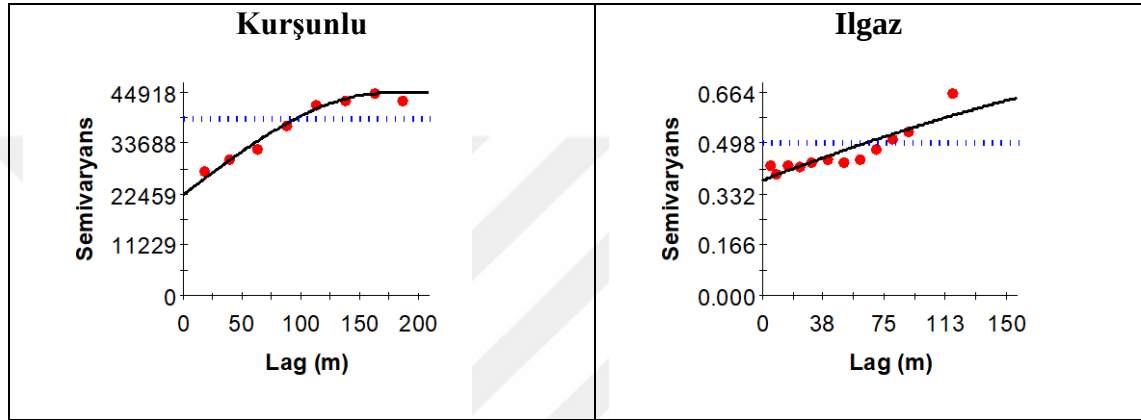
Şekil 4. 49 Meralarda toprakların Na içeriğine ilişkin deneysel (küre) ve teorik (çizgi) semivaryogramları
