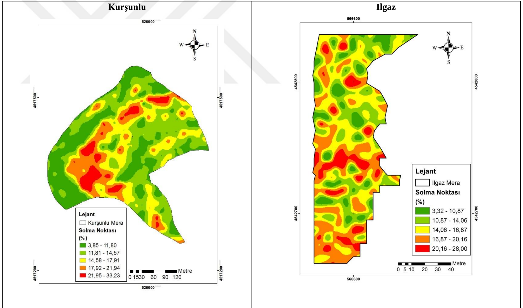
Şekil 4. 24 Solma noktasının mera topraklarında uzaysal değişim deseni
