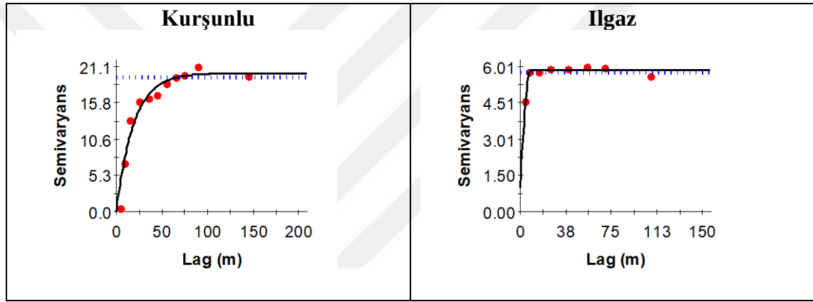
řekil 4. 46 Meralarda toprakların katyon deęiřim kapasitesine iliřkin deneysel (kre) ve teorik (izgi) semivaryogramları
