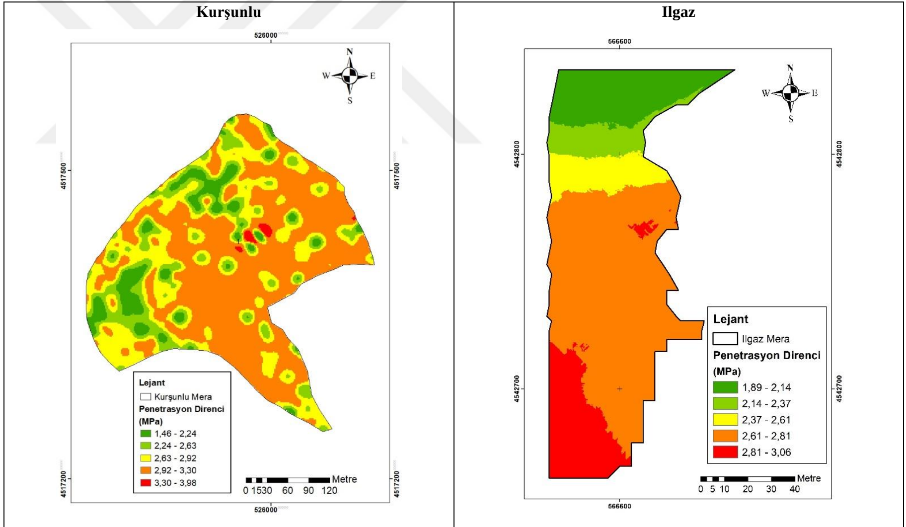
Şekil 4. 45 Penetrasyon direncinin mera topraklarında uzaysal değişim deseni
