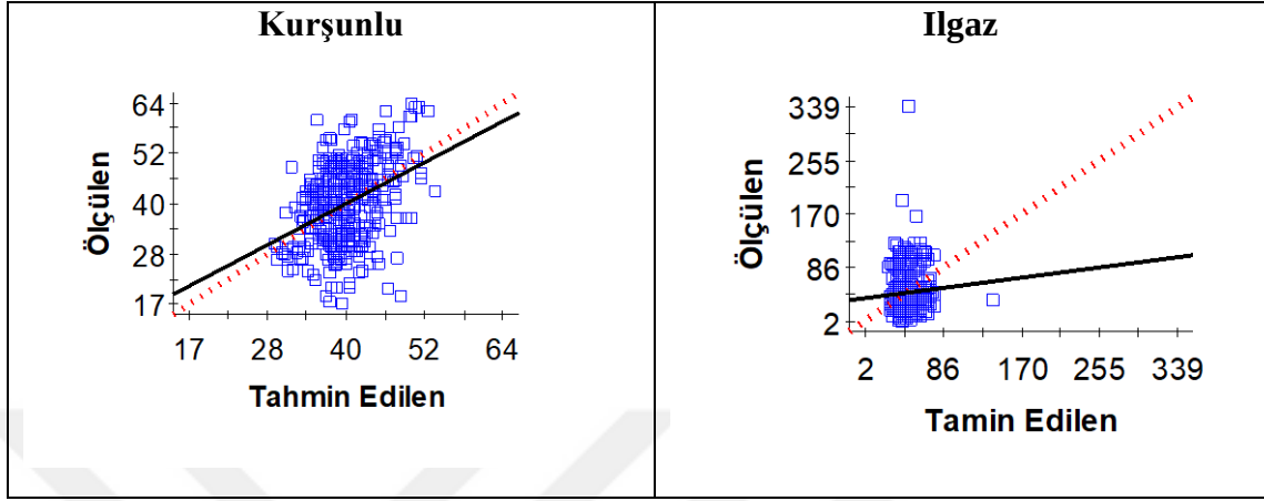
Şekil 4. 59 Mera topraklarının Mg içeriğine ilişkin çapraz doğrulama grafikleri
