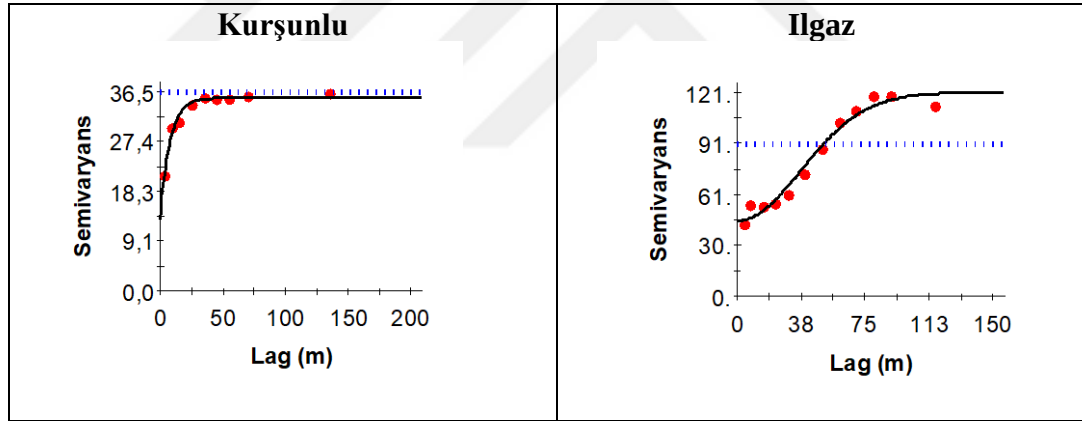
Şekil 4. 13 Meralarda toprakların örnekleme esnasında toprak su içeriğine ilişkin deneysel (küre) ve teorik (çizgi) semivaryogramları
