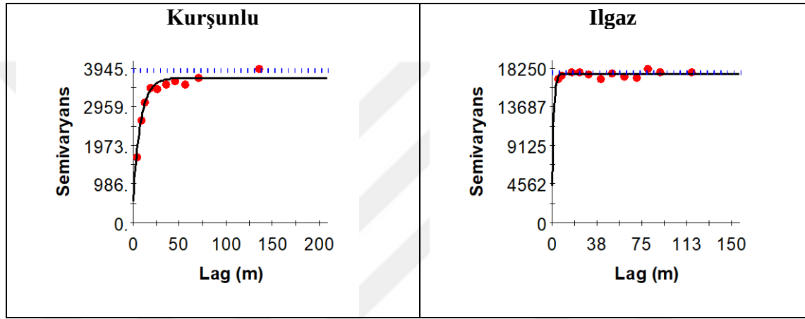
Şekil 4. 55 Meralarda toprakların Ca içeriğine ilişkin deneysel (küre) ve teorik (çizgi) semivaryogramları
