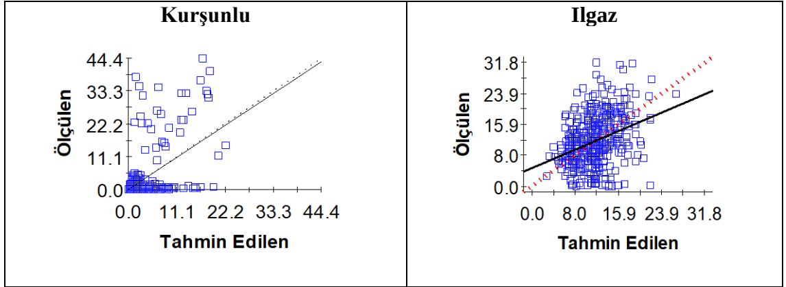
Şekil 4. 74 Mera toprakların Zn içeriğine ilişkin çapraz doğrulama grafikleri
