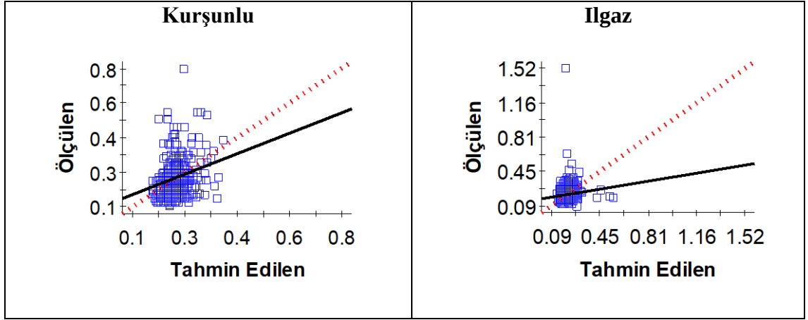
Şekil 4. 62 Mera toprakların P içeriğine ilişkin çapraz doğrulama grafiği
