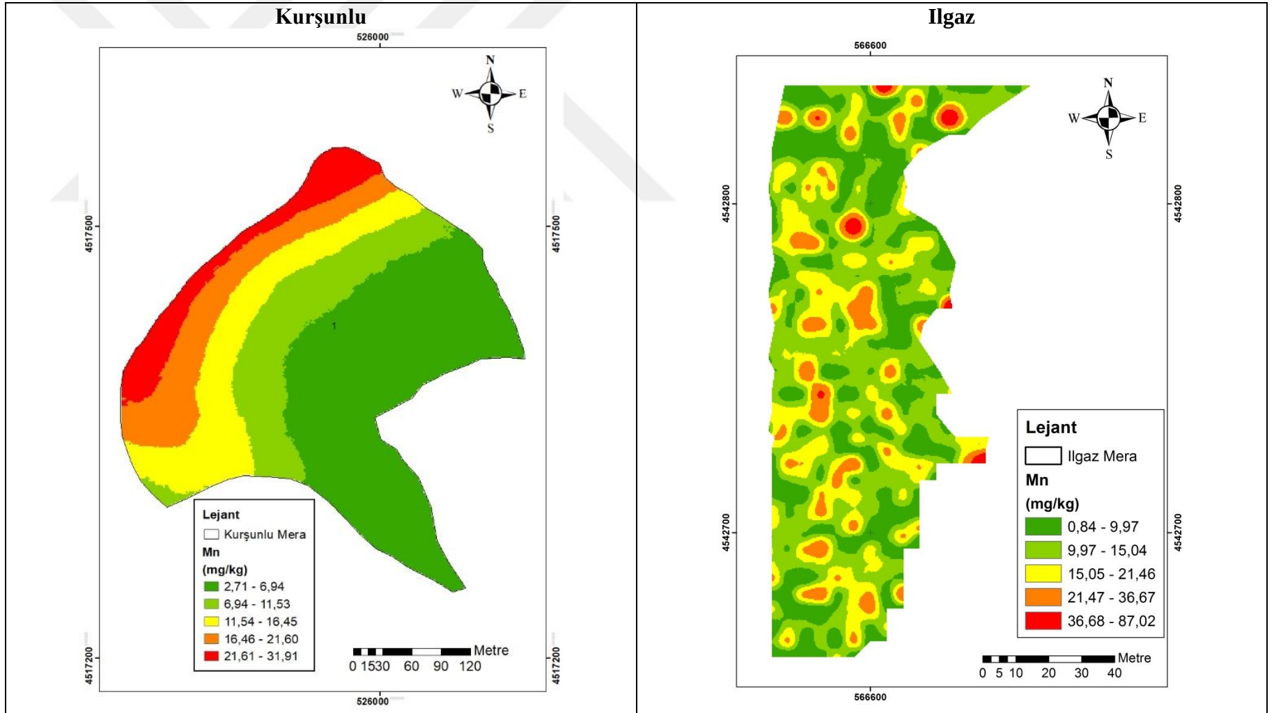
Şekil 4. 72 Manganez (Mn) içeriğinin mera topraklarında uzaysal değişim deseni
