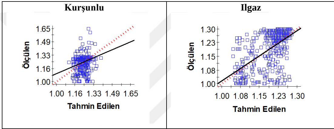
Şekil 4. 11 Mera topraklarının hacim ağırlığına ilişkin çapraz doğrulama grafikleri
