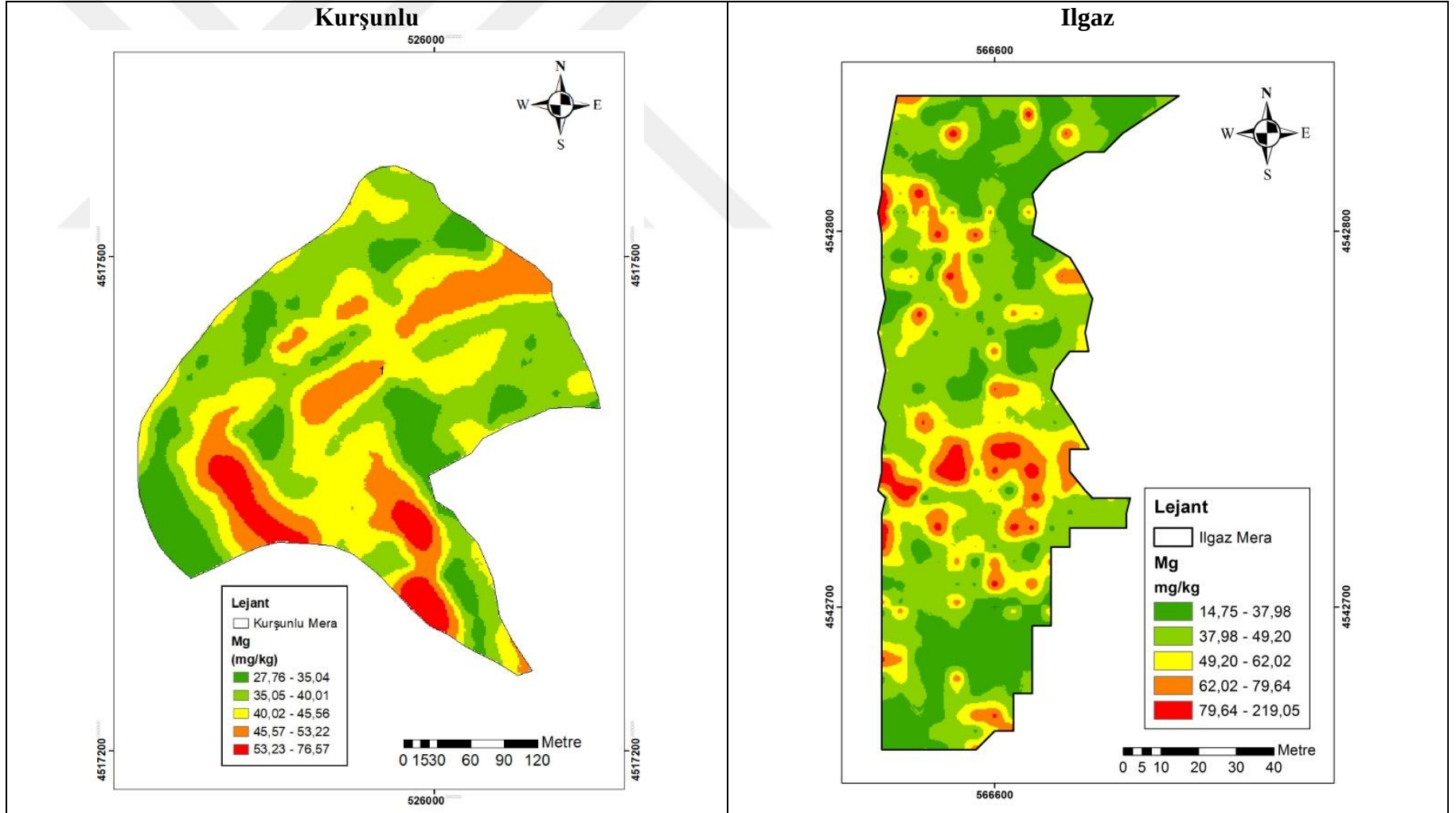
Şekil 4. 60 Magnezyum (Mg) içeriğinin mera topraklarında uzaysal değişim deseni
