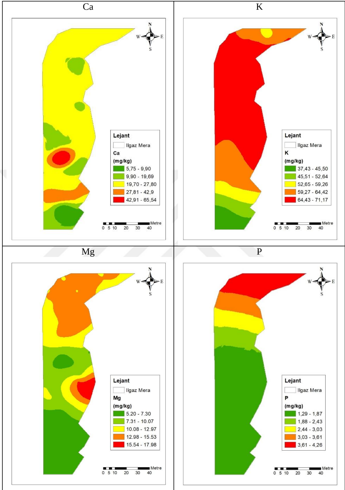
Şekil 4. 79 Ilgaz merasında bitki örneklerinin makro besin elementlerinin uzaysal değişim desenleri
