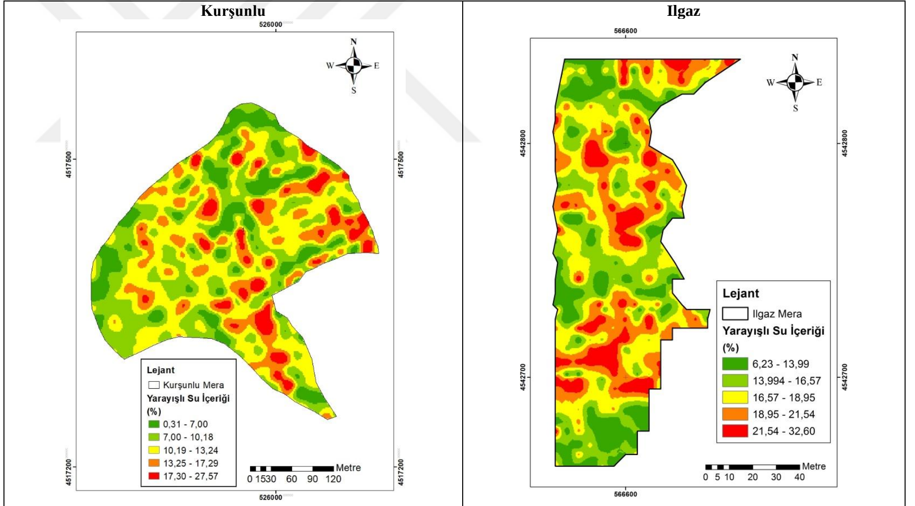
Şekil 4. 27 Bitkiye yarayırlı su içeriğinin mera topraklarında uzaysal değişim deseni
