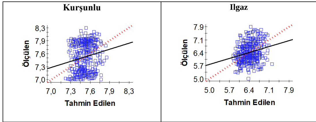
Şekil 4. 38 Mera topraklarının pH'sına ilişkin çapraz doğrulama grafikleri
