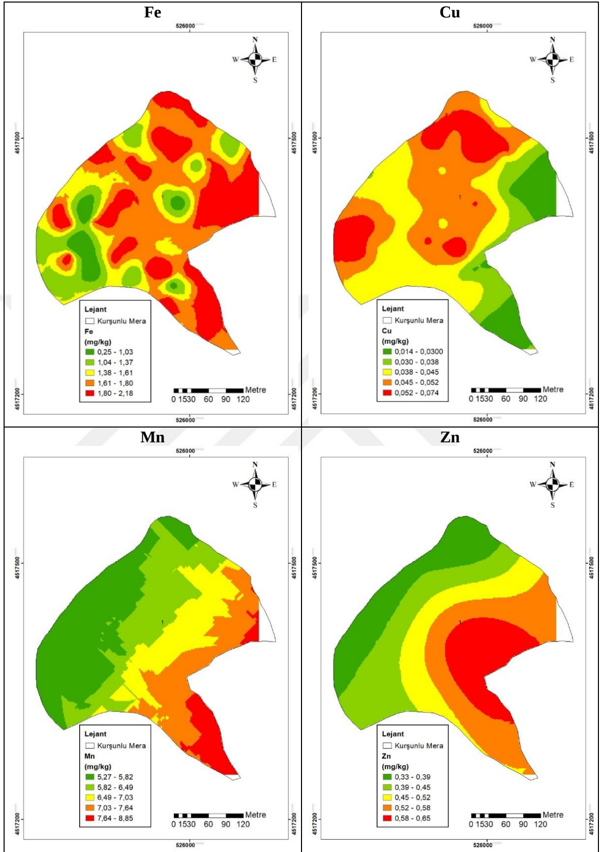
Şekil 4. 82 Kurşunlu merası bitki örneklerinin mikro besin elementlerinin uzaysal değişim desenleri
