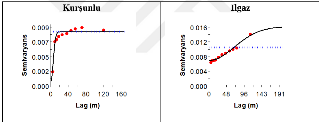
Şekil 4. 10 Meralarda toprakların hacim ağırlığına ilişkin deneysel (küre) ve teorik (çizgi) semivaryogramları
