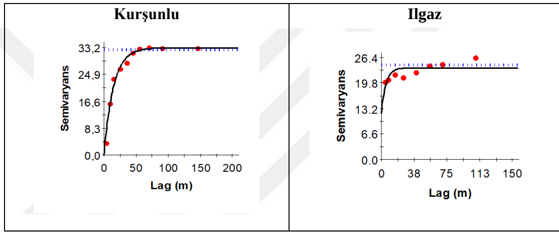
Şekil 4. 7 Meralarda toprakların silt içeriğine ilişkin deneysel (küre) ve teorik (çizgi) semivaryogramları
