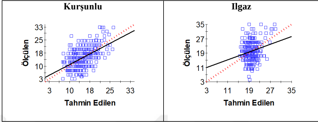
Şekil 4. 8 Mera topraklarının silt içeriğine ilişkin çapraz doğrulama grafiği
