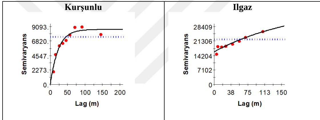
Şekil 4. 40 Meralarda toprakların elektriksel iletkenliğe ilişkin deneysel (küre) ve teorik (çizgi) semivaryogramları
