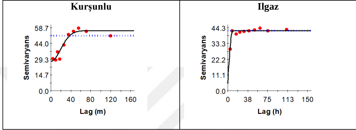
Şekil 4. 73 Meralarda toprakların Zn içeriğine ilişkin deneysel (küre) ve teorik (çizgi) semivaryogramları
