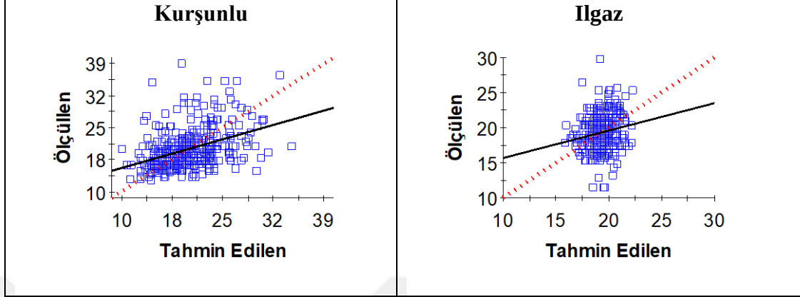
Şekil 4. 47 Mera topraklarının katyon değişim kapasitesine ilişkin çapraz doğrulama grafikleri
