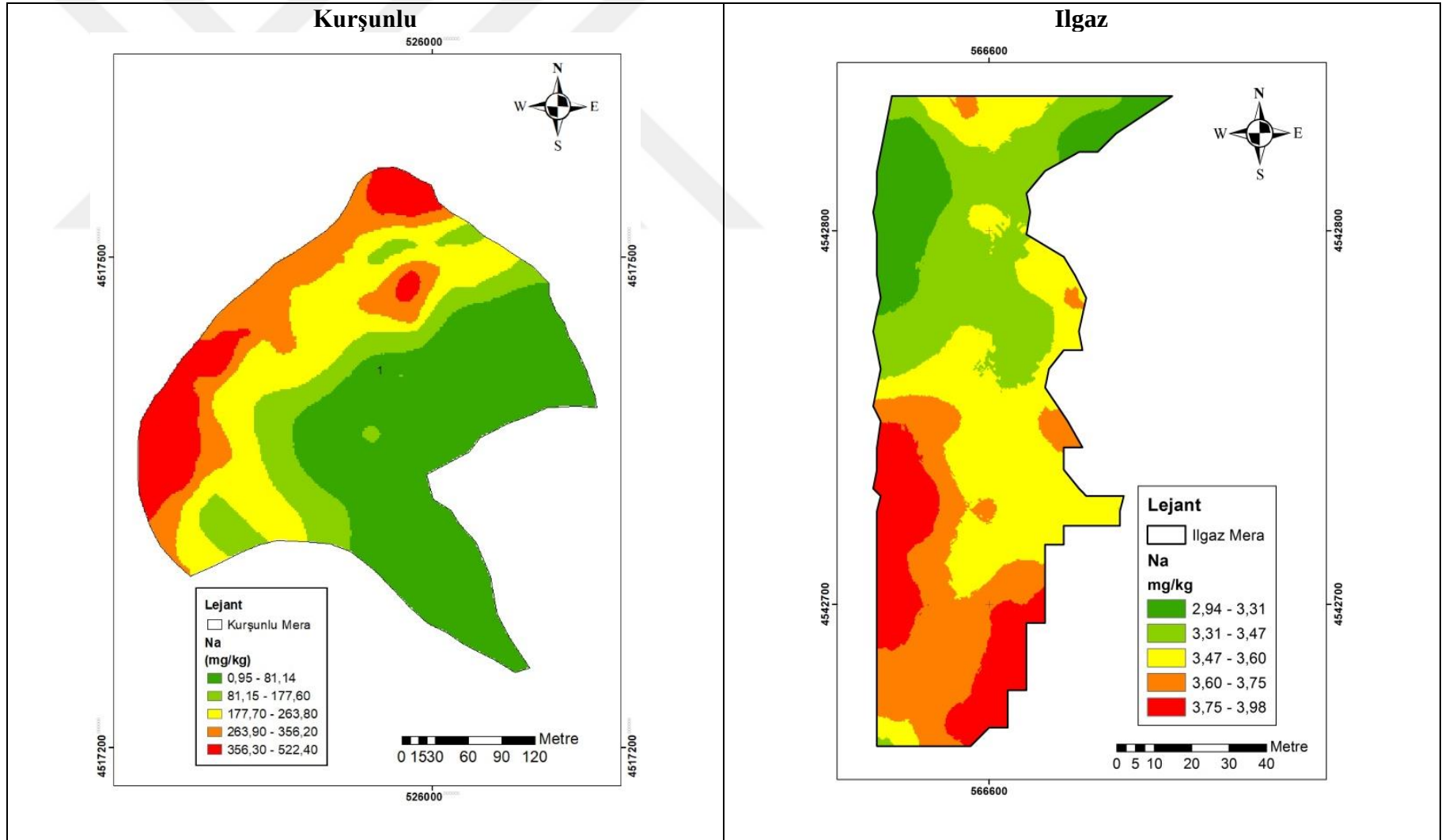
Şekil 4. 51 Sodyum (Na) içeriğinin mera topraklarında uzaysal değişim deseni
