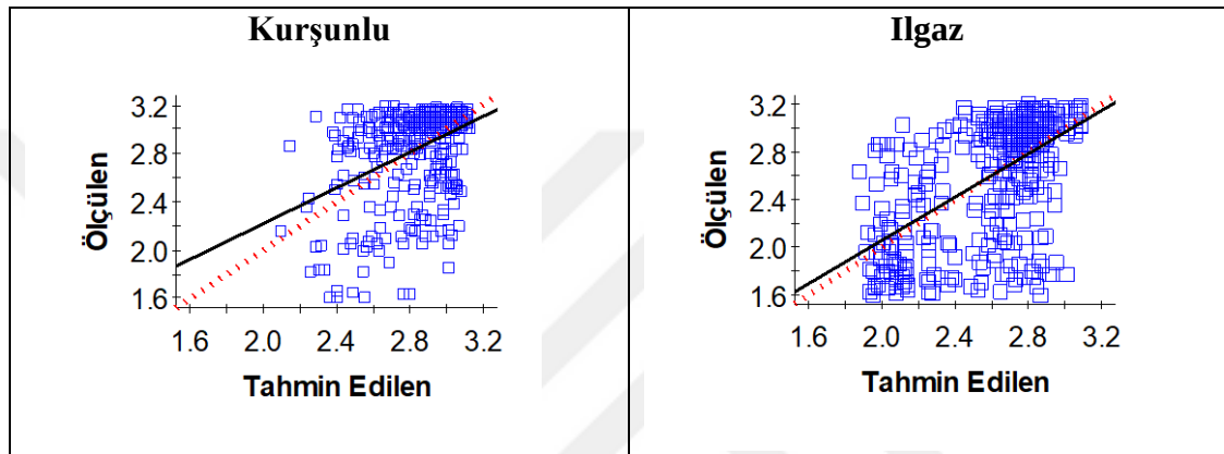
Şekil 4. 44 Mera topraklarının penetrasyon direncine ilişkin çapraz doğrulama grafikleri
