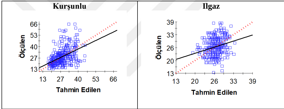
Şekil 4. 5 Mera topraklarının kil içeriğine ilişkin çapraz doğrulama grafiği
