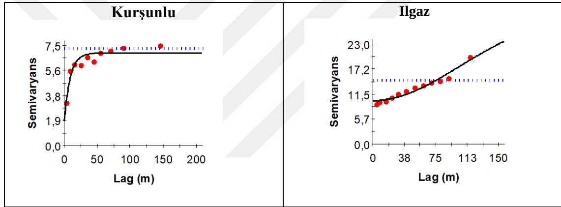
Şekil 4. 16 Meralarda toprak gözenekliliğine ilişkin deneysel (küre) ve teorik (çizgi) semivaryogramları
