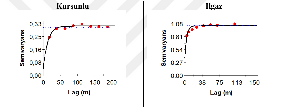
Şekil 4. 34 Meralarda toprakların organik madde içeriğine ilişkin deneysel (küre) ve teorik (çizgi) semivaryogramları
