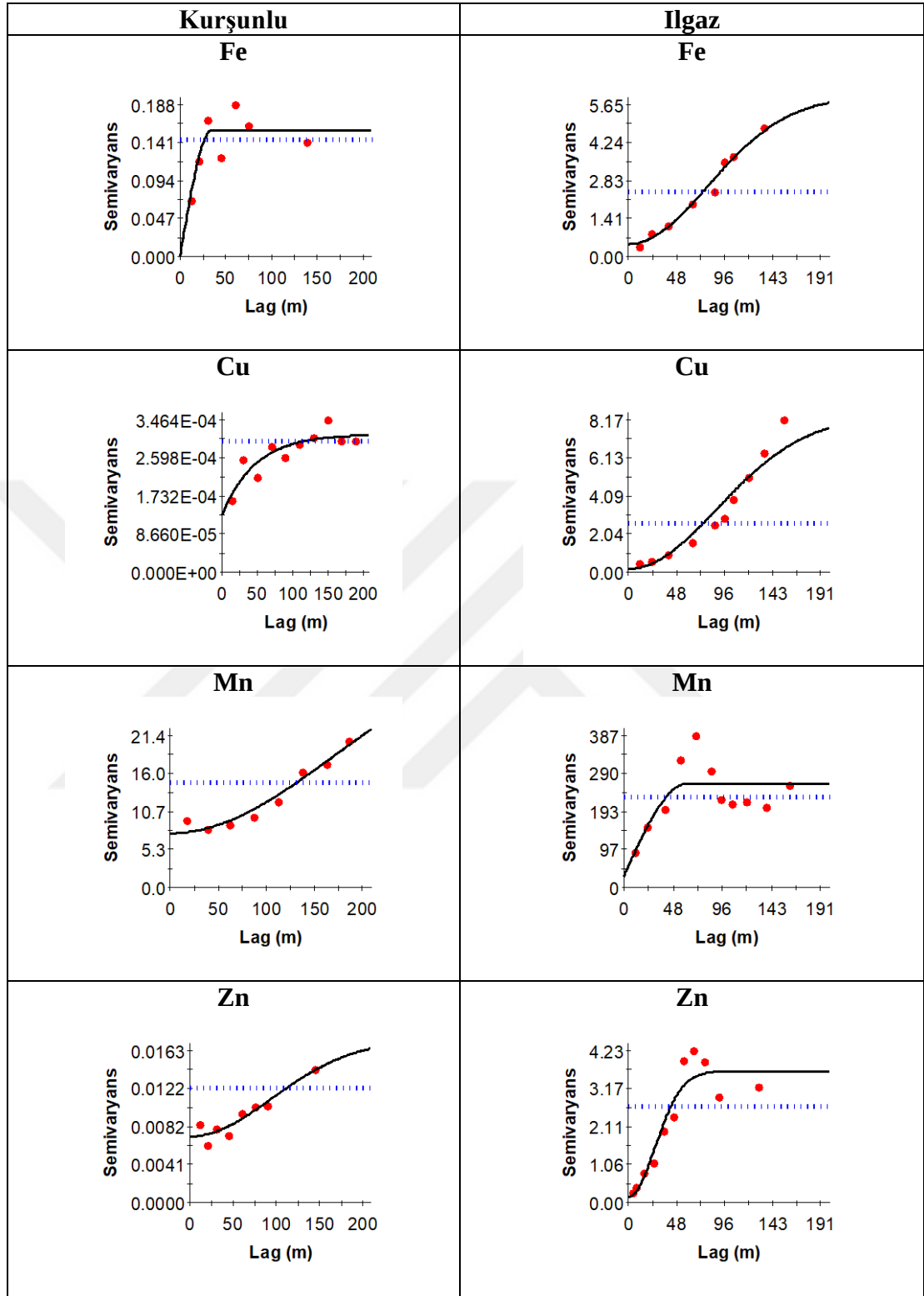
Şekil 4. 80 Mera bitki örneklerinin mikro besin elementleri içeriklerine ilişkin ilişkili deneysel (küre) ve teorik (çizgi) semivaryogramları
