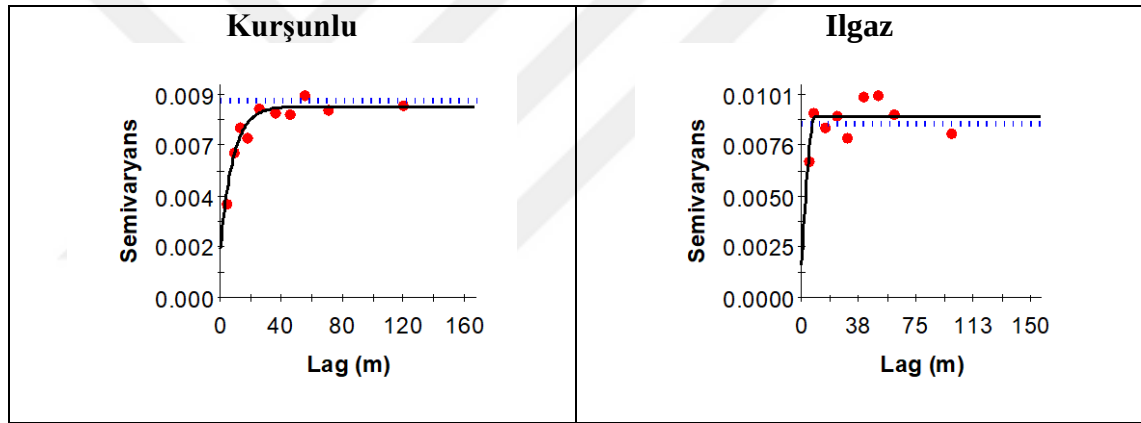
Şekil 4. 61 Meralarda toprakların P içeriğine ilişkin deneysel (küre) ve teorik (çizgi) semivaryogramları
