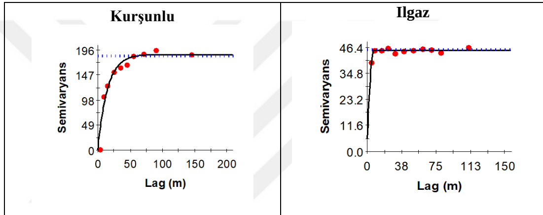
Şekil 4. 1 Meralarda toprakların kum içeriğine ilişkin deneysel (küre) ve teorik (çizgi) semivaryogramları
