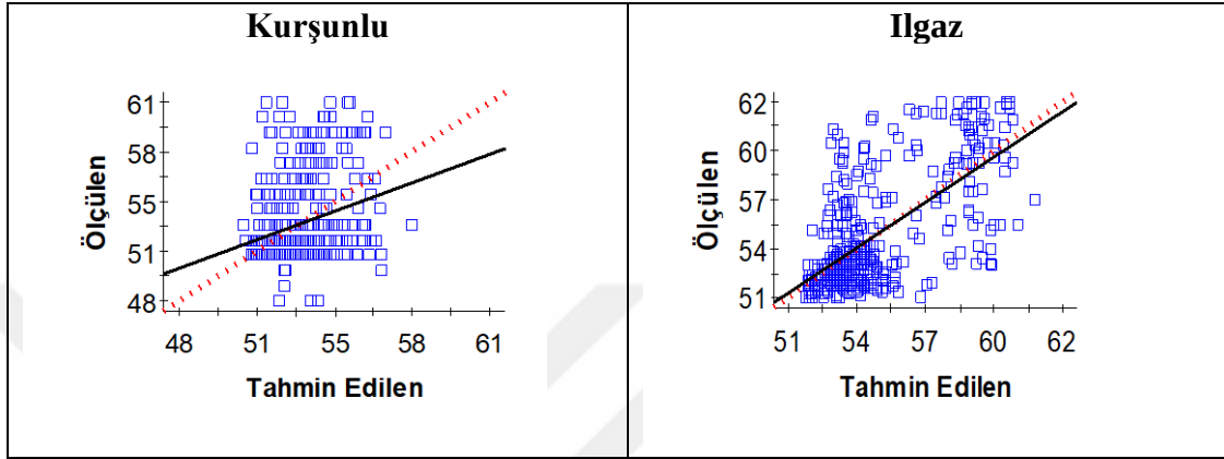
Şekil 4. 17 Mera toprak gözenekliliğine ilişkin çapraz doğrulama grafikleri
