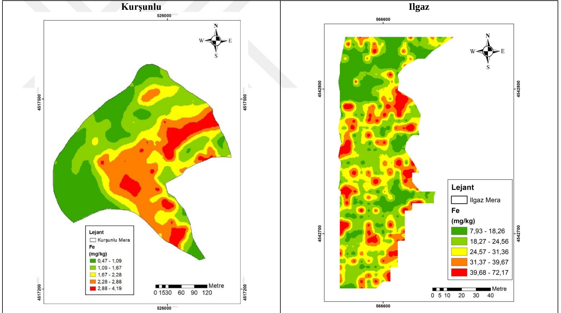
Şekil 4. 66 Demir (Fe) içeriğinin mera topraklarında uzaysal değişim deseni
