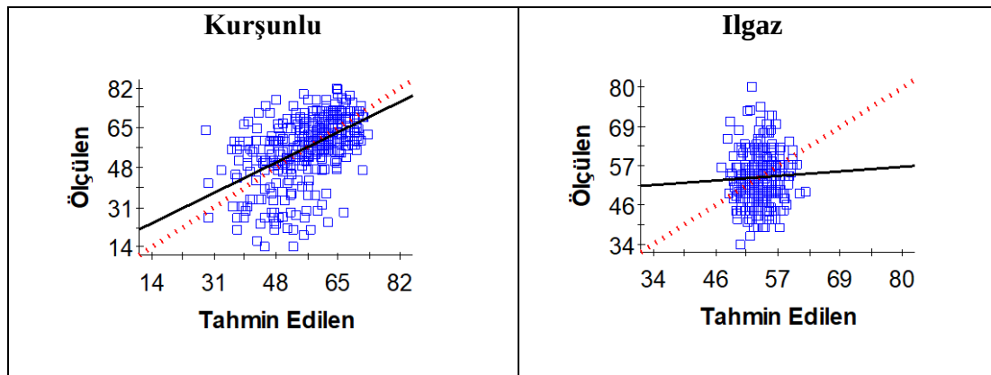
Şekil 4. 2 Mera topraklarının kum içeriğine ilişkin çapraz doğrulama grafiği
