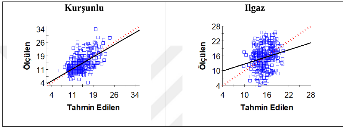
Şekil 4. 23 Mera topraklarının solma noktasına ilişkin çapraz doğrulama grafikleri
