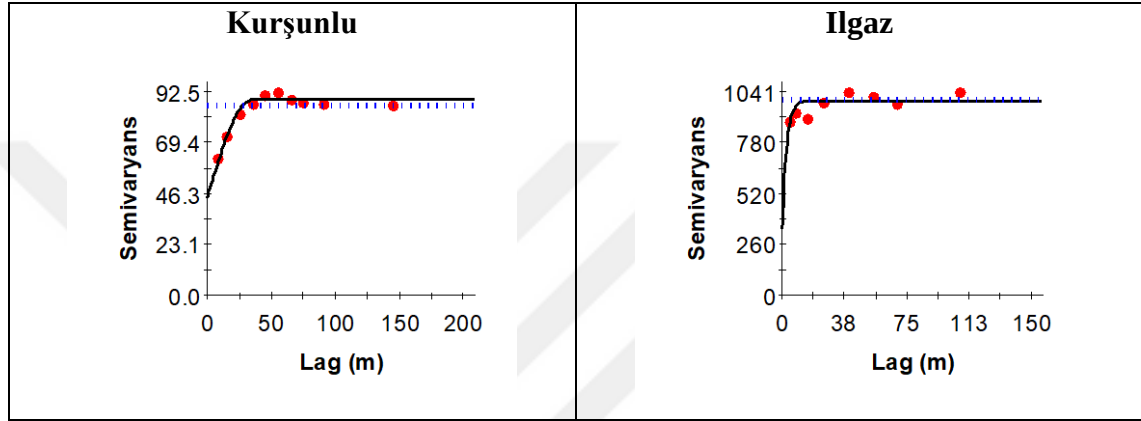
Şekil 4. 58 Meralarda toprakların Mg içeriğine ilişkin deneysel (küre) ve teorik (çizgi) semivaryogramları
