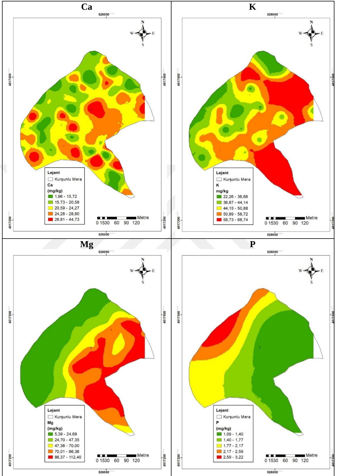
Şekil 4. 78 Kurşunlu merasında bitki örneklerinin makro besin elementlerinin uzaysal değişim desenleri
