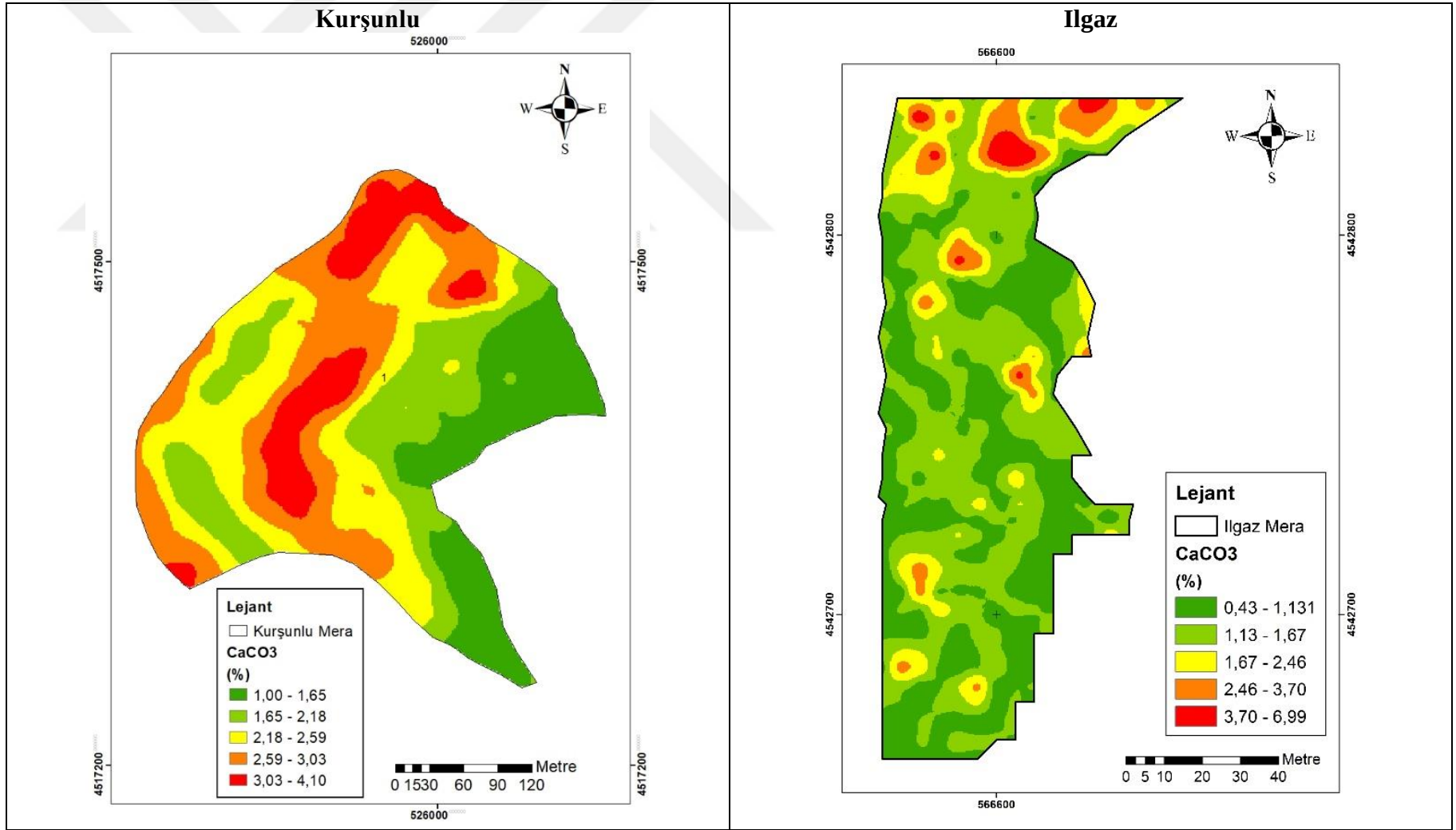
Şekil 4. 33 % \text{CaCO}_3 içeriğinin mera topraklarında uzaysal değişim deseni
