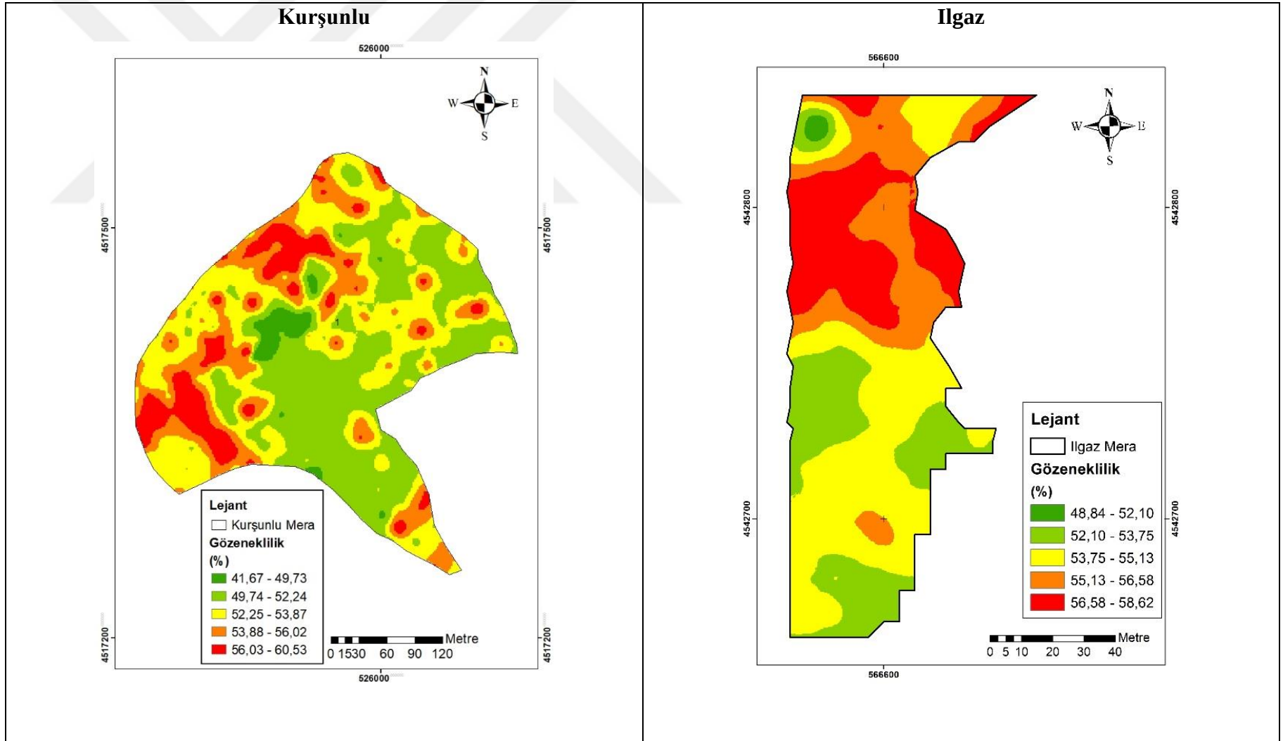
Şekil 4. 18 Toplam gözenekliliğin meralarda uzaysal değişim deseni
