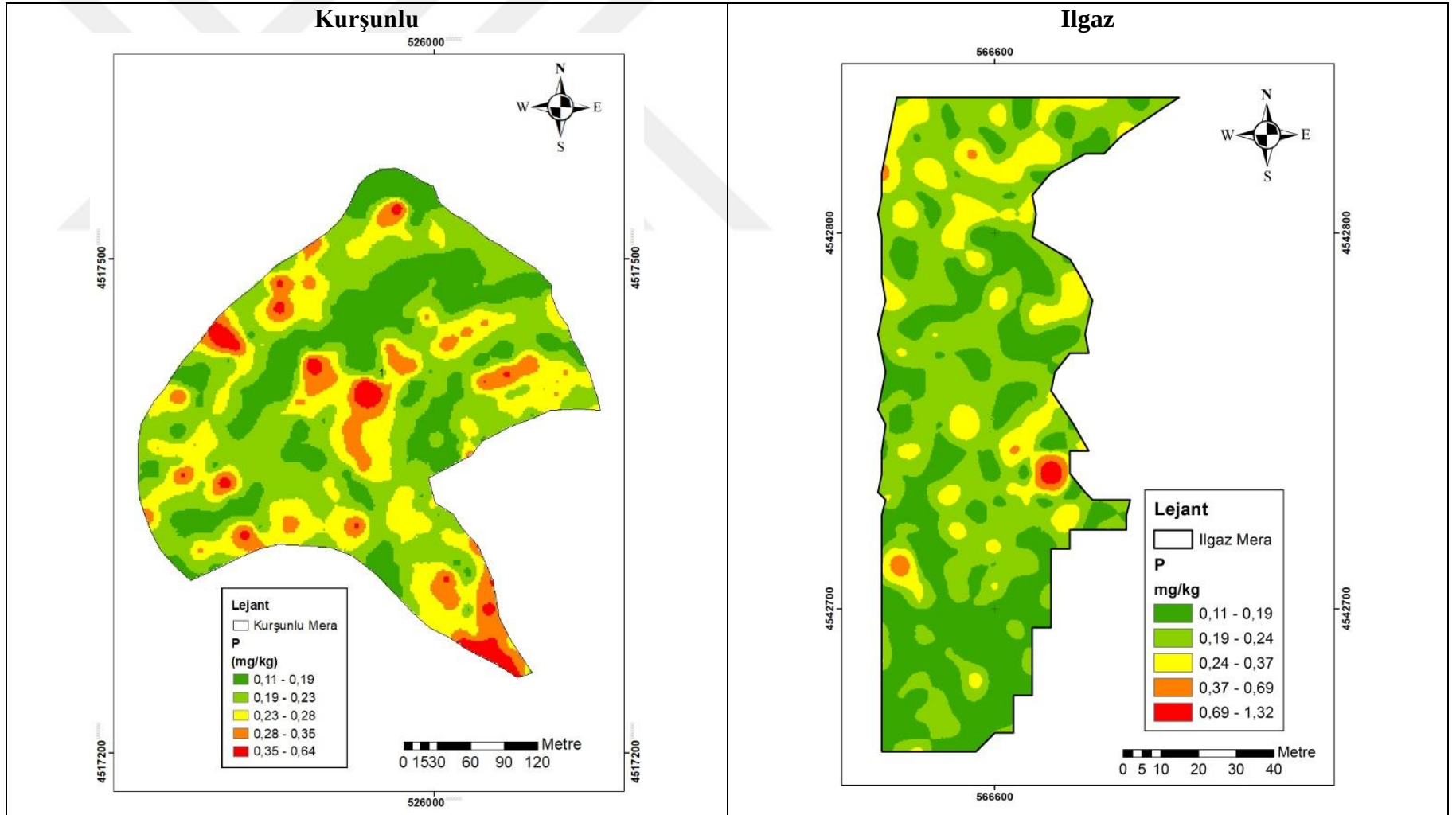
Şekil 4. 63 Fosfor (P) içeriğinin mera topraklarında uzaysal değişim deseni
