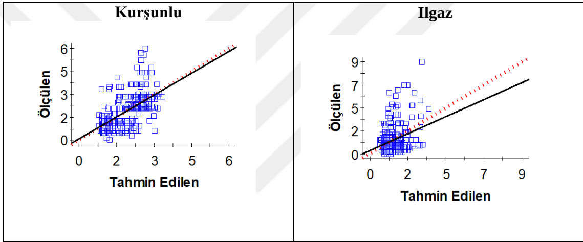
Şekil 4.32 Mera topraklarının \text{CaCO}_3 içeriğine ilişkin çapraz doğrulama grafikleri
