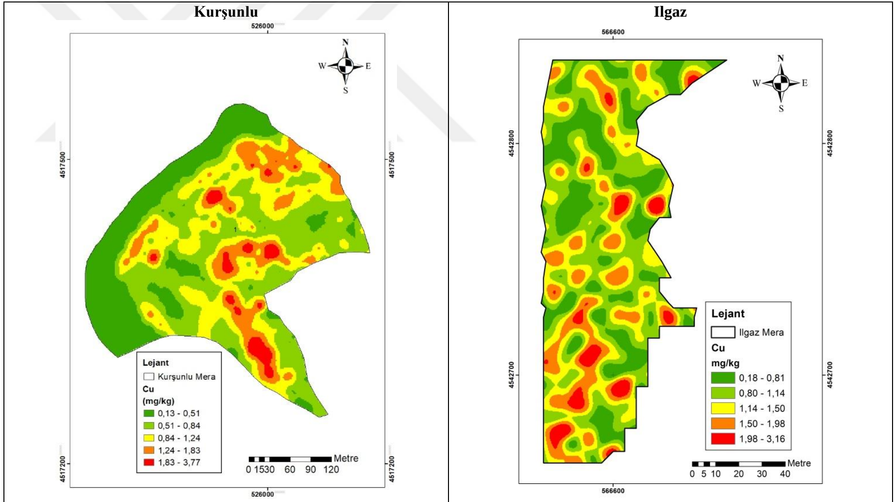
Şekil 4. 69 Bakır (Cu) içeriğinin mera topraklarında uzaysal değişim deseni
