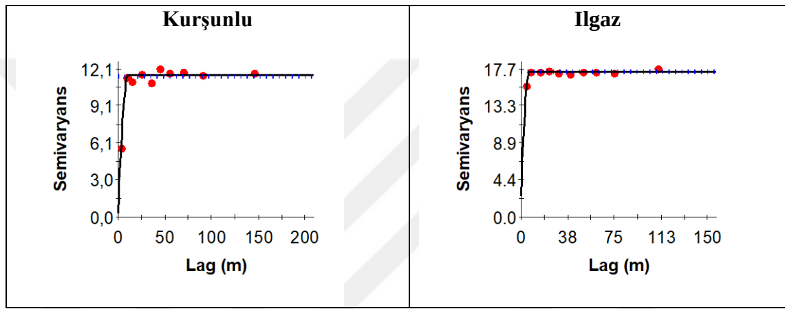
Şekil 4. 28 Mera toprakların agregat stabilitesine ilişkin deneysel (küre) ve teorik (çizgi) semivaryogramları
