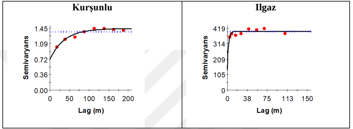
Şekil 4. 64 Meralarda toprakların Fe içeriğine ilişkin deneysel (küre) ve teorik (çizgi) semivaryogramları
