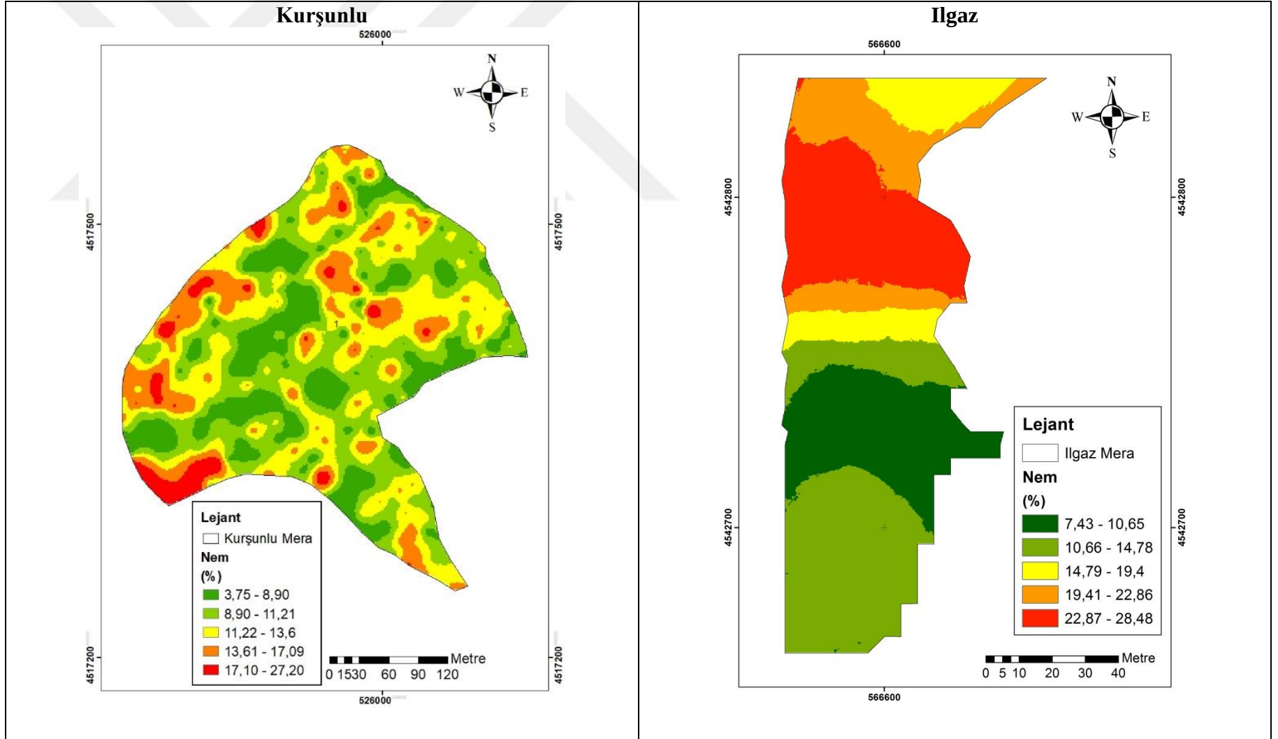
Şekil 4. 15 Örnekleme esnasında toprak su içeriğinin mera topraklarında uzaysal değişim deseni
