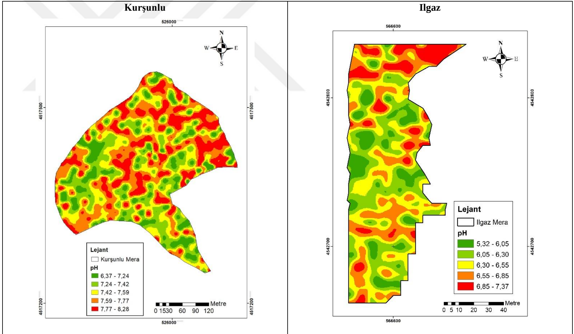
Şekil 4. 39 pH'nın mera topraklarında uzaysal değişim deseni
