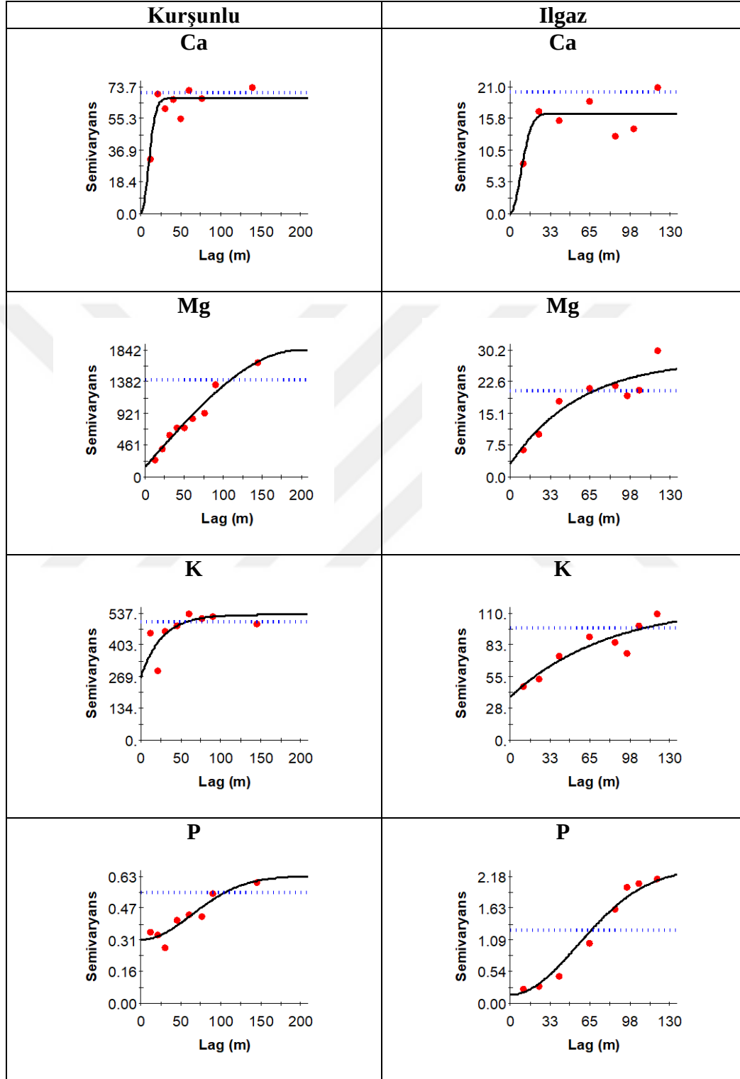
Şekil 4. 76 Mera bitki örneklerindeki makro besin elementi içeriklerine ilişkin deneysel (küre) ve teorik (çizgi) semivaryogramları
