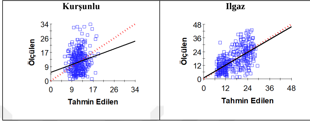
Şekil 4. 14 Mera topraklarının örnekleme esnasında toprak su içeriğine ilişkin çapraz doğrulama grafikleri
