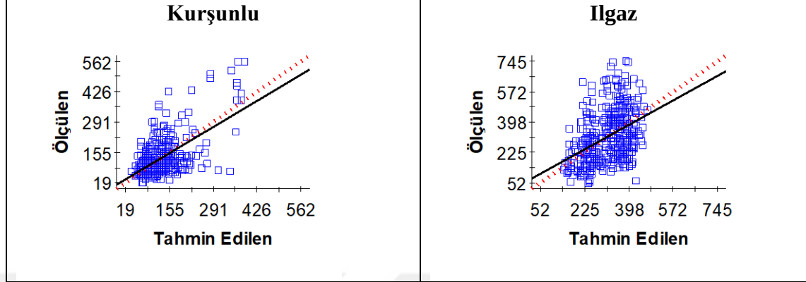
Şekil 4. 41 Mera topraklarının elektriksel iletkenliğe ilişkin çapraz doğrulama grafikleri
