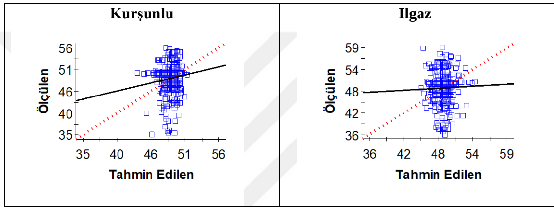
Şekil 4. 29 Mera topraklarının agregat stabilitesine ilişkin çapraz doğrulama grafikleri
