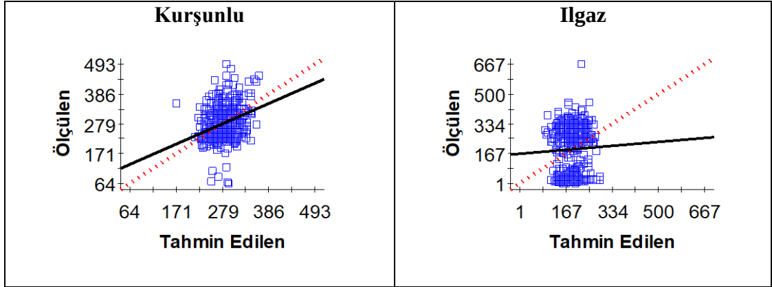
Şekil 4. 56 Mera topraklarının Ca içeriğine ilişkin çapraz doğrulama grafikleri
