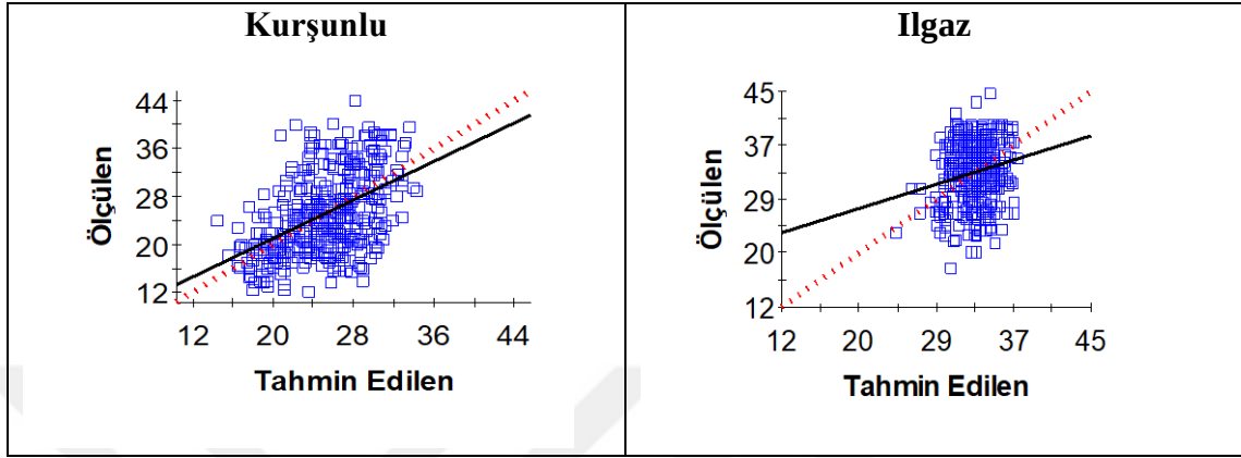
Şekil 4. 20 Mera topraklarının tarla kapasitesine ilişkin çapraz doğrulama grafikleri
