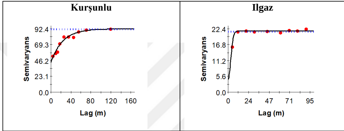
Şekil 4. 4 Meralarda toprakların kil içeriğine ilişkin deneysel (küre) ve teorik (çizgi) semivaryogramları
