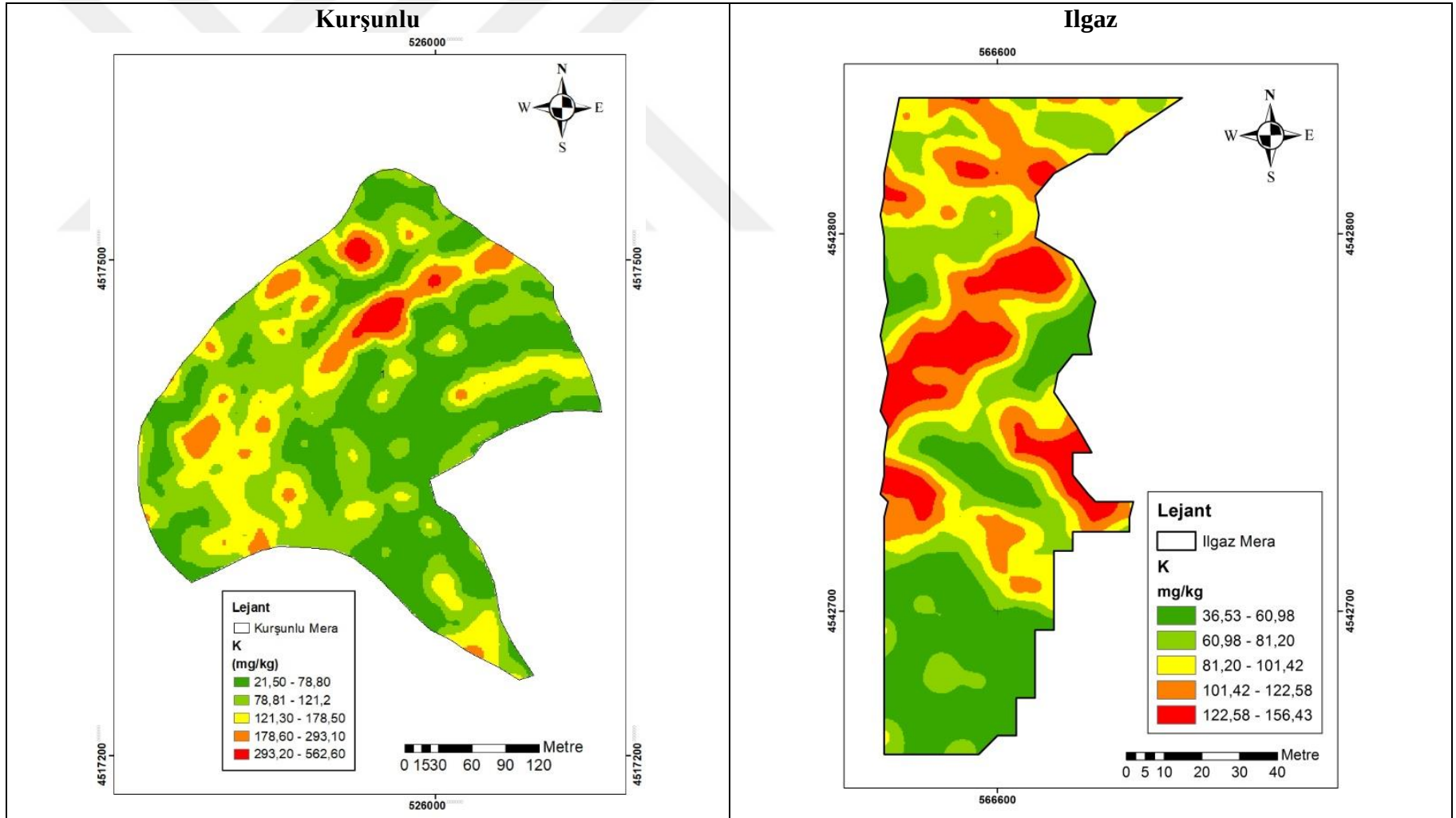
Şekil 4. 54 Potasyum (K) içeriğinin mera topraklarında uzaysal değişim deseni
