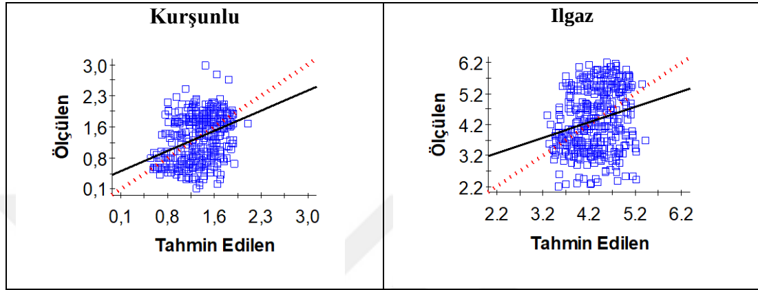
Şekil 4. 35 Mera topraklarının organik madde içeriğine ilişkin çapraz doğrulama grafikleri
