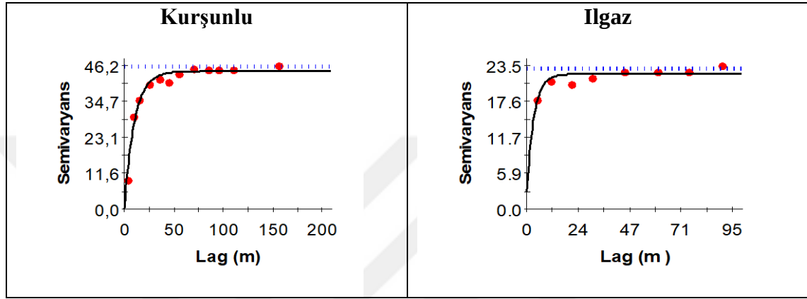
Şekil 4. 19 Meralarda toprakların tarla kapasitesine ilişkin deneysel (küre) ve teorik (çizgi) semivaryogramları
