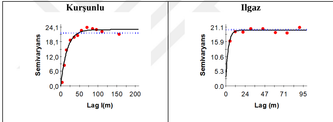
Şekil 4. 22 Meralarda toprakların solma noktasına ilişkin deneysel (küre) ve teorik (çizgi) semivaryogramları
