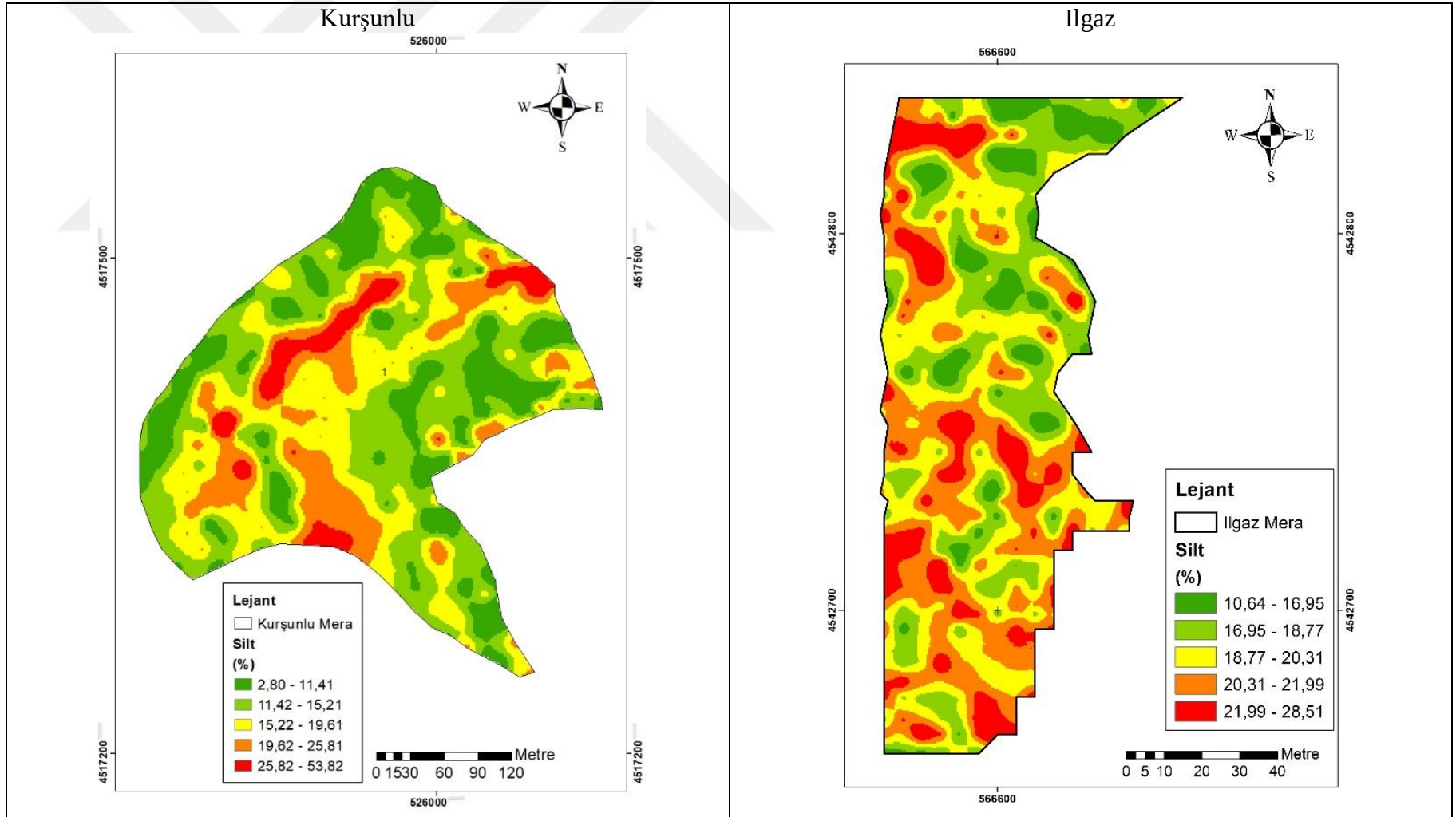
Şekil 4. 9 Silt içeriğinin mera topraklarında uzaysal değişim deseni
