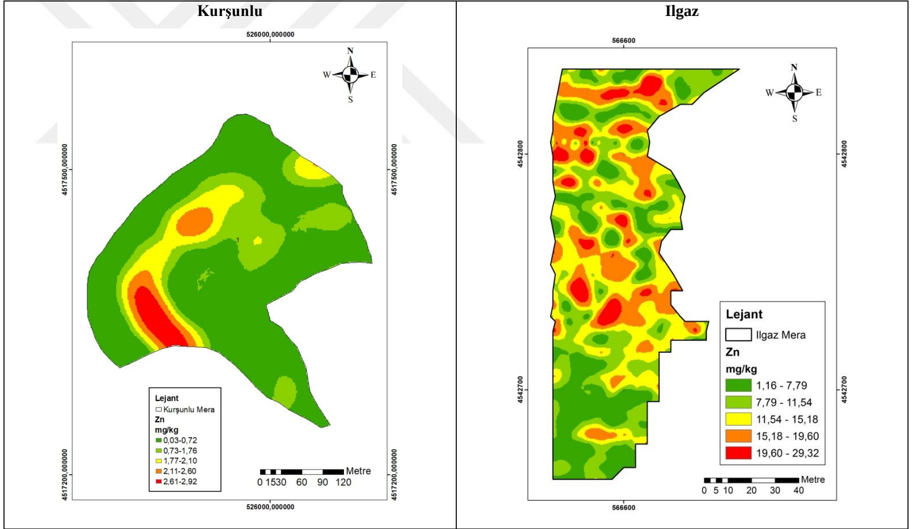
Şekil 4. 75 Çinko (Zn) içeriğinin mera topraklarında uzaysal değişim deseni
