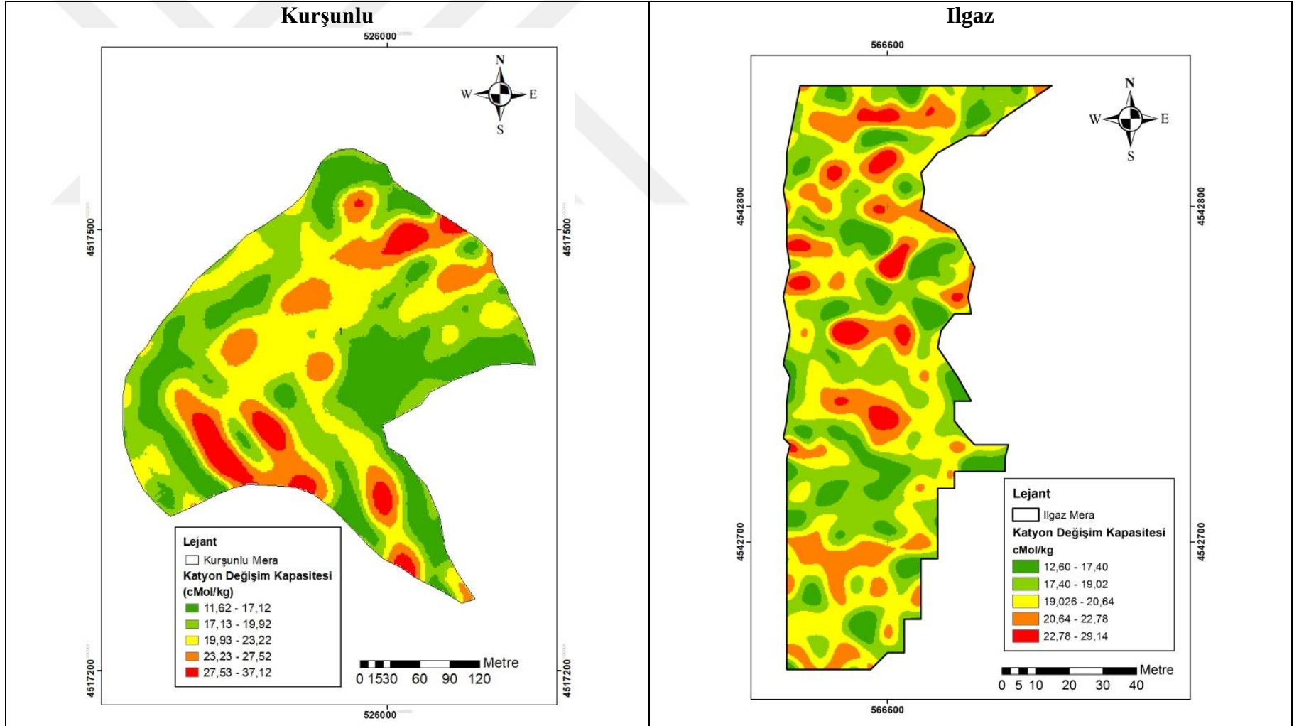
Şekil 4. 48 Kasyon değişim kapasitesinin mera topraklarında uzaysal değişim deseni
