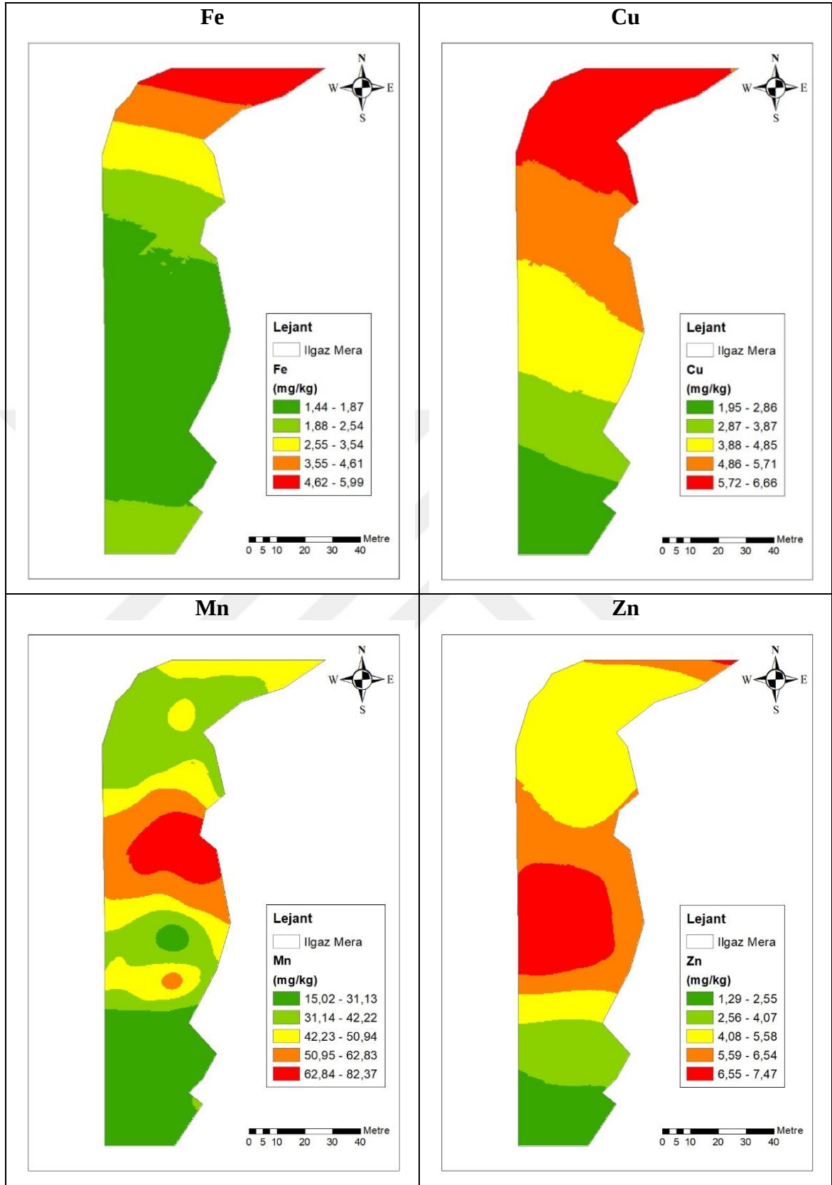
Şekil 4. 83 Ilgaz merası bitki örneklerinin mikro besin elementlerinin uzaysal değişim desenleri
