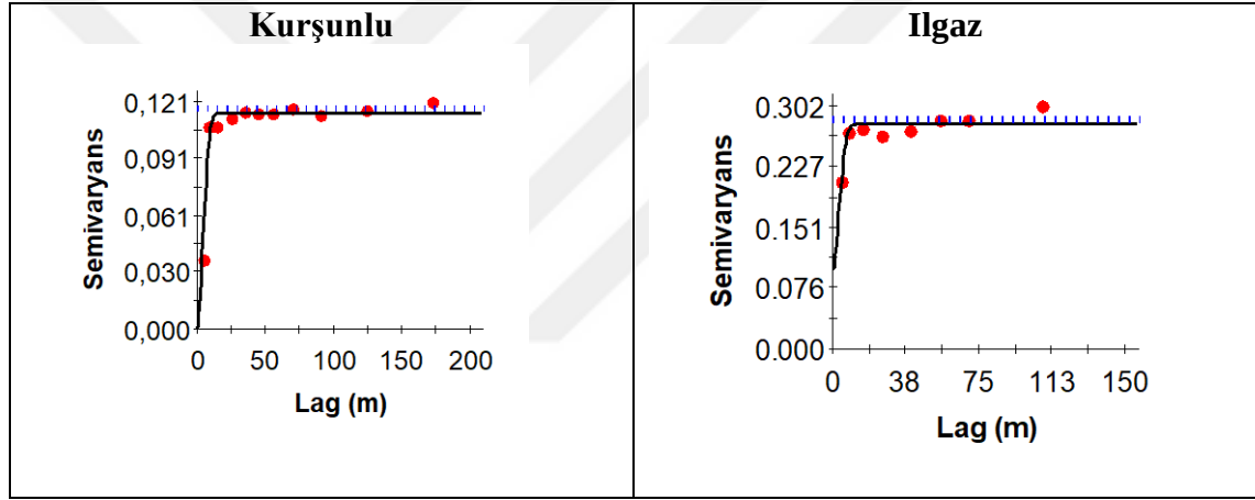
Şekil 4. 37 Meralarda toprakların pH'sına ilişkin deneysel (küre) ve teorik (çizgi) semivaryogramları
