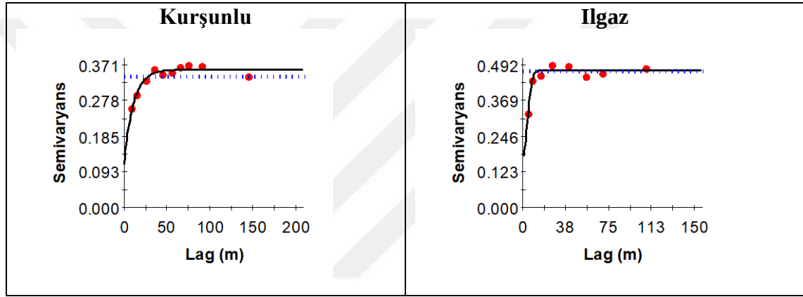
Şekil 4. 67 Meralarda toprakların Cu içeriğine ilişkin deneysel (küre) ve teorik (çizgi) semivaryogramları
