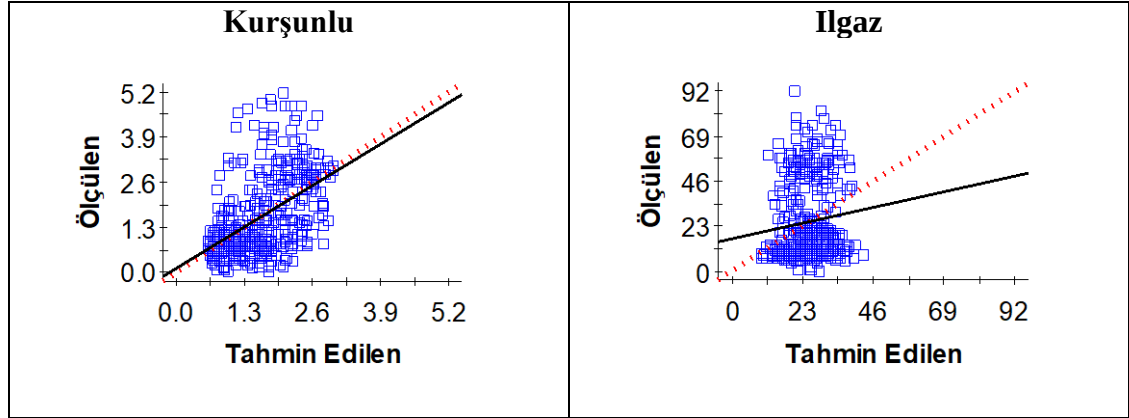
Şekil 4. 65 Kurşunlu merası toprakların Fe içeriğine ilişkin çapraz doğrulama grafikleri
