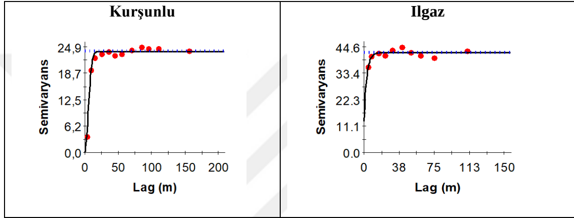
Şekil 4. 25 Meralarda toprakların bitkiye yarayışlı su içeriğine ilişkin deneysel (küre) ve teorik (çizgi) semivaryogramları
