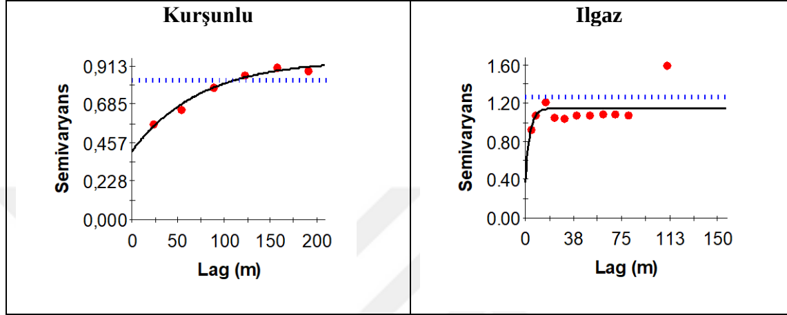
Şekil 4. 31 Mera toprakların CaCO 3 içeriğine (%) ilişkin deneysel (küre) ve teorik (çizgi) semivaryogramları
