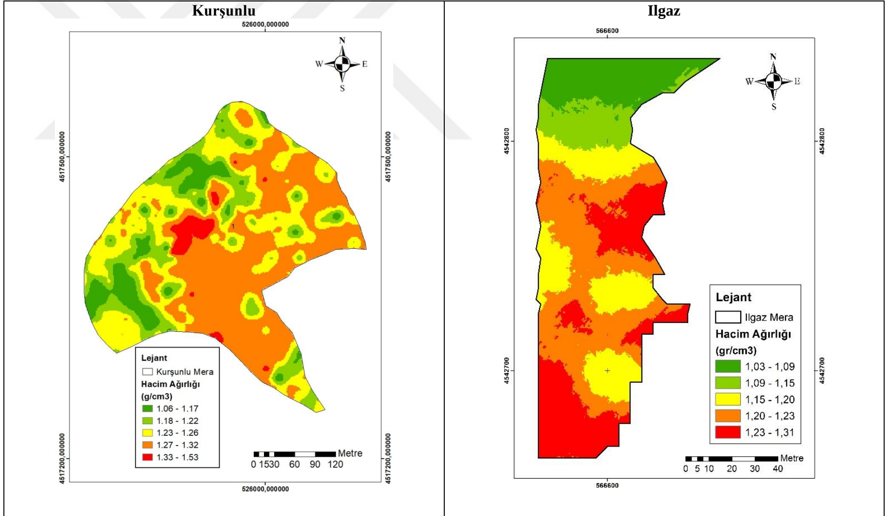
Şekil 4. 12 Hacim ağırlığının mera topraklarında uzaysal değişim deseni
