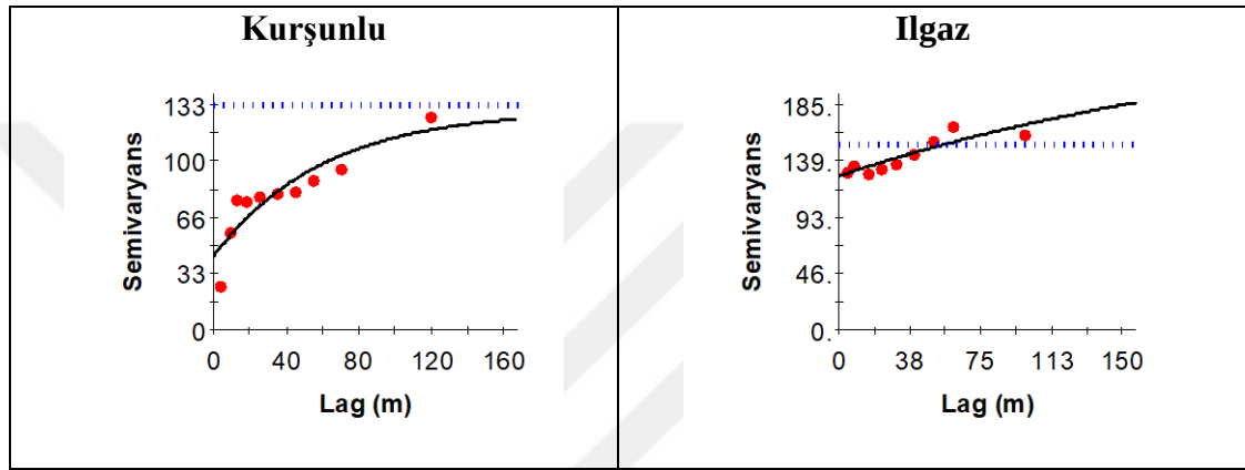
Şekil 4. 70 Meralarda toprakların Mn içeriğine ilişkin deneysel (küre) ve teorik (çizgi) semivaryogramları
