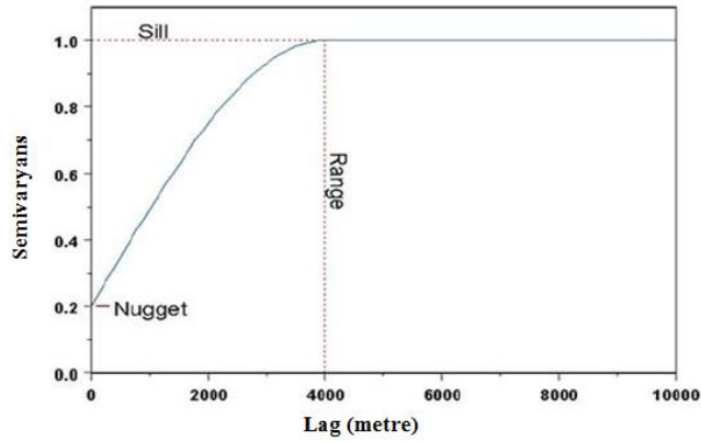
Şekil 3 9 Tipik bir semivaryogram ve bileşenleri
