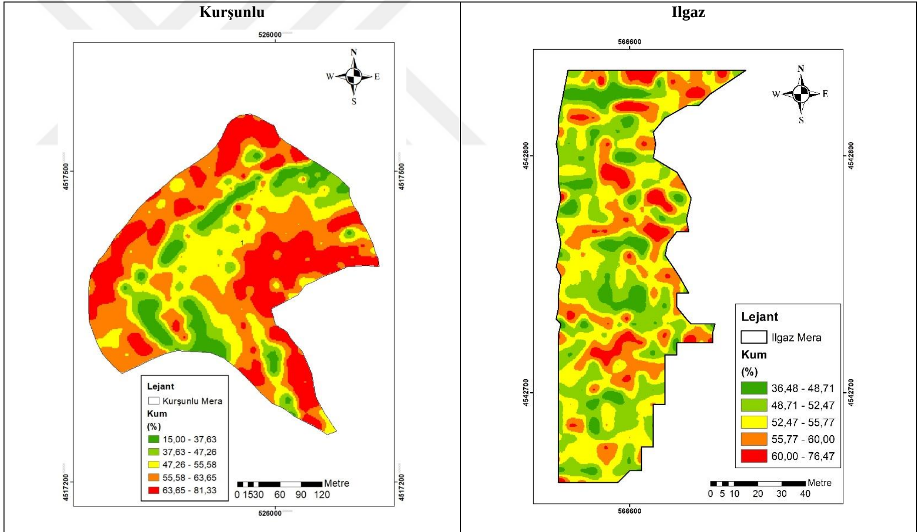
Şekil 4. 3 Kum içeriğinin mera topraklarında uzaysal değişim deseni
