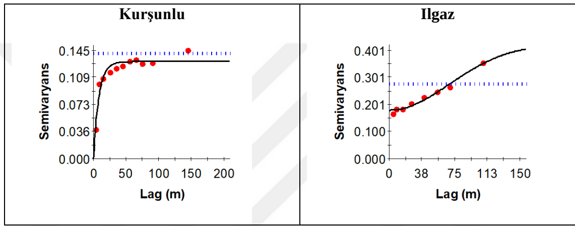
Şekil 4. 43 Meralarda toprakların penetrasyon direncine ilişkin deneysel (küre) ve teorik (çizgi) semivaryogramları
