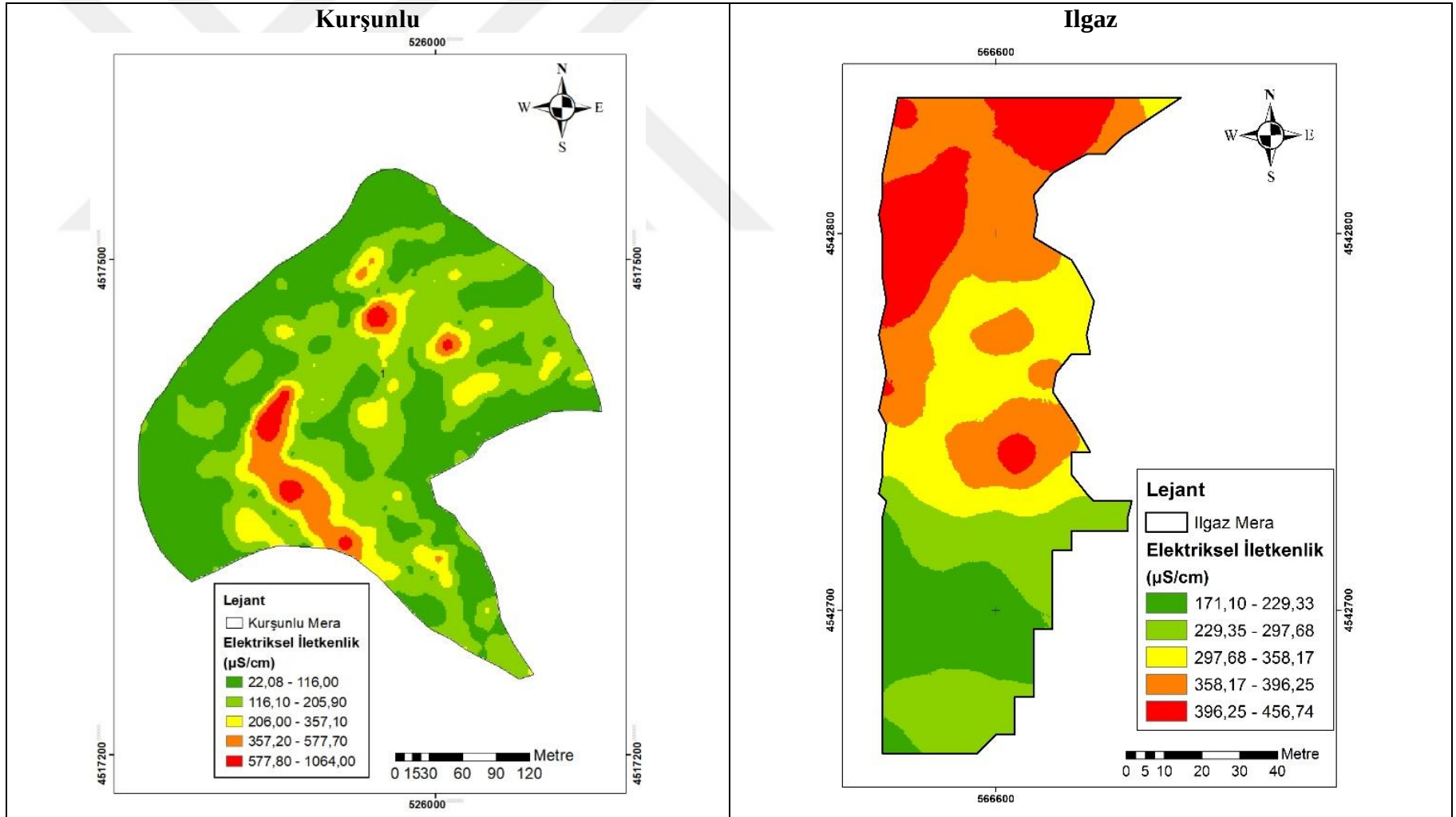
Şekil 4. 42 Elektriksel iletkenliğin mera topraklarında uzaysal değişim deseni
