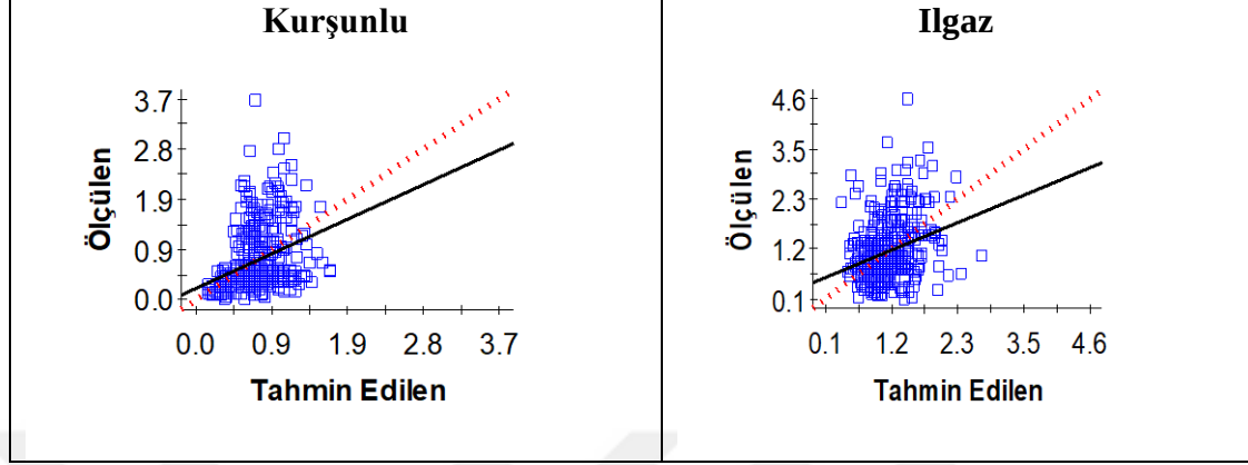
Şekil 4. 68 Mera toprakların Cu içeriğine ilişkin çapraz doğrulama grafikleri
