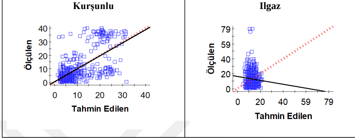
Şekil 4. 71 Mera topraklarının Mn içeriğine ilişkin çapraz doğrulama grafikleri
