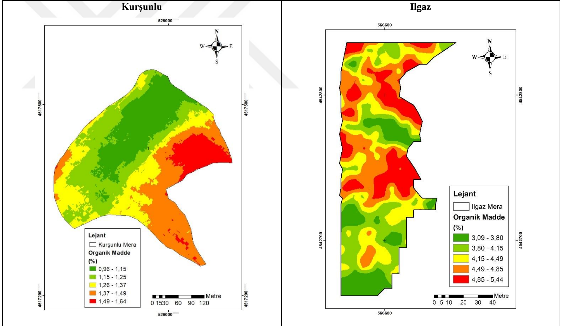
Şekil 4. 36 Organik madde içeriğinin mera topraklarında uzaysal değişim deseni
