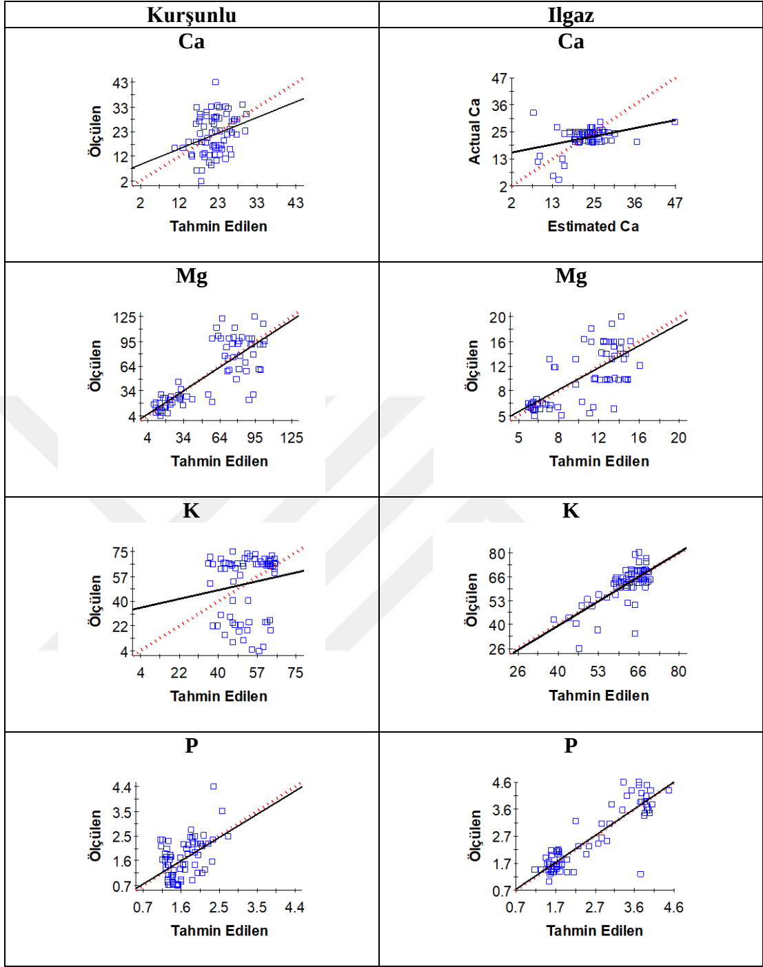
Şekil 4. 77 Mera bitki örneklerinin makro besin elementi içeriklerine ilişkin çapraz doğrulama grafikleri
