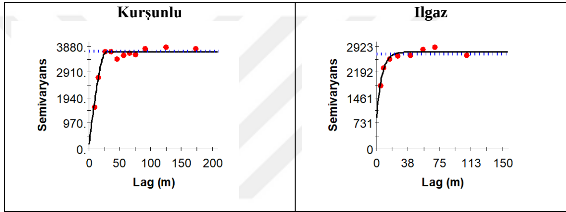
Şekil 4. 52 Meralarda toprakların K içeriğine ilişkin deneysel (küre) ve teorik (çizgi) semivaryogramları
