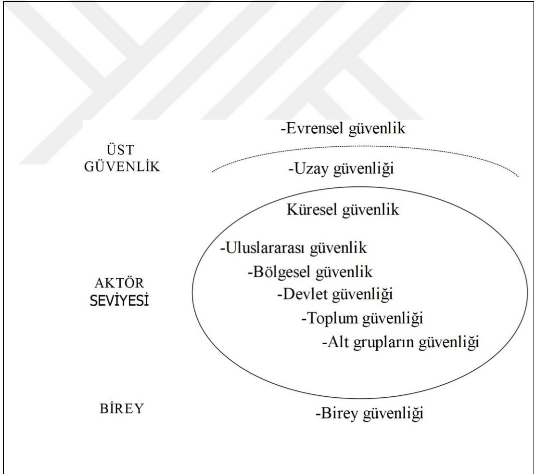
Şekil 2.1: Güvenliğin Katmanları
