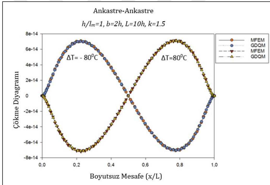
Şekil 4.11 Farklı \Delta T değerlerine göre hem MFEM hem de GDQM kullanılarak ankastrre-ankastrre FD mikro kirişlerinin çökme değişimi
