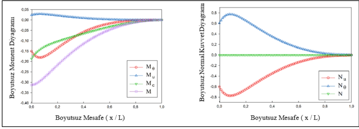
Şekil 4.7 Ankastre-Serbest mesnetli FD mikro kirişlerin boyutsuz moment ve normal kuvvet diyagramları
