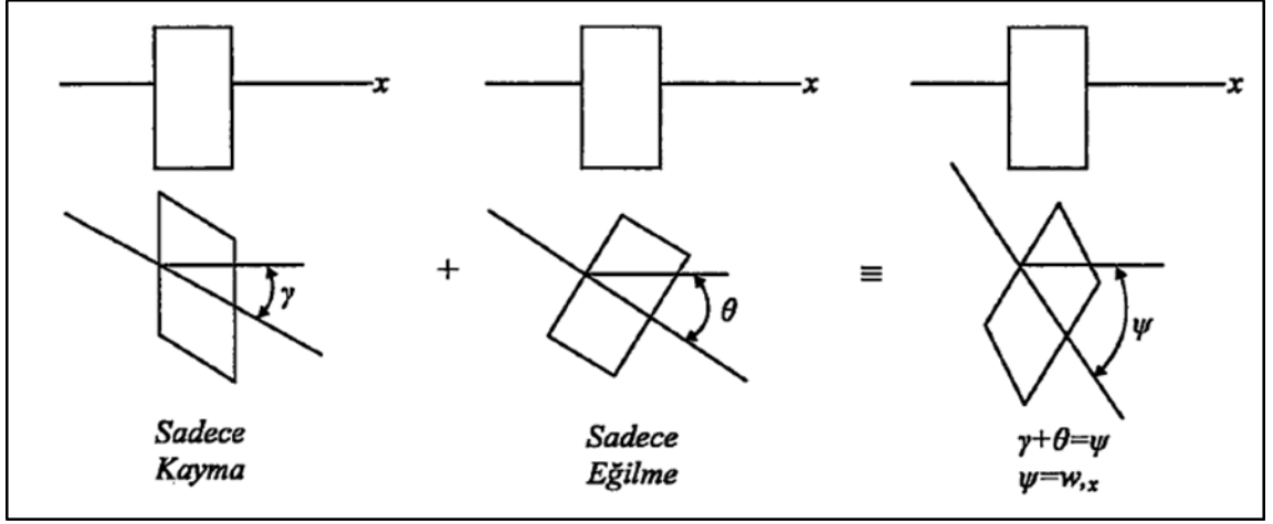
Şekil 2.5 Timoshenko kirişinde şekil değişiminin süperpozisyonla elde edilşinin geometrik gösterimi [90]
