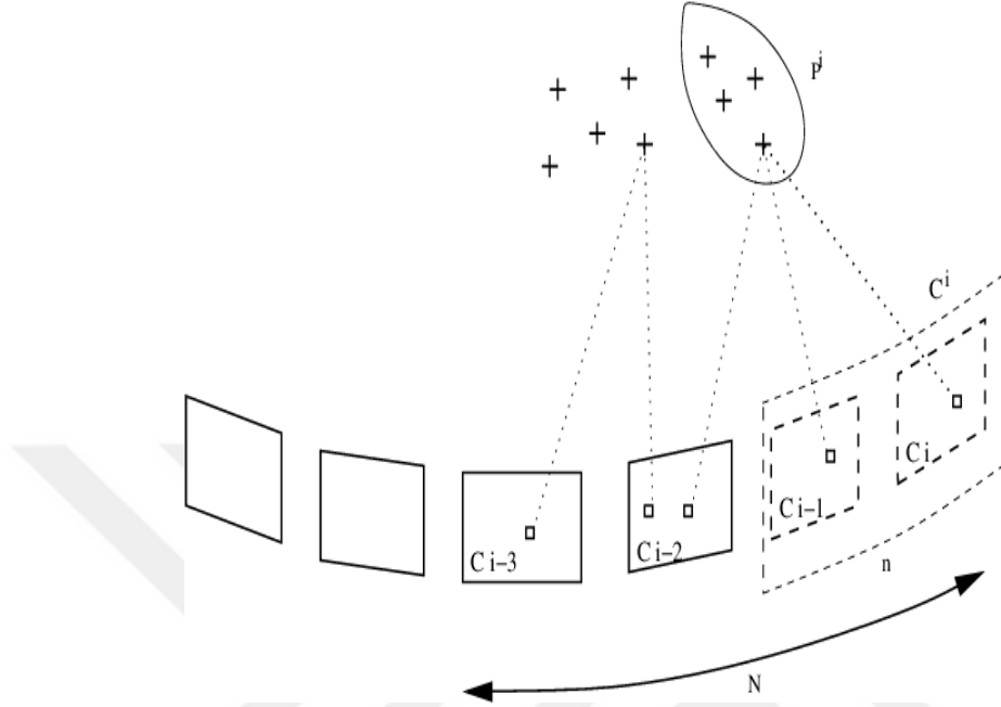
Şekil 3.7: 3 boyutlu noktaların farklı kamera düzlemlerine yansımaları (Mouragnon vd., 2006).
