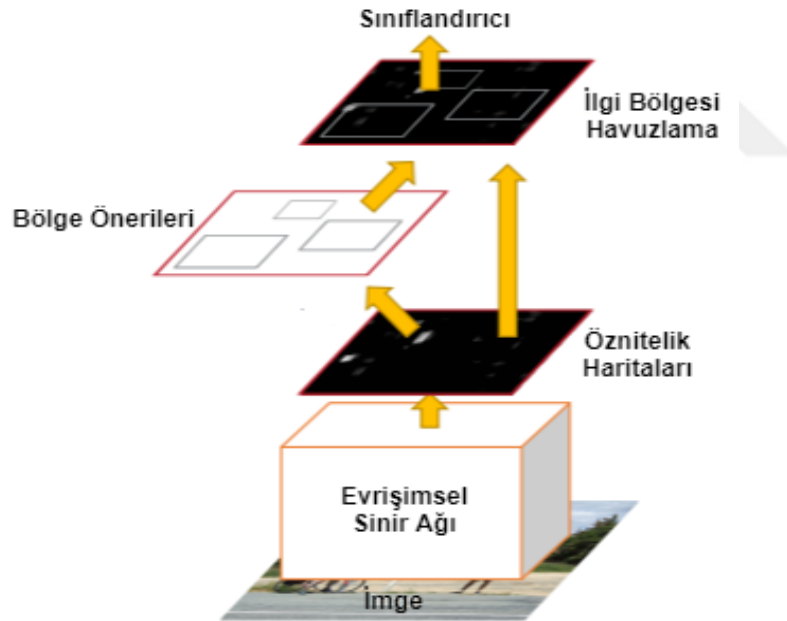
Şekil 2.3: Bölge önerici ağ ile nesne tespiti (Ren vd., 2015).
