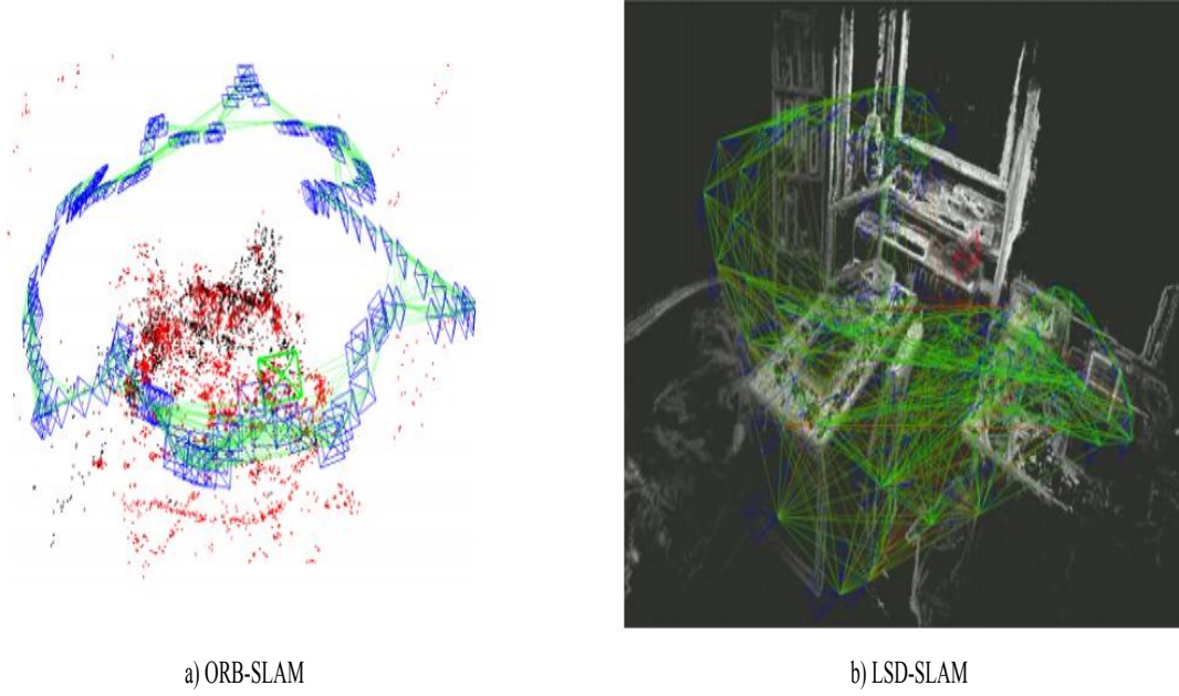
Şekil 2.1: Sol tarafta ORB-SLAM ile oluşturulan seyrek nokta bulutu, sağ tarafta ise LSD-SLAM ile oluşturulan yoğun nokta bulutu gösterilmektedir.
