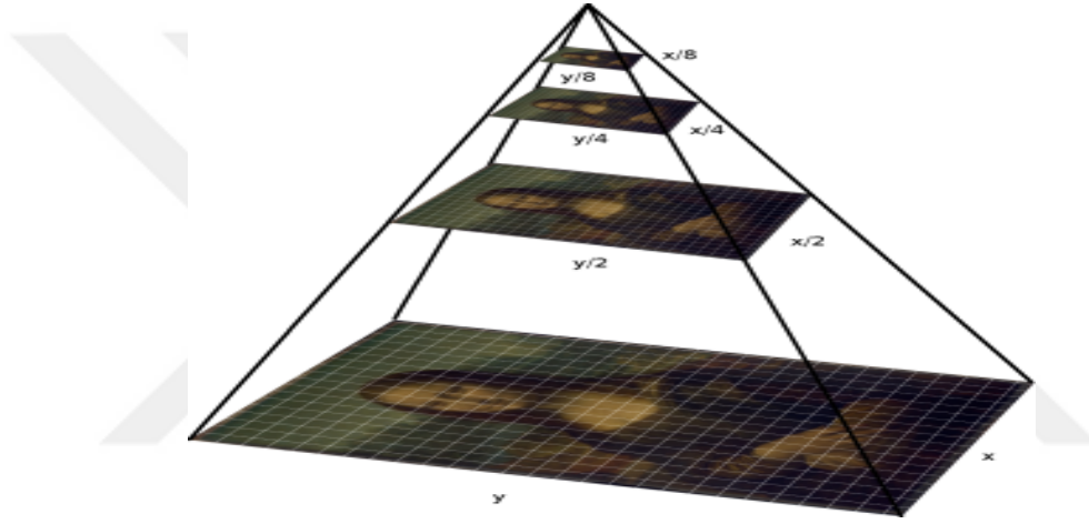
Şekil 3.2: İmge piramidi.
