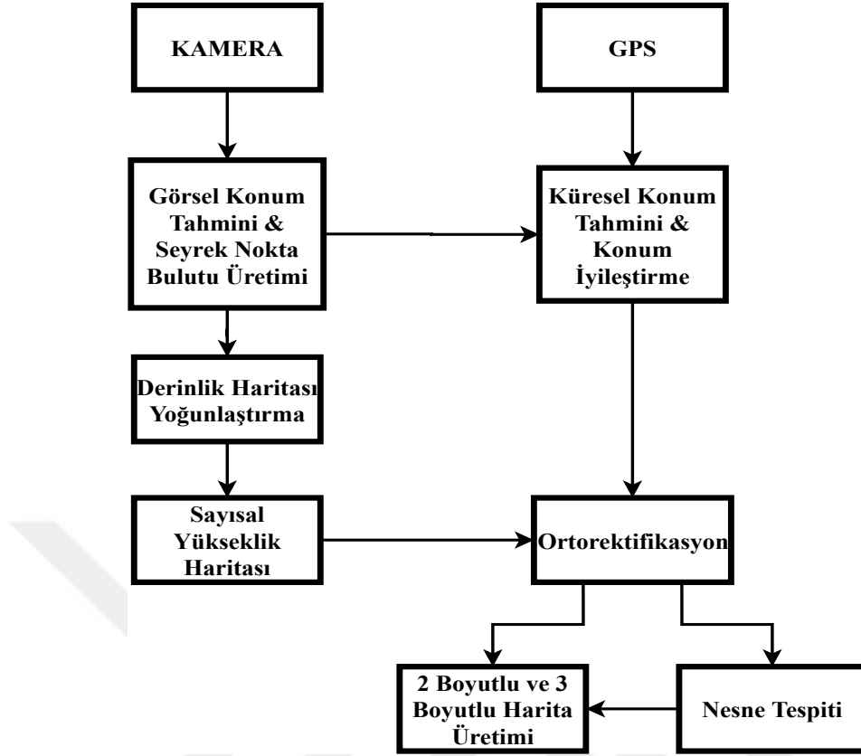
Şekil 3.9: Haritalama ve konumlandırma yönteminin adımları.
