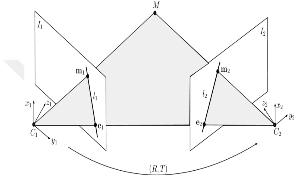
Şekil 3.6: Epipolar geometri.
