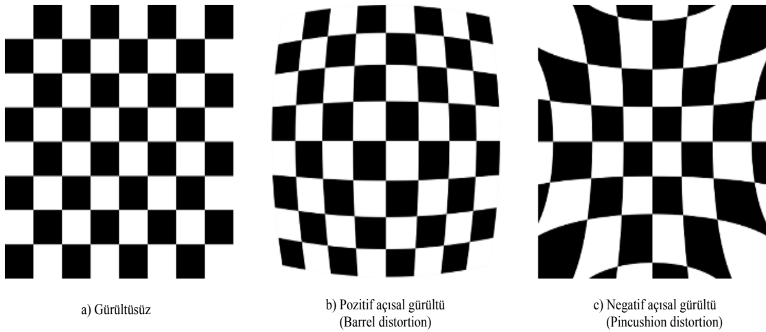
Şekil 3.5: Lens gürültüleri.
