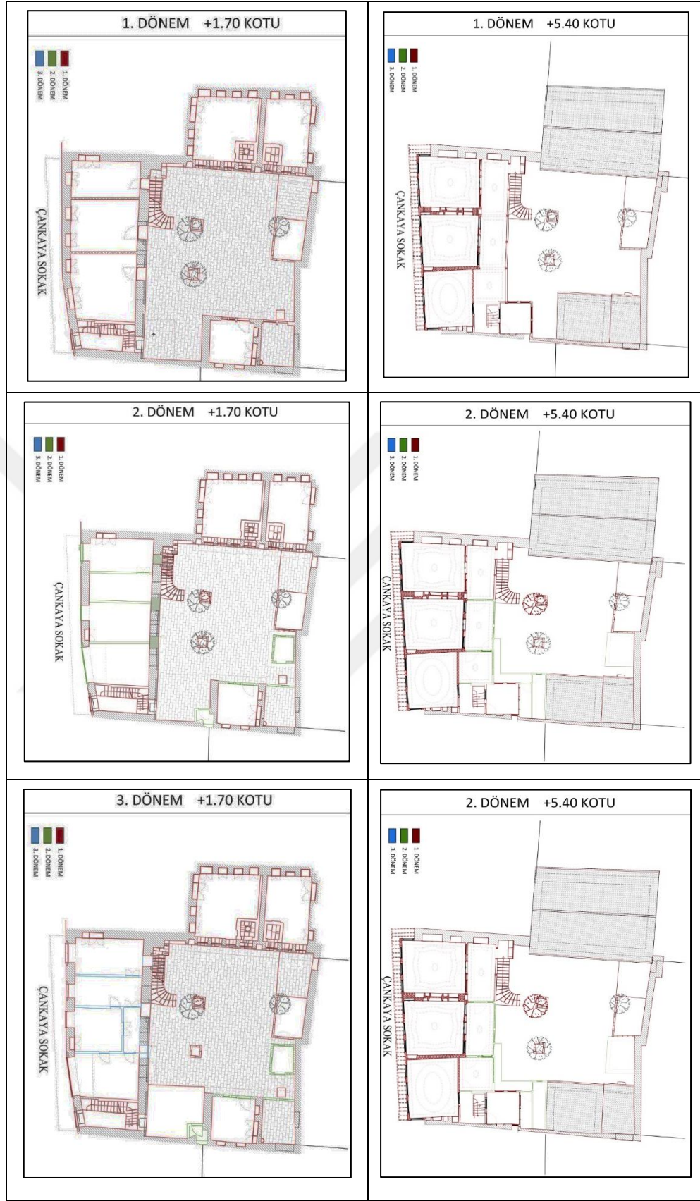
Şekil 3.61 Geleneksel avlulu ev (1339 Parsel) zemin ve üst kat mimari özellikleri (Sırım, 2015)
