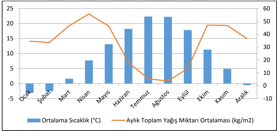
Grafik 4: Van’ın aylara göre yağış ve sıcaklık durumu.
