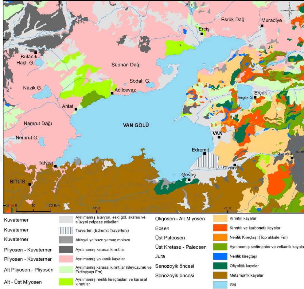
Harita 4: Van Gölü Havzası'nın jeomorfolojisi.
