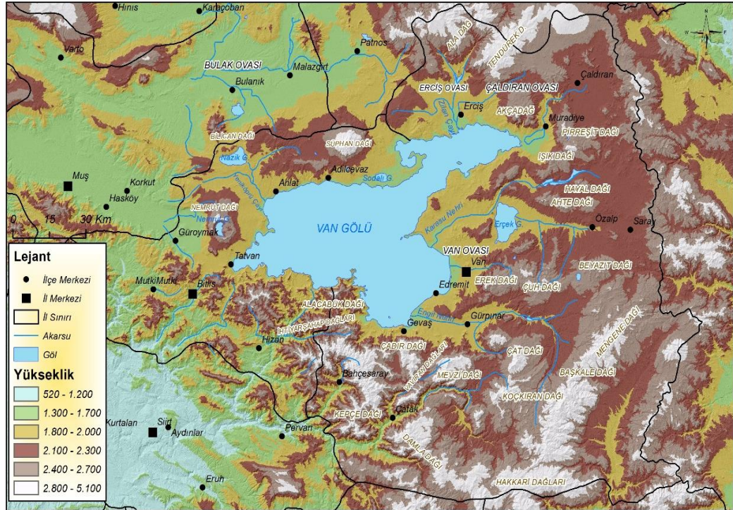
Harita 2: Van'ın topografyası.
