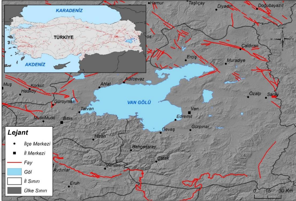
Harita 5: Van ve çevresindeki fayların dağılımı.
