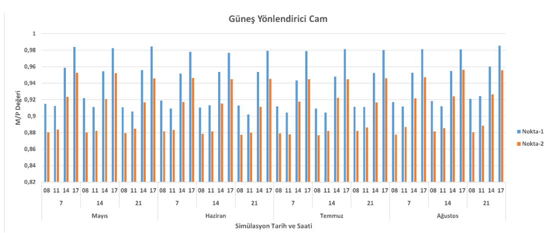
Şekil 42. Güneş yönlendirici cam M/P değerleri
