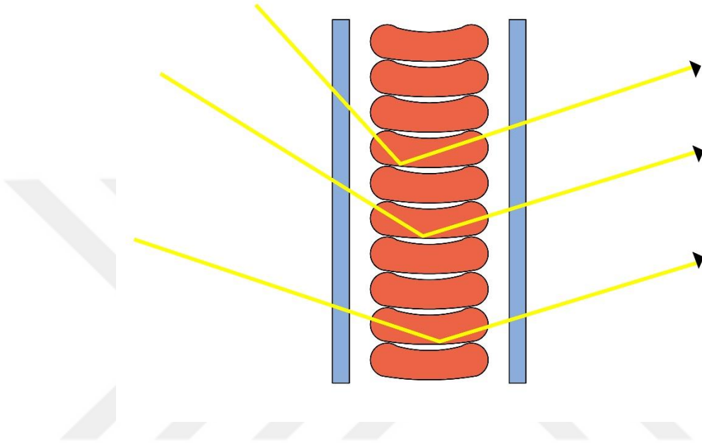
Şekil 13. Güneş yönlendirici cam çalışma prensibi
