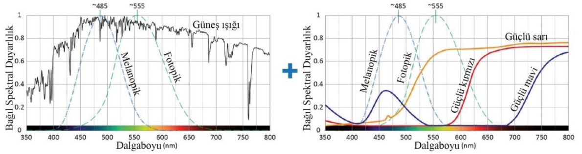
Şekil 24. IF ve NIF tepkilerinin spektral hassasiyetinin farklı ışık tipleri ile karşılaştırılması
