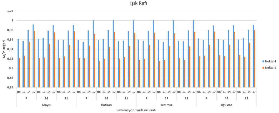
Şekil 39. Işık rafı M/P değerleri
