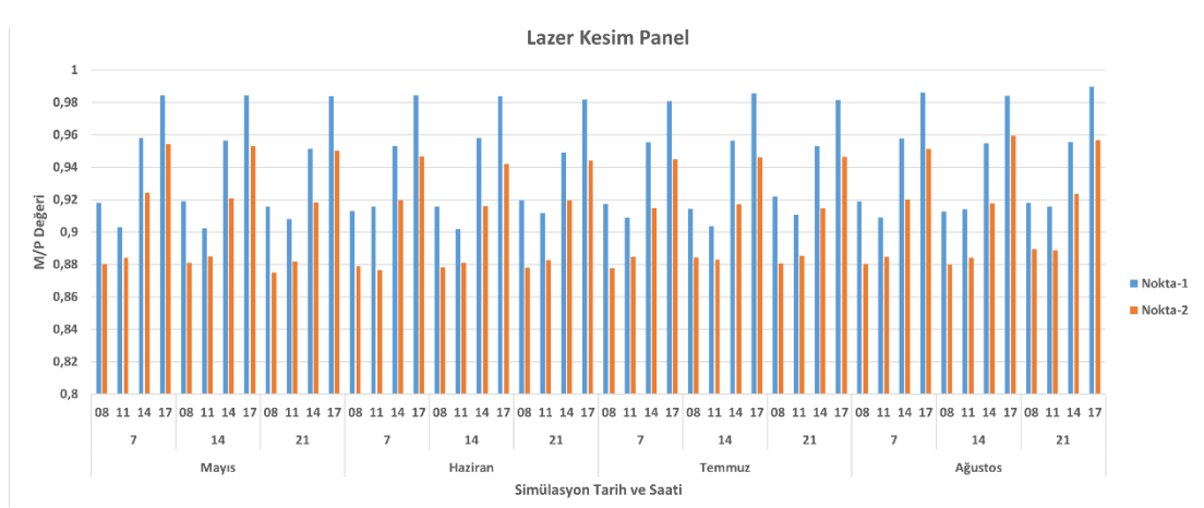
Şekil 41. Lazer kesim panel M/P değerleri
