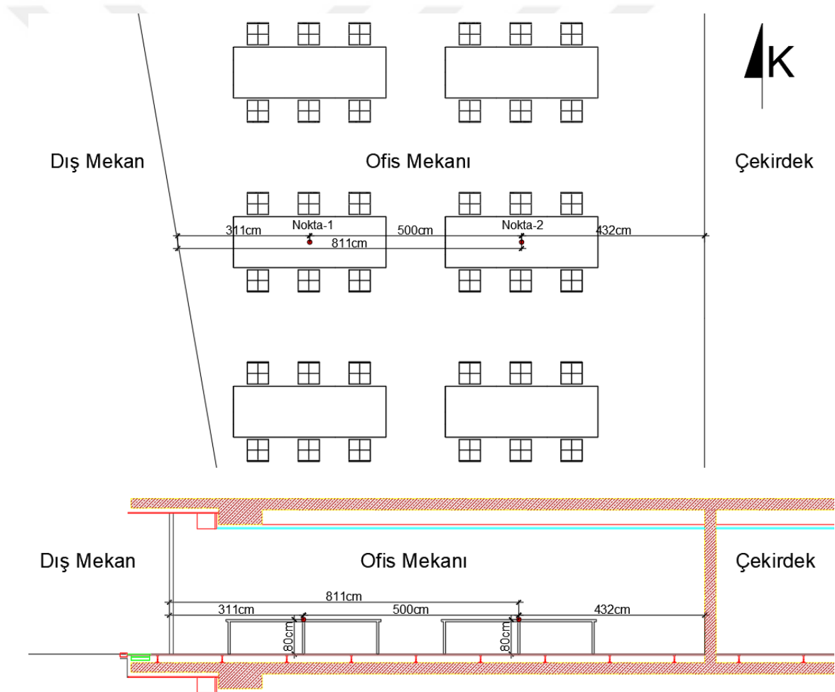
Şekil 38. M/P oranı ölçülen noktaların konumları
