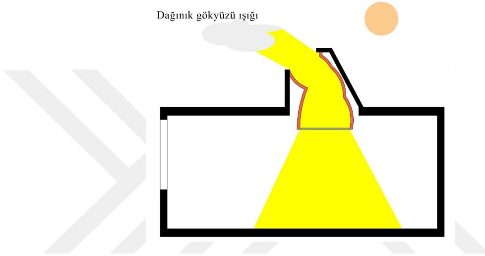
Şekil 17. Anidolik tavan sistemi şematik gösterimi
