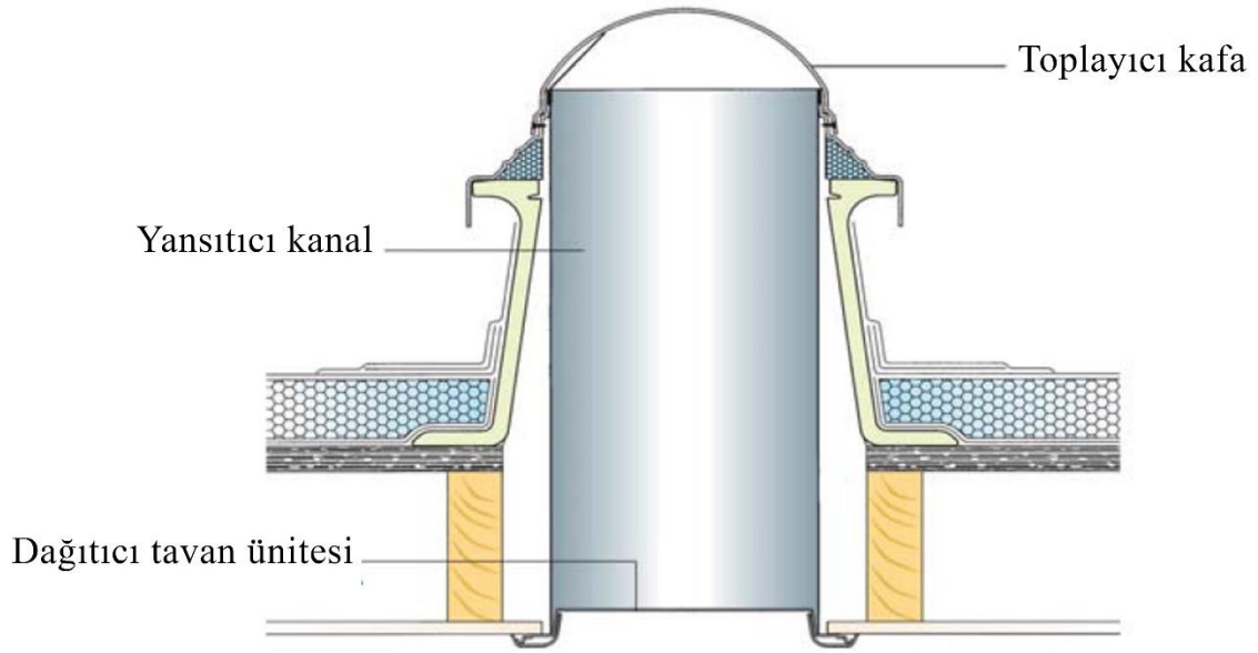
Şekil 21. Işık tüpü kesiti
