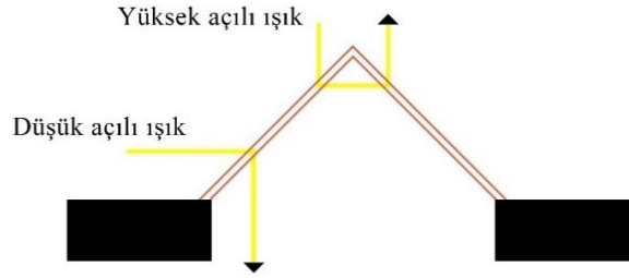
Şekil 12. Açısal seçici tavan penceresi çalışma prensibi
