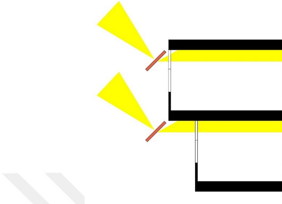
Şekil 15. Işık yönlendirici cam çalışma prensibi
