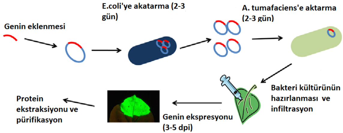
Şekil 2.4. Agroinfiltrasyon mekanizması
