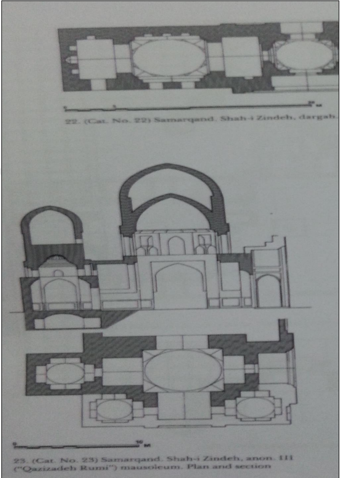
Şekil 7: Semerkand, Şâh-ı Zinde, (üstte) dergâh, (altta) Kadızâde-i Rûmî Türbe plânı (L. Golombek, D. Wilber, The Timurid Architecture of Iran and Turan , 1988).
