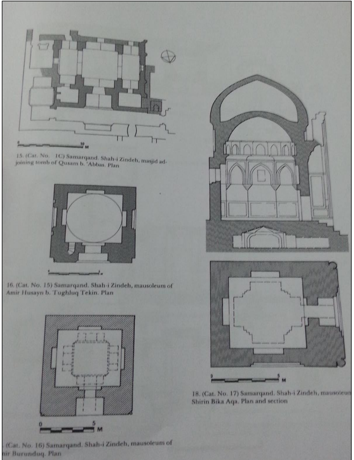
Şekil 5: Semerkand, (solda) Şâh-ı Zinde yapılarından üstten aşağıya doğru Kusem b. Abbas, Emîr Hüseyin b. Tuğluk Tekin ve Emir Burunduk, (sağda) ise Şîrin Bike Aka türbelerine ait plânlar var (L. Golombek, D. Wilber, The Timurid Architecture of Iran and Turan , 1988).
